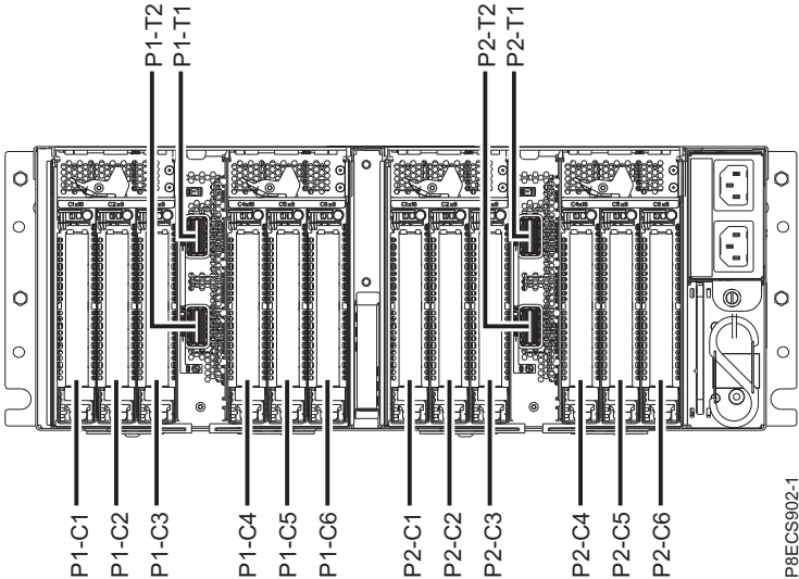
Рисунок 2. Блок расширения EMX0 PCIe3 (вид сзади) с кодами расположения разъемов PCIe
