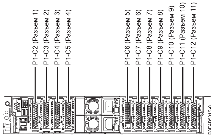
Рисунок 1. Смонтированный в стойке сервер 5148-21L, 5148-22L, 8247-21L,8247-22L,8284-21A или 8284-22A - вид сзади с кодами расположения разъемов PCIe.
