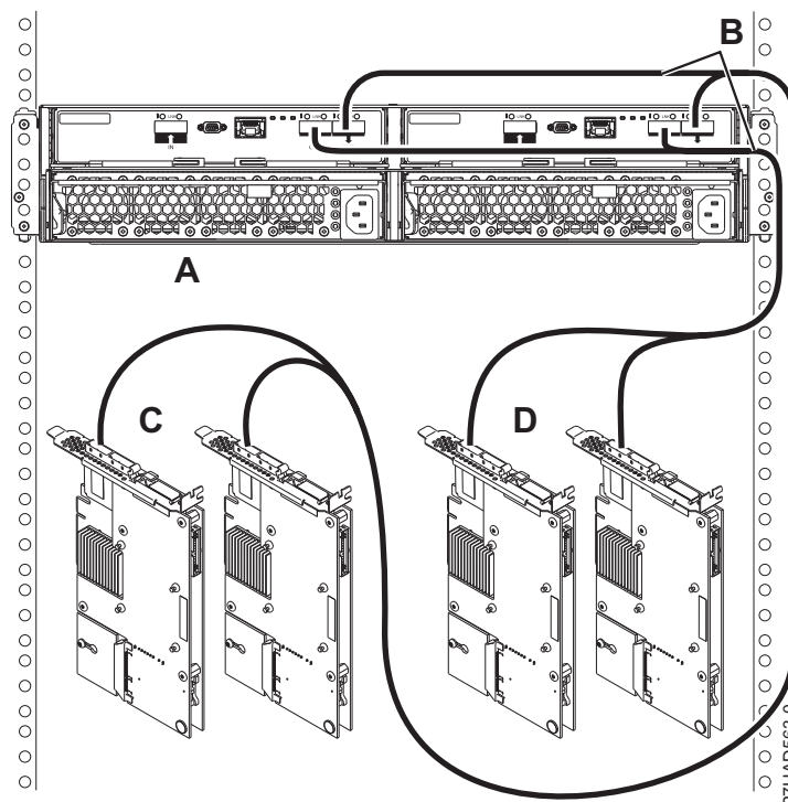
Figura 80. Două perechi de adaptoare FC 5805 sau FC 5903 la o incintă 5887 via o conexiune de mod 2.
