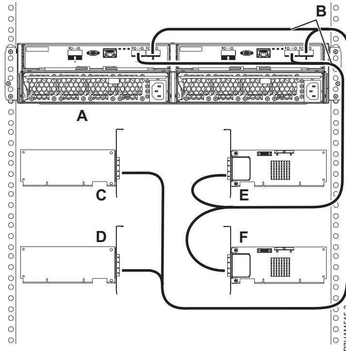
Figura 78. Conexiune de mod 4 a unei incinte 5887 utilizând cabluri X la patru adaptoare SAS simple
