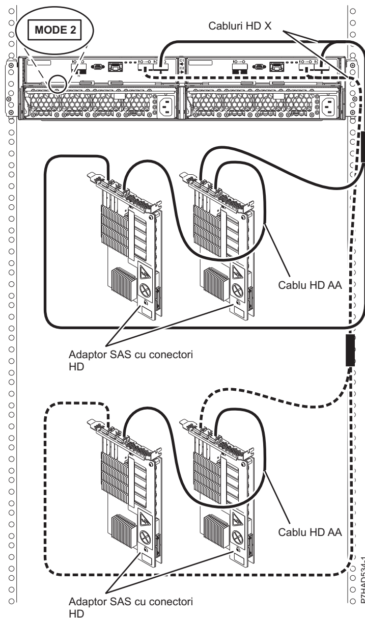
Figura 84. Conexiune de mod 2 a unei incinte 5887 utilizând cabluri HD la două perechi de adaptoare SAS PCIe2
