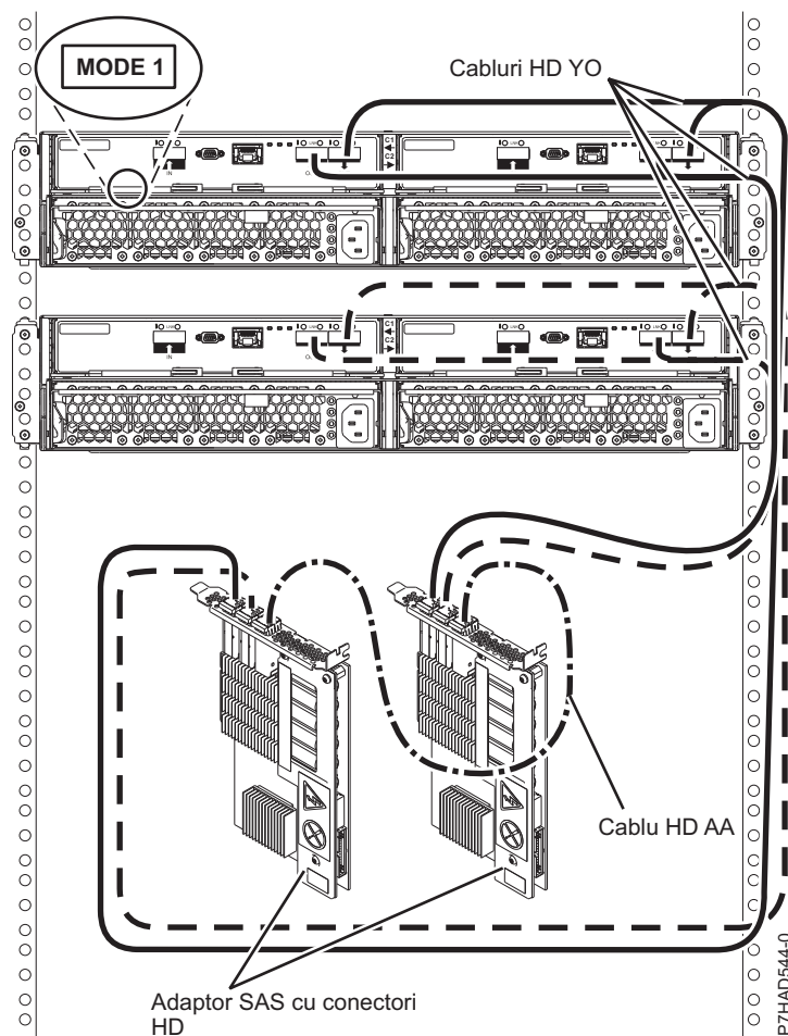
Figura 82. Conexiune mod 1 a două incinte 5887 folosind conectori HD la două adaptoare SAS PCIe2
