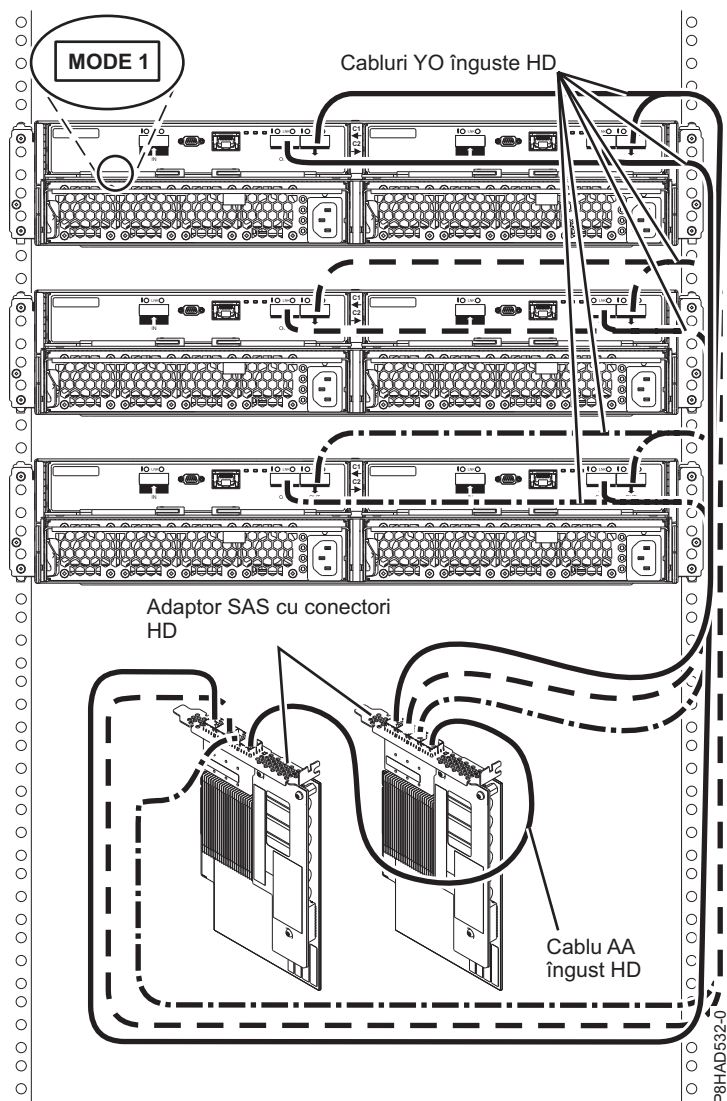
Figura 87. Conexiune mod 1 a trei incinte 5887 la două adaptoare SAS PCIe3 cu conectori înguști HD.
