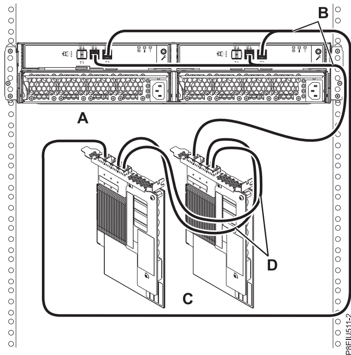
Figura 93. Conexiune de mod 1 a unui Incintă de stocare ESLL sau ESLS folosind cabluri YO12 la o pereche de adaptoare SAS
