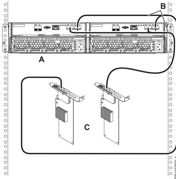
Figura 75. Conectarea de mod 1 a unei incinte 5887 utilizând cabluri YO la adaptoare SAS duale
