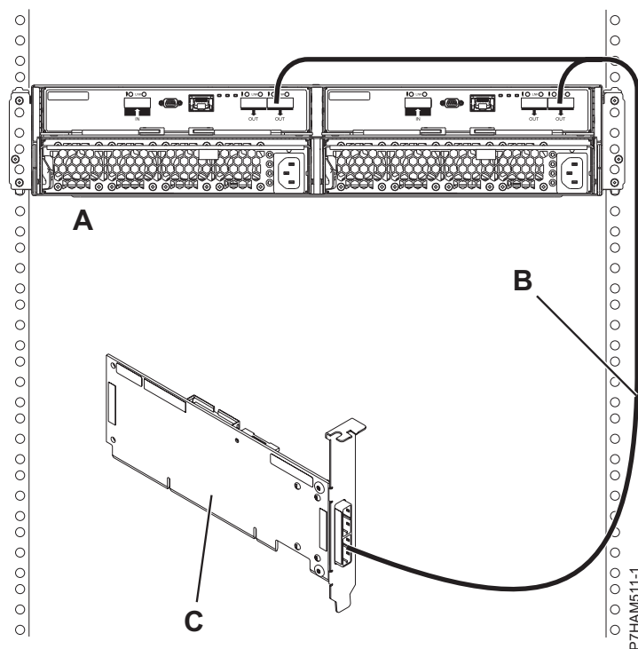
Figura 74. Conectarea de mod 1 a unei incinte 5887 utilizând un cablu YO la un singur adaptor SAS
