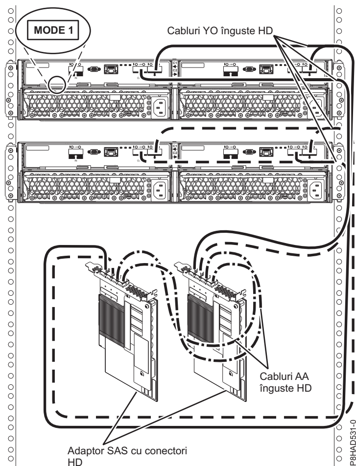
Figura 86. Conexiune mod 1 a două incinte 5887 la două adaptoare SAS PCIe3 cu conectori înguști HD.
