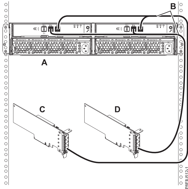
Figura 95. Conexiune de mod 2 a Incintă de stocare ESLL sau ESLS folosind cabluri YO12 la două adaptoare SAS independente
