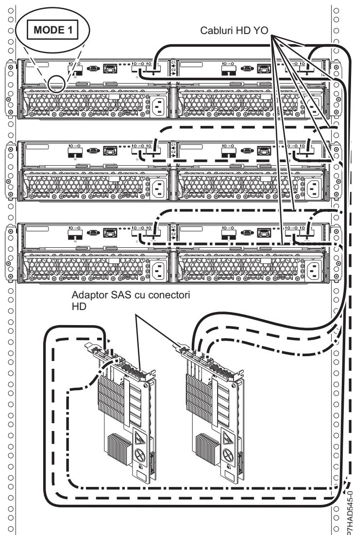
Figura 83. Conexiune mod 1 a trei incinte 5887 la două adaptoare SAS PCIe3 cu conectori HD
