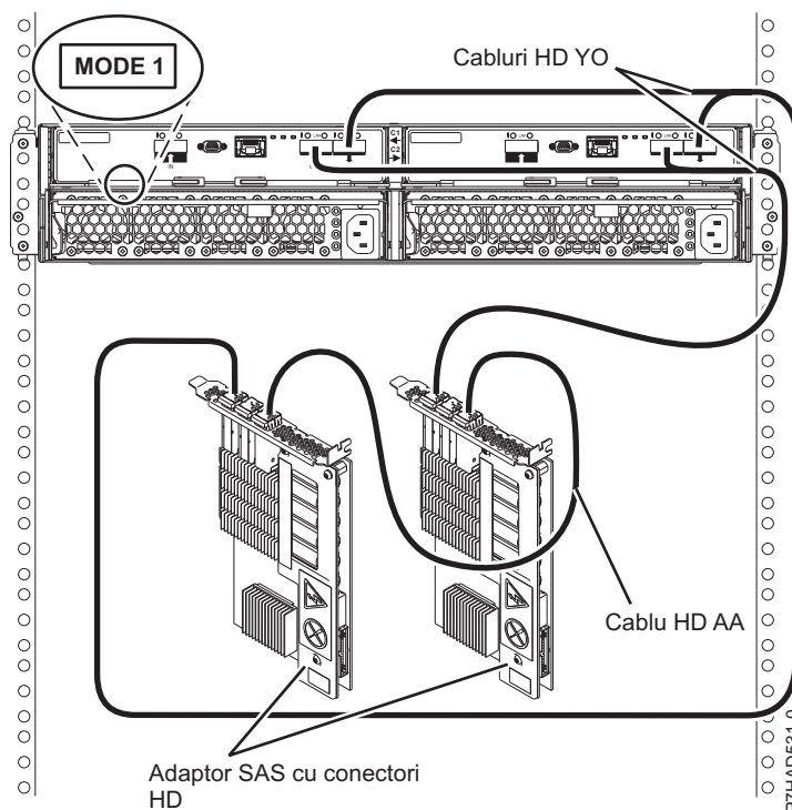
Figura 81. Conexiune mod 1 a unei incinte 5887 la două adaptoare SAS PCIe2 cu conectori HD
