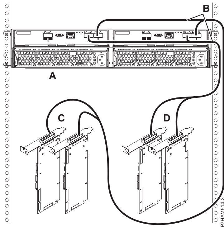
Figura 77. Conexiune de mod 2 a unei incinte 5887 utilizând cabluri X la două adaptoare SAS duble
