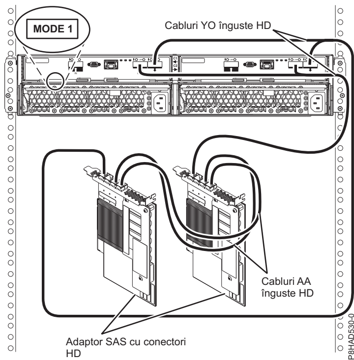
Figura 85. Conexiune mod 1 a unei incinte 5887 la două adaptoare SAS PCIe3 cu conectori înguști HD.
