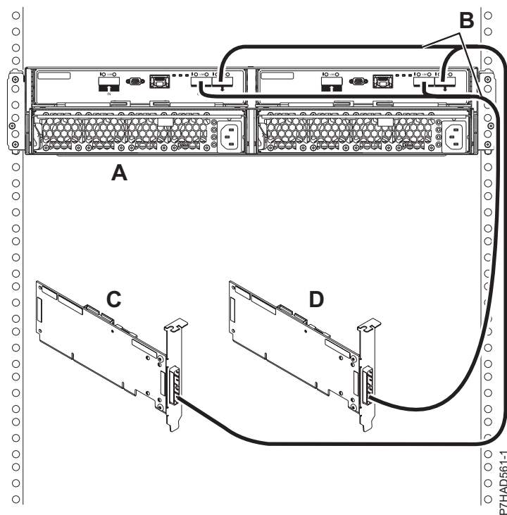
Figura 76. Conexiune de mod 2 a unei incinte 5887 utilizând cabluri YO la două adaptoare SAS simple
