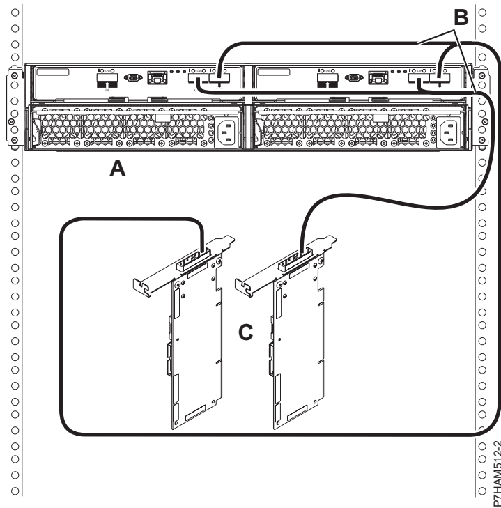
Figura 79. Conectarea de mod 1 a unei incinte 5887 utilizând cabluri YO la adaptoare SAS duale
