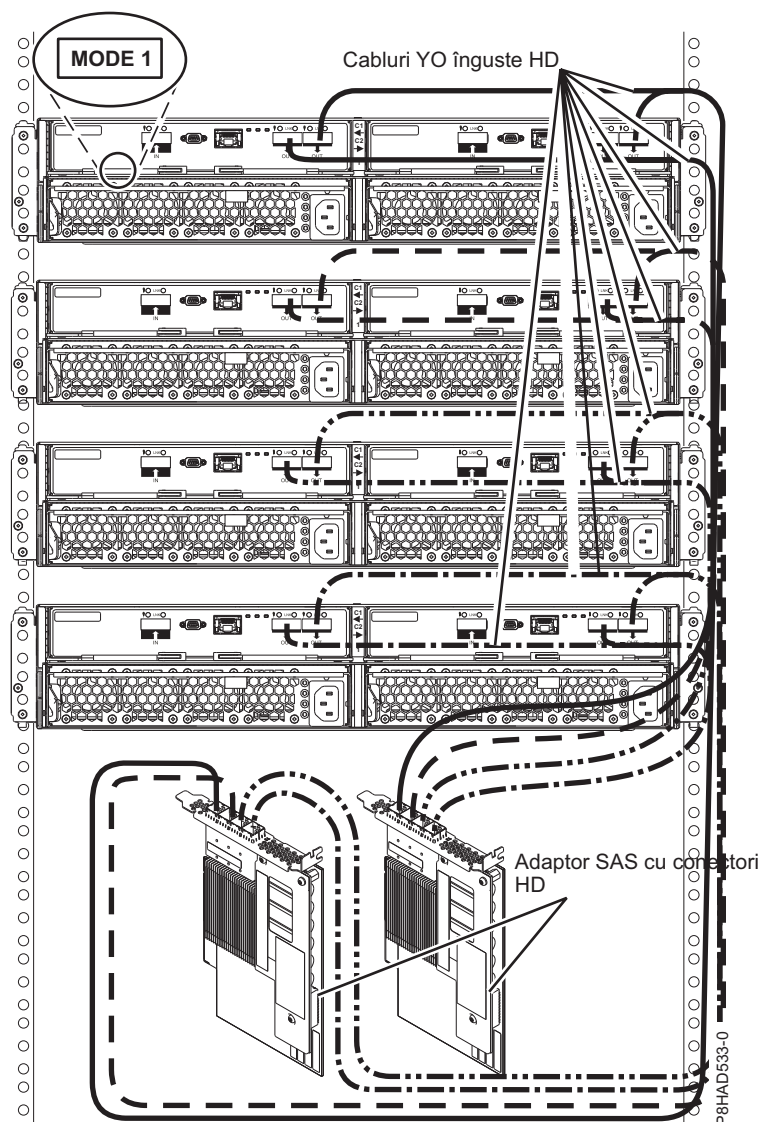
Figura 88. Conexiune mod 1 a patru incinte 5887 la două adaptoare SAS PCIe3 cu conectori înguști HD.
