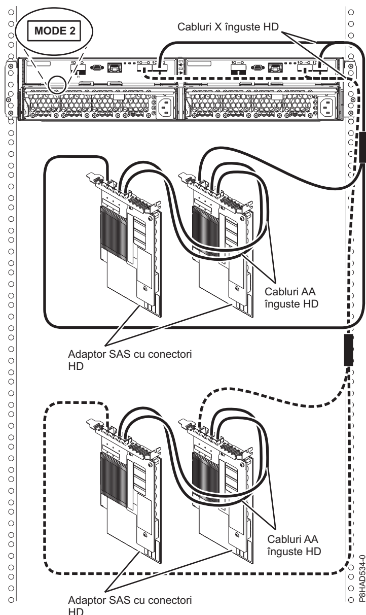
Figura 89. Conexiune mod 2 a unei incinte 5887 la două perechi de adaptoare SAS PCIe3 cu conectori înguști HD.
