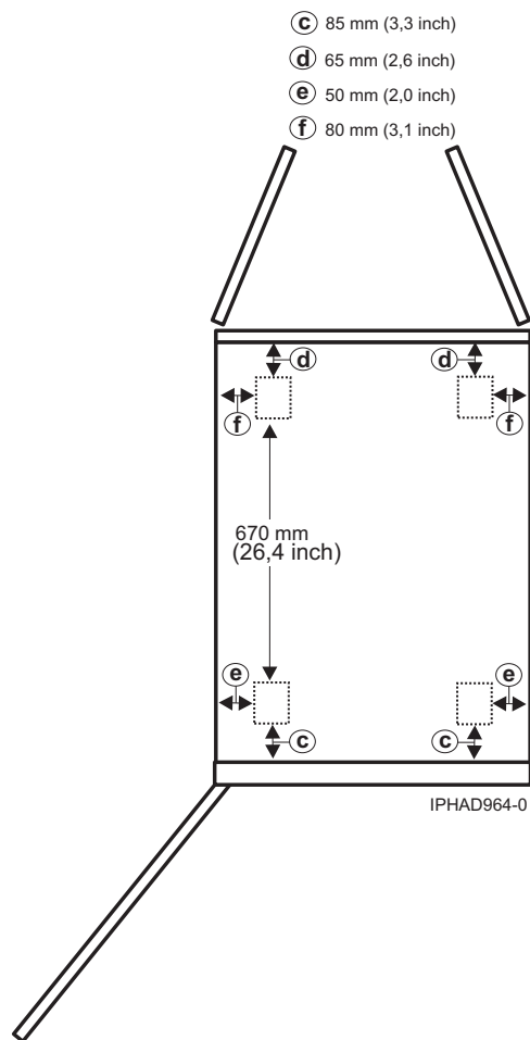
Figura 25. Locațiile roților pentru modelul 0555 și 7014-S25
