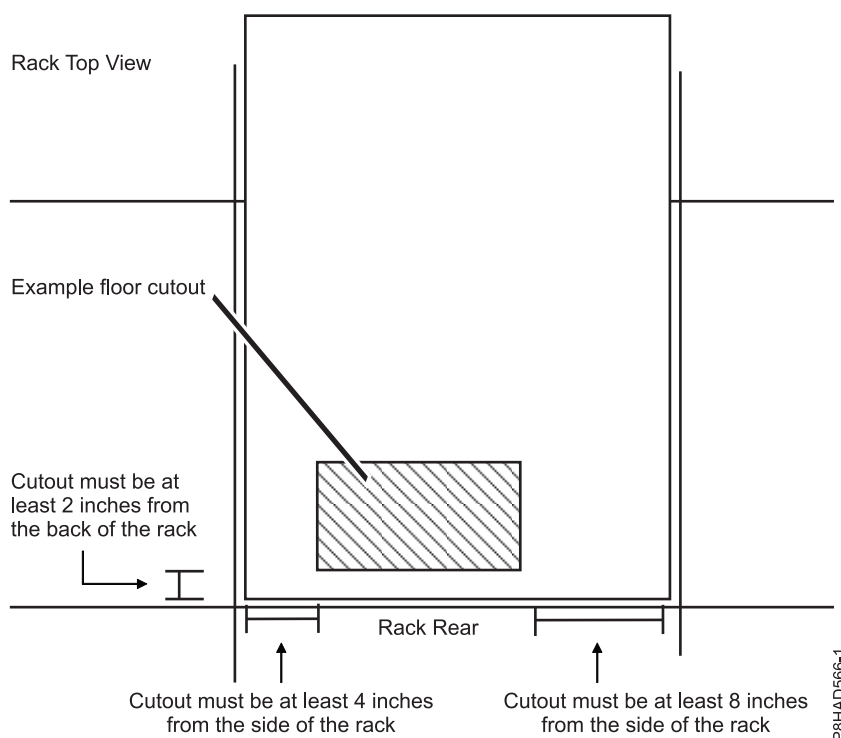
Figura 47. Decuparea în podea
