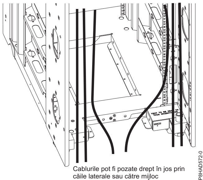
Figura 50. Cablarea sub podea
