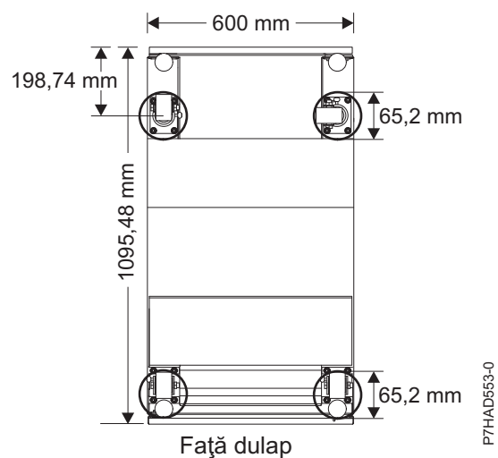
Figura 31. Locațiile roților
