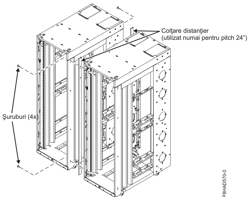
Figura 52. Unirea mai multor dulapuri
