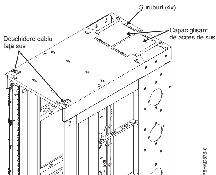
Figura 51. Proiectare cablare
