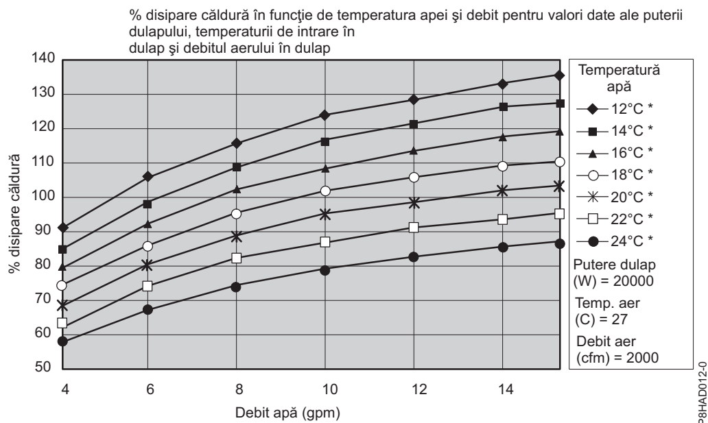
Figura 53. Performanța tipică a schimbătorului de căldură, 20 kW sarcină termică
