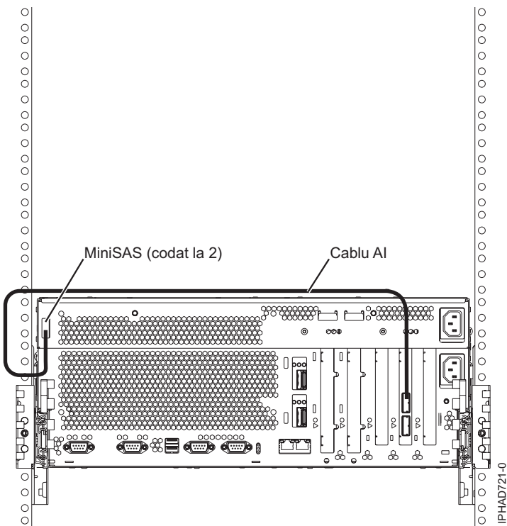
Figura 76. Adaptorul SAS la sloturi de disc SAS intern prin portul SAS extern al sistemului
