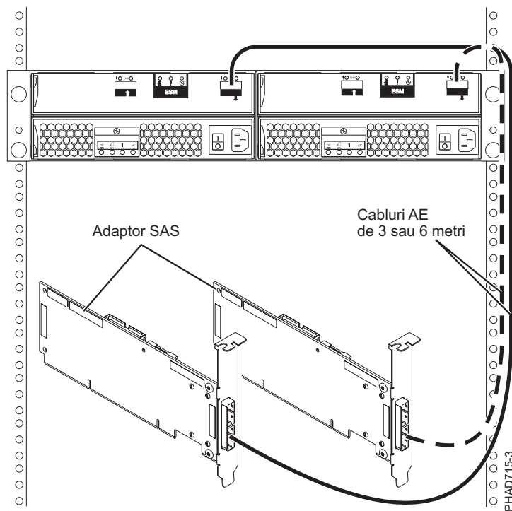
Figura 86. Două adaptoare SAS RAID la un sertar de expansiune pentru discuri într-o configurație JBOD HA inițializator multiplu
