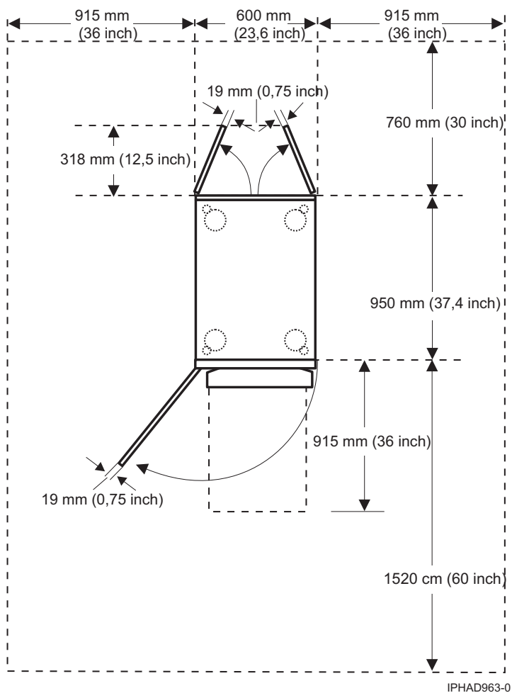
Figura 24. Vedere în plan pentru modelul 0555 și 7014-S25
