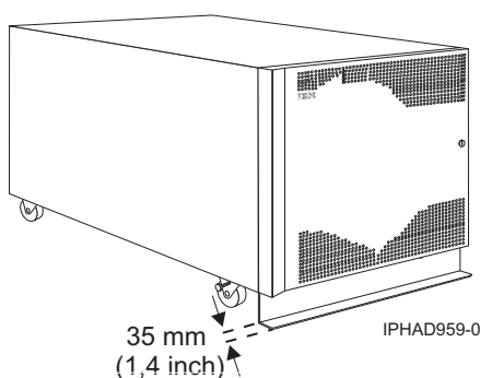
Figura 20. Modelul 0554 și 7014-S11 cu bară stabilizatoare
