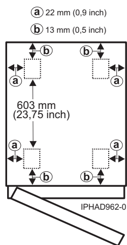
Figura 22. Locațiile roților pentru modelul 0554 și 7014-S11
