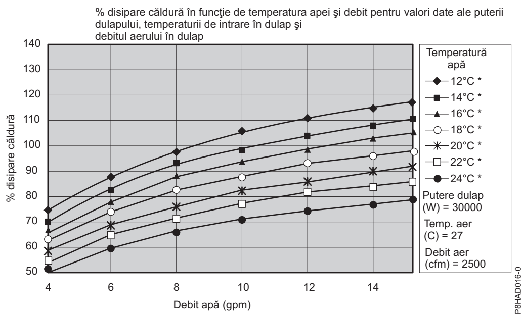
Figura 54. Performanța tipică a schimbătorului de căldură, 30 kW sarcină termică
