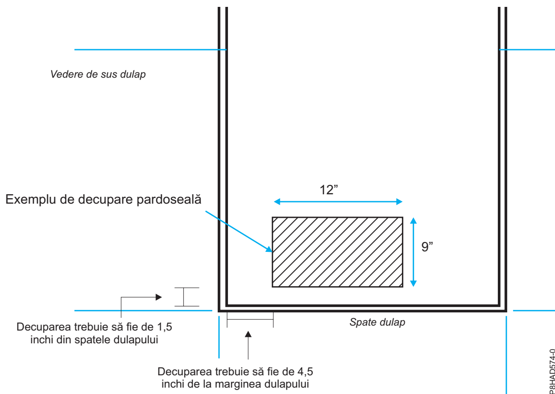
Figura 48. Decuparea în podea
