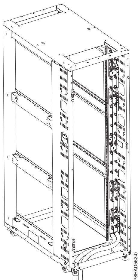
Figura 41. Dulapul și ansamblul furtunurilor de alimentare și retur ce ies prin partea de jos a dulapului
