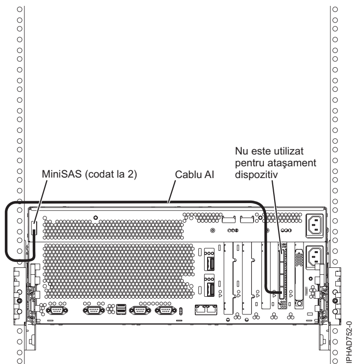
Figura 77. Adaptor FC5904 sau FC5908 atașat la sertare de expansiune pentru discuri
