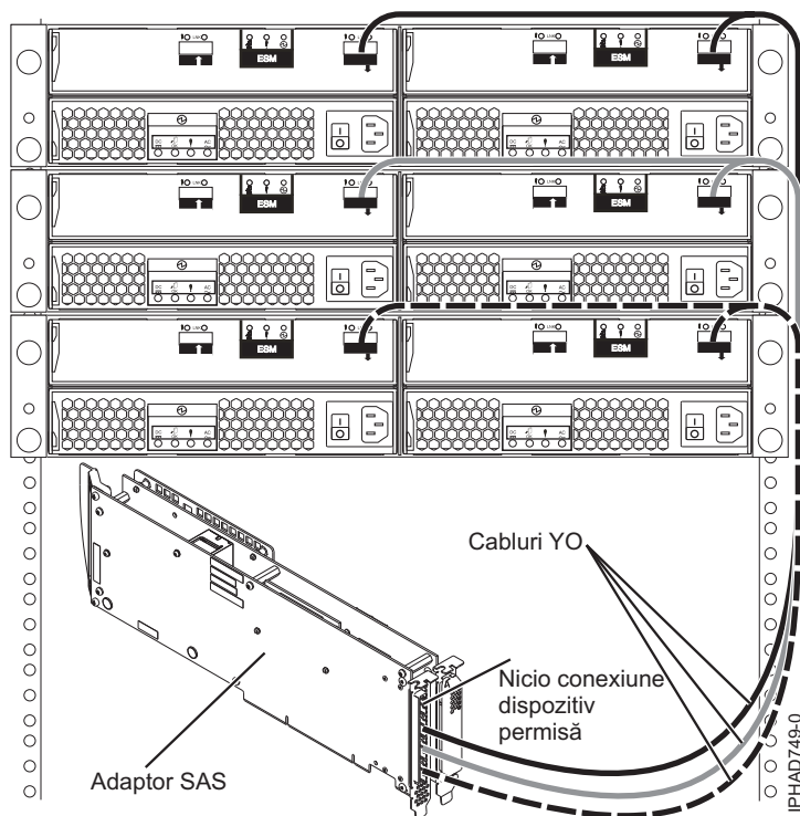
Figura 72. Adaptor SAS cu trei porturi la sertare de expansiune pentru discuri
