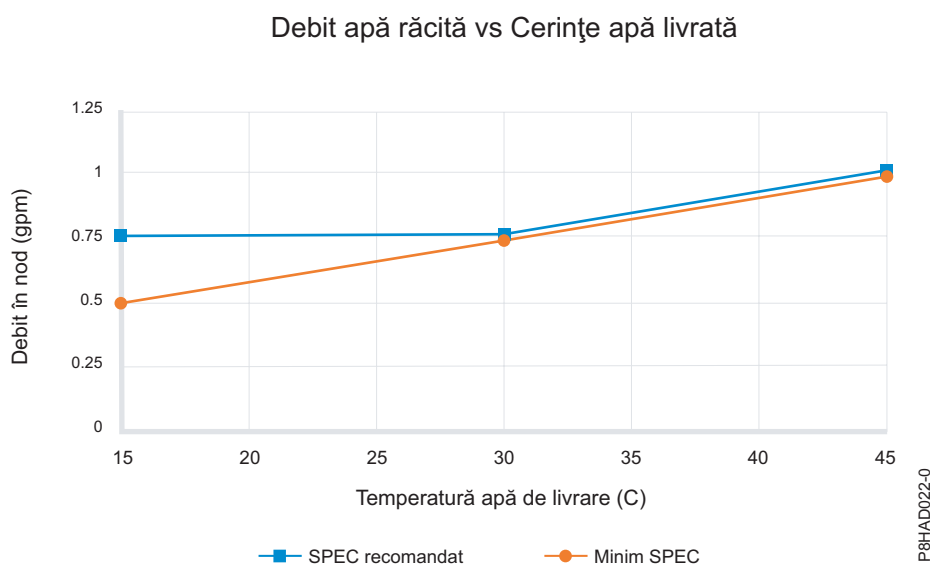
Figura 2. Debitul apei răcite versus cerințele apei de alimentare (unități standard)
