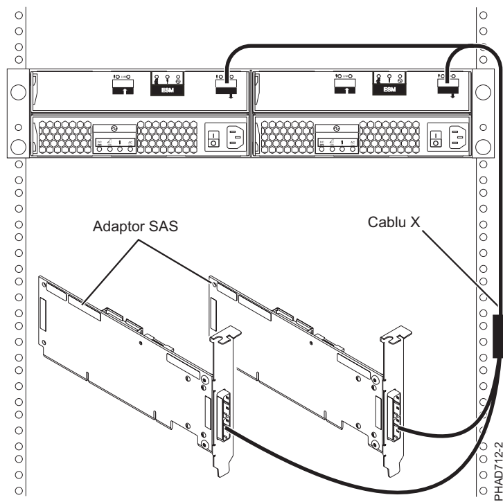
Figura 78. Două adaptoare RAID SAS la un sertar de expansiune pentru discuri într-o configurație RAID HA inițiator multiplu
