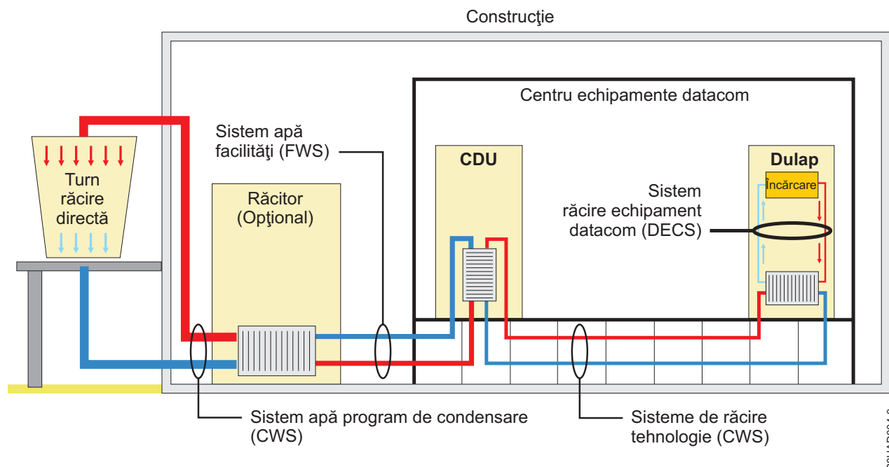
Figura 87. Exemplu de bucle și sisteme de răcire cu lichide într-un centru de date
