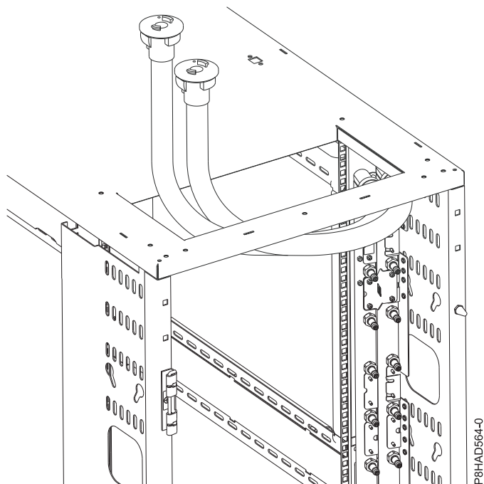
Figura 42. Locațiile de ieșire a furtunurilor în partea de sus
