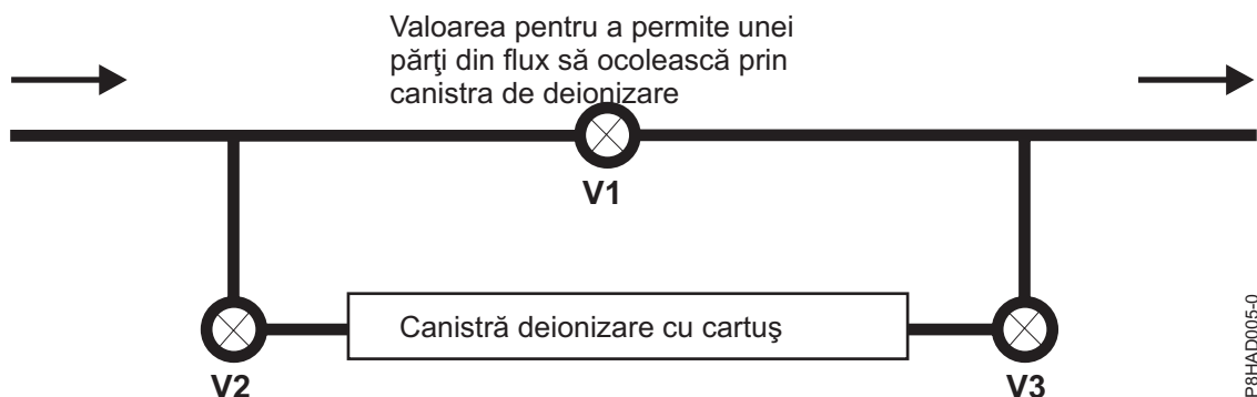
Figura 88. Deionizarea apei folosind cartușe de deionizare instalate în bucla de răcire
