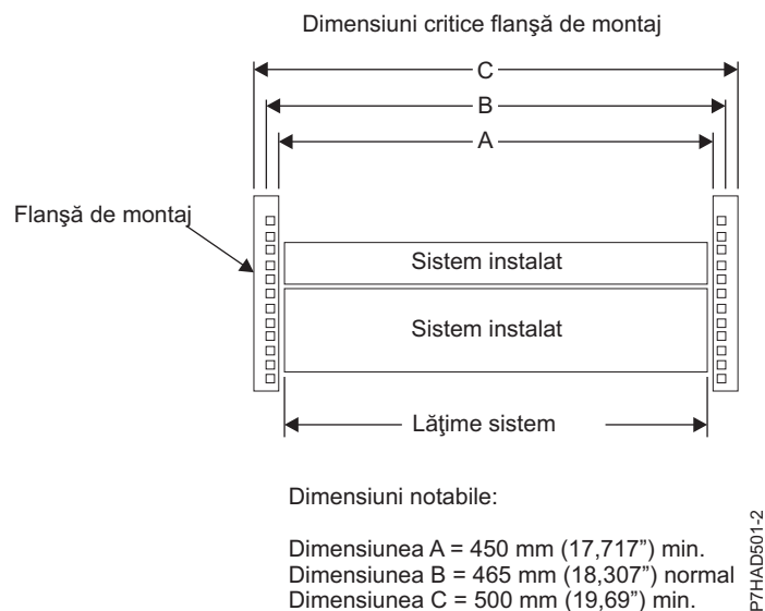
Figura 56. Dimensiuni de bordură de montare critice
