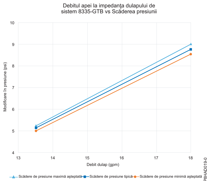
Figura 3. Debitul versus scăderea presiunii (unități standard) - Dulap plin cu 18 servere
