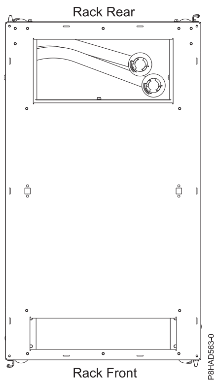
Figura 43. Locațiile de ieșire a furtunurilor în partea de sus (privind de sus)
