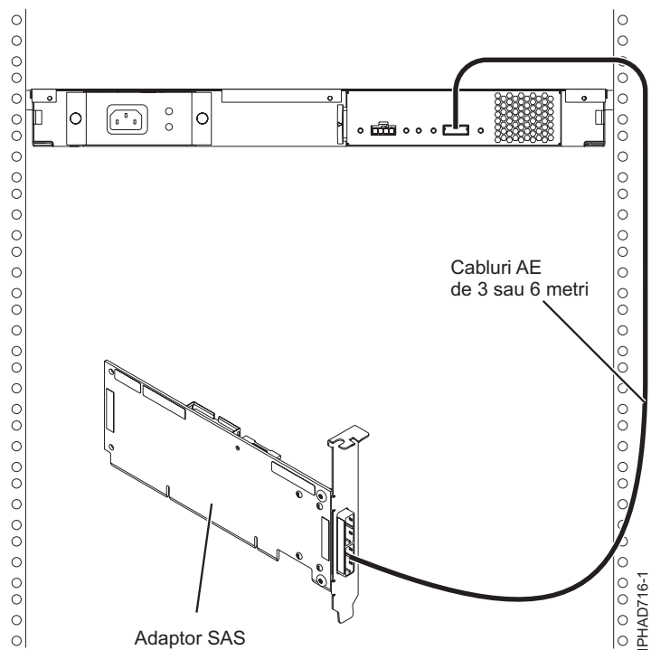
Figura 73. Adaptor SAS la un sertar de expansiune pentru medii
