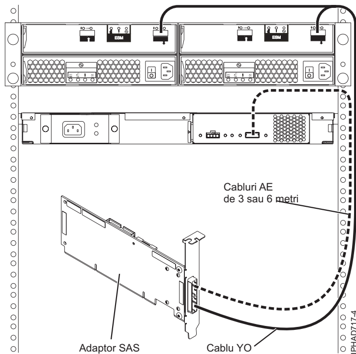
Figura 74. Adaptor SAS la un sertar de expansiune pentru discuri sau un sertar de expansiune pentru medii
