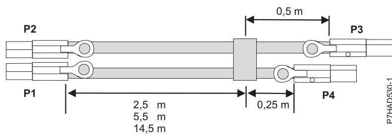
Figura 66. Lungimile de cablu pentru ansamblul cablu X extern SAS
