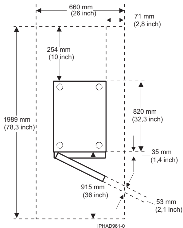
Figura 21. Vedere în plan pentru modelul 0554 și 7014-S11
