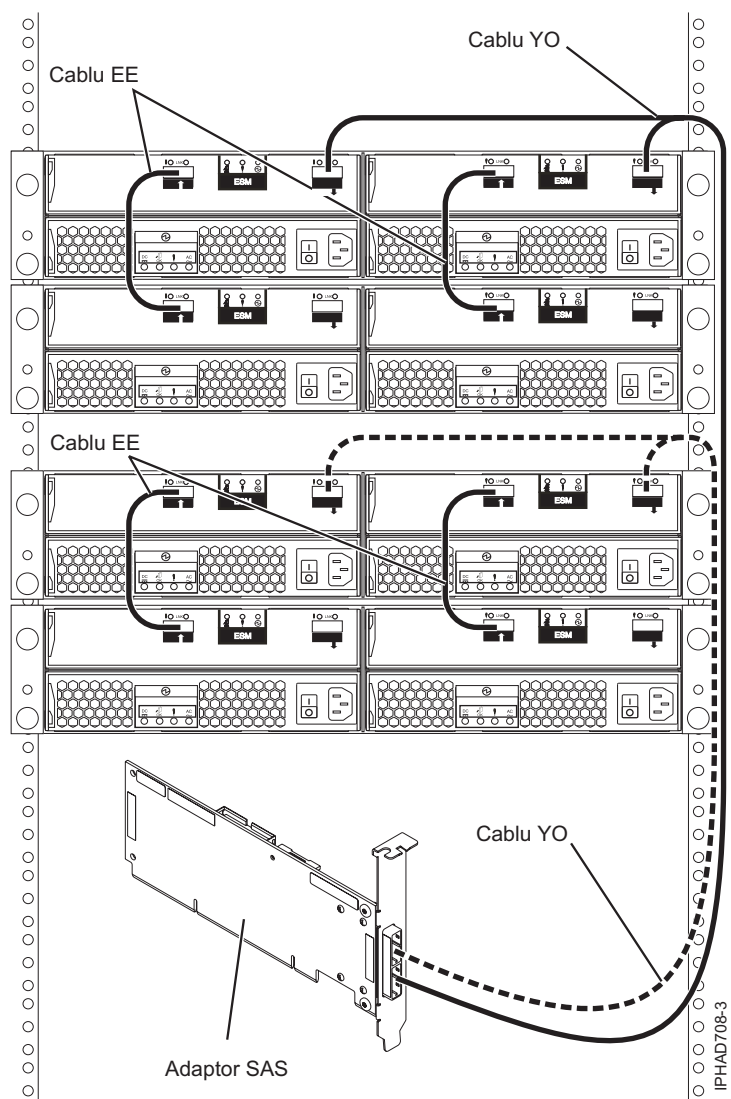
Figura 71. Adaptor SAS la patru sertare de expansiune pentru discuri
