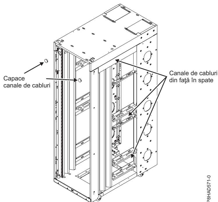
Figura 49. Cablarea în dulap
