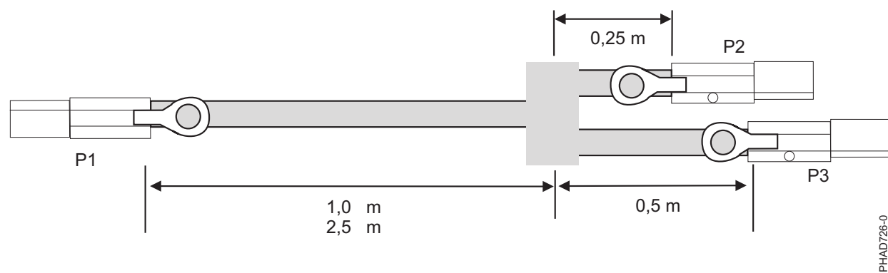
Figura 68. Lungimile de cablu pentru ansamblul cablu YI extern SAS
