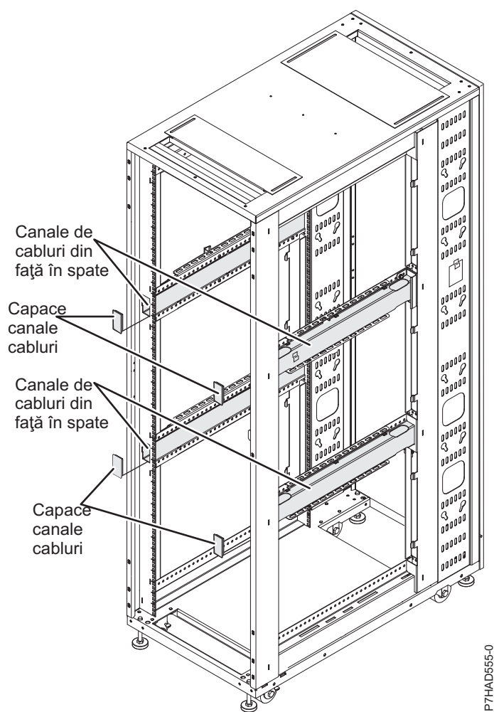
Figura 32. Cablarea în dulap
