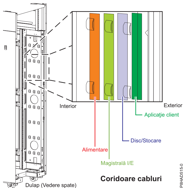
Figura 63. Clemele punții de pozare a cablurilor
