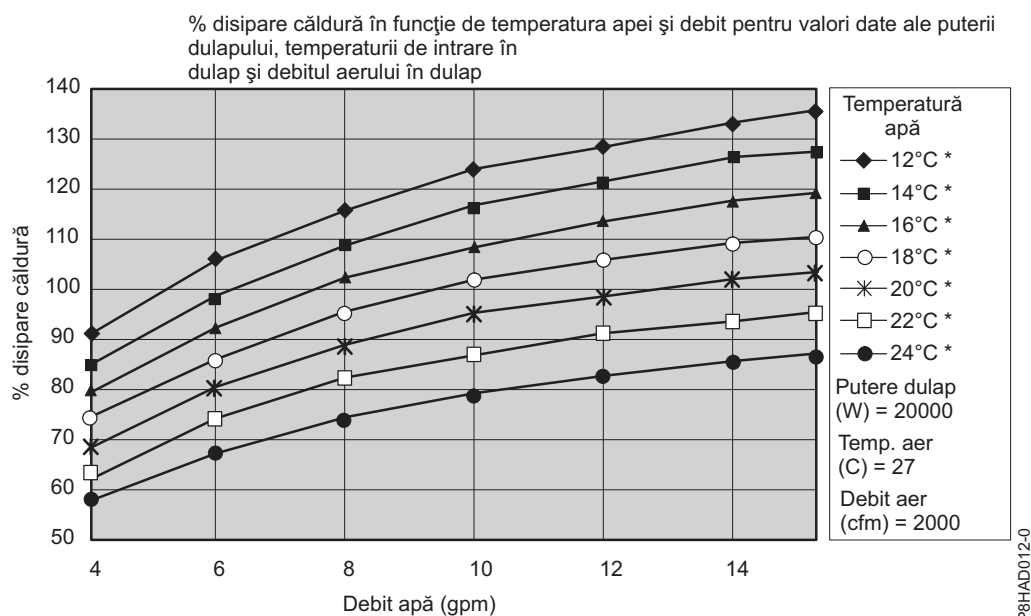
Figura 37. Performanța tipică a schimbătorului de căldură, 20 kW sarcină termică
