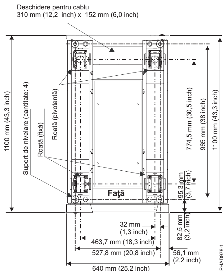
Figura 9. Locațiile roților și nivelatoarelor
