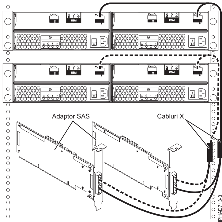
Figura 79. Două adaptoare RAID SAS la două sertare de expansiune disc într-o configurație RAID HA inițiator multiplu
