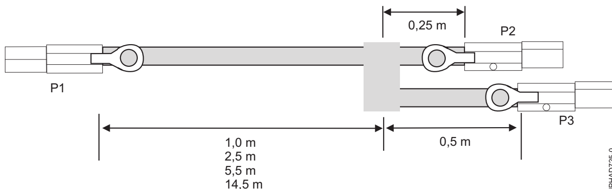
Figura 67. Lungimile de cablu pentru ansamblul cablu YO extern SAS
