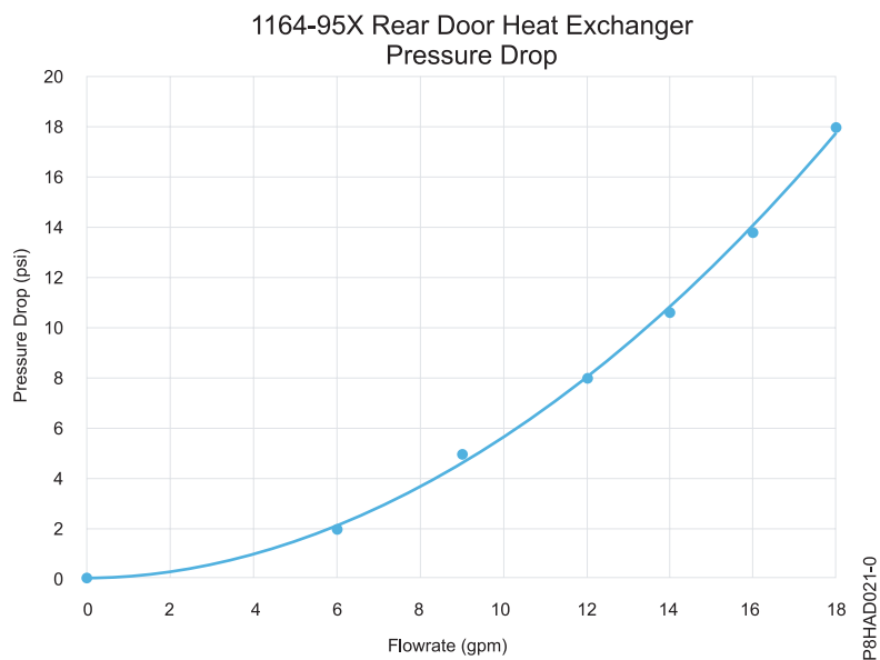
Figura 39. Scăderea presiunii (unități standard)
