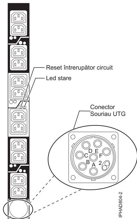
Figura 60. Desen priză PDU
