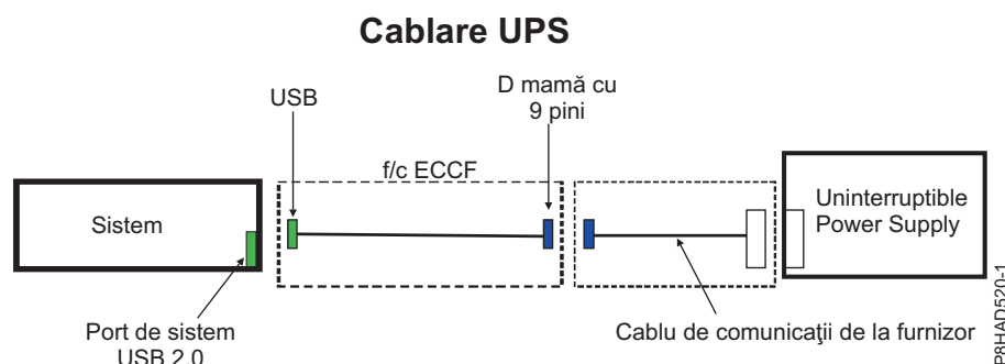
Figura 58. Cablarea UPS pentru 5148-21L, 5148-22L, 8247-21L, 8247-21L, 8247-22L, 8247-42L, 8284-22A, 8286-41A și 8286-42A
