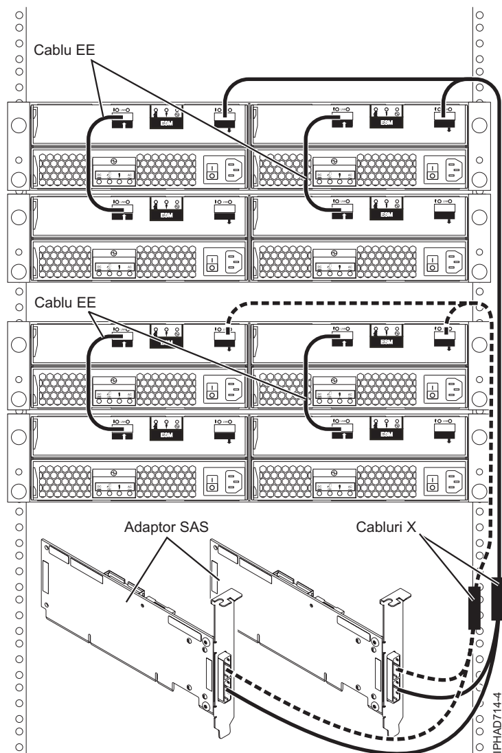
Figura 80. Două adaptoare RAID SAS la patru sertare de expansiune pentru discuri într-o configurație RAID HA inițiator multiplu
