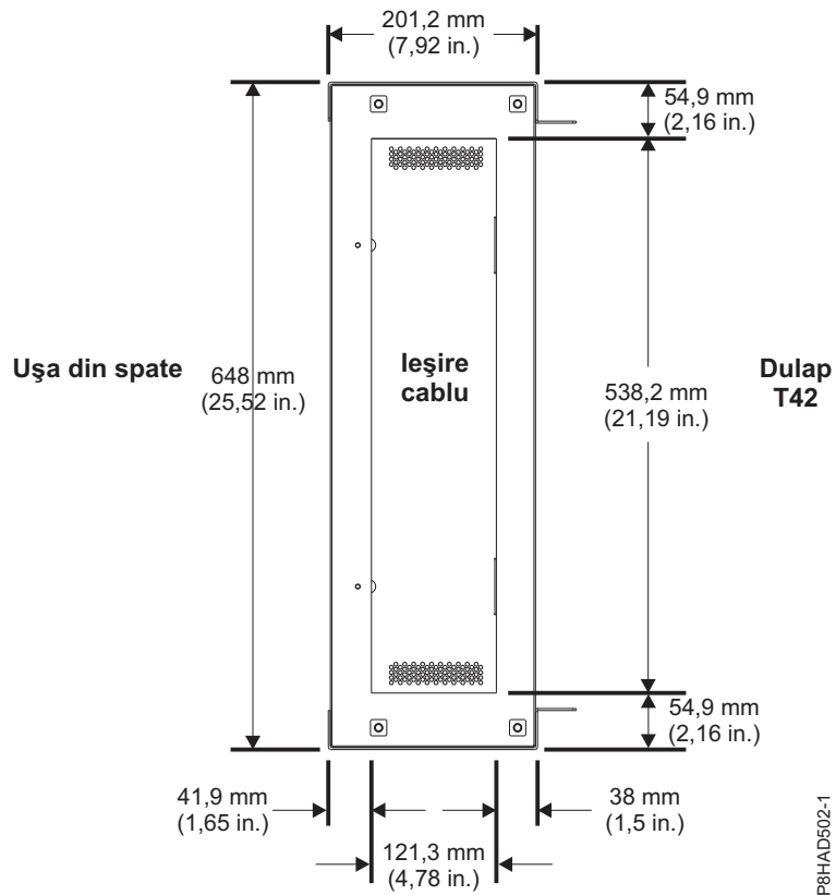
Figura 29. Extenderul de dulap spate FC ERG0 (vizualizare de sus în jos)
