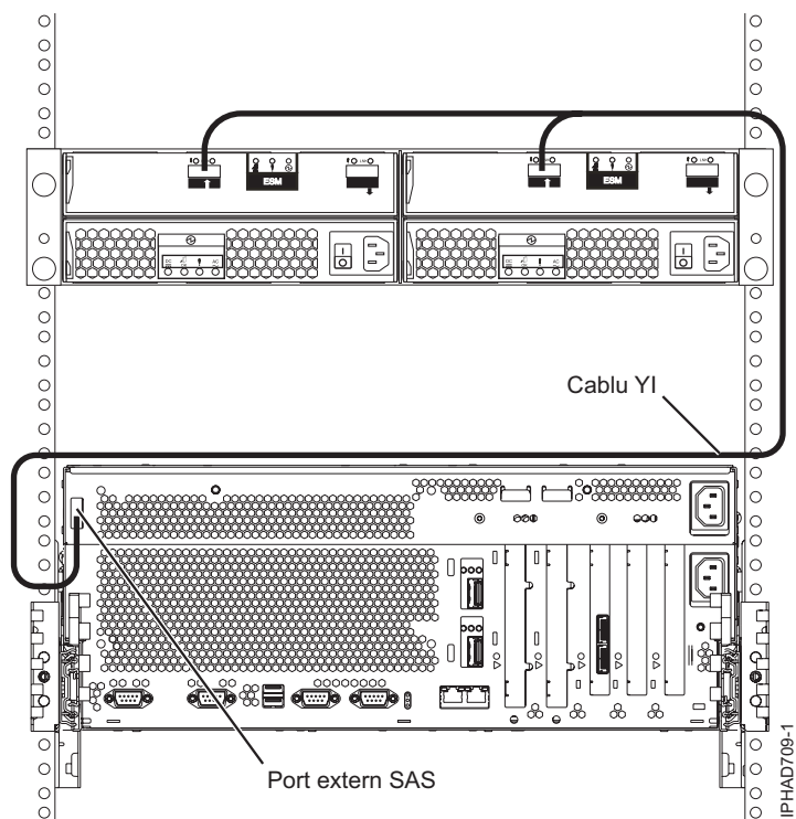
Figura 75. Port de adaptor SAS extern de sistem la un sertar de expansiune pentru discuri
