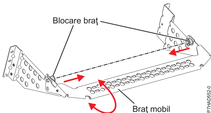
Figura 65. Colțar pentru pozarea cablurilor
