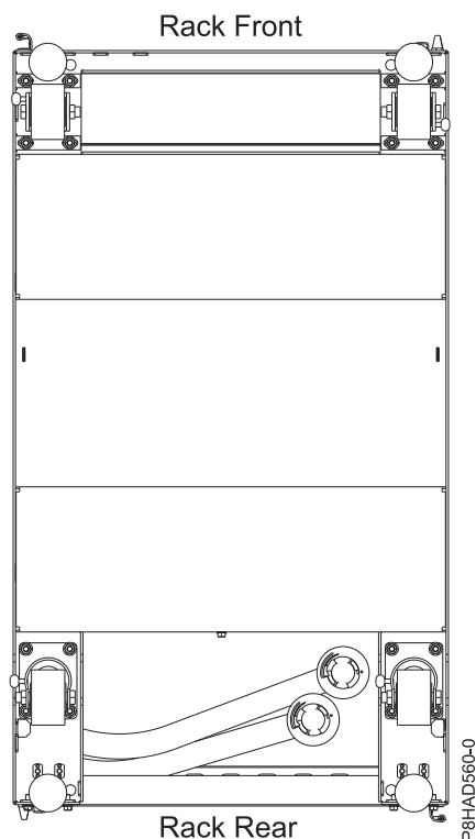
Figura 45. Locațiile de ieșire a furtunurilor în partea de sus (privind de jos)
