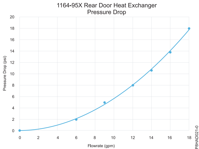
Figura 55. Scăderea presiunii (unități standard)
