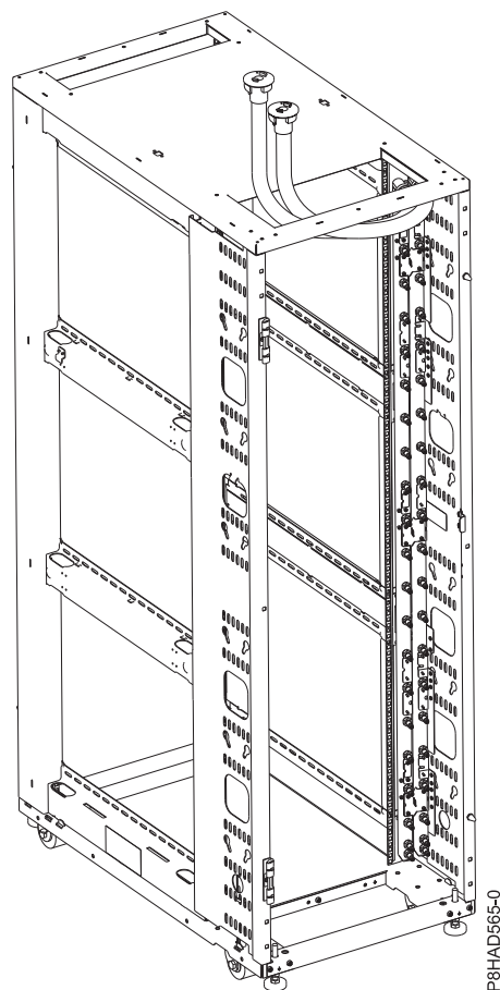
Figura 40. Dulapul și ansamblul furtunurilor de alimentare și retur ce ies prin partea de sus a dulapului
