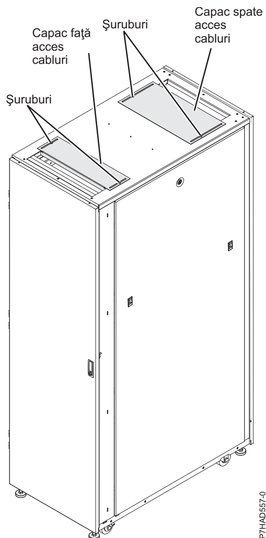
Figura 34. Capace de acces cabluri
