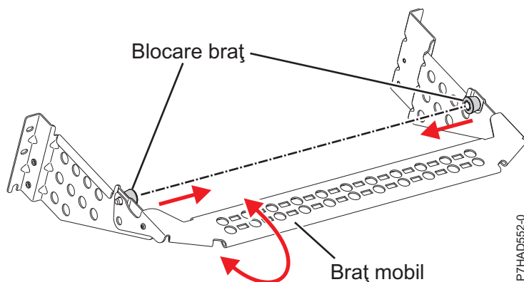
Figura 52. Colțar pentru pozarea cablurilor
