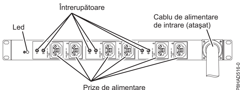
Figura 49. HVDC PDU
