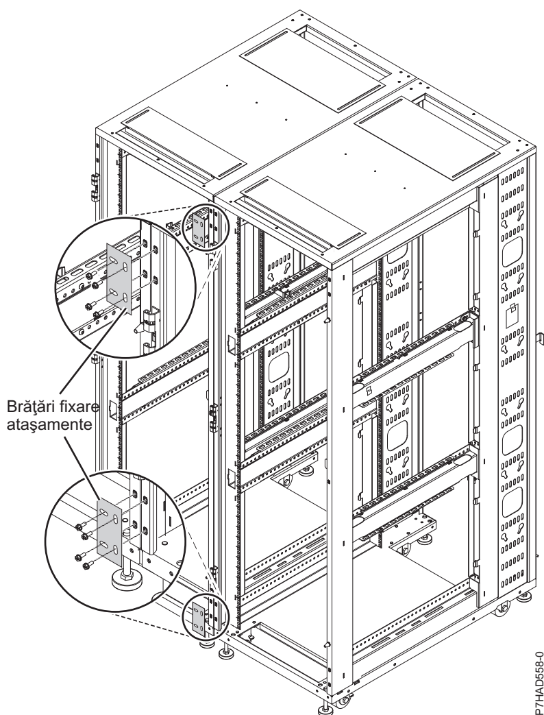
Figura 31. Inele de legătură
