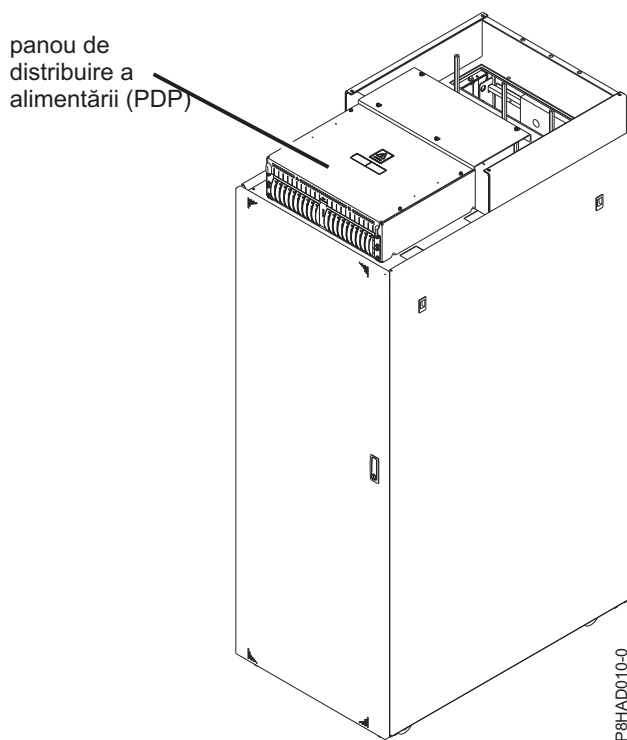
Figura 21. FC EPB8 - panou de distribuție a alimentării
