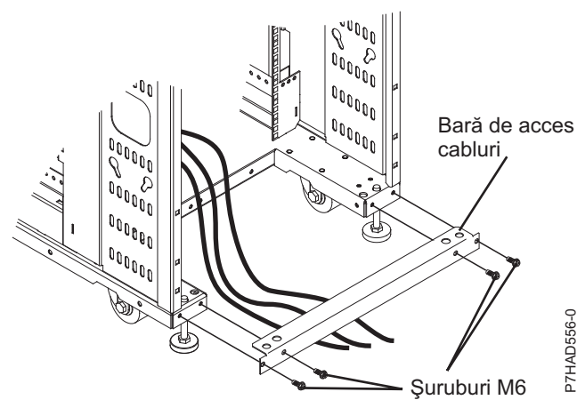
Figura 28. Bara de acces cabluri
