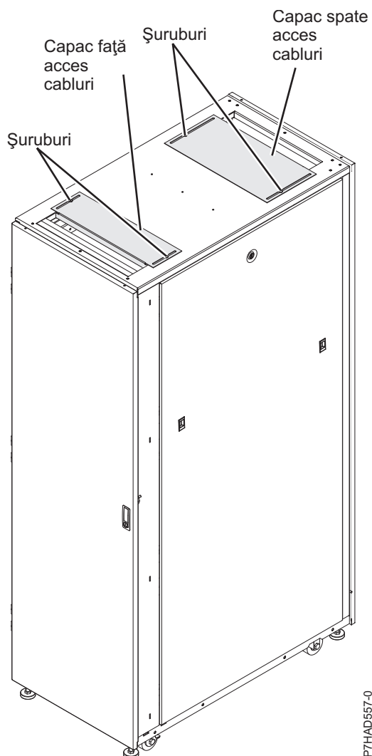
Figura 29. Capace de acces cabluri
