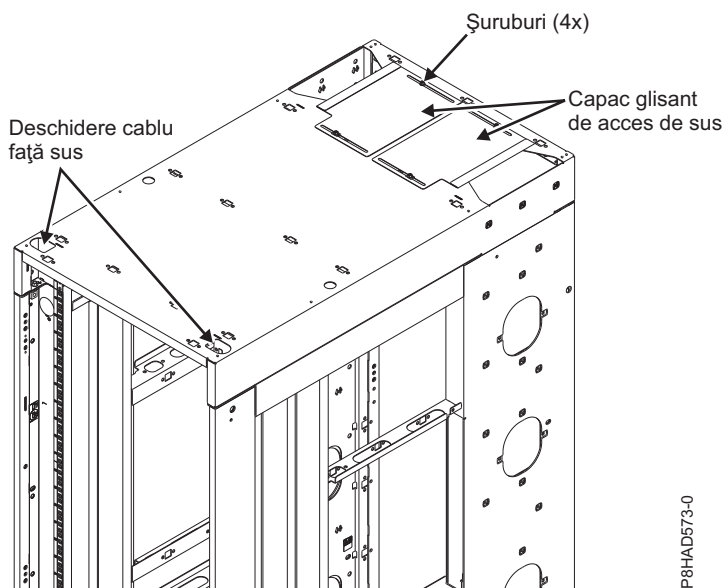
Figura 38. Proiectare cablare
