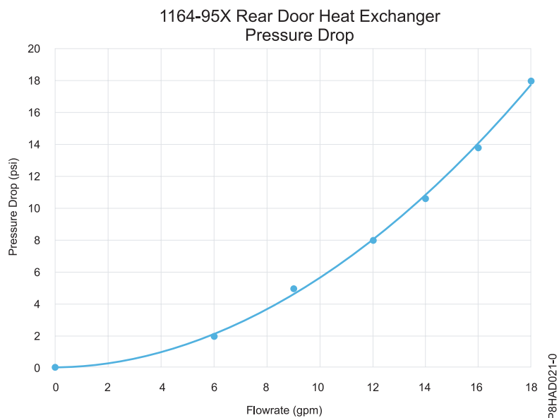
Figura 42. Scăderea presiunii (unități standard)
