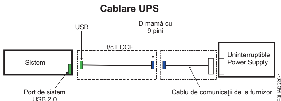
Figura 45. Cablarea UPS pentru 5148-21L, 5148-22L, 8247-21L, 8247-21L, 8247-22L, 8247-42L, 8284-22A, 8286-41A și 8286-42A
