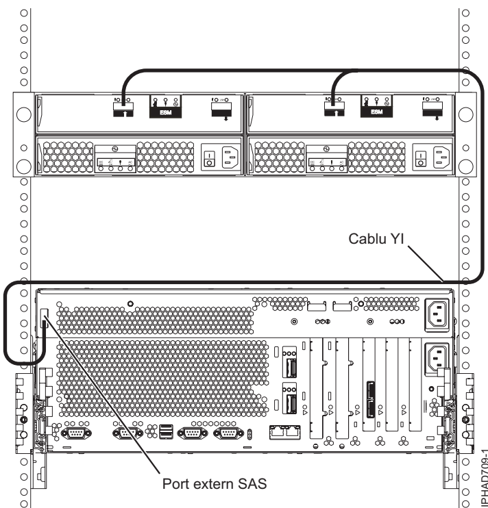
Figura 62. Port de adaptor SAS extern de sistem la un sertar de expansiune pentru discuri
