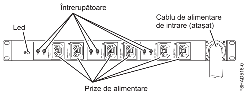
Figura 49. HVDC PDU
