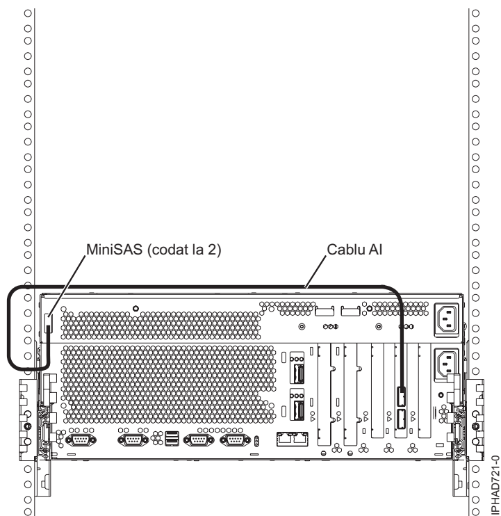
Figura 63. Adaptorul SAS la sloturi de disc SAS intern prin portul SAS extern al sistemului
