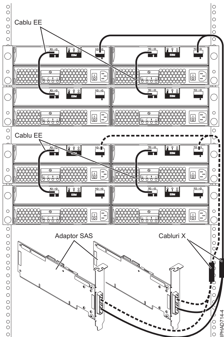
Figura 67. Două adaptoare RAID SAS la patru sertare de expansiune pentru discuri într-o configurație RAID HA inițiator multiplu
