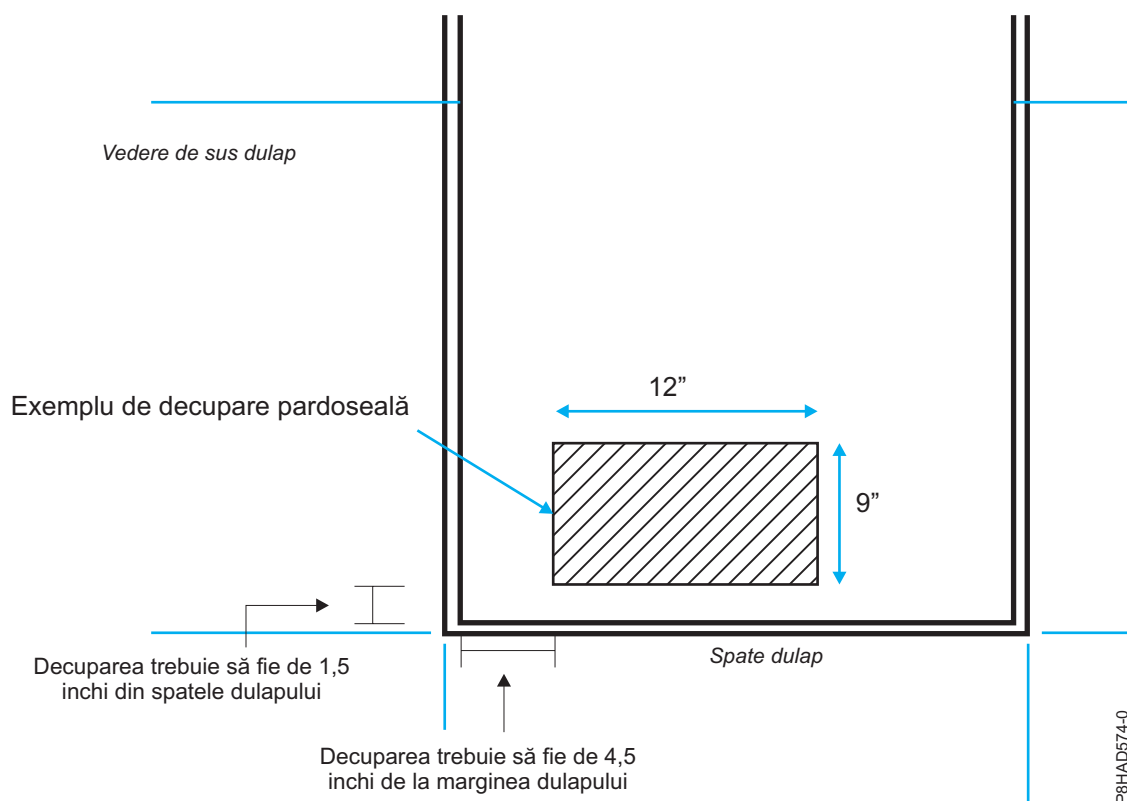
Figura 35. Decuparea în podea
