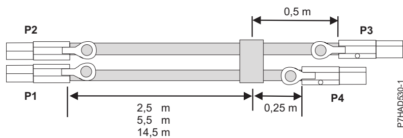
Figura 53. Lungimile de cablu pentru ansamblul cablu X extern SAS
