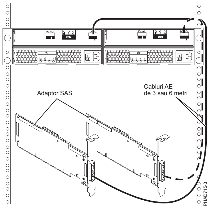
Figura 73. Două adaptoare SAS RAID la un sertar de expansiune pentru discuri într-o configurație JBOD HA inițializator multiplu
