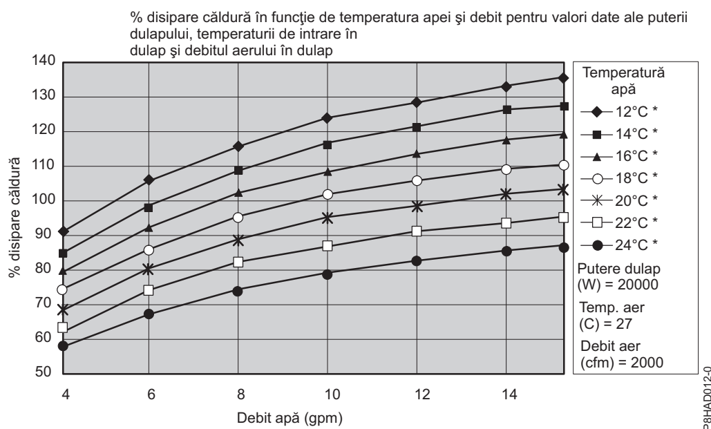
Figura 40. Performanța tipică a schimbătorului de căldură, 20 kW sarcină termică
