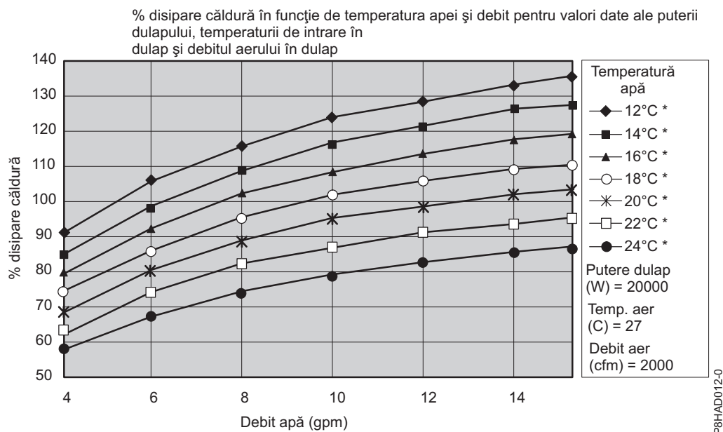
Figura 32. Performanța tipică a schimbătorului de căldură, 20 kW sarcină termică
