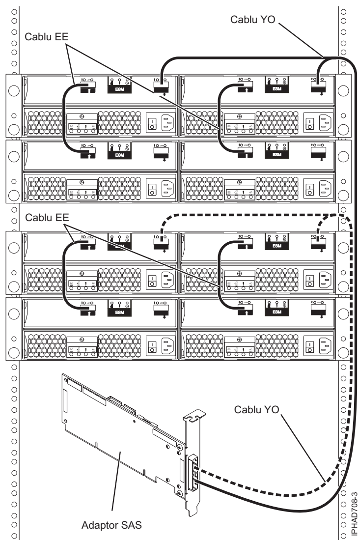
Figura 58. Adaptor SAS la patru sertare de expansiune pentru discuri
