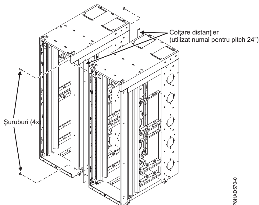
Figura 39. Unirea mai multor dulapuri
