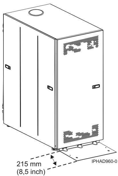
Figura 18. Modelul 0555 și 7014-S25 cu picior stabilizator
