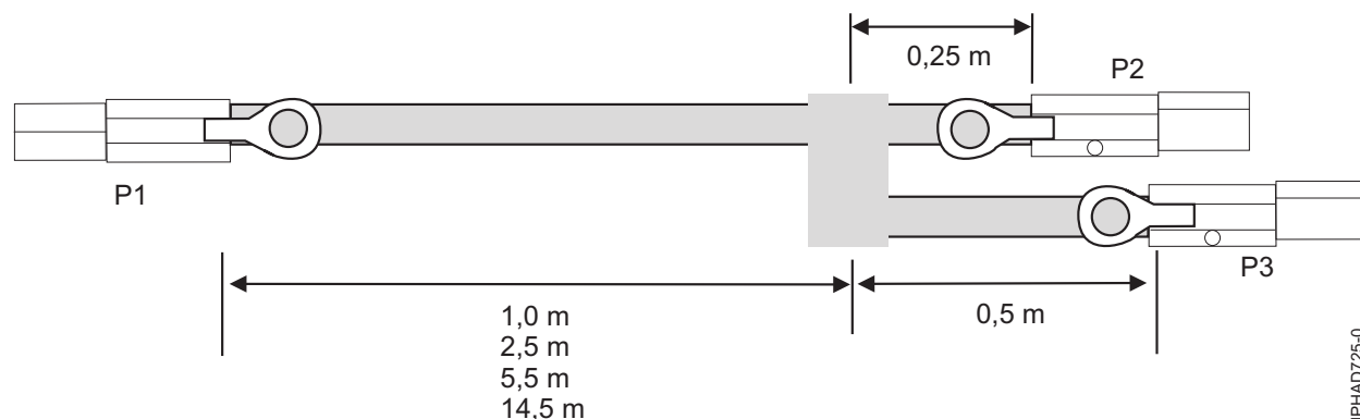
Figura 54. Lungimile de cablu pentru ansamblul cablu YO extern SAS
