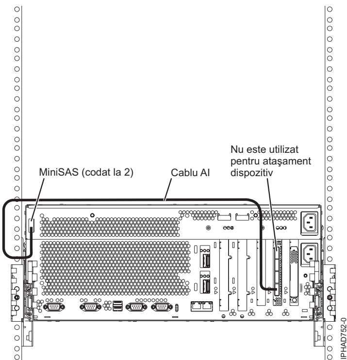
Figura 64. Adaptor FC5904 sau FC5908 atașat la sertare de expansiune pentru discuri
