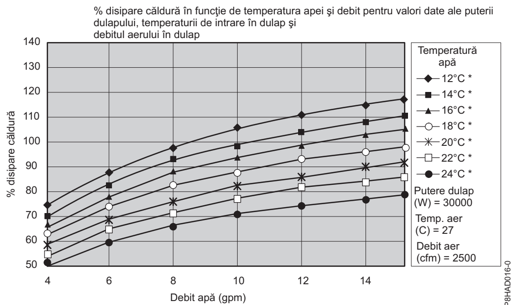
Figura 41. Performanța tipică a schimbătorului de căldură, 30 kW sarcină termică
