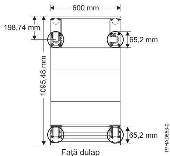
Figura 26. Locațiile roților
