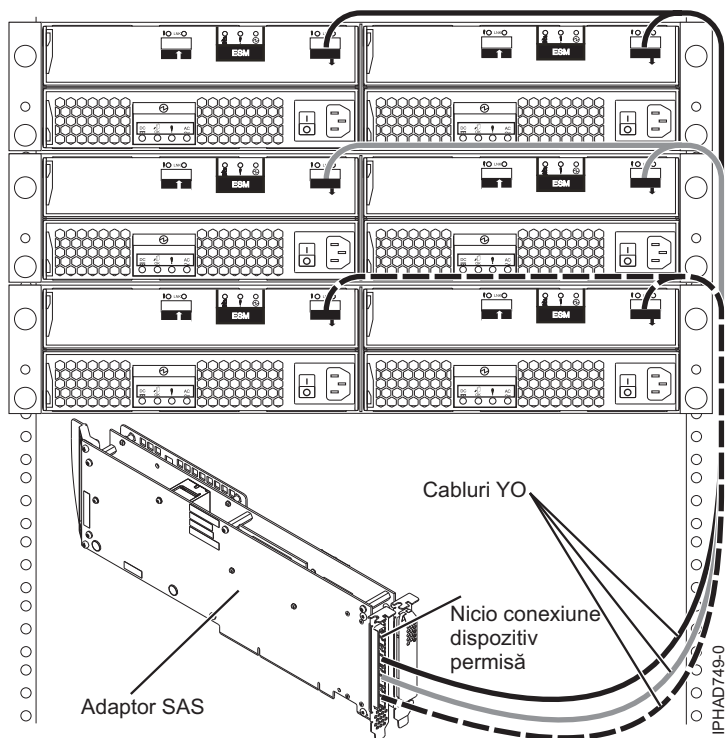
Figura 59. Adaptor SAS cu trei porturi la sertare de expansiune pentru discuri
