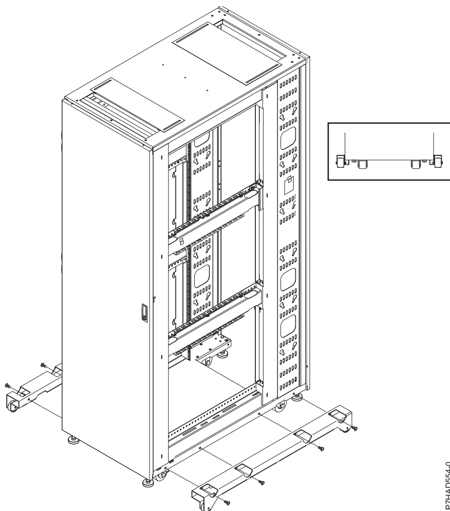
Figura 30. Locaţii console
