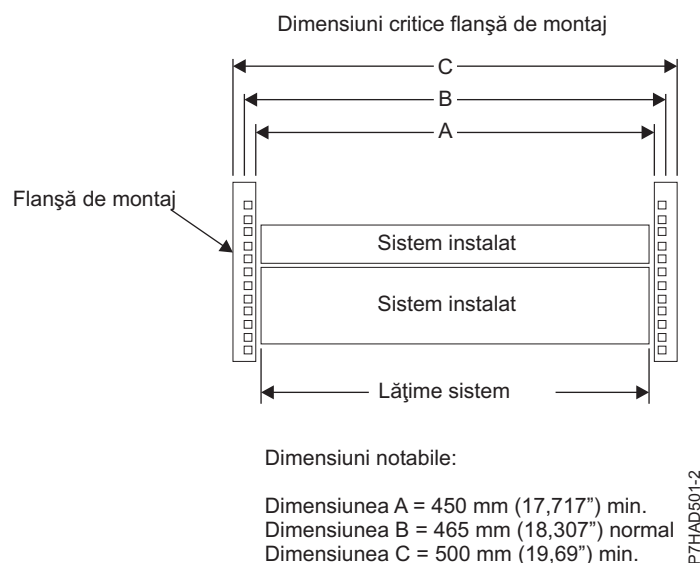
Figura 43. Dimensiuni de bordură de montare critice
