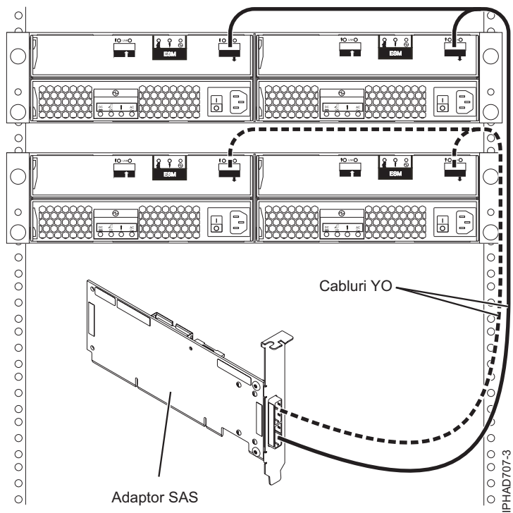
Figura 57. Adaptor SAS la două sertare de expansiune pentru discuri
