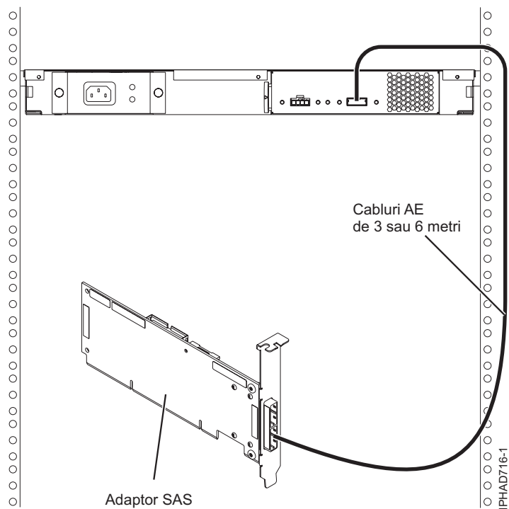
Figura 60. Adaptor SAS la un sertar de expansiune pentru medii
