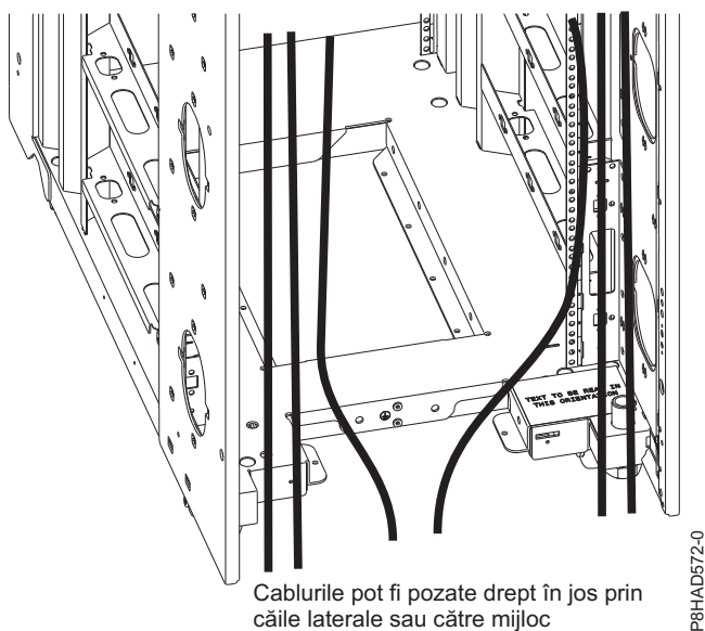
Figura 37. Cablarea sub podea
