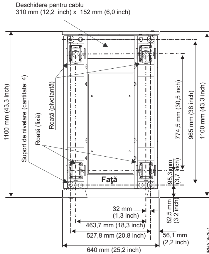
Figura 23. Locațiile roților și nivelatoarelor
