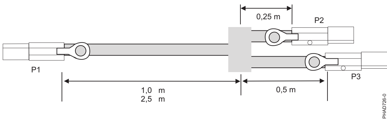
Figura 55. Lungimile de cablu pentru ansamblul cablu YI extern SAS
