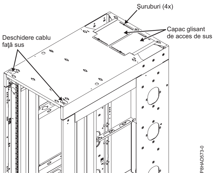
Figura 38. Proiectare cablare
