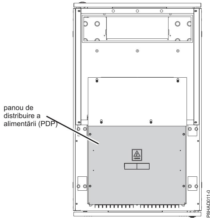
Figura 22. FC EPB8 - panou de distribuire a alimentării (vizualizare de sus în jos)
