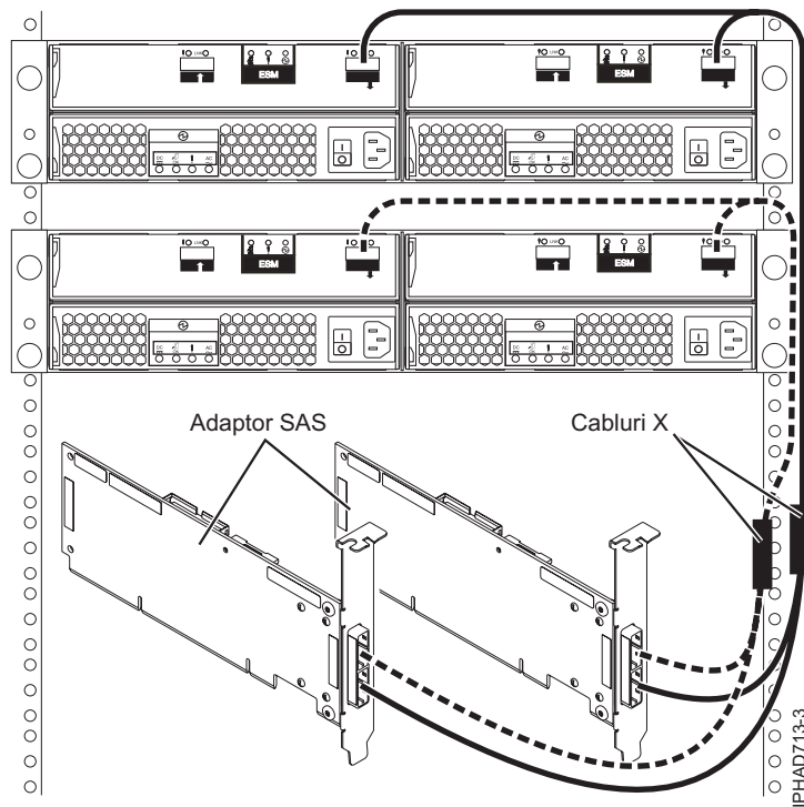
Figura 66. Două adaptoare RAID SAS la două sertare de expansiune disc într-o configurație RAID HA inițiator multiplu
