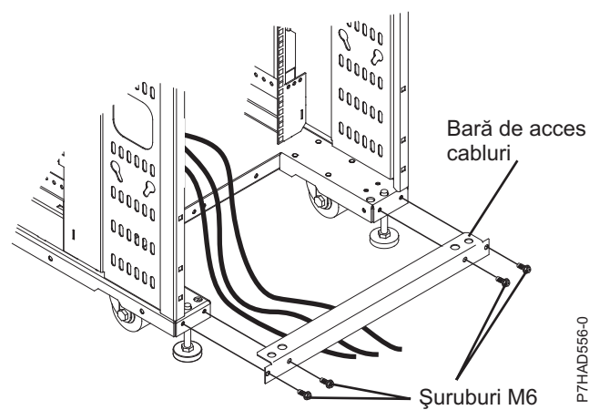
Figura 28. Bară de acces cabluri
