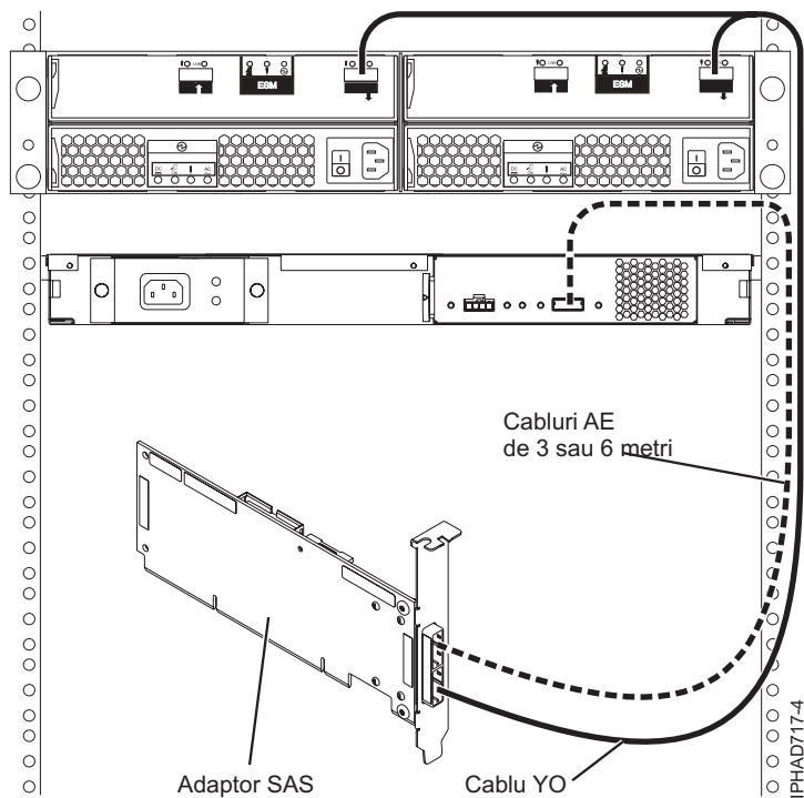
Figura 61. Adaptor SAS la un sertar de expansiune pentru discuri sau un sertar de expansiune pentru medii
