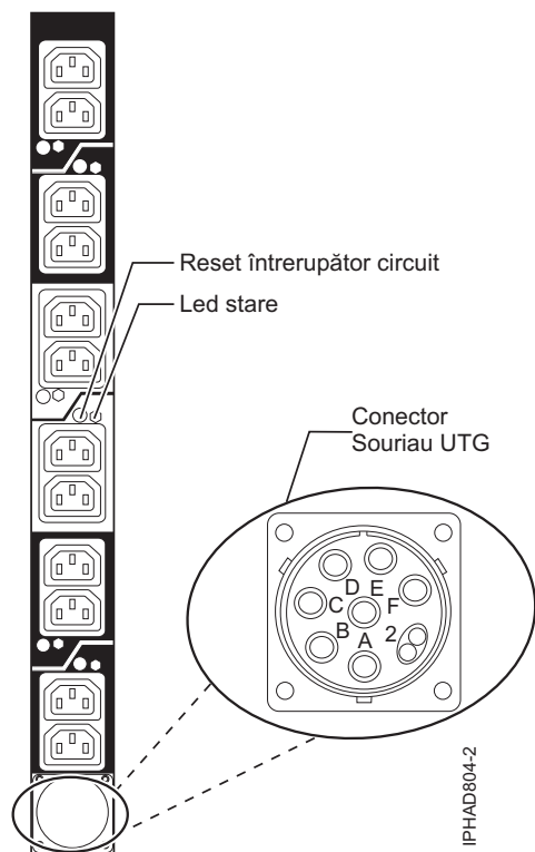
Figura 47. Desen priză PDU
