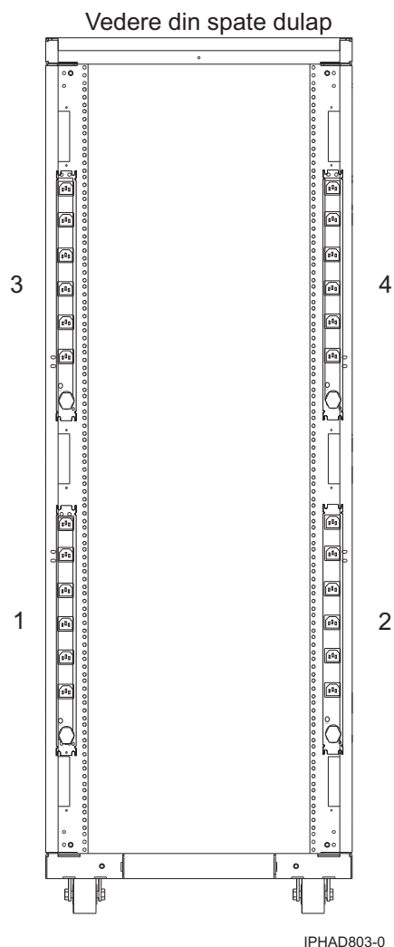
Figura 46. Locații verticale pentru Unitatea de distribuție alimentare
