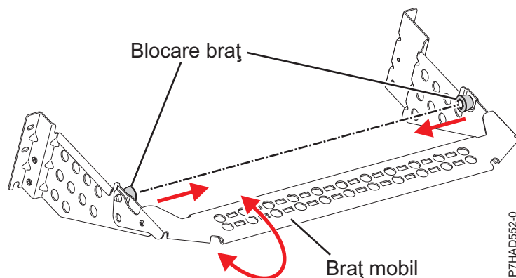
Figura 52. Colțar pentru pozarea cablurilor
