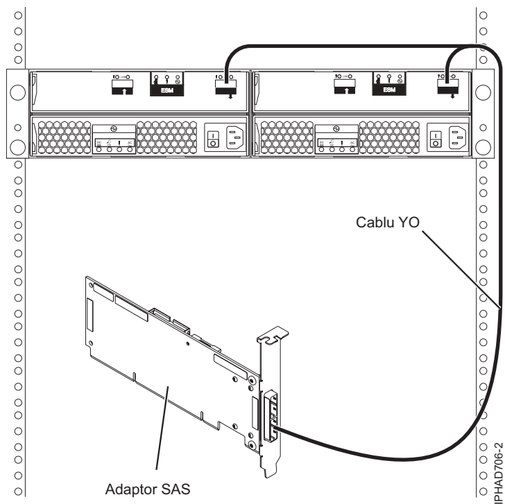
Figura 56. Adaptor SAS la un sertar de expansiune pentru discuri
