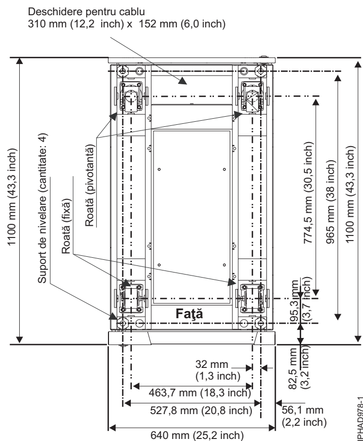
Figura 4. Locațiile roților și nivelatoarelor
