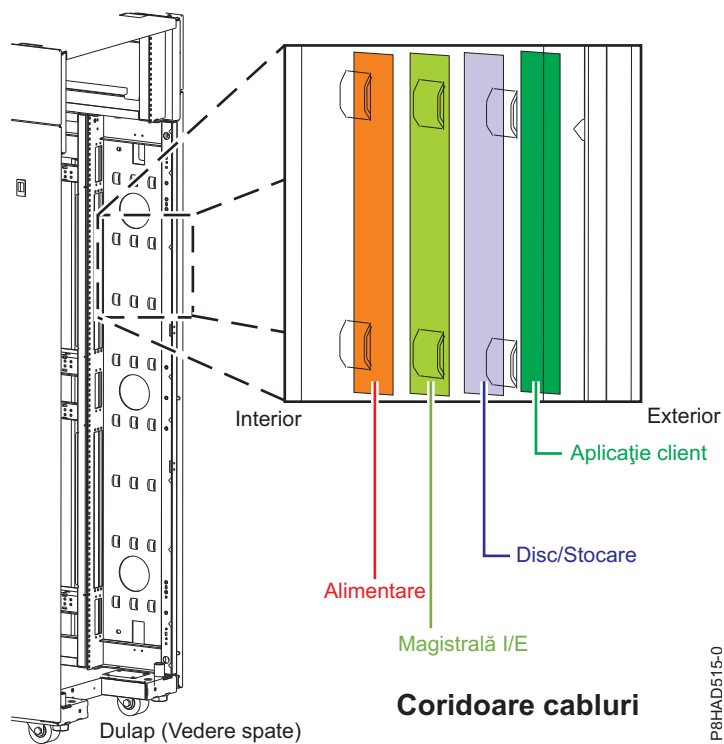
Figura 50. Clemele punții de pozare a cablurilor
