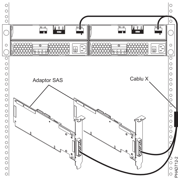
Figura 65. Două adaptoare RAID SAS la un sertar de expansiune pentru discuri într-o configurație RAID HA inițiator multiplu
