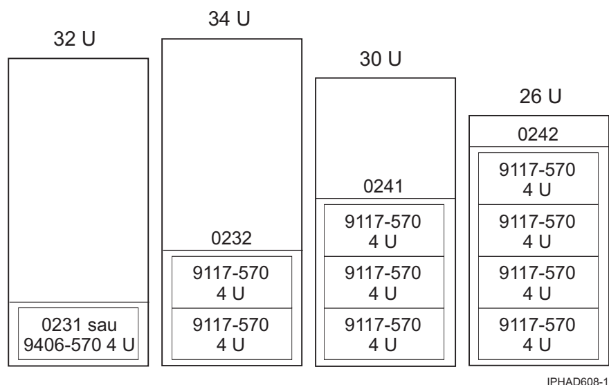
Figura 7. 570 în dulap
