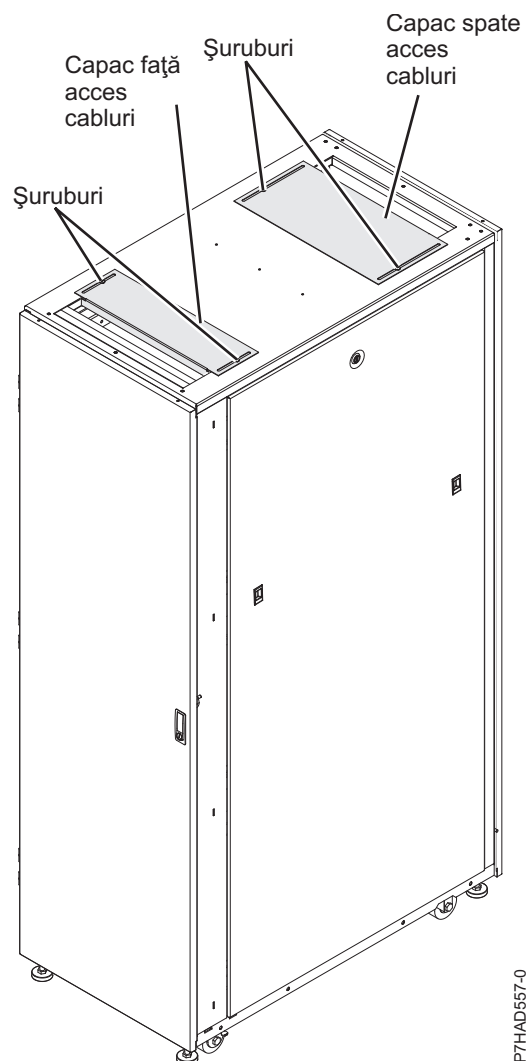
Figura 29. Capace de acces cabluri
