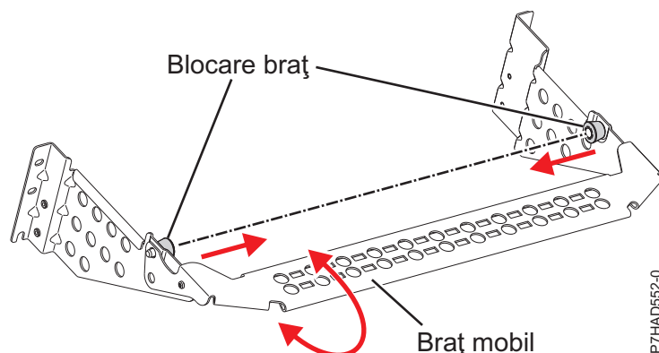
Figura 52. Colțar pentru pozarea cablurilor
