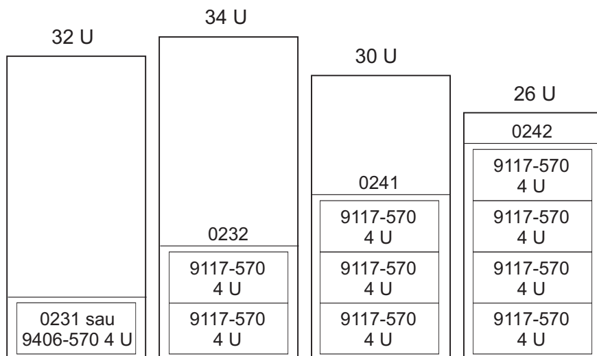
Figura 7. 570 în dulap
