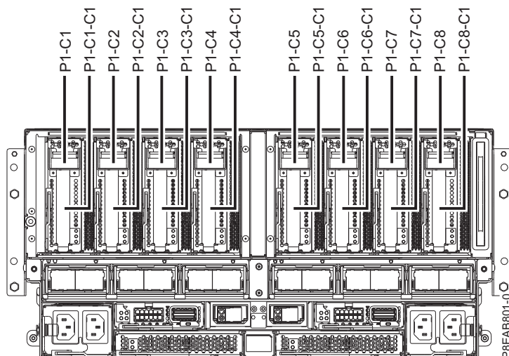
Figura 1. Vederea din spate a unui sistem 9080-MHE, 9080-MME, 9119-MHE sau 9119-MME, cu codurile de locație pentru sloturile PCIe
