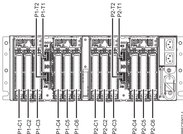
Figura 2. Vederea din spate a sertarul de expansiune PCIe3, cu codurile de locație pentru sloturile PCIe
