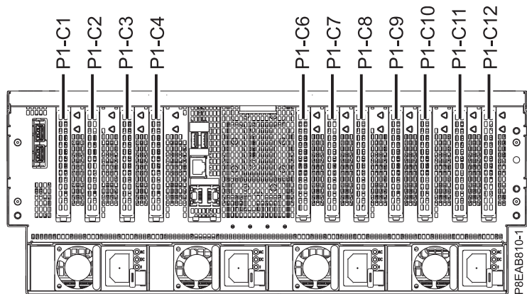
Figura 1. Vederea din spate a unui sistem 8408-44E sau 8408-E8E, cu codurile de locație pentru sloturile PCIe
