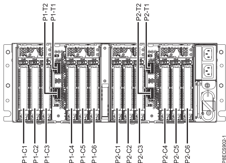
Figura 2. Vederea din spate a sertarului de expansiune PCIe3, cu codurile de locație pentru sloturile PCIe
