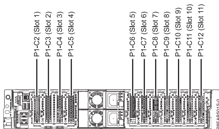
Figura 1. Vederea din spate a unui sistem 5148-21L, 5148-22L, 8247-21L,8247-22L,8284-21A,sau 8284-22A, cu codurile de locație pentru sloturile PCIe
