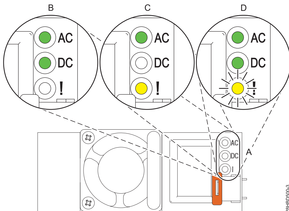
Figura 3. LEDs para uma fonte de alimentação em funcionamento e em falha
