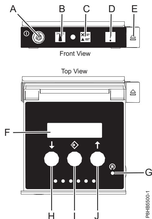
Figura 13. LEDs do painel de controlo
