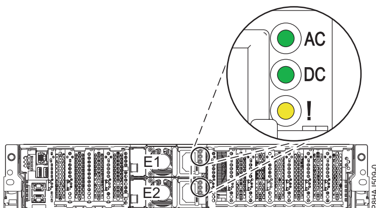
Figura 7. Localização das fontes de alimentação e LEDs no sistema
