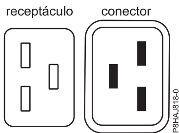
Figura 22. Conectores para o sistema 8408-44E
