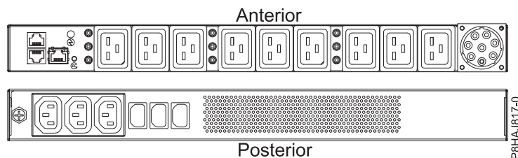
Figura 23. PDU para o sistema 8408-44E
