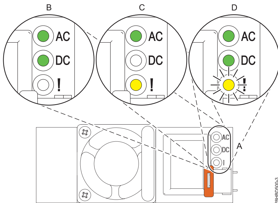
Figura 8. LEDs para uma fonte de alimentação em funcionamento e em falha
