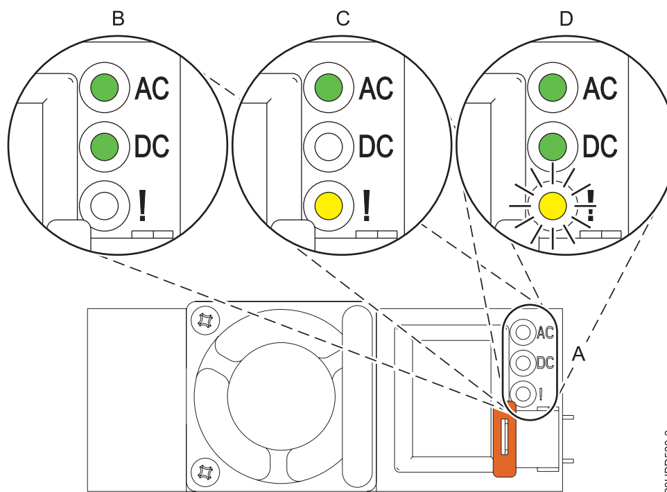
Figura 12. LEDs para uma fonte de alimentação em funcionamento e em falha
