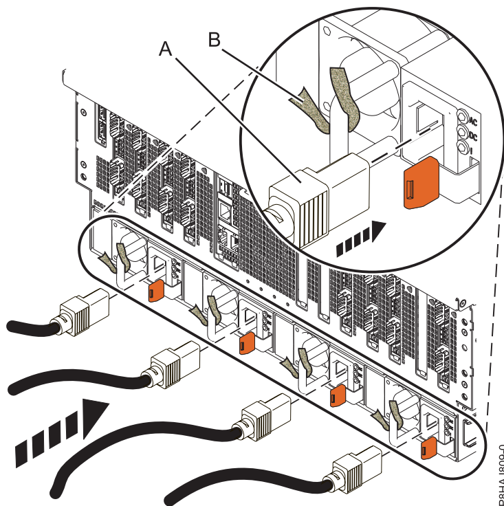
Figura 26. Ligar os cabos de alimentação a um sistema 8408-44E ou 8408-E8E
