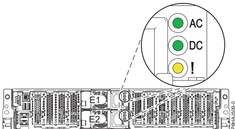
Figura 1. Localização das fontes de alimentação e LEDs no sistema
