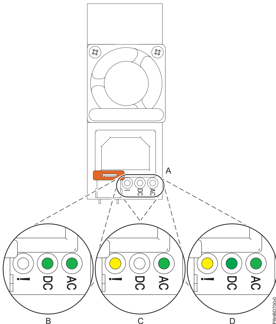
Figura 4. LEDs para uma fonte de alimentação em funcionamento e em falha num sistema autónomo
