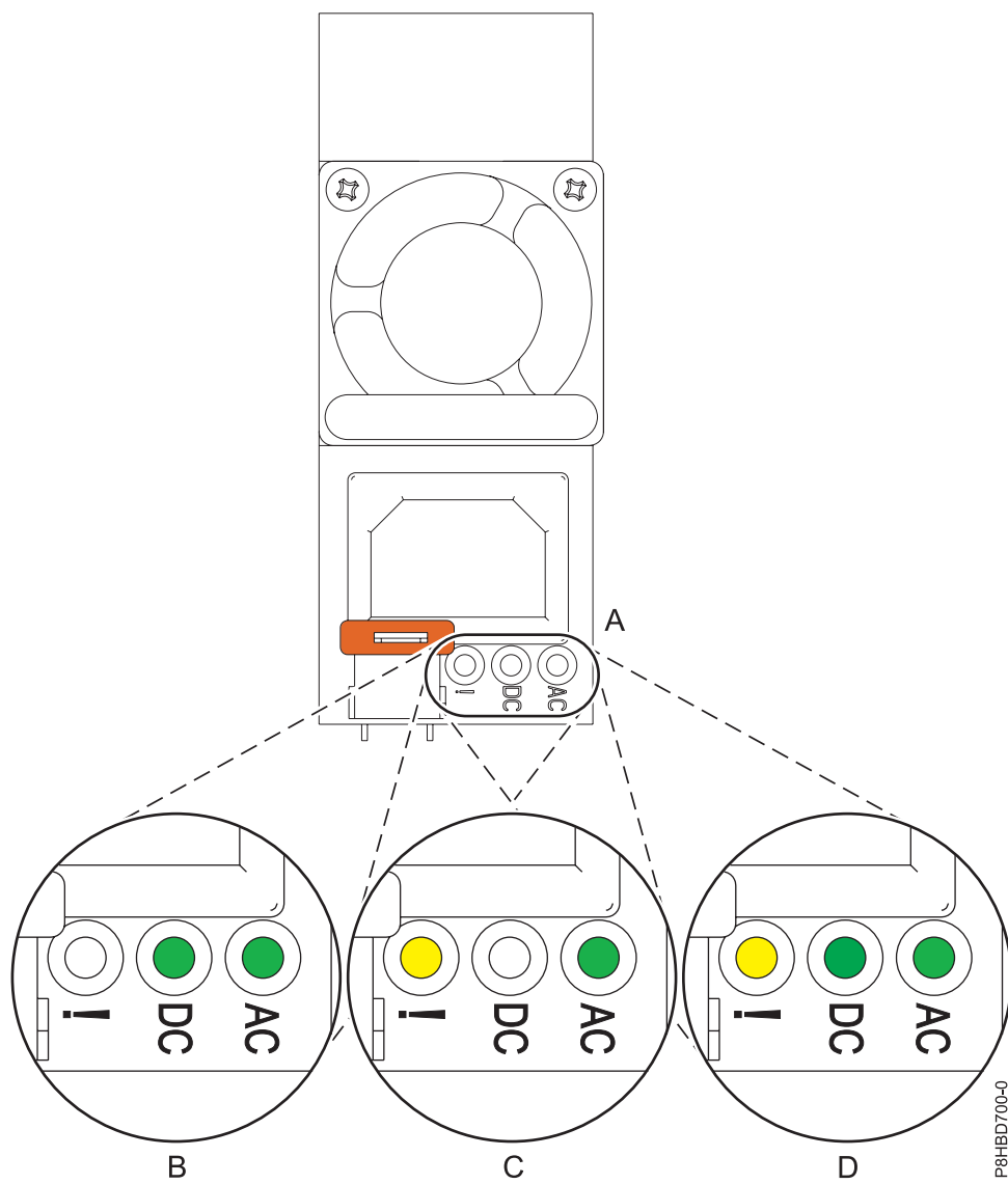
Figura 24. LEDs para uma fonte de alimentação em funcionamento e em falha num sistema autónomo
