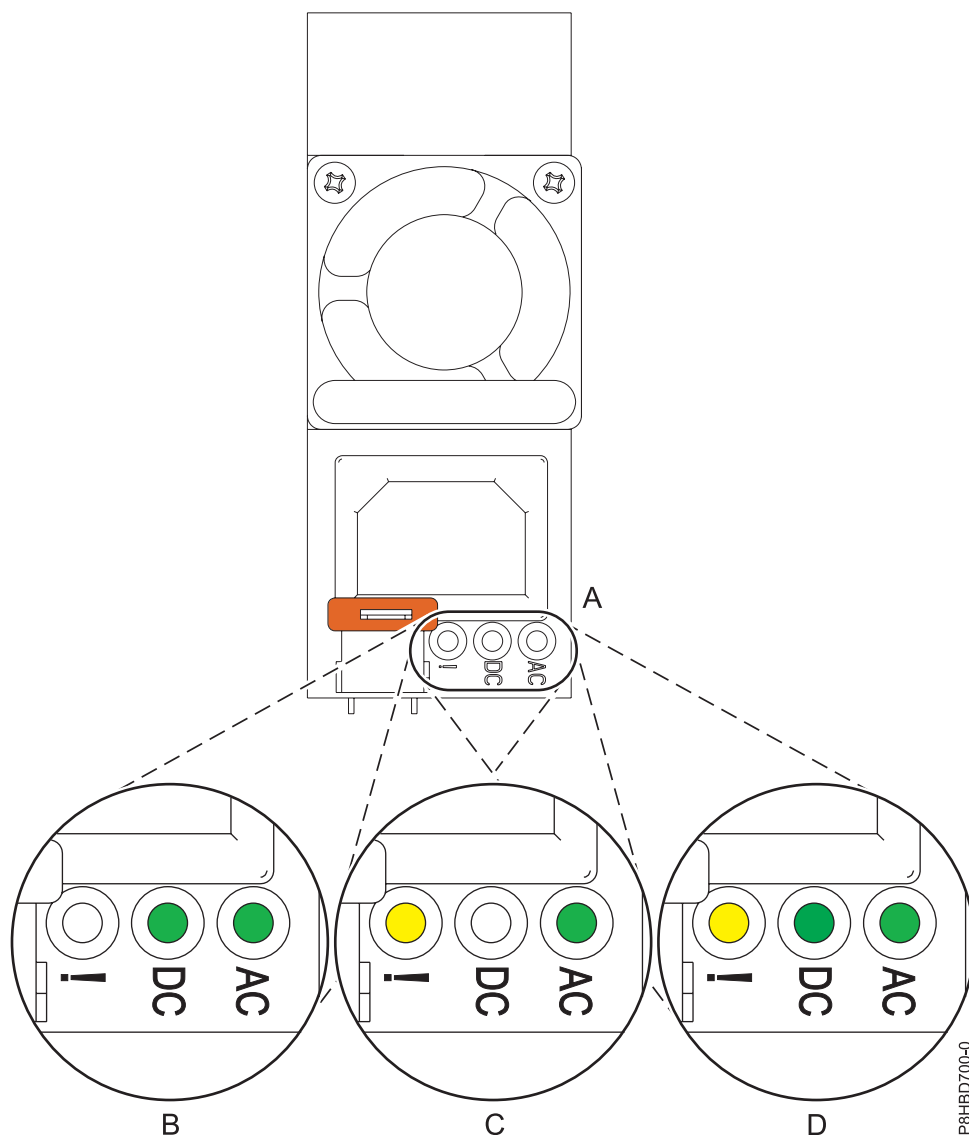
Figura 12. LEDs para uma fonte de alimentação em funcionamento e em falha num sistema autónomo
