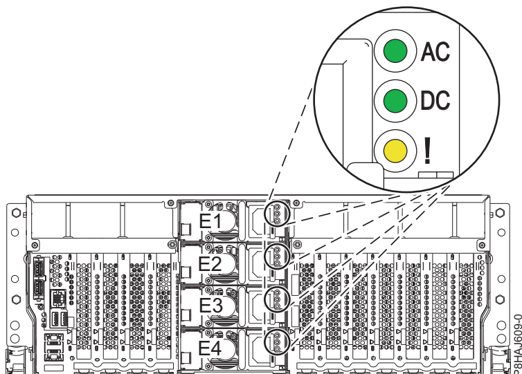
Figura 1. Localização das fontes de alimentação e LEDs num sistema montado em bastidor
