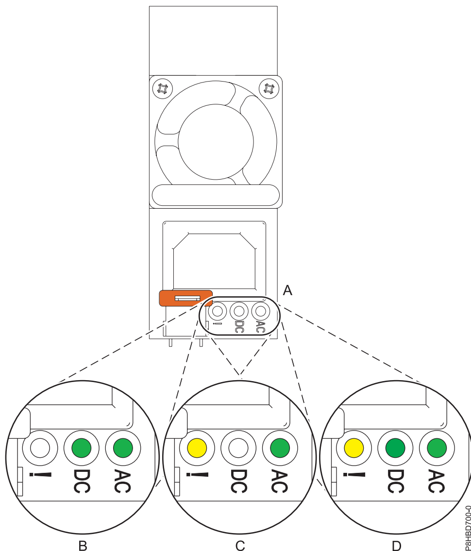
Figura 16. LEDs para uma fonte de alimentação em funcionamento e em falha num sistema autónomo
