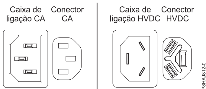
Figura 33. Conectores de AC e de HVDC
