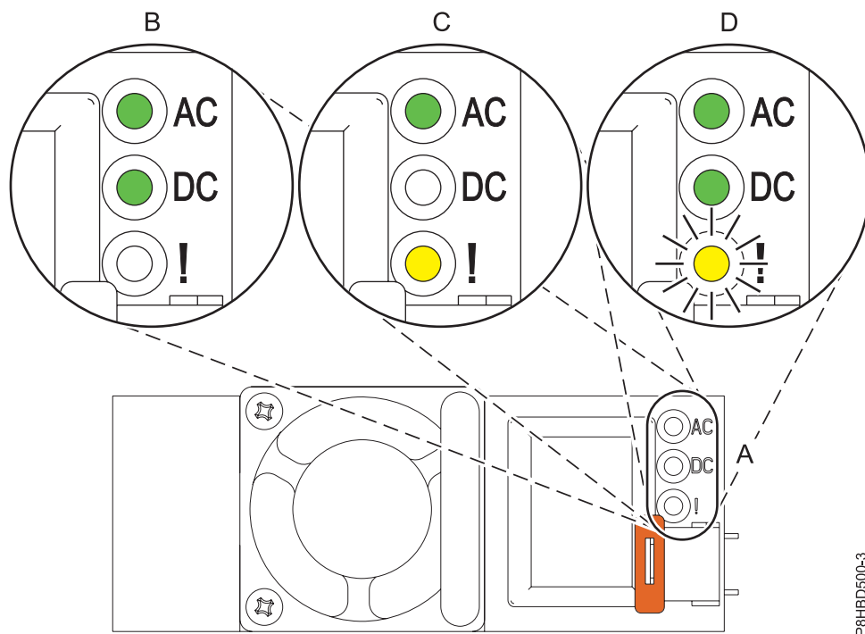
Figura 23. LEDs para uma fonte de alimentação em funcionamento e em falha num sistema montado em bastidor
