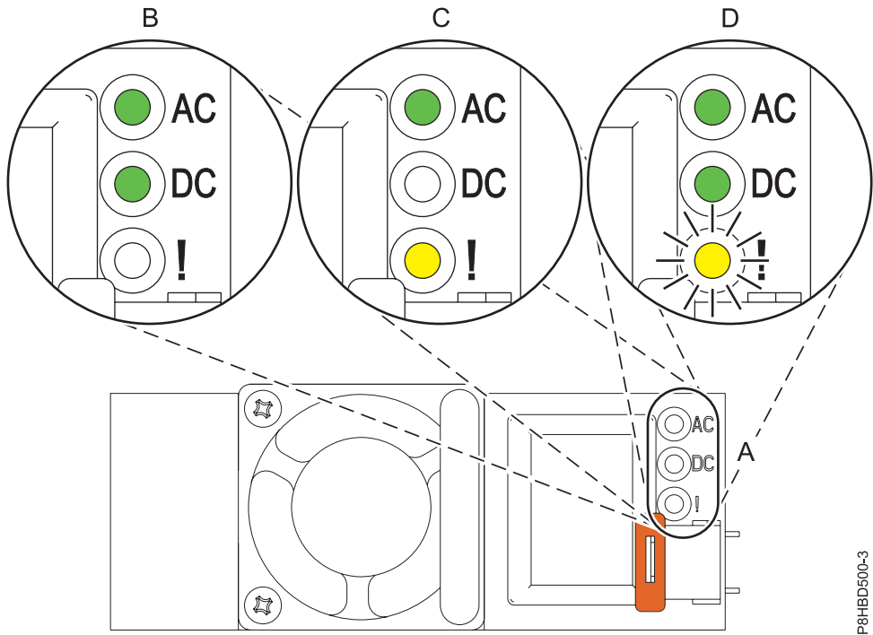
Figura 3. LEDs para uma fonte de alimentação em funcionamento e em falha num sistema montado em bastidor
