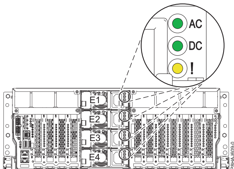
Figura 13. Localização das fontes de alimentação e LEDs num sistema montado em bastidor
