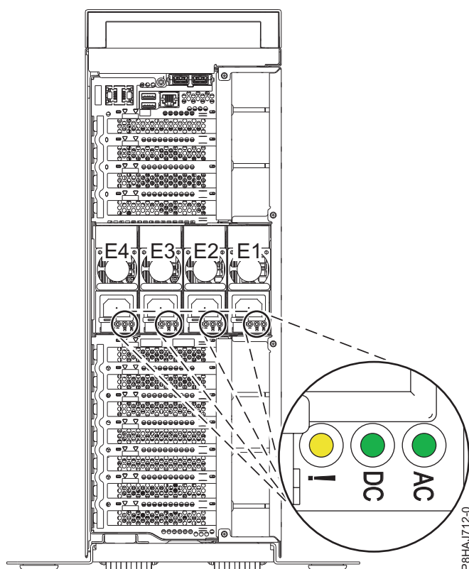
Figura 2. Localização das fontes de alimentação e LEDs num sistema autónomo
