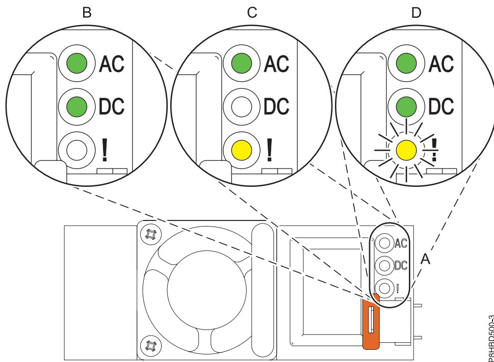
Figura 11. LEDs para uma fonte de alimentação em funcionamento e em falha num sistema montado em bastidor
