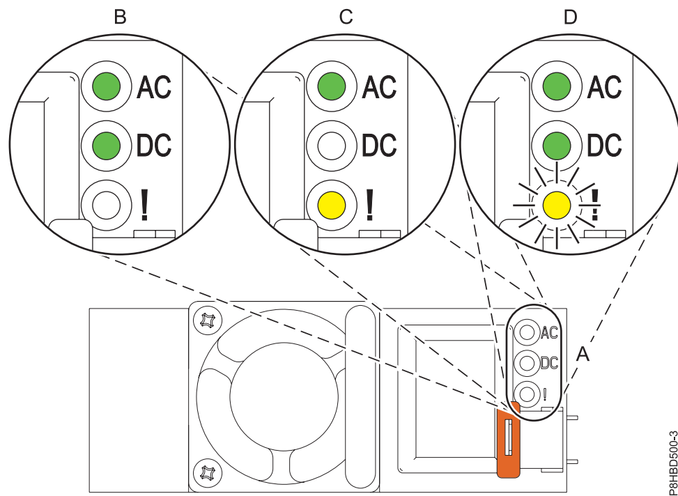
Figura 15. LEDs para uma fonte de alimentação em funcionamento e em falha num sistema montado em bastidor
