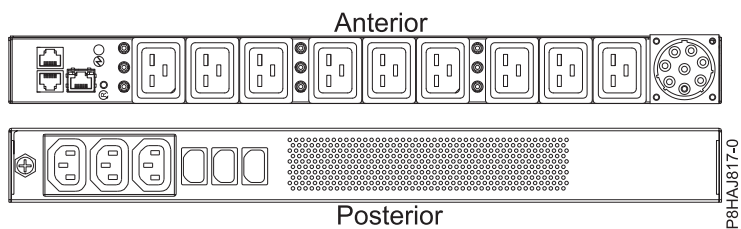
Figura 29. PDU para o sistema 8408-44E
