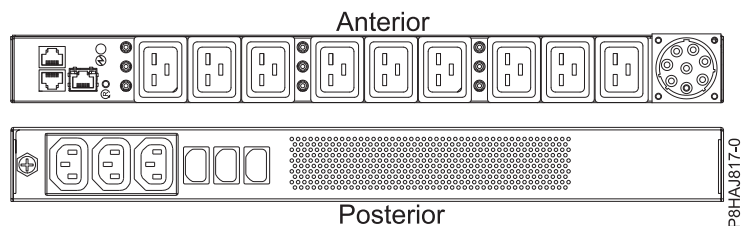
Figura 35. PDU para o sistema 8408-44E
