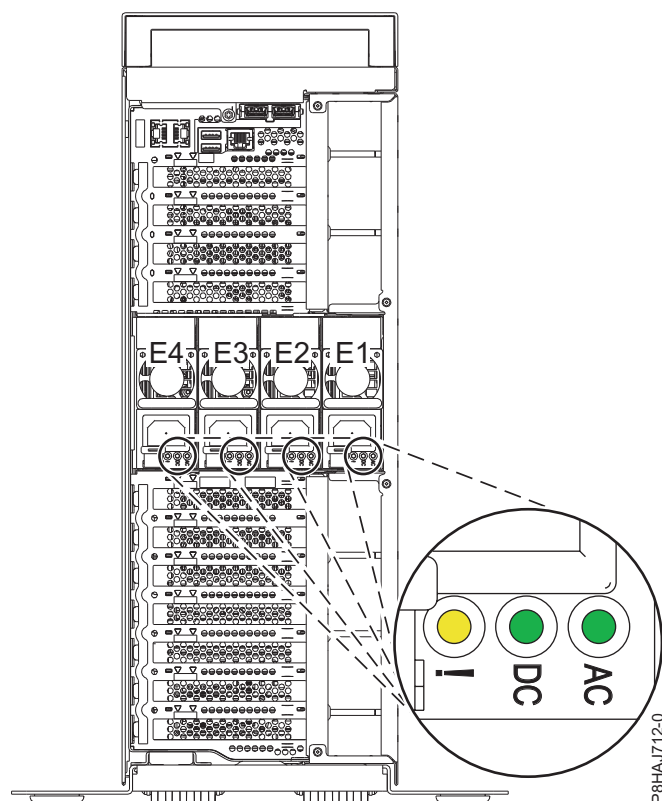
Figura 14. Localização das fontes de alimentação e LEDs num sistema autónomo
