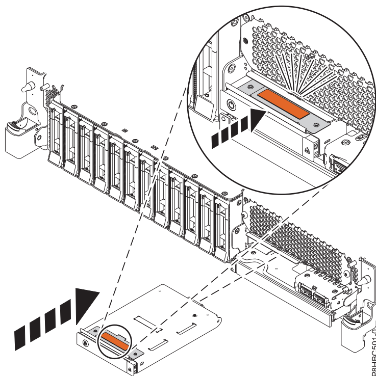
Figura 5. Substituir o painel de controlo
