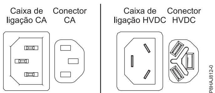
Figura 34. Conectores de AC e de HVDC
