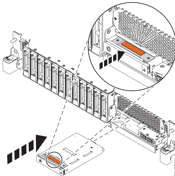
Figura 2. Substituir o painel de controlo
