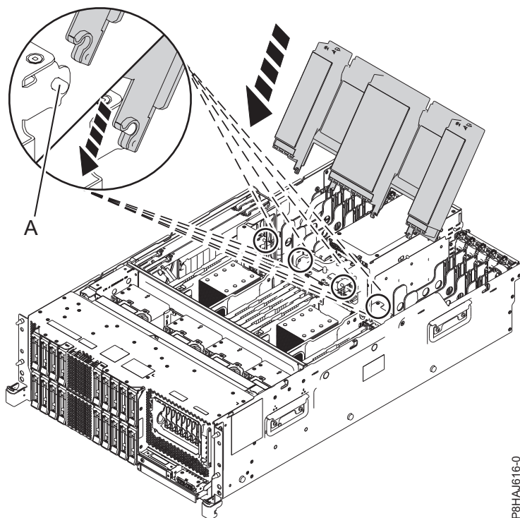
Figura 30. Substituir a conduta de ventilação
