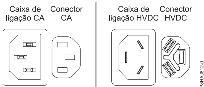
Figura 40. Conectores de AC e de HVDC
