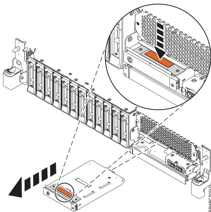
Figura 1. Remover o painel de controlo
