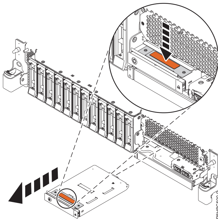
Figura 4. Remover o painel de controlo
