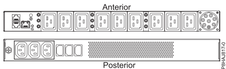
Figura 40. PDU para o sistema 8408-44E
