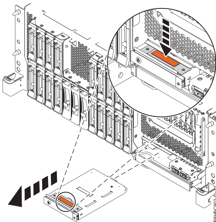
Figura 1. Remover um painel de controlo de um sistema instalado em bastidor
