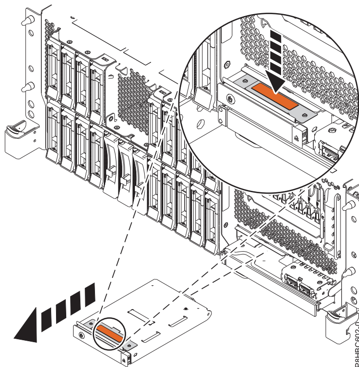
Figura 6. Remover um painel de controlo de um sistema instalado em bastidor
