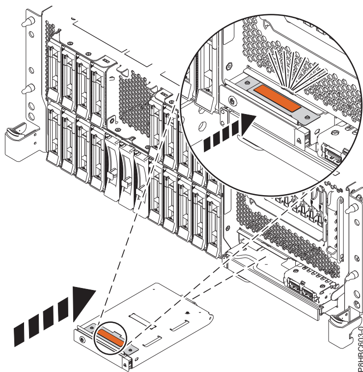
Figura 3. Substituir o painel de controlo num sistema instalado em bastidor
