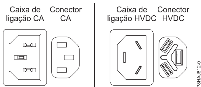
Figura 44. Conectores de AC e de HVDC
