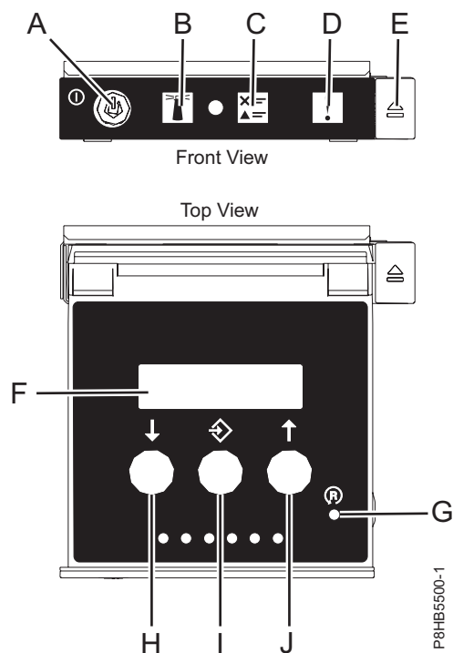
Figura 11. Painel de controlo
