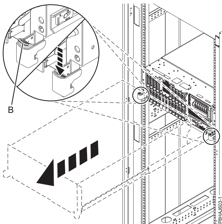
Figura 36. Soltar as patilhas laterais
