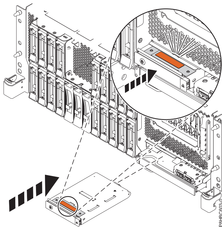
Figura 8. Substituir o painel de controlo num sistema instalado em bastidor
