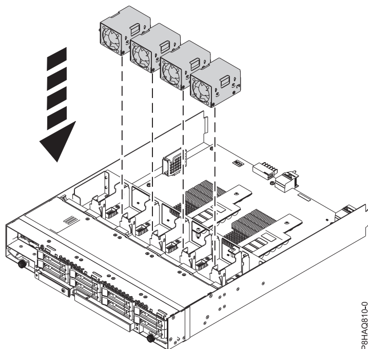
Figura 11. Substituir ventoinhas internas no conjunto RAID
