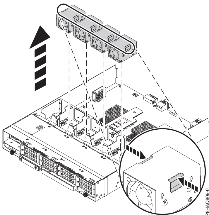
Figura 10. Remover ventoinhas internas do conjunto RAID
