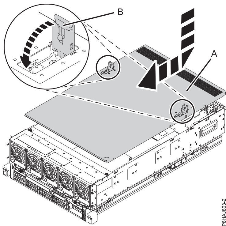
Figura 32. Instalar a tampa de acesso a assistência
