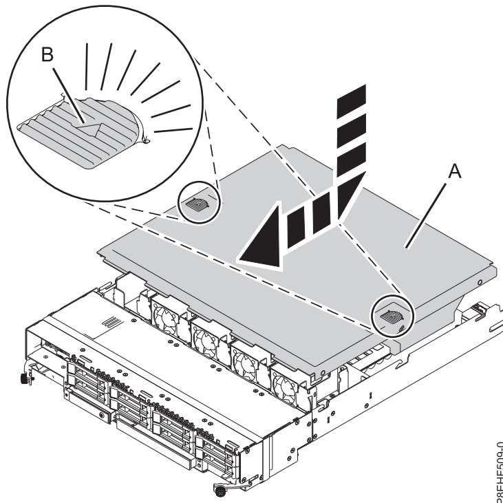
Figura 12. Substituir a tampa do conjunto RAID
