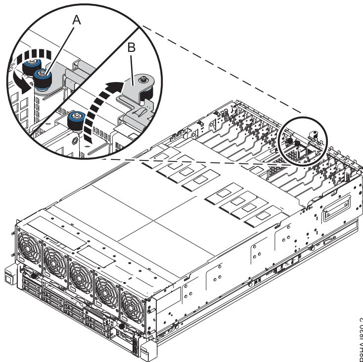
Figura 35. Abrir o trinco de E/S
