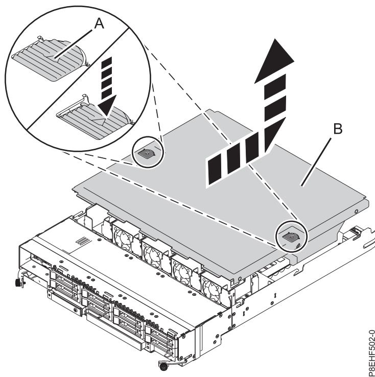
Figura 8. Remover a tampa do conjunto RAID
