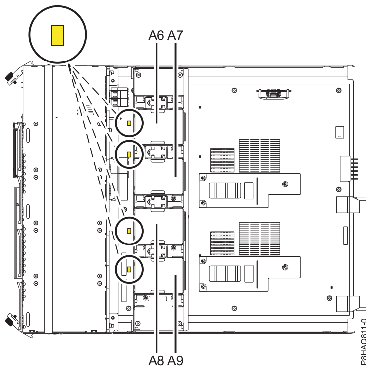
Figura 9. Localização das ventoinhas internas e LEDs de identificação
