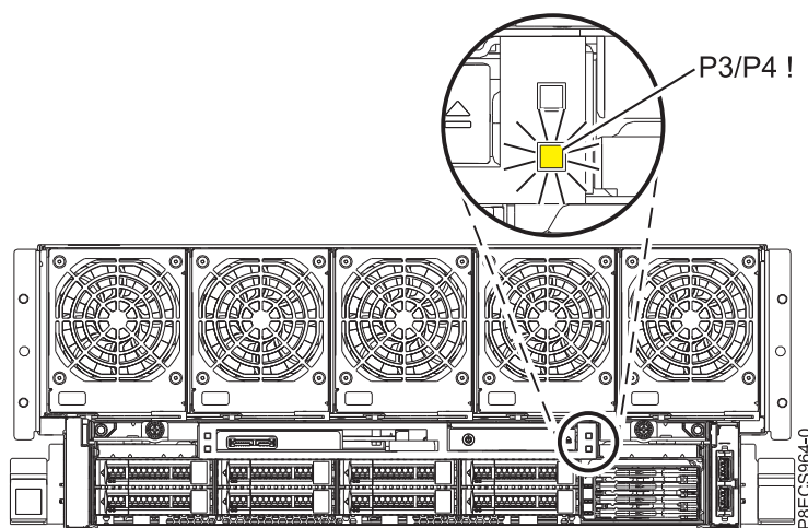
Figura 4. LED de recuo de falha P3/P4 ! frontal no sistema 8408-44E ou 8408-E8E.
