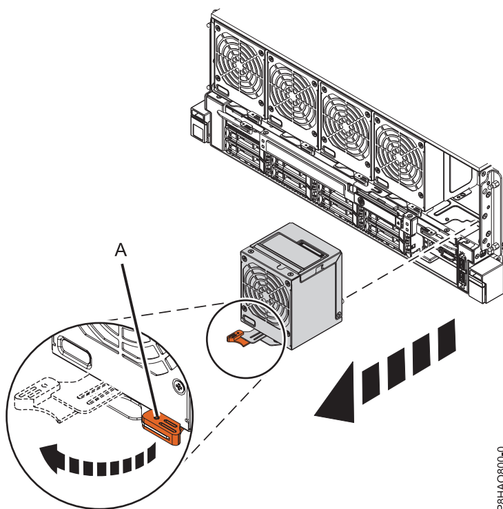
Figura 2. Remover uma ventoinha frontal do sistema
