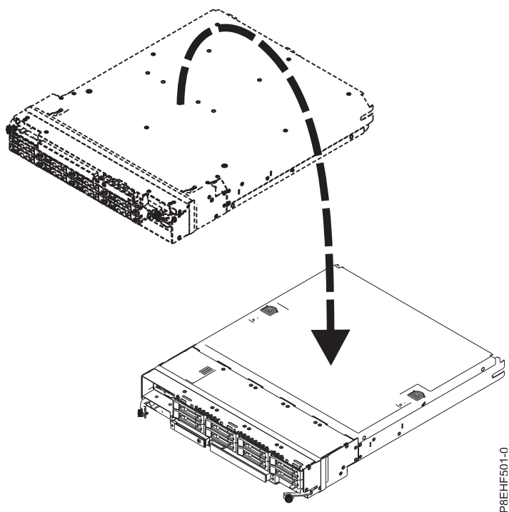
Figura 7. Virar o conjunto RAID ao contrário
