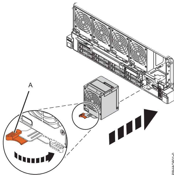
Figura 3. Substituir uma ventoinha frontal no sistema
