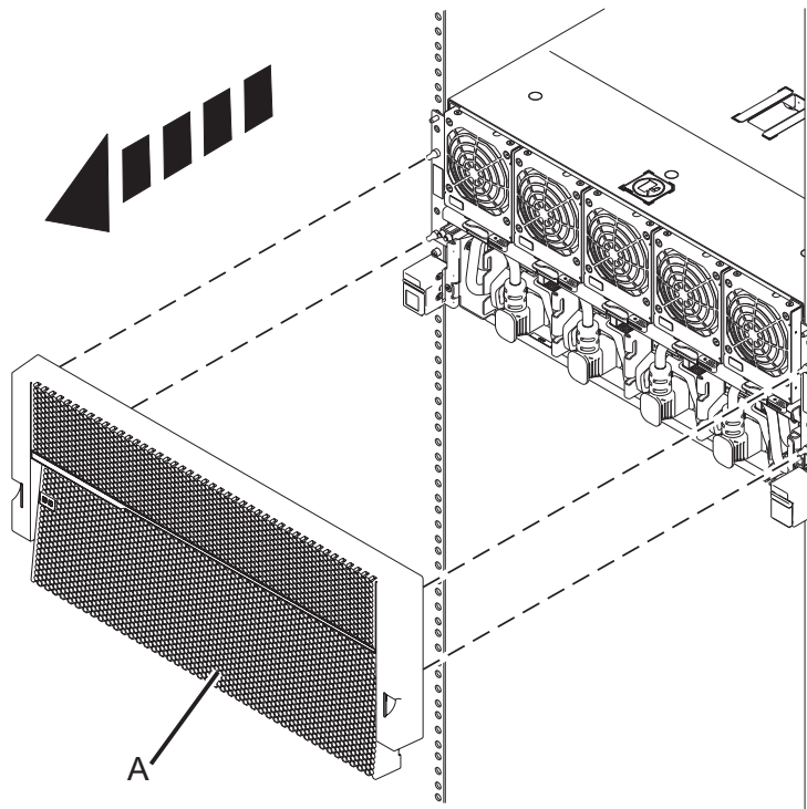
Figura 39. Remover a tampa anterior
