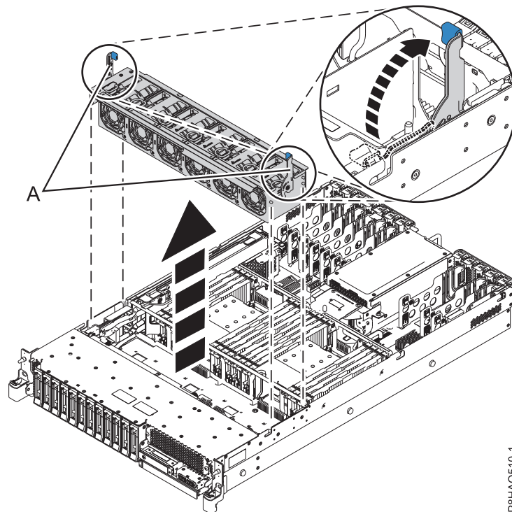
Figura 4. Remover a caixa da ventoinha
