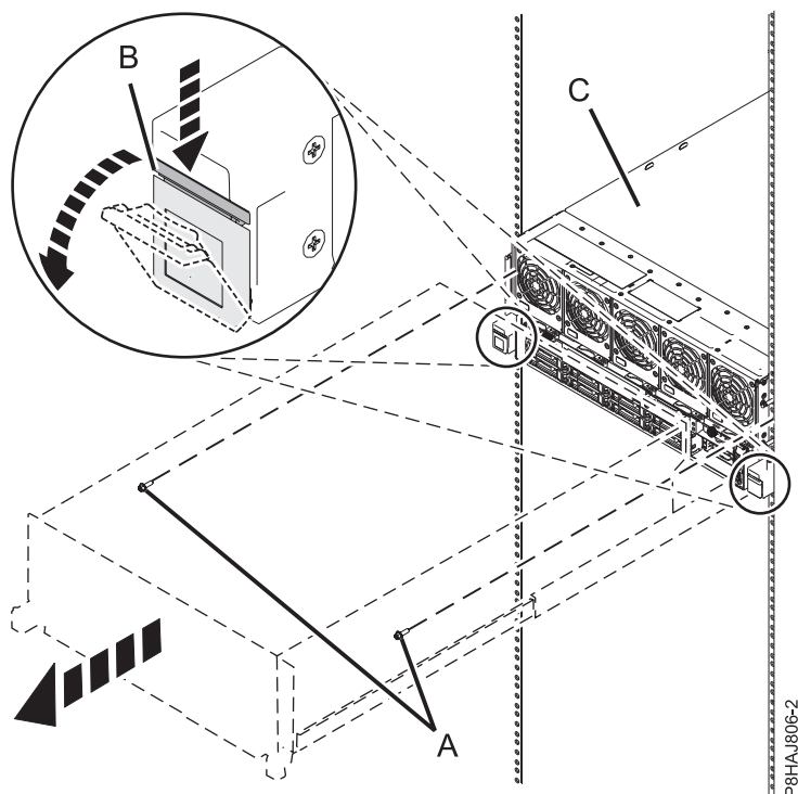
Figura 46. Colocar o sistema na posição de assistência
