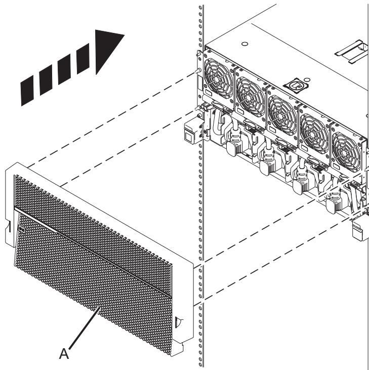
Figura 41. Instalar a tampa anterior
