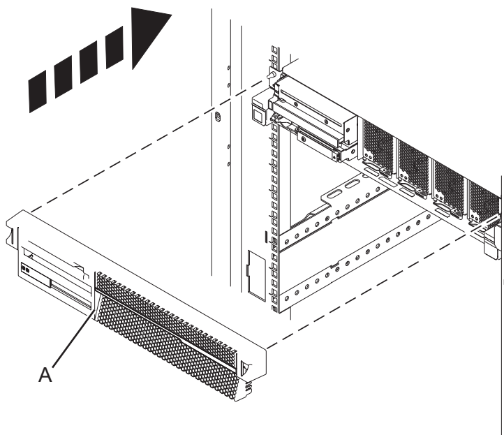
Figura 42. Instalar a tampa anterior da unidade de controlo do sistema
