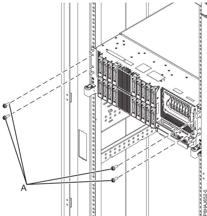
Figura 43. Remover os parafusos anteriores
