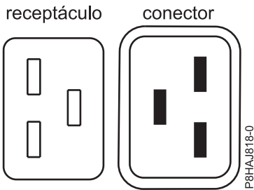
Figura 49. Conectores para o sistema 8408-44E
