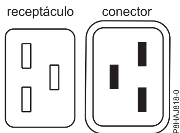
Figura 55. Conectores para o sistema 8408-44E
