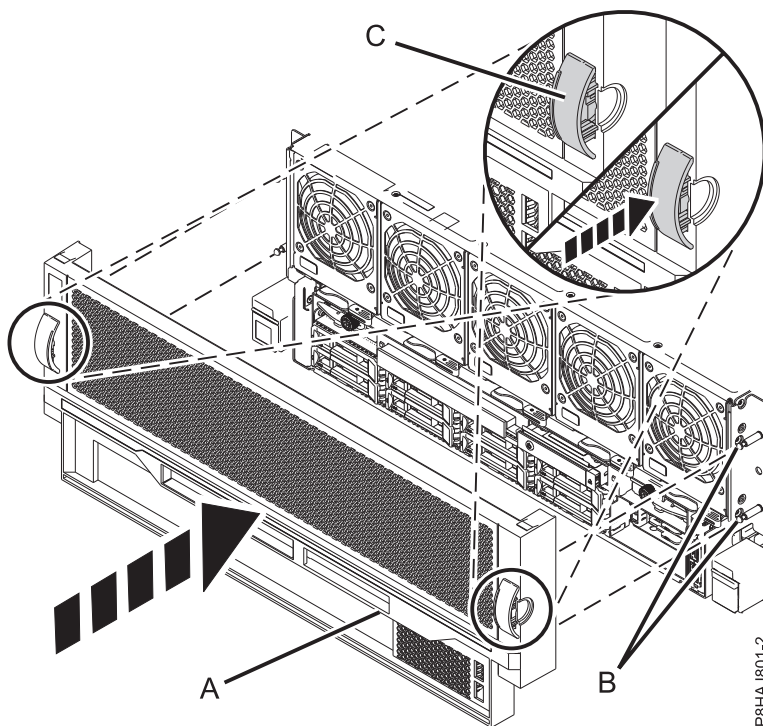
Figura 32. Instalar a tampa anterior
