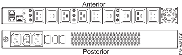
Figura 50. PDU para o sistema 8408-44E
