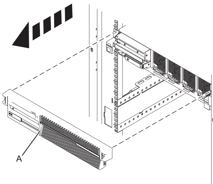
Figura 40. Remover a tampa anterior da unidade de controlo do sistema
