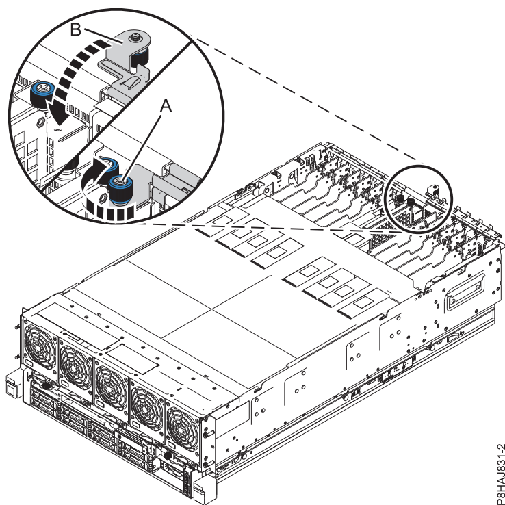
Figura 38. Fechar o trinco de E/S
