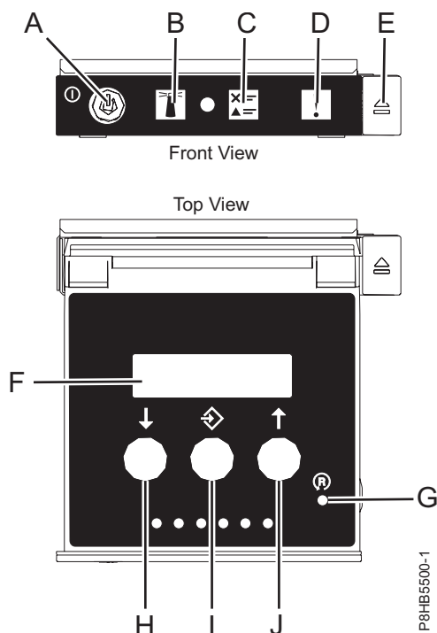
Figura 13. Painel de controlo
