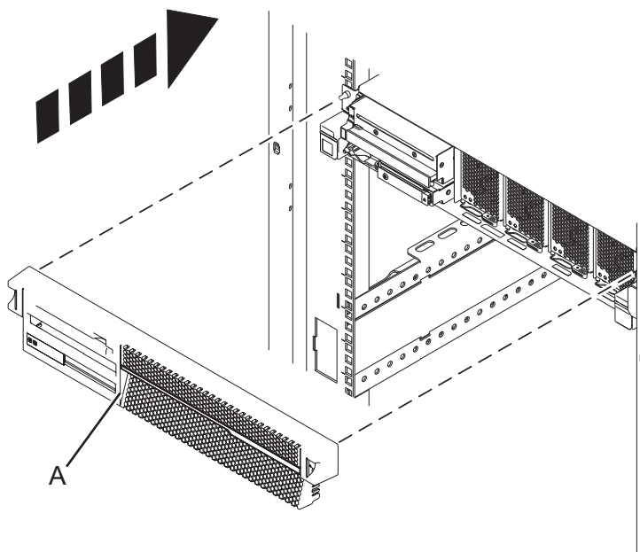
Figura 17. Instalar a tampa anterior da unidade de controlo do sistema
