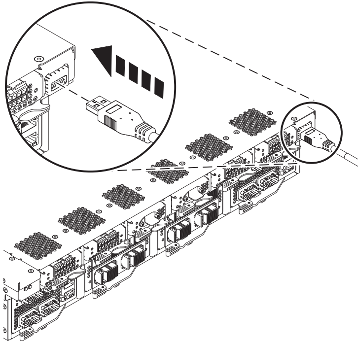
Figura 4. Ligue o cabo USB à porta USB posterior da unidade de controlo do sistema 9080-MHE, 9080-MME, 9119-MHE ou 9119-MME na ranhura P1-C11-T1
