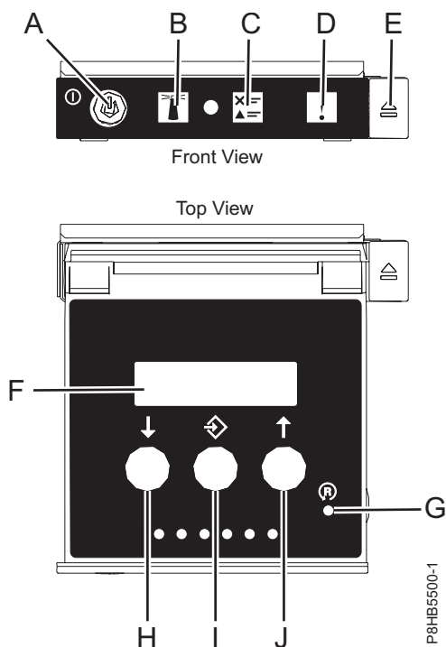
Figura 12. LEDs do painel de controlo
