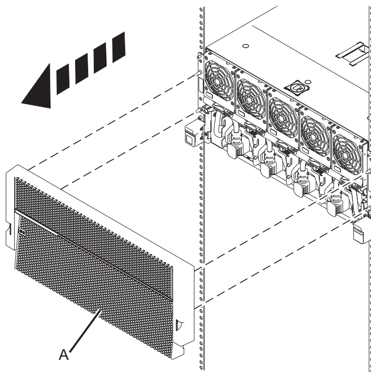
Figura 14. Remover a tampa anterior
