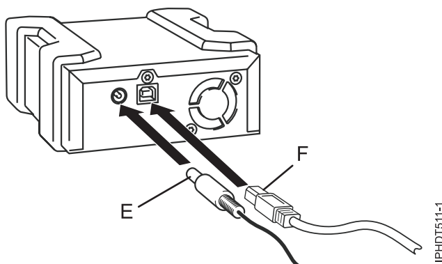
Figura 11. Ligar USB e cabos de alimentação
