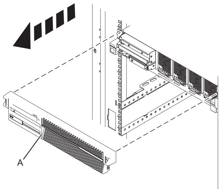
Figura 15. Remover a tampa anterior da unidade de controlo do sistema
