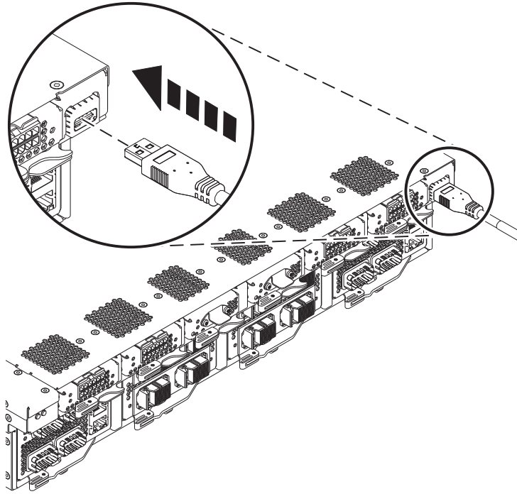
Figura 8. Ligue o cabo USB à porta USB posterior da unidade de controlo do sistema 9080-MHE, 9080-MME, 9119-MHE ou 9119-MME na ranhura P1-C11-T1
