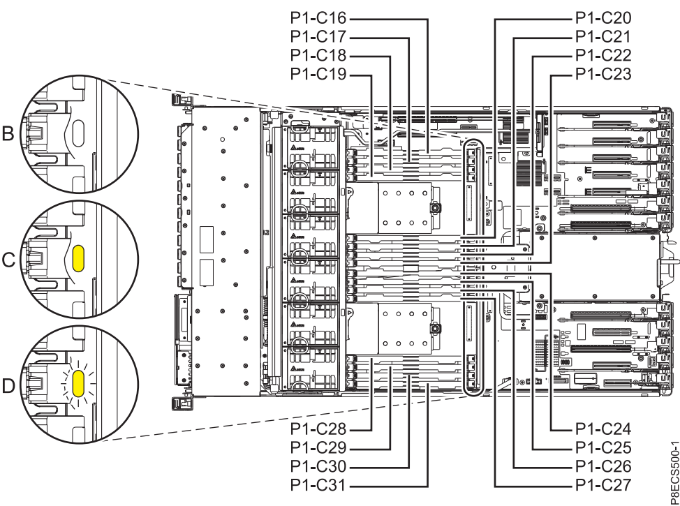
Figura 10. Sequência de ligação do módulo de memória
