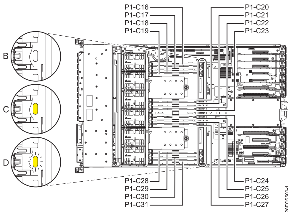
Figura 1. Localizações dos módulos de memória e os indicadores de assistência no sistema 5148-21L, 5148-22L, 8247-21L, 8247-22L, 8284-21A ou 8284-22A
