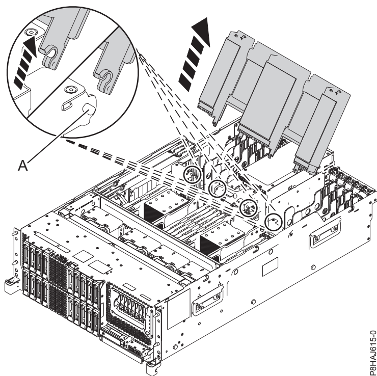
Figura 46. Remover a conduta de ventilação
