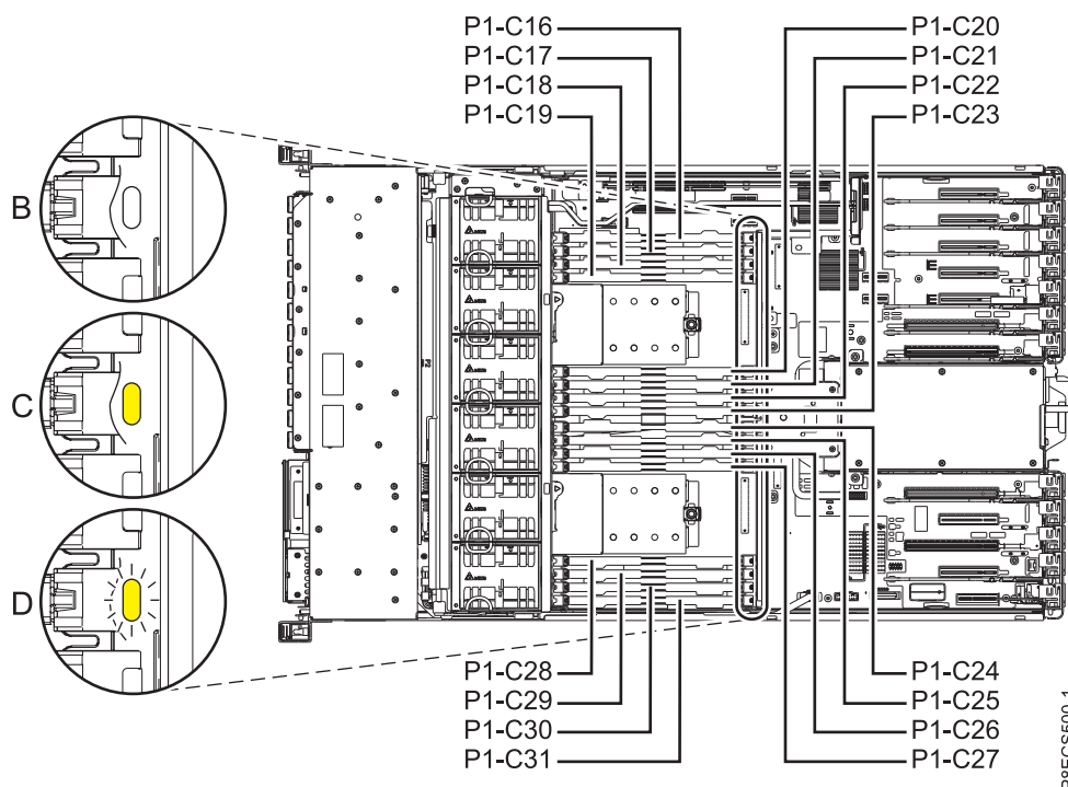
Figura 4. Localizações dos módulos de memória e os indicadores de assistência no sistema 5148-21L, 5148-22L, 8247-21L, 8247-22L, 8284-21A ou 8284-22A
