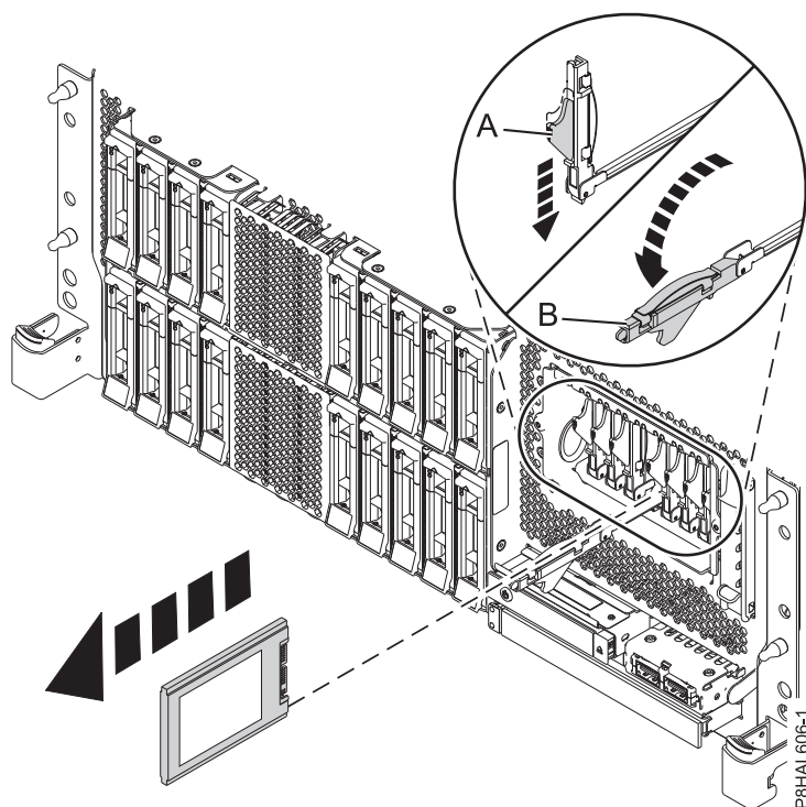
Figura 91. Remover uma unidade SSD de um sistema de função expandida montado em bastidor
