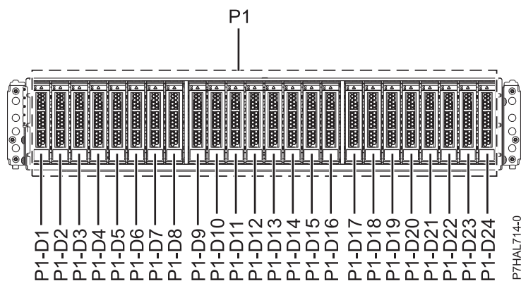
Figura 145. Vista anterior do 5887 suporte de unidades de disco mostrando a localização das unidades de disco
