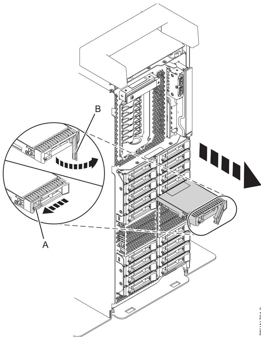
Figura 60. Remover uma unidade de disco de um sistema de função expandida autônomo
