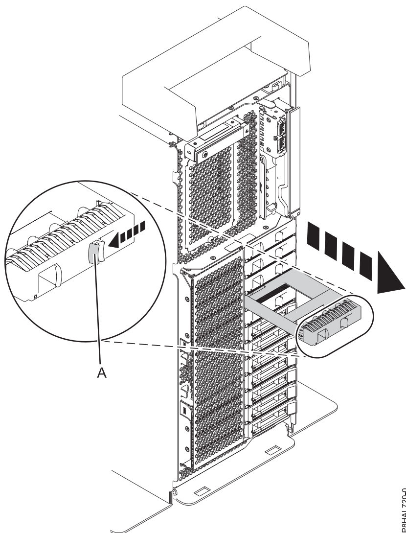
Figura 135. Remover um enchimento de uma unidade de disco de um sistema de função base autónomo
