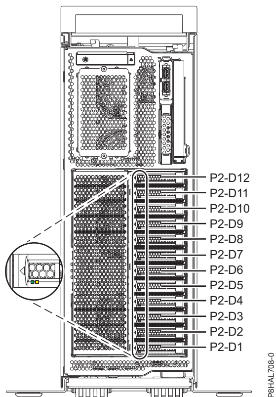
Figura 55. Localizações da unidade de disco, da unidade de disco de segunda geração e do indicador de assistência num sistema função base 8286-41A autónomo
