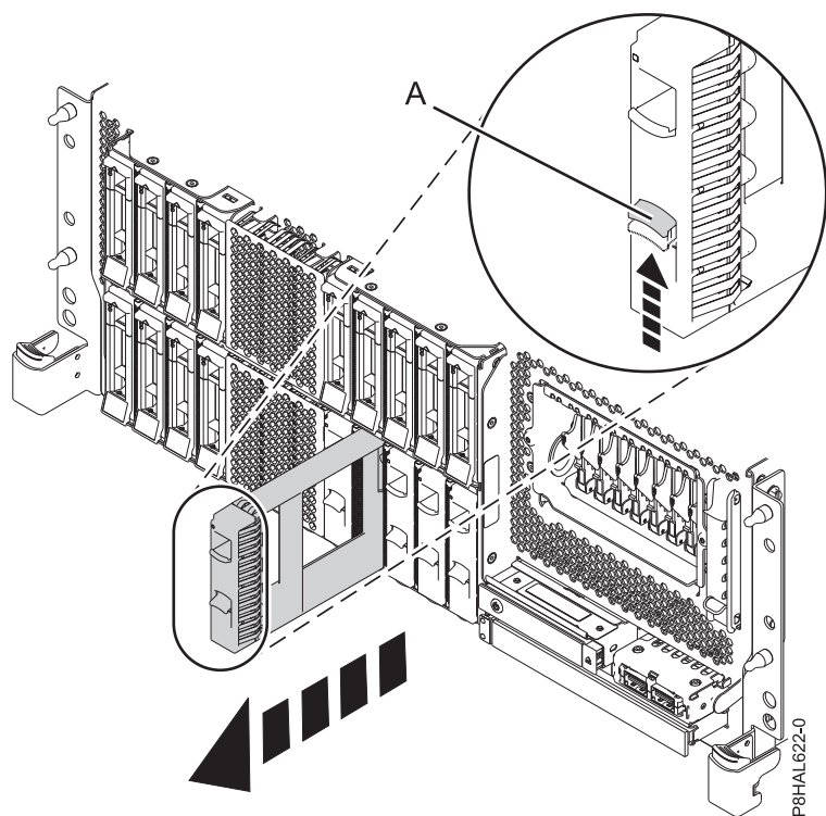
Figura 134. Remover um enchimento de uma unidade de disco num sistema de função expandida montado em bastidor
