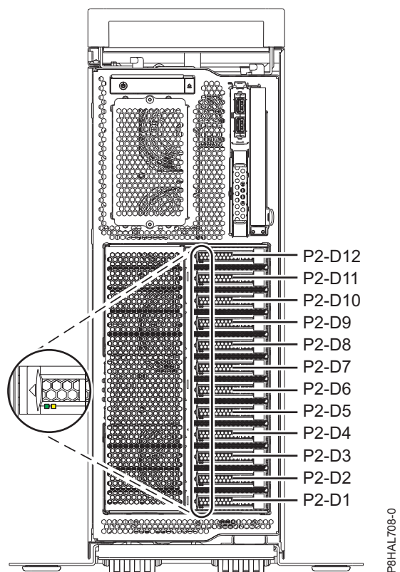
Figura 12. Localizações da unidade de disco, da unidade de disco de segunda geração e do indicador de assistência num sistema função base 8286-41A autónomo
