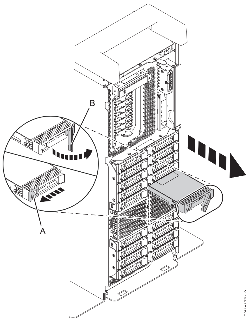
Figura 90. Remover uma unidade de disco de um sistema de função expandida autónomo
