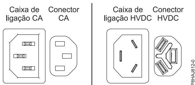
Figura 162. Conectores de AC e de HVDC
