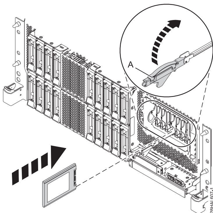
Figura 25. Instalar uma unidade SSD num sistema de função expandida montado em bastidor
