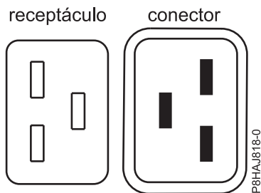
Figura 163. Conectores para o sistema 8408-44E
