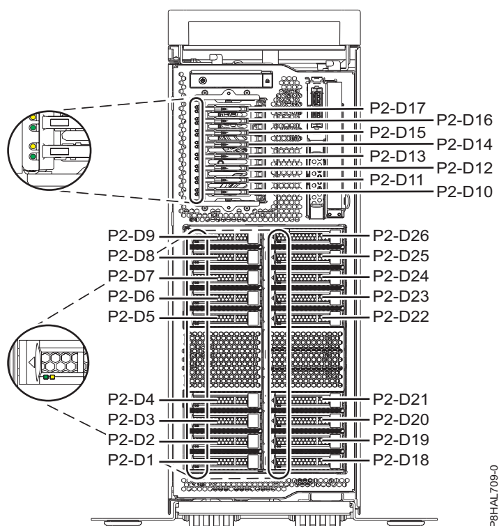
Figura 144. Localização da unidade de disco, unidade de segunda geração e indicador de assistência num sistema de função expandida 8286-41A autónomo
