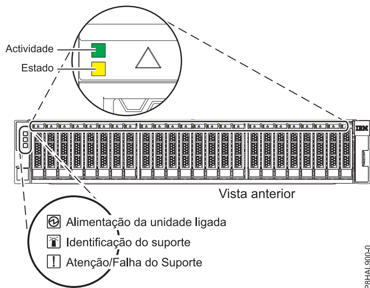
Figura 151. Vista anterior do suporte que demonstra os indicadores de assistência
