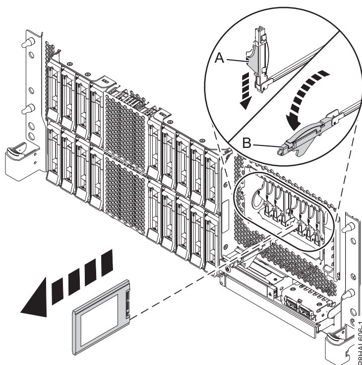
Figura 105. Remover uma unidade SSD de um sistema de função expandida montado em bastidor
