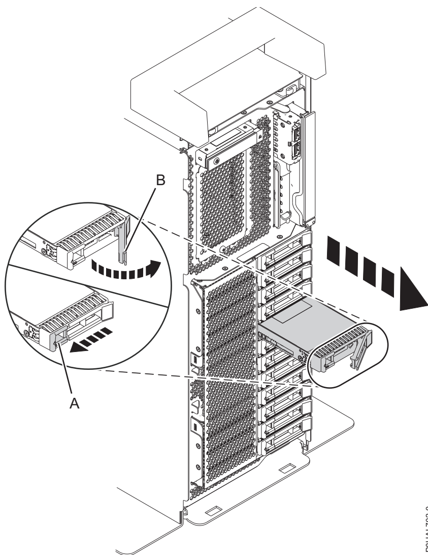
Figura 59. Remover uma unidade de disco de um sistema de função base autónomo
