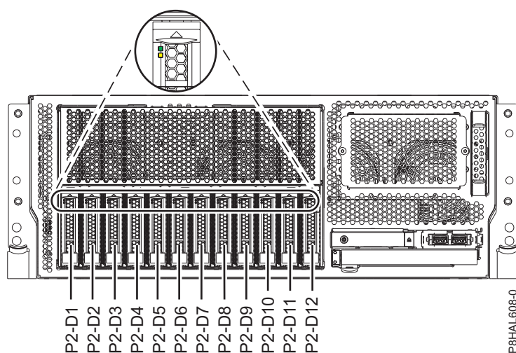
Figura 10. Localizações da unidade de disco, da unidade de disco de segunda geração e do indicador de assistência num sistema função base 8247-42L, 8286-41A ou 8286-42A montado em bastidor
