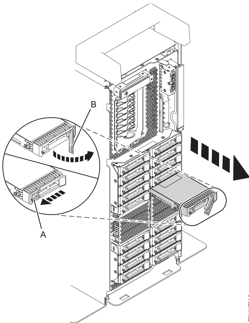
Figura 104. Remover uma unidade de disco de um sistema de função expandida autónomo
