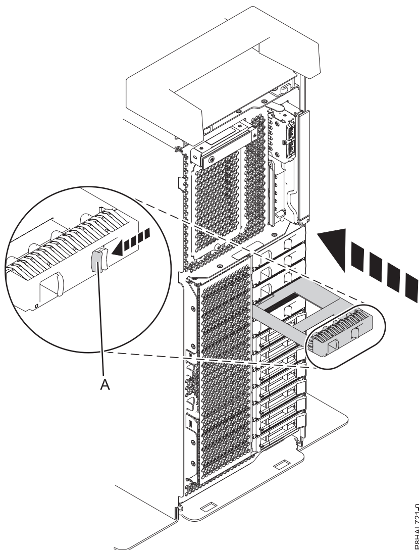
Figura 139. Instalar um enchimento de uma unidade num sistema de função base autónomo
