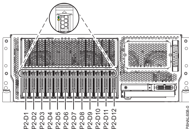
Figura 27. Localizações da unidade de disco, da unidade de disco de segunda geração e do indicador de assistência num sistema função base 8247-42L, 8286-41A ou 8286-42A montado em bastidor
