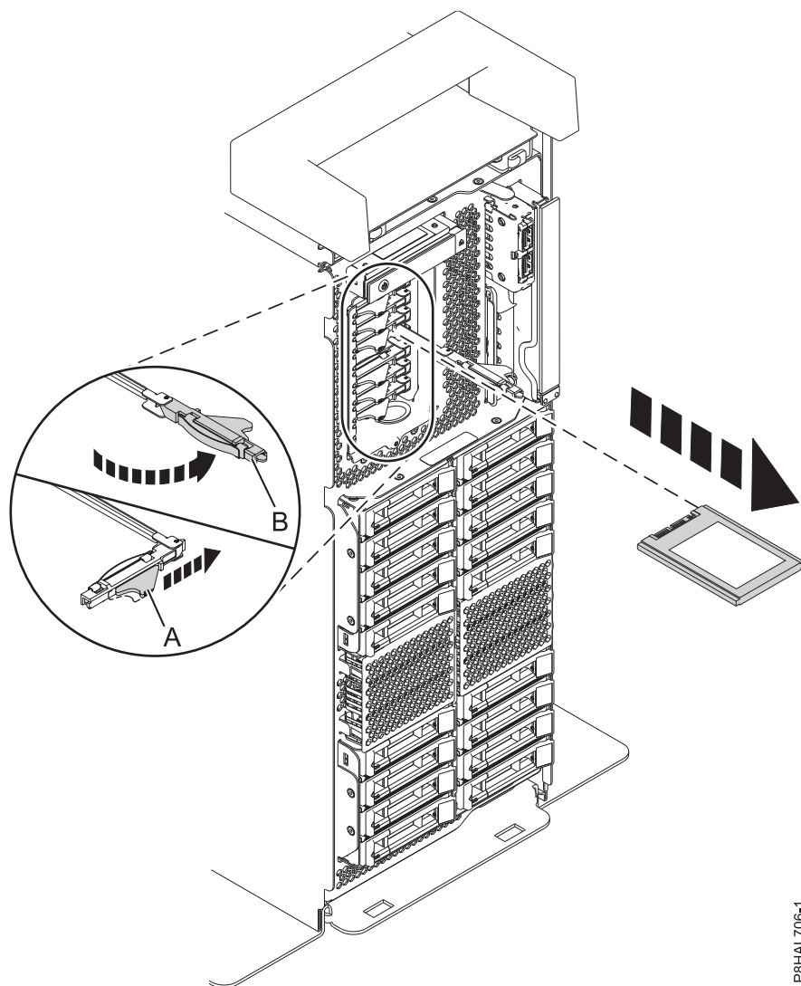
Figura 62. Remover uma unidade SSD de um sistema de função expandida autónomo
