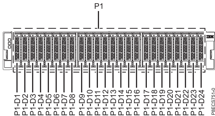
Figura 149. Vista anterior da unidade de expansão ESLS que demonstra as localizações das unidades de disco
