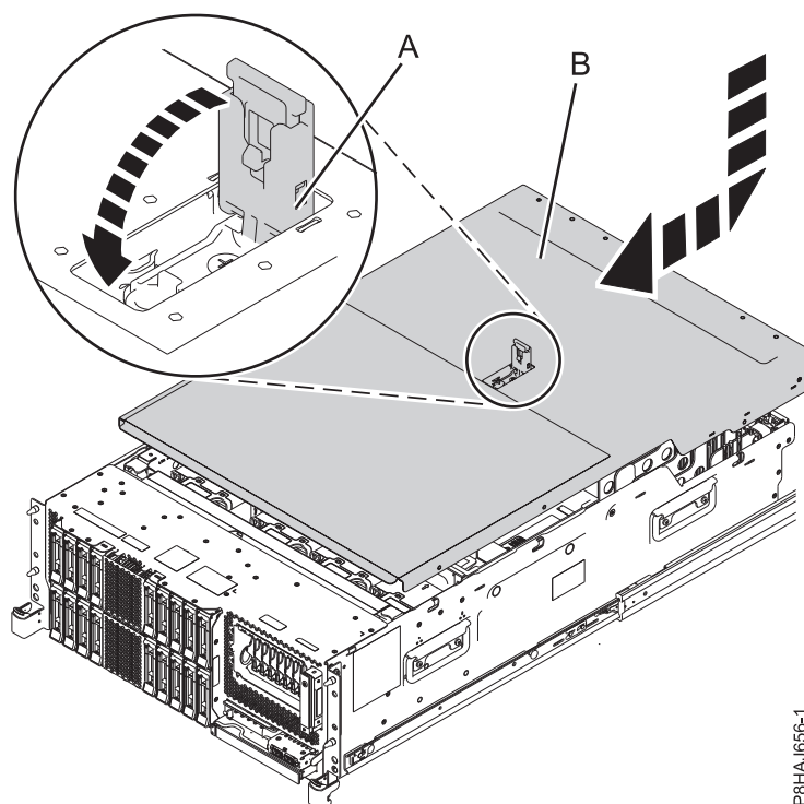
Figura 185. Instalar a tampa de acesso para assistência
