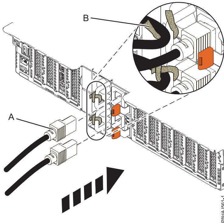
Figura 166. Ligar os cabos de alimentação a um sistema 5148-21L, 5148-22L, 8247-21L, 8247-22L, 8284-21A ou 8284-22A
