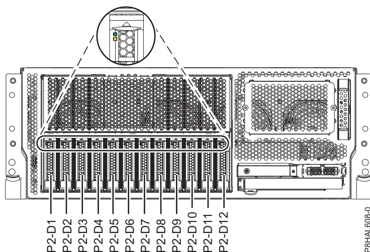
Figura 40. Localizações da unidade de disco, da unidade de disco de segunda geração e do indicador de assistência num sistema função base 8247-42L, 8286-41A ou 8286-42A montado em bastidor
