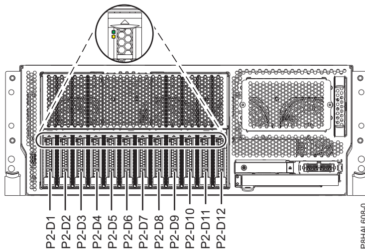
Figura 16. Localizações da unidade de disco, da unidade de disco de segunda geração e do indicador de assistência num sistema função base 8247-42L, 8286-41A ou 8286-42A montado em bastidor
