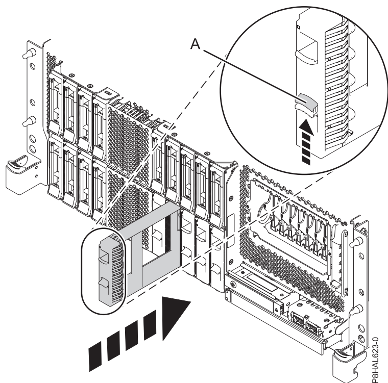
Figura 138. Instalar um enchimento de uma unidade de disco num sistema de função expandida montado em bastidor
