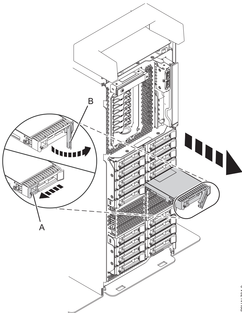
Figura 121. Remover uma unidade de disco de um sistema de função expandida autónomo
