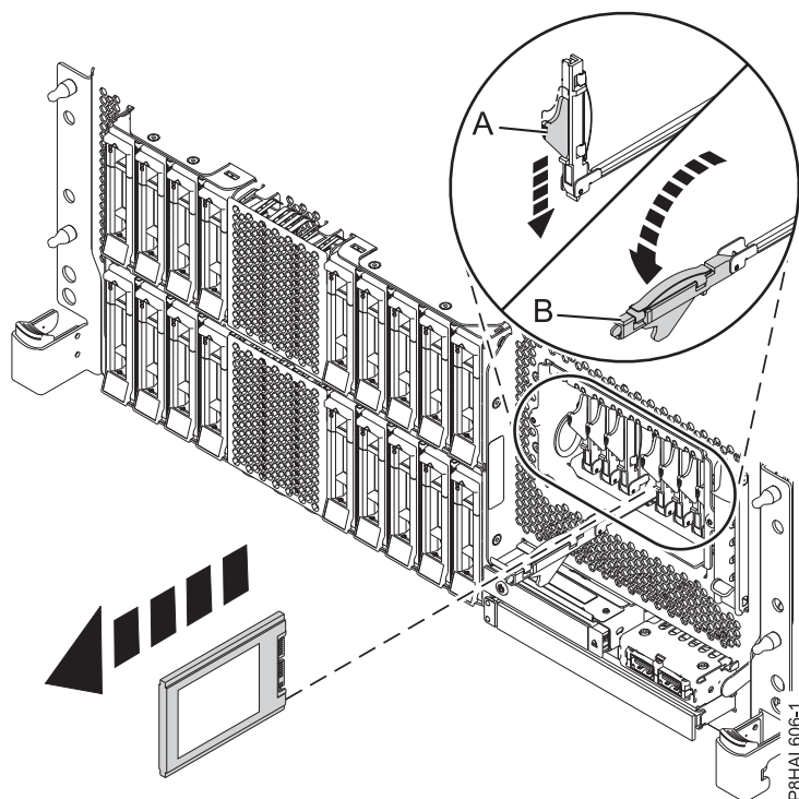
Figura 77. Remover uma unidade SSD de um sistema de função expandida montado em bastidor
