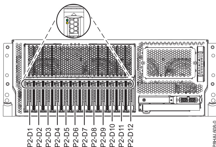
Figura 53. Localizações da unidade de disco, da unidade de disco de segunda geração e do indicador de assistência num sistema função base 8247-42L, 8286-41A ou 8286-42A montado em bastidor
