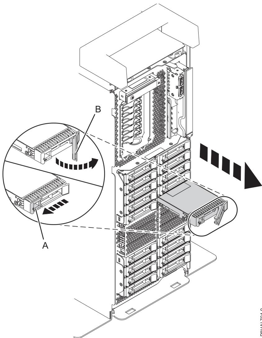
Figura 76. Remover uma unidade de disco de um sistema de função expandida autônomo
