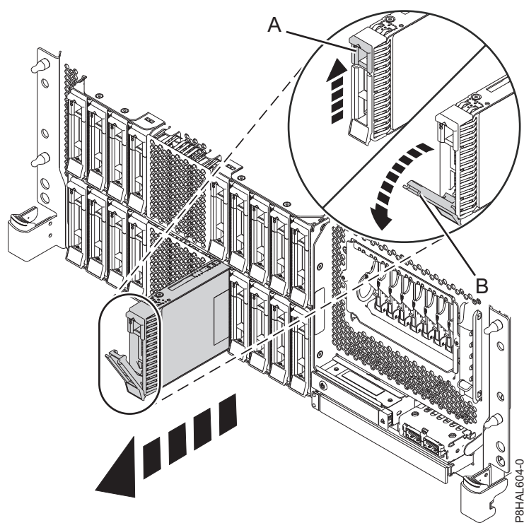
Figura 119. Remover uma unidade de disco de um sistema de função expandida montado em bastidor
