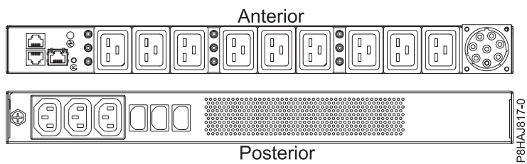
Figura 158. PDU para o sistema 8408-44E
