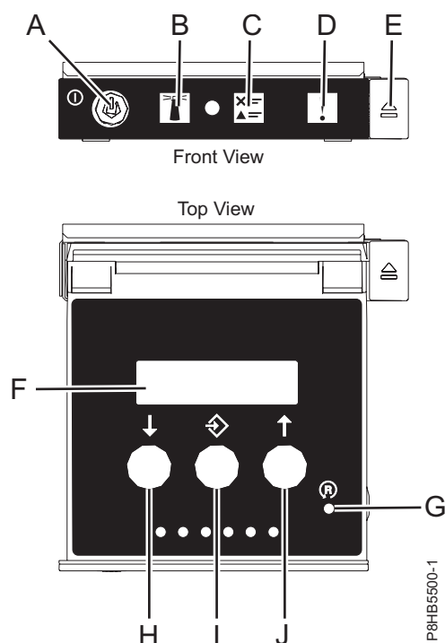
Figura 155. Painel de controlo
