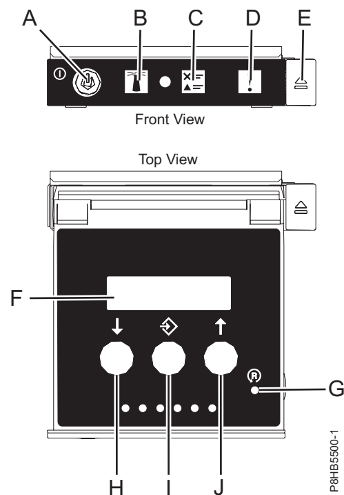
Figura 154. LEDs do painel de controlo
