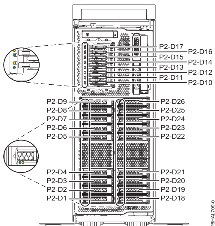
Figura 4. Localização da unidade de disco, unidade de segunda geração e indicador de assistência num sistema de função expandida 8286-41A autônomo
