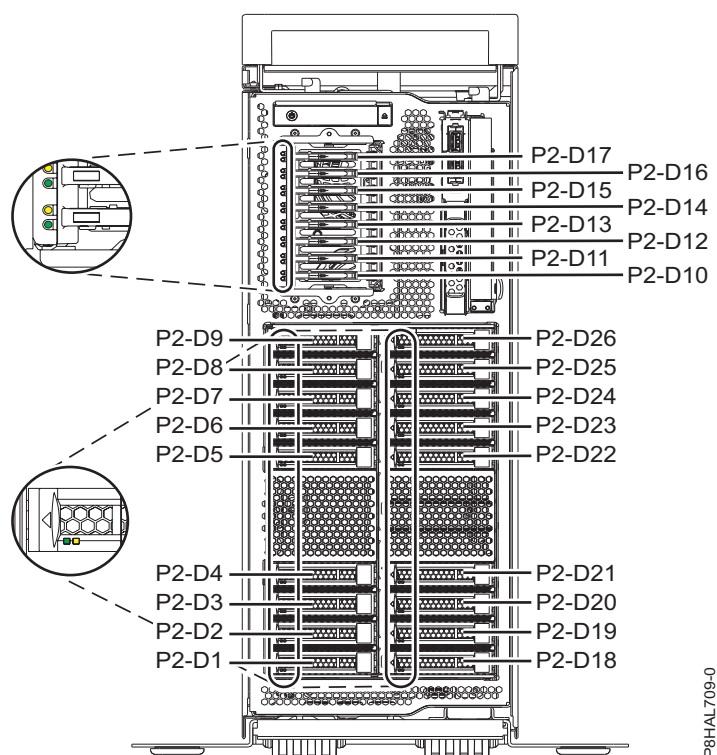
Figura 30. Localização da unidade de disco, unidade de segunda geração e indicador de assistência num sistema de função expandida 8286-41A autónomo
