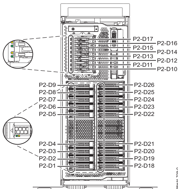
Figura 19. Localização da unidade de disco, unidade de segunda geração e indicador de assistência num sistema de função expandida 8286-41A autónomo
