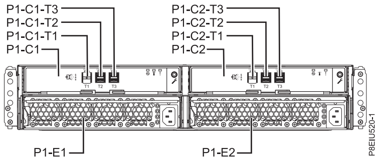
Figura 150. Vista posterior do suporte
