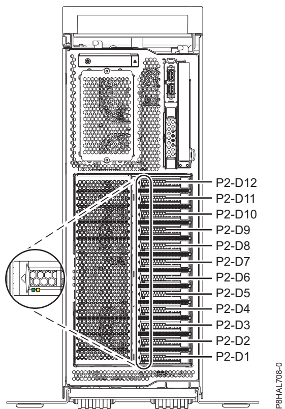
Figura 143. Localizações da unidade de disco, da unidade de disco de segunda geração e do indicador de assistência num sistema função base 8286-41A autónomo
