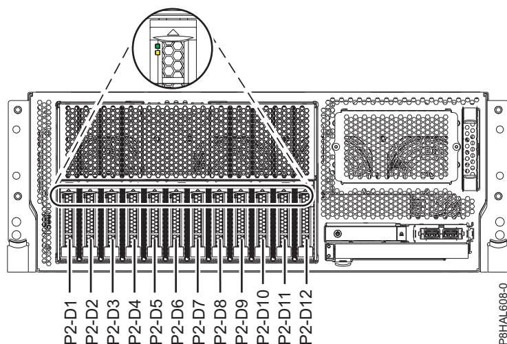
Figura 141. Localizações da unidade de disco ou da unidade de disco de segunda geração e do indicador de assistência num sistema função base 8247-42L, 8286-41A ou 8286-42A montado em bastidor
