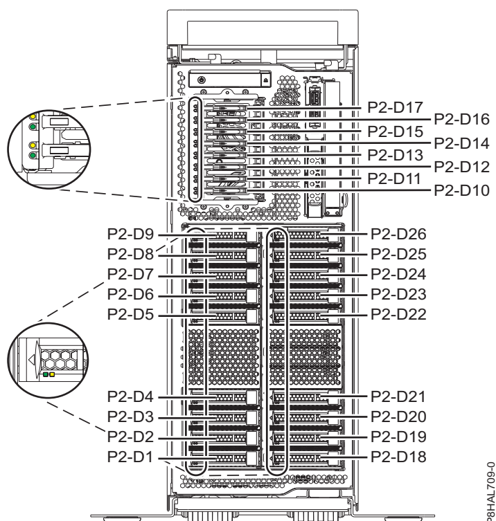
Figura 13. Localização da unidade de disco, unidade de segunda geração e indicador de assistência num sistema de função expandida 8286-41A autónomo
