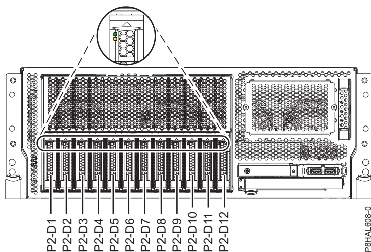
Figura 1. Localizações da unidade de disco, da unidade de disco de segunda geração e do indicador de assistência num sistema função base 8247-42L, 8286-41A ou 8286-42A montado em bastidor
