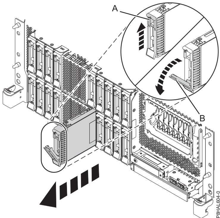
Figura 88. Remover uma unidade de disco de um sistema de função expandida montado em bastidor
