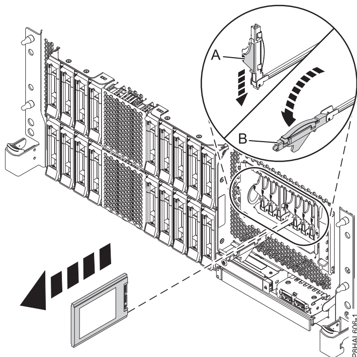
Figura 122. Remover uma unidade SSD de um sistema de função expandida montado em bastidor
