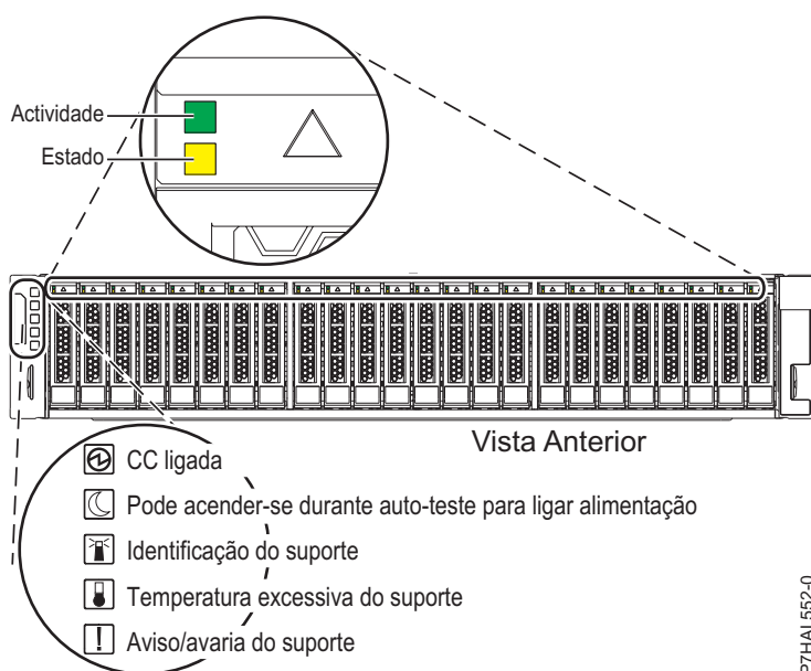
Figura 147. Vista anterior do 5887 suporte de unidades de disco mostrando os indicadores de assistência
