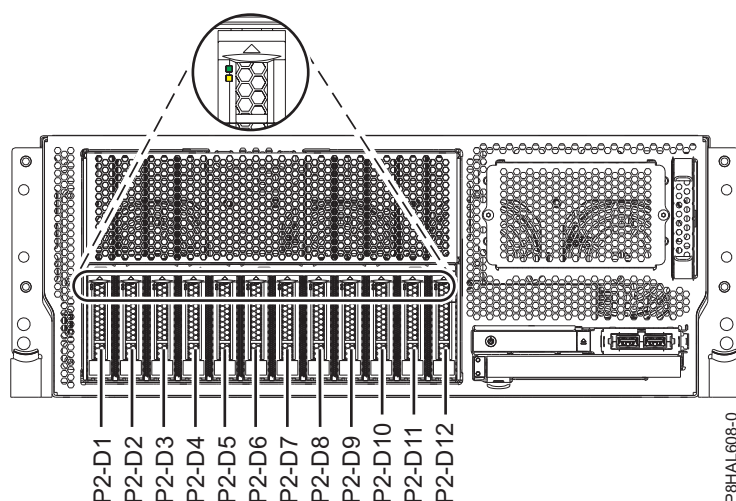
Figura 69. Localizações da unidade de disco, da unidade de disco de segunda geração e do indicador de assistência num sistema função base 8247-42L, 8286-41A ou 8286-42A montado em bastidor
