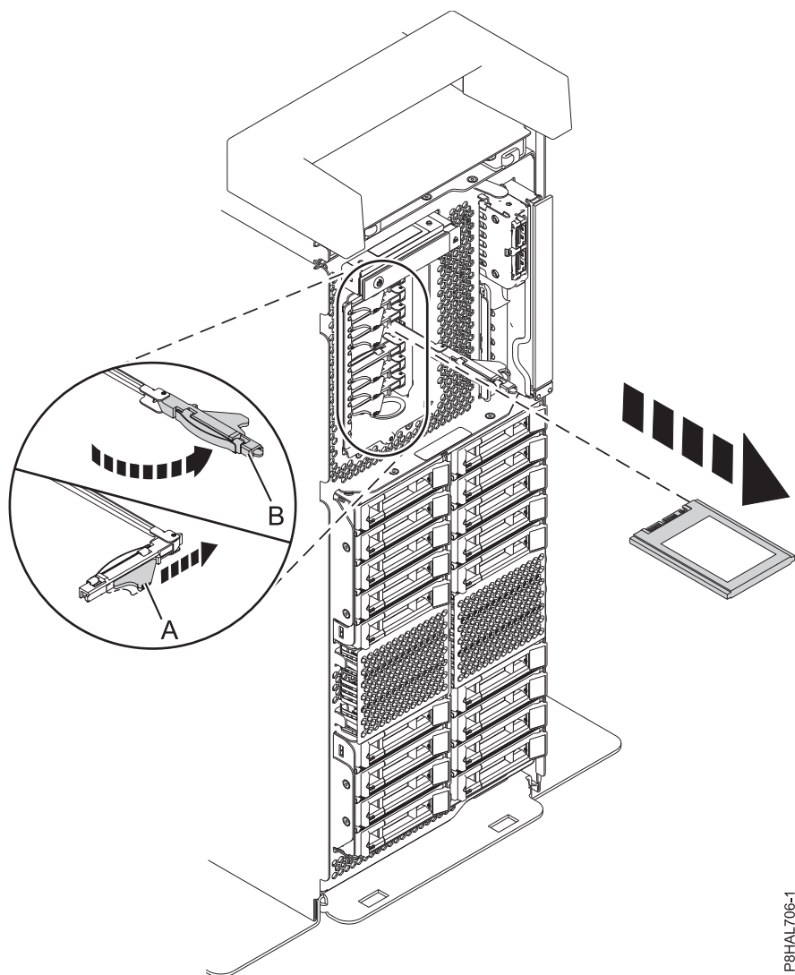
Figura 92. Remover uma unidade SSD de um sistema de função expandida autónomo
