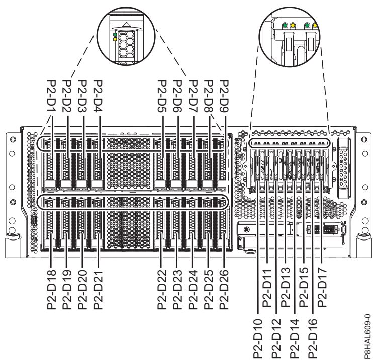
Figura 11. Localização da unidade de disco, unidade de segunda geração e indicadores de assistência num sistema de função expandida 8286-41A ou 8286-42A montado em bastidor
