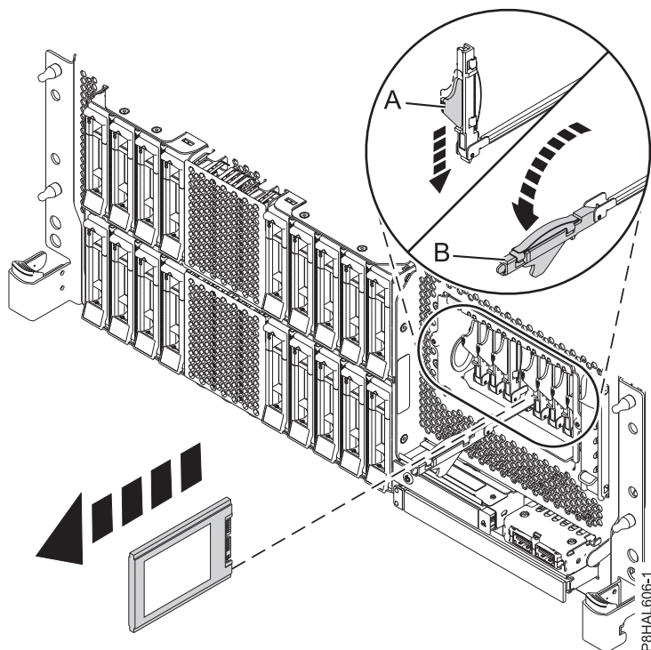
Figura 61. Remover uma unidade SSD de um sistema de função expandida montado em bastidor
