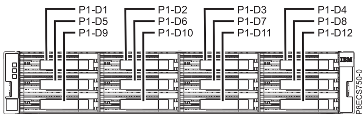
Figura 148. Vista anterior da unidade de expansão ESLL que demonstra as localizações das unidades de disco
