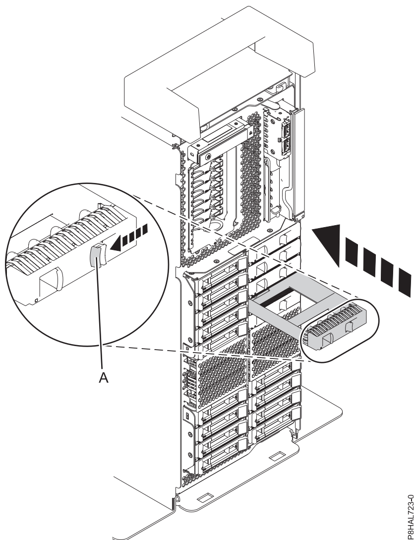
Figura 140. Instalar um enchimento de uma unidade de disco num sistema de função expandida autônomo
