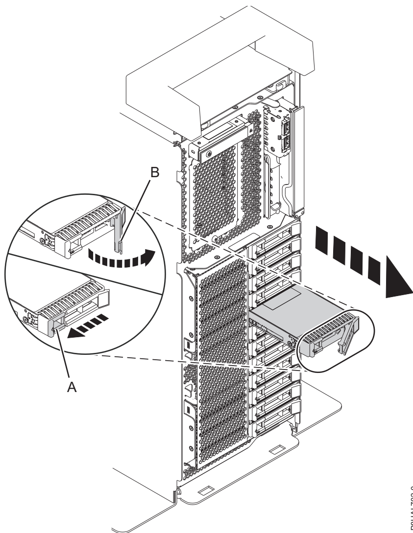
Figura 89. Remover uma unidade de disco de um sistema de função base autónomo
