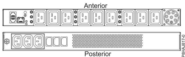
Figura 164. PDU para o sistema 8408-44E
