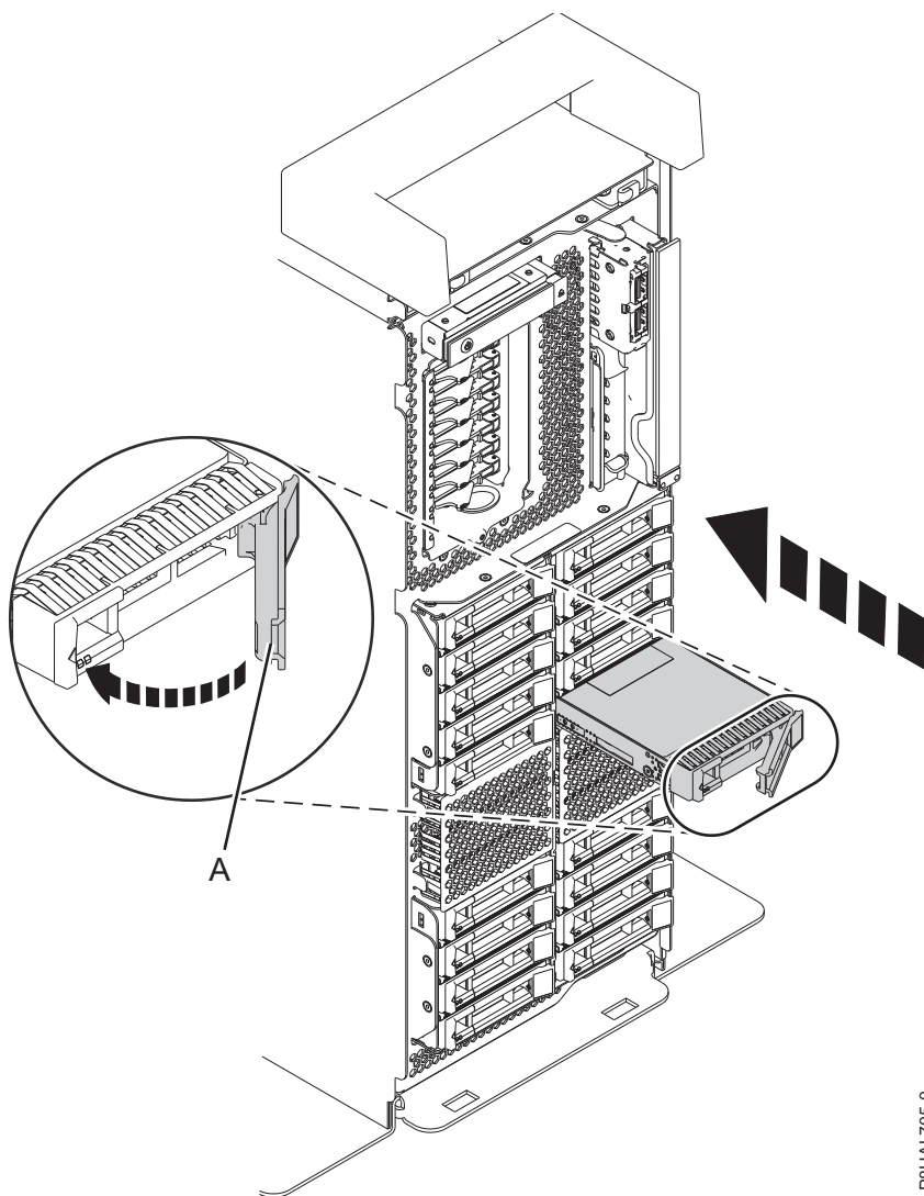
Figura 82. Substituir uma unidade de disco num sistema de função expandida autónomo
