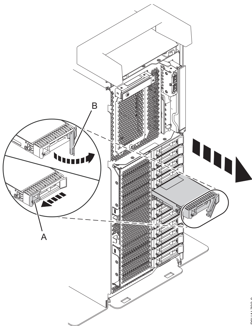
Figura 103. Remover uma unidade de disco de um sistema de função base autónomo
