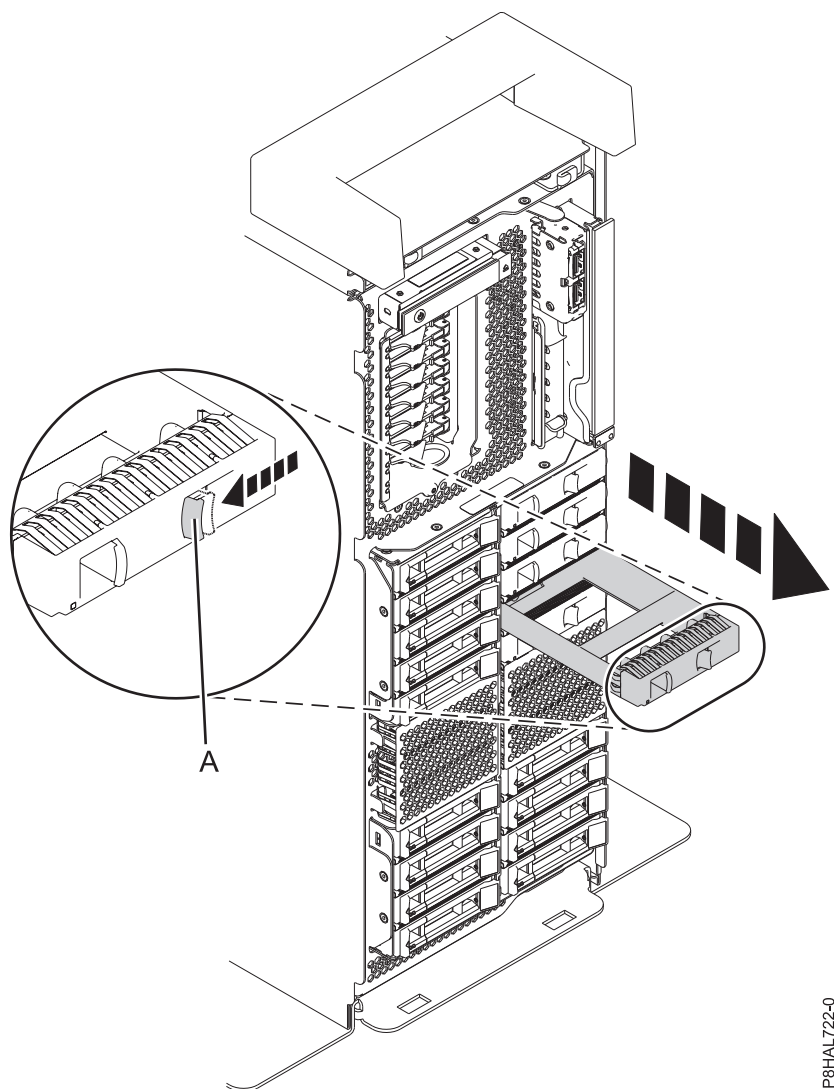
Figura 136. Remover um enchimento de uma unidade de disco de um sistema de função expandida autónomo
