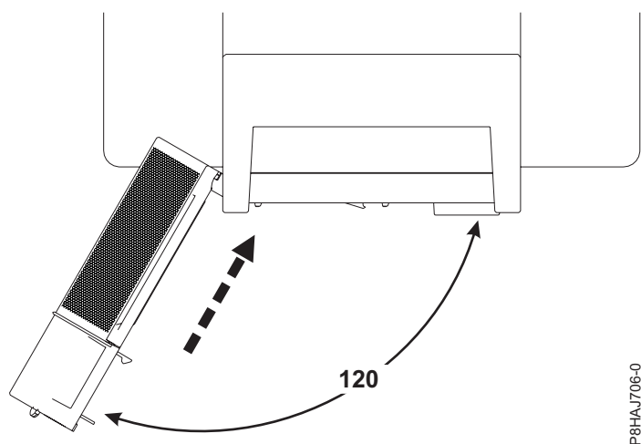
Figura 65. Rodar a tampa frontal
