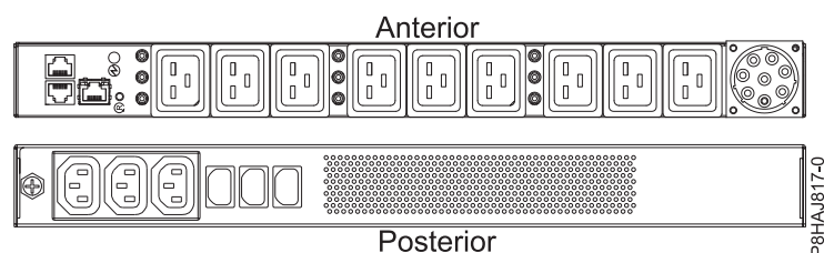
Figura 45. PDU para o sistema 8408-44E
