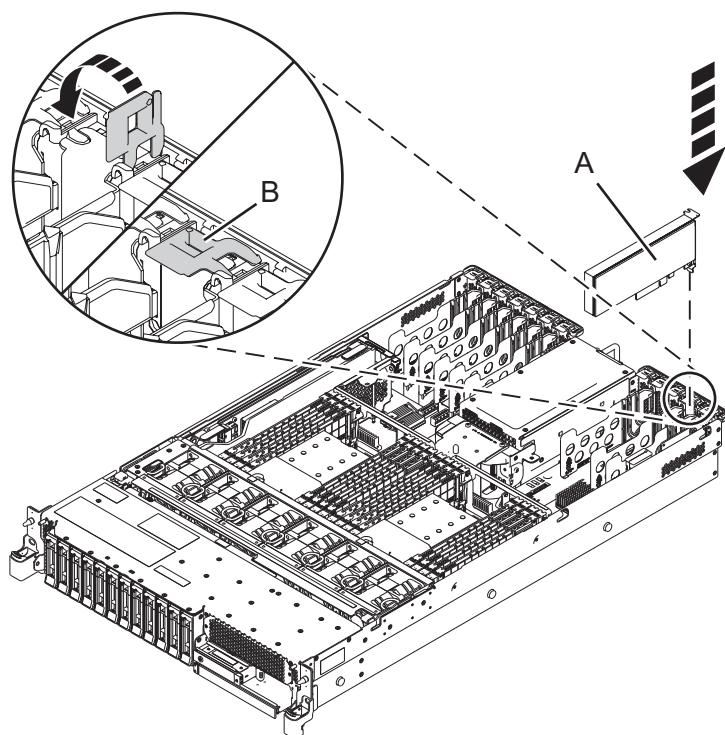
Figura 22. Instalar ou substituir um adaptador PCIe no sistema 5148-21L, 5148-22L, 8247-21L, 8247-22L, 8284-21A ou 8284-22A
