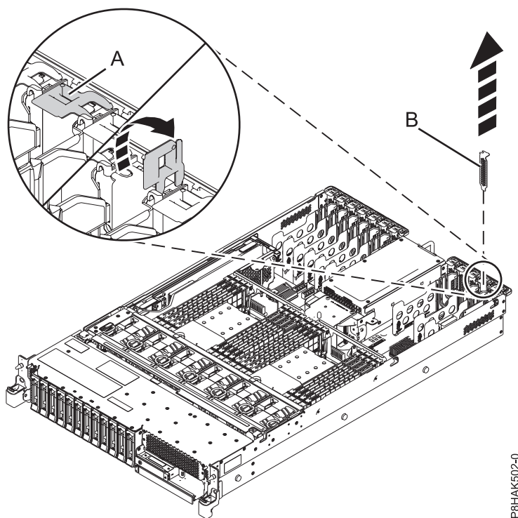
Figura 28. Remover um enchimento da ranhura do adaptador PCIe num sistema 5148-21L, 5148-22L, 8247-21L, 8247-22L, 8284-21A ou 8284-22A
