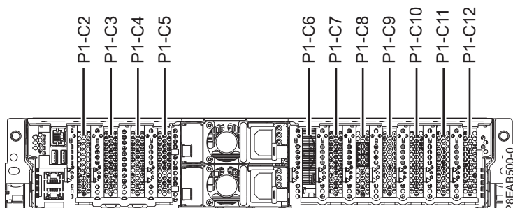
Figura 10. Localizações de ranhuras de adaptadores PCIe num sistema 5148-21L, 5148-22L, 8247-21L, 8247-22L, 8284-21A ou 8284-22A
