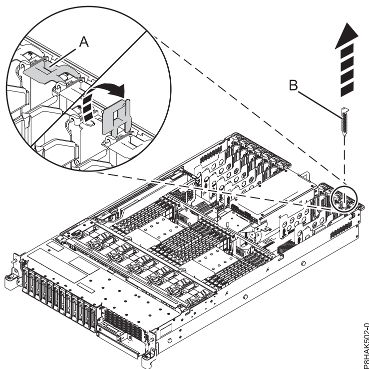
Figura 11. Remover um enchimento da ranhura do adaptador PCIe num sistema 5148-21L, 5148-22L, 8247-21L, 8247-22L, 8284-21A ou 8284-22A
