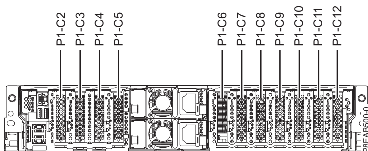
Figura 7. Localizações de ranhuras de adaptadores PCIe num sistema 5148-21L, 5148-22L, 8247-21L, 8247-22L, 8284-21A ou 8284-22A
