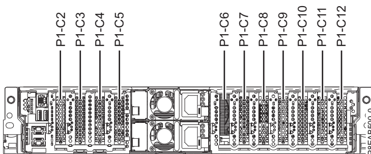
Figura 4. Localizações de ranhuras de adaptadores PCIe num sistema 5148-21L, 5148-22L, 8247-21L, 8247-22L, 8284-21A ou 8284-22A
