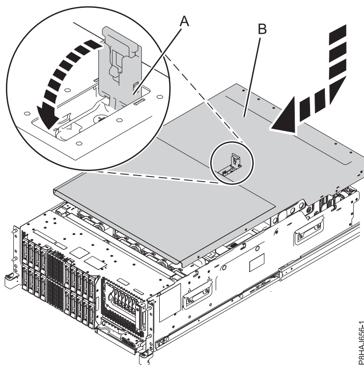
Figura 72. Instalar a tampa de acesso a assistência
