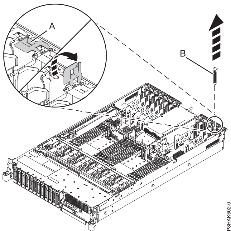
Figura 5. Remover um enchimento da ranhura do adaptador PCIe num sistema 5148-21L, 5148-22L, 8247-21L, 8247-22L, 8284-21A ou 8284-22A
