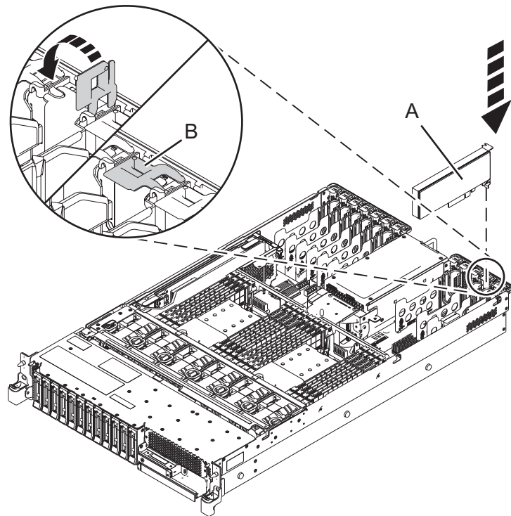
Figura 35. Instalar ou substituir um adaptador PCIe no sistema 5148-21L, 5148-22L, 8247-21L, 8247-22L, 8284-21A ou 8284-22A
