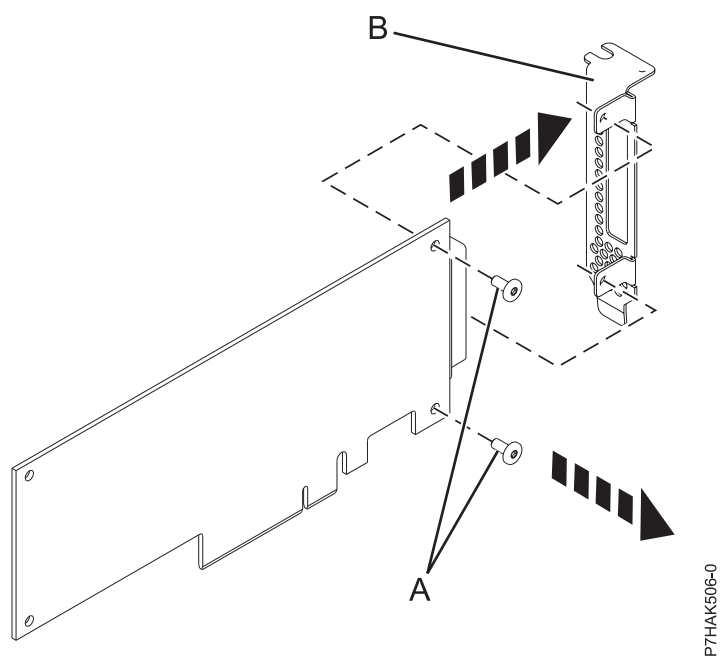
Figura 36. Remover o contraponto de baixo perfil de um adaptador PCIe
