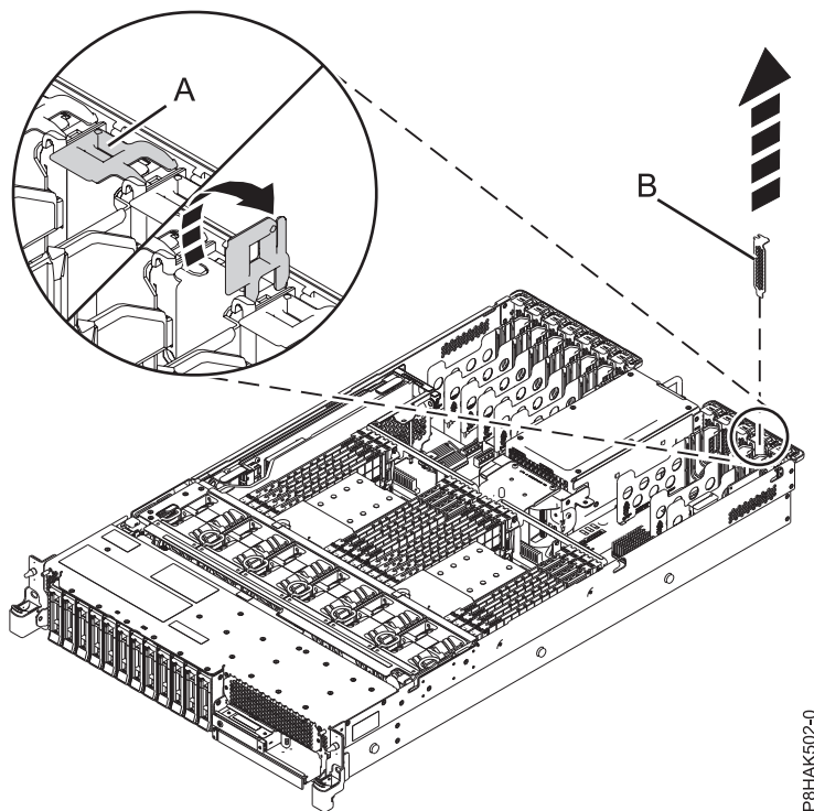
Figura 8. Remover um enchimento da ranhura do adaptador PCIe num sistema 5148-21L, 5148-22L, 8247-21L, 8247-22L, 8284-21A ou 8284-22A
