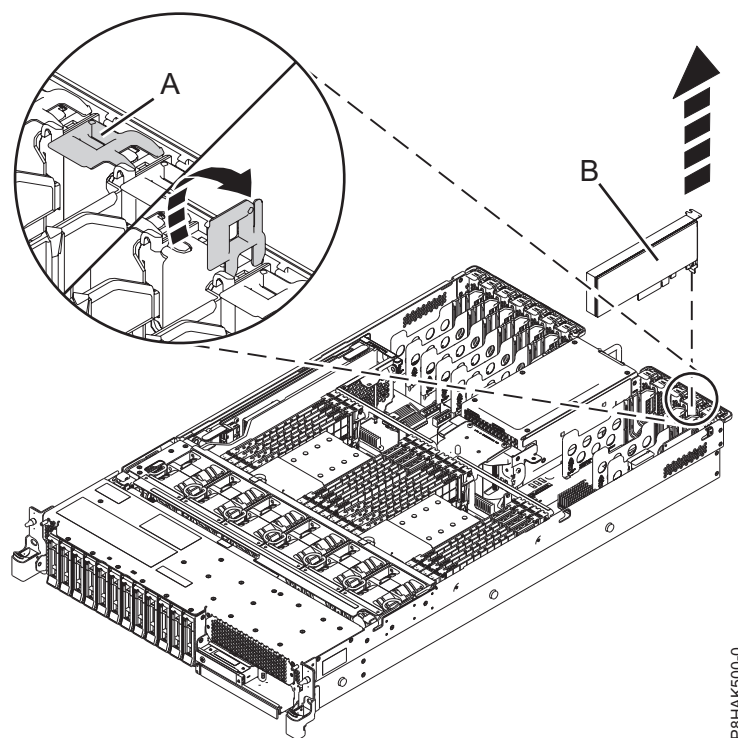
Figura 20. Remover um adaptador PCIe do sistema 5148-21L, 5148-22L, 8247-21L, 8247-22L, 8284-21A ou 8284-22A
