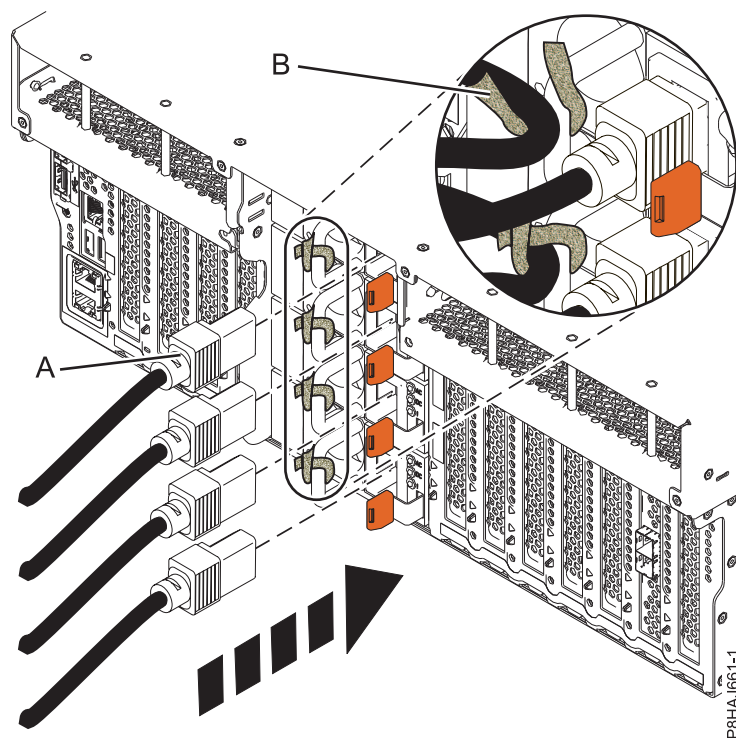
Figura 52. Ligar os cabos de alimentação a um sistema 8247-42L, 8286-41A ou 8286-42A
