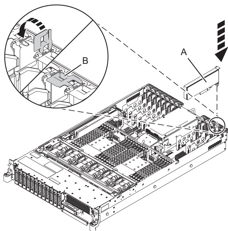
Figura 17. Instalar ou substituir um adaptador PCIe no sistema 5148-21L, 5148-22L, 8247-21L, 8247-22L, 8284-21A ou 8284-22A
