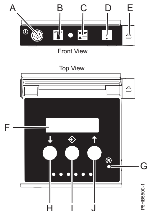
Figura 41. LEDs do painel de controlo
