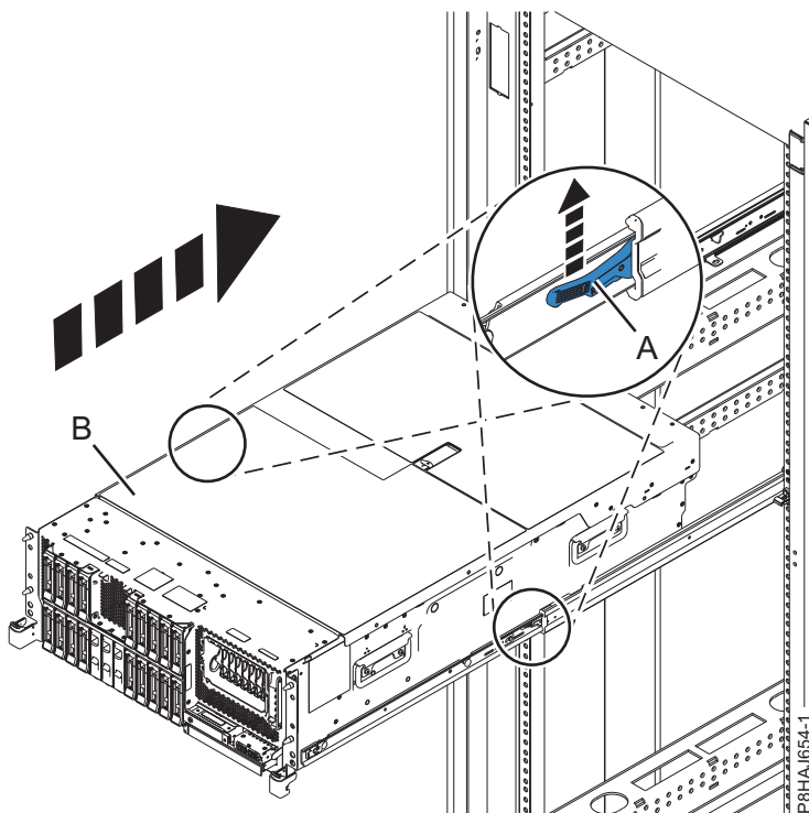
Figura 80. Colocar o sistema na posição de funcionamento
