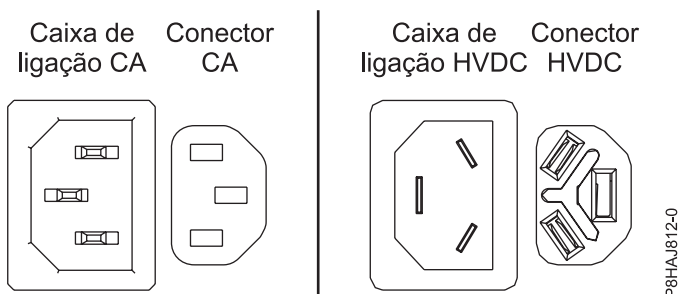
Figura 49. Conectores de AC e de HVDC
