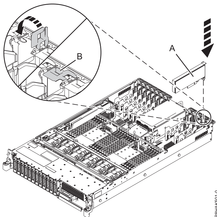
Figura 9. Instalar ou substituir um adaptador PCIe no sistema 5148-21L, 5148-22L, 8247-21L, 8247-22L, 8284-21A ou 8284-22A
