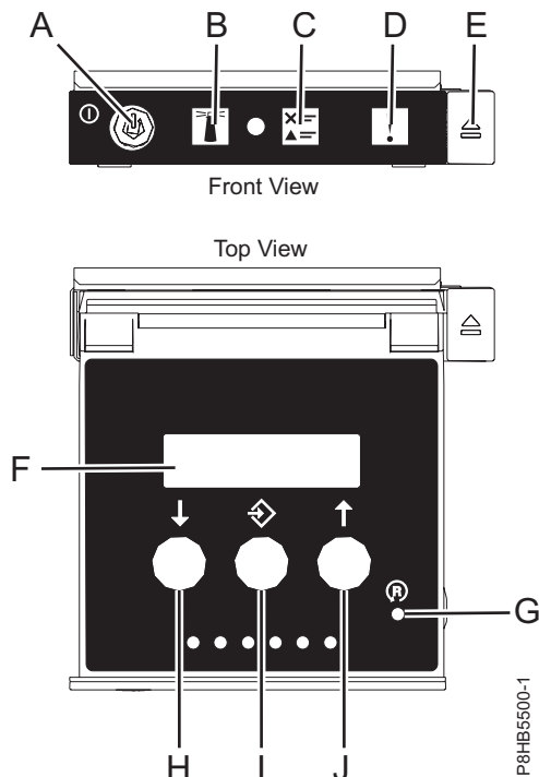
Figura 42. Painel de controlo
