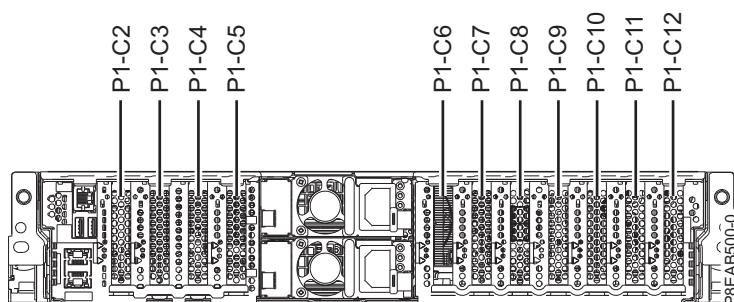
Figura 1. Localizações de ranhuras de adaptadores PCIe num sistema 5148-21L, 5148-22L, 8247-21L, 8247-22L, 8284-21A ou 8284-22A
