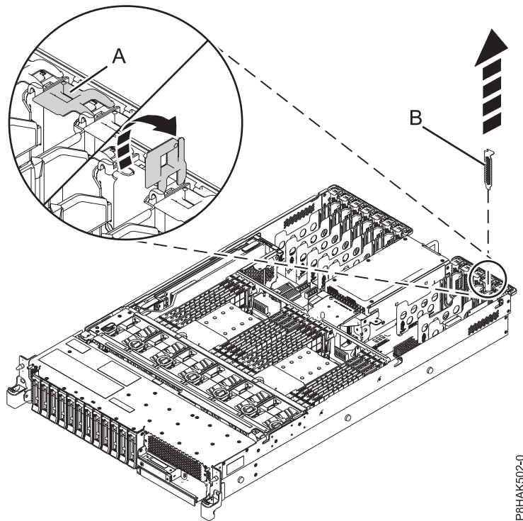
Figura 2. Remover um enchimento da ranhura do adaptador PCIe num sistema 5148-21L, 5148-22L, 8247-21L, 8247-22L, 8284-21A ou 8284-22A
