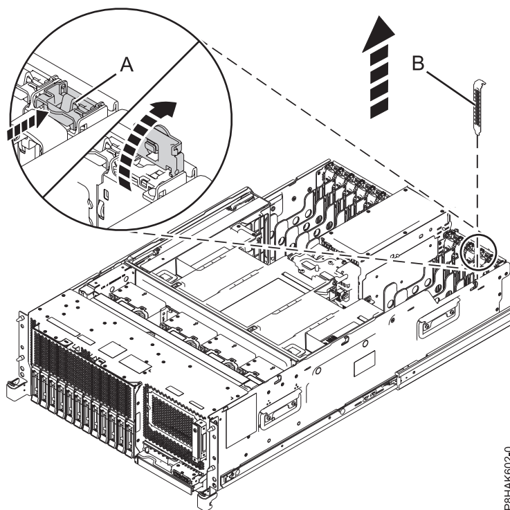
Figura 19. Remover um preenchimento de uma ranhura do adaptador PCIe num sistema montado em bastidor
