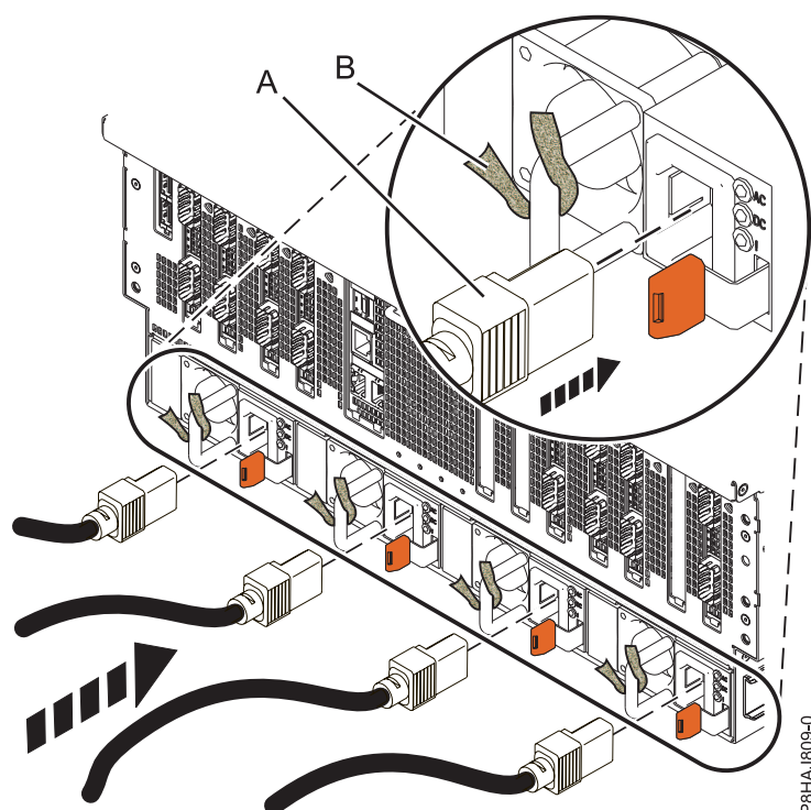
Figura 94. Ligar os cabos de alimentação a um sistema 8408-44E ou 8408-E8E
