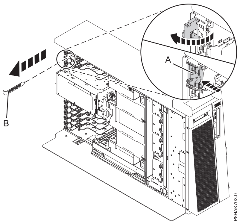
Figura 20. Remover um preenchimento de uma ranhura do adaptador PCIe num sistema 8286-41A autónomo
