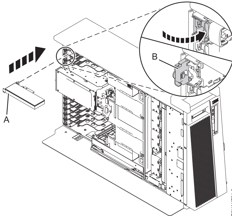
Figura 65. Instalar ou substituir um adaptador PCIe num sistema 8286-41A autónomo
