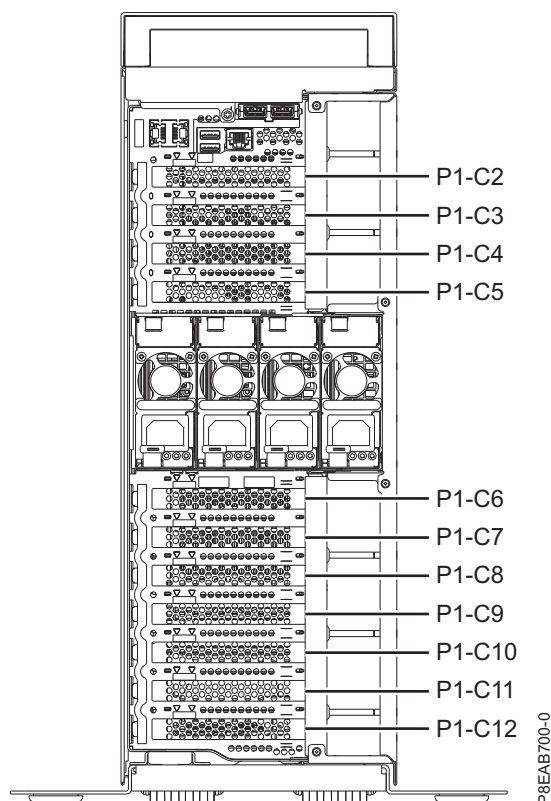
Figura 2. Localizações de ranhuras de adaptadores PCIe num sistema 8286-41A autónomo
