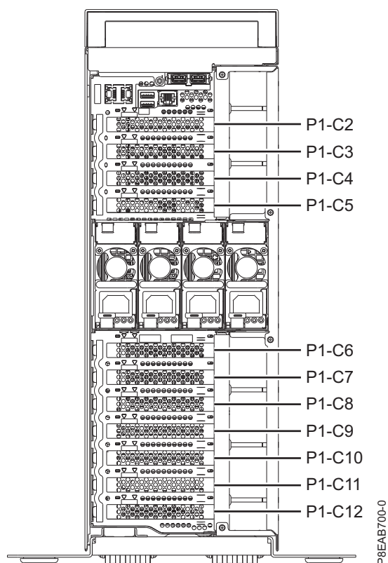
Figura 24. Localizações de ranhuras de adaptadores PCIe num sistema 8286-41A autónomo
