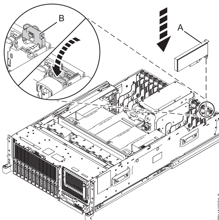
Figura 64. Instalar ou substituir um adaptador PCIe num sistema montado em bastidor
