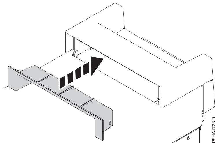
Figura 107. Inserir a peça na tampa da pega num sistema autónomo 8286-41A
