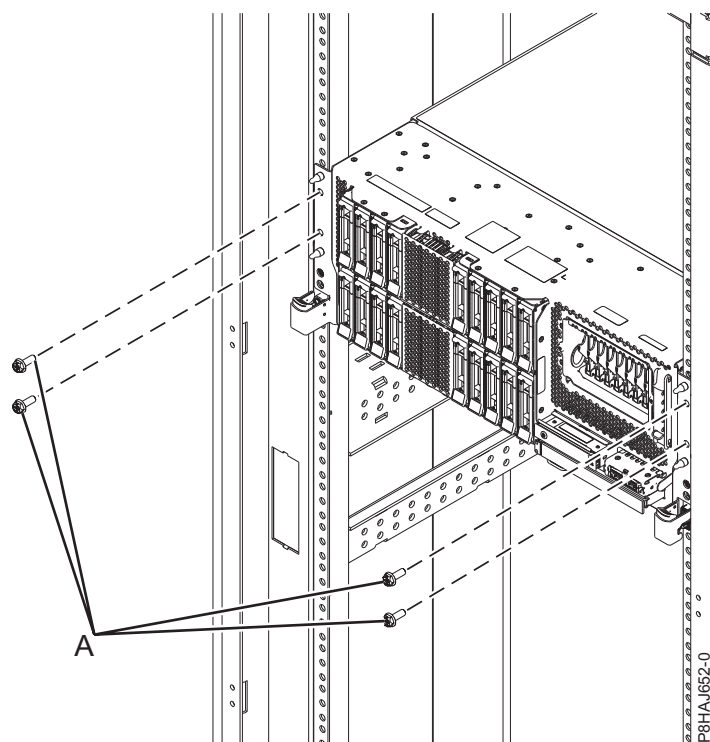
Figura 118. Remover os parafusos frontais
