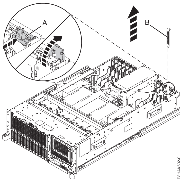
Figura 25. Remover um preenchimento de uma ranhura do adaptador PCIe num sistema montado em bastidor
