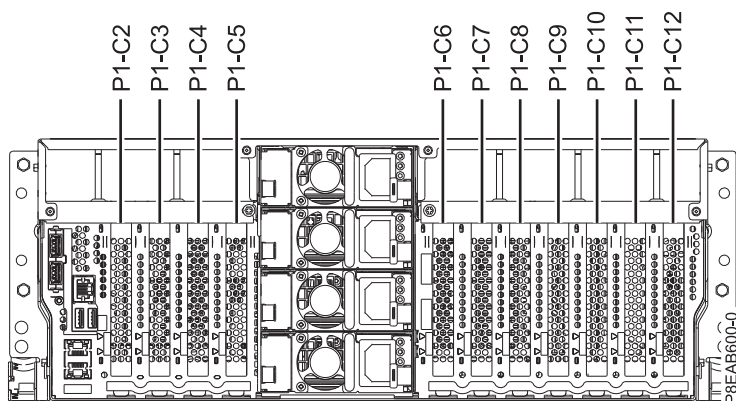
Figura 1. Localizações de ranhuras de adaptadores PCIe num sistema montado em bastidor
