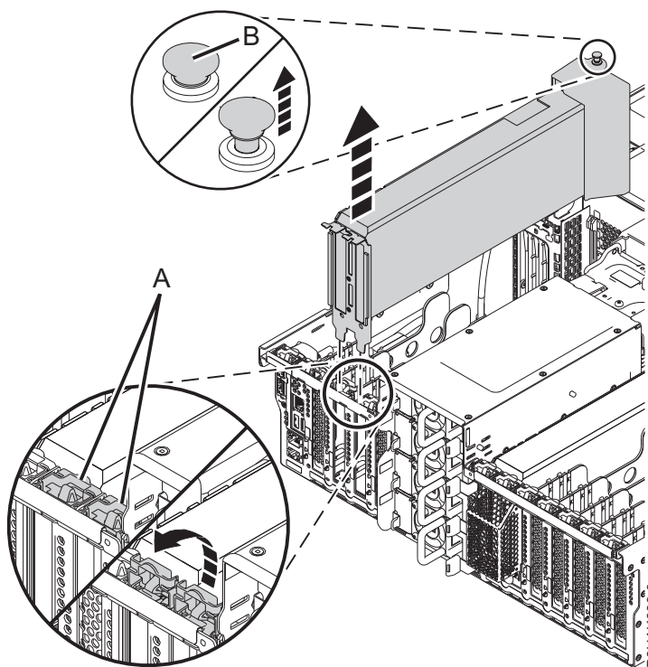
Figura 35. Remover o adaptador GPU adaptador PCIe do sistema 8247-42L
