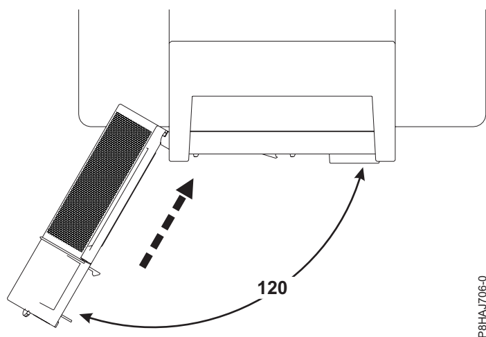
Figura 105. Rodar a tampa frontal
