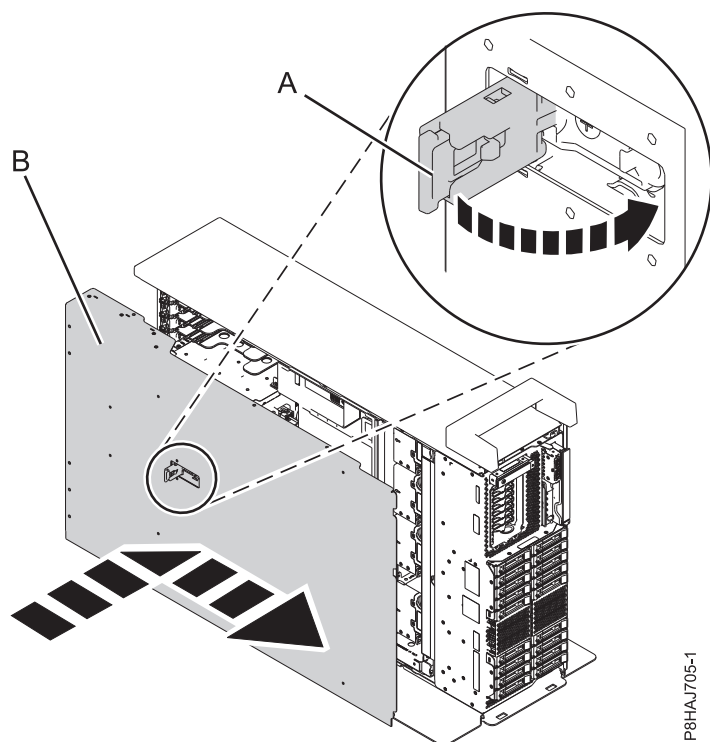
Figura 113. Instalar a tampa de acesso a assistência
