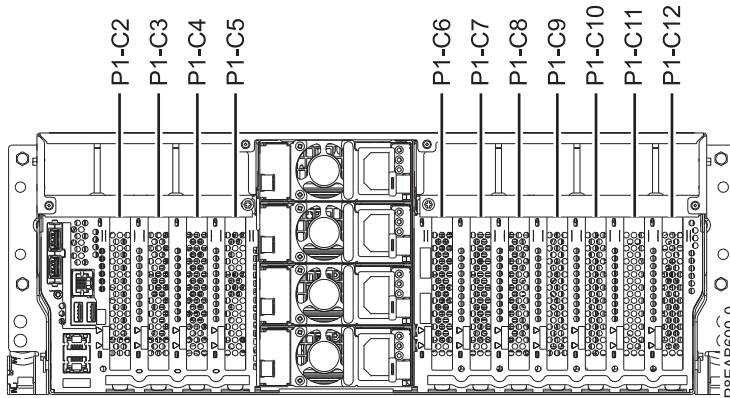
Figura 11. Localizações de ranhuras de adaptadores PCIe num sistema montado em bastidor
