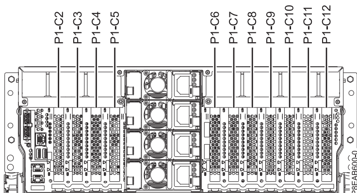
Figura 17. Localizações de ranhuras de adaptadores PCIe num sistema montado em bastidor
