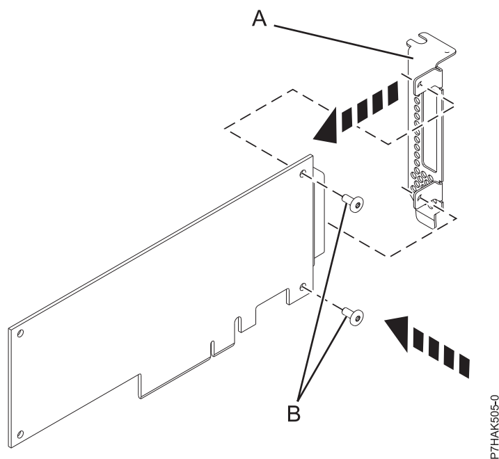
Figura 79. Fixar o contraponto de perfil baixo a um adaptador PCIe
