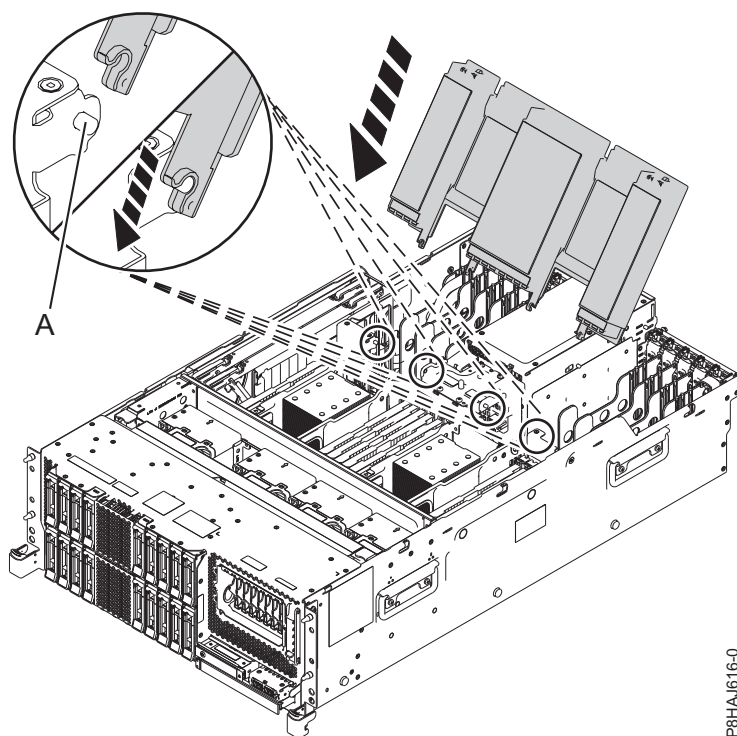
Figura 117. Substituir a conduta de ventilação
