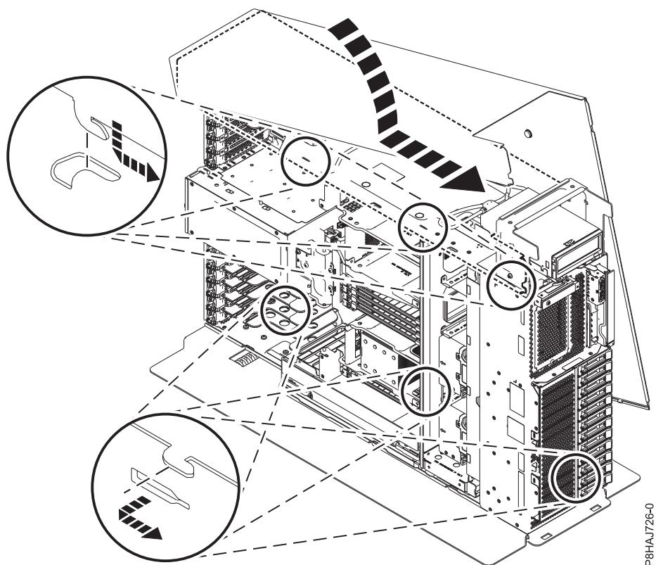
Figura 108. Instalar a tampa lateral do 8286-41A
