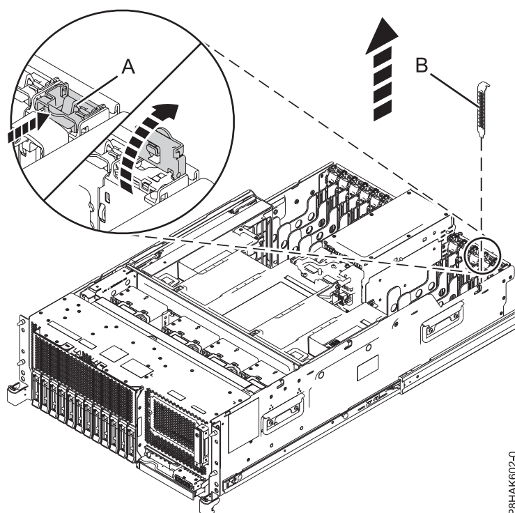
Figura 13. Remover um preenchimento de uma ranhura do adaptador PCIe num sistema montado em bastidor
