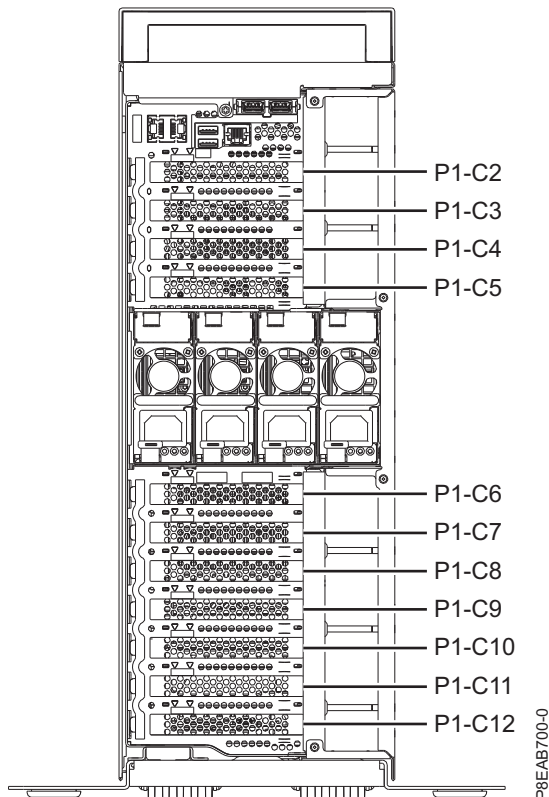
Figura 12. Localizações de ranhuras de adaptadores PCIe num sistema 8286-41A autónomo
