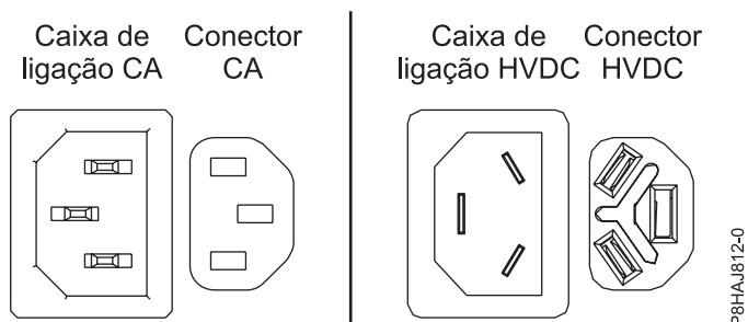
Figura 89. Conectores de AC e de HVDC
