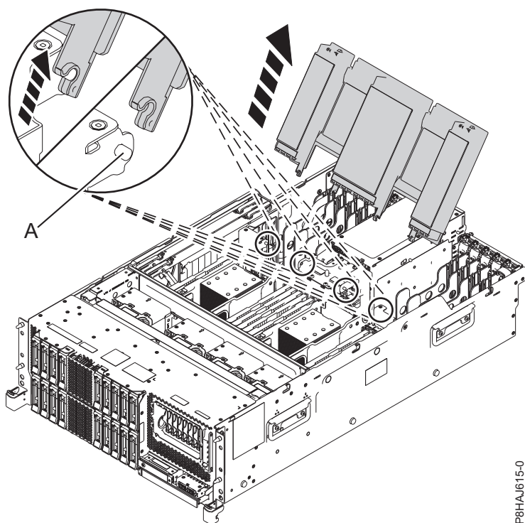
Figura 116. Remover a conduta de ventilação
