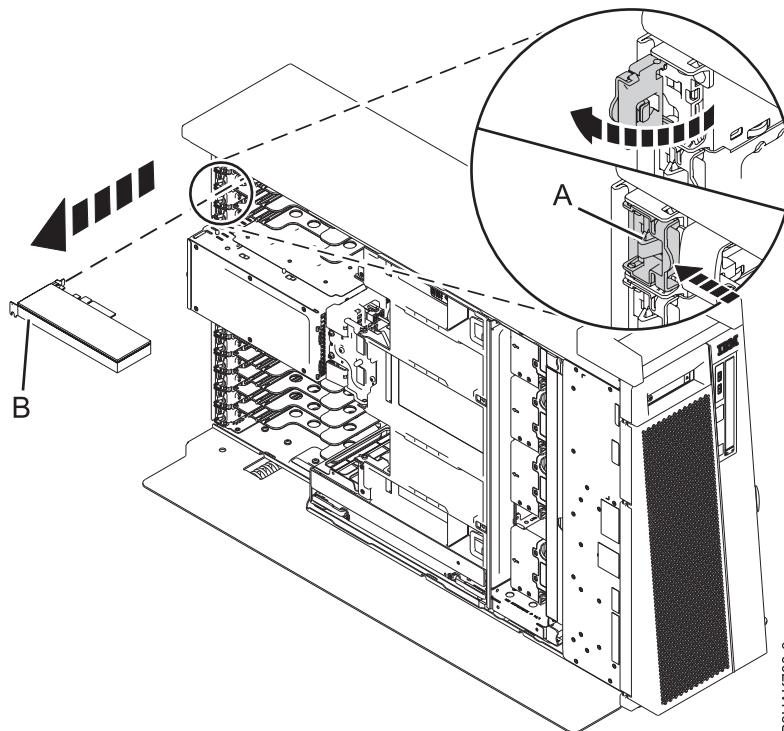
Figura 37. Remover um adaptador PCIe de um sistema 8286-41A autónomo
