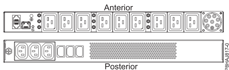
Figura 91. PDU para o sistema 8408-44E
