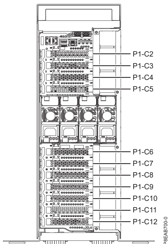
Figura 18. Localizações de ranhuras de adaptadores PCIe num sistema 8286-41A autónomo
