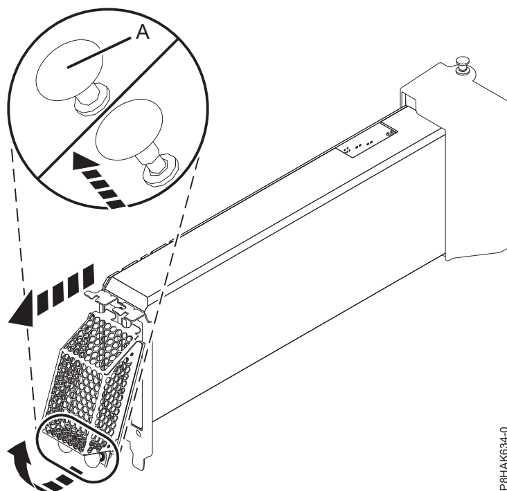
Figura 5. Remover a blindagem protectora do adaptador GPU
