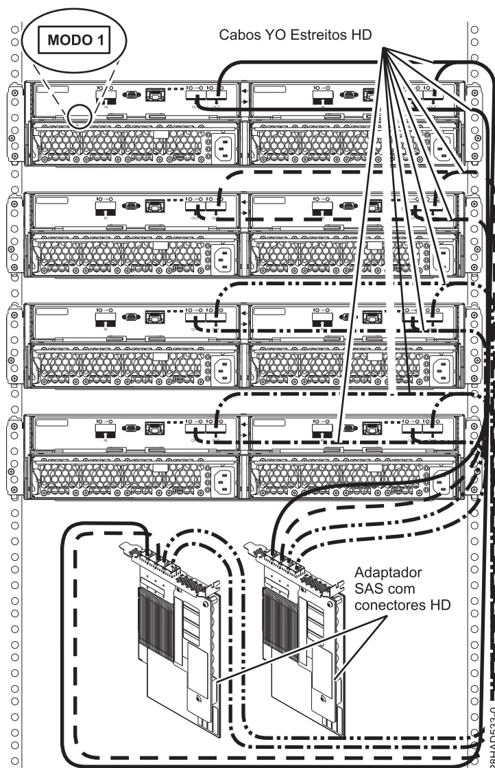
Figura 88. Ligação de modo 1 de quatro suportes 5887 para dois adaptadores SAS PCIe3 com conectores estreitos HD.
