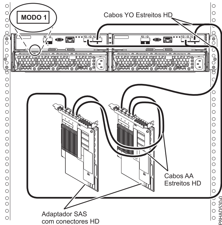
Figura 85. Ligação de modo 1 de um suporte 5887 para dois adaptadores SAS PCIe3 com conectores estreitos HD.
