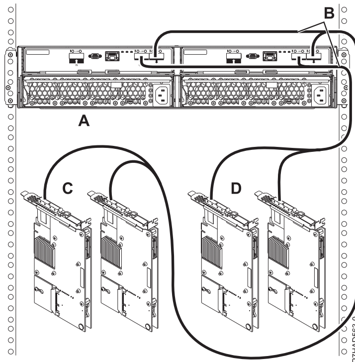
Figura 80. Dois pares de adaptadores FC 5805 ou FC 5903 para um suporte de 5887 através de uma ligação de modo 2
