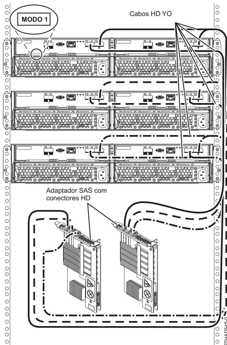
Figura 83. Ligação de modo 1 de três suportes de 5887 para dois adaptadores SAS PCIe2 com conectores HD
