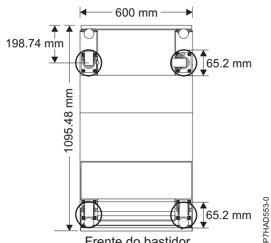
Frente do bastidor Figura 26. Localizações dos rodízios
