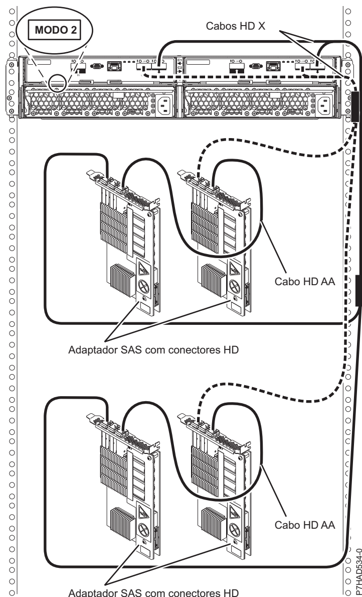
Figura 84. Ligação de modo 2 de um suporte de 5887 ao utilizar conectores HD para dois pares de adaptadores SAS PCIe2
