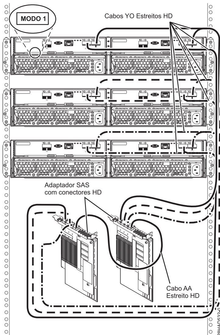
Figura 87. Ligação de modo 1 de três suportes 5887 para dois adaptadores SAS PCIe3 com conectores estreitos HD.
