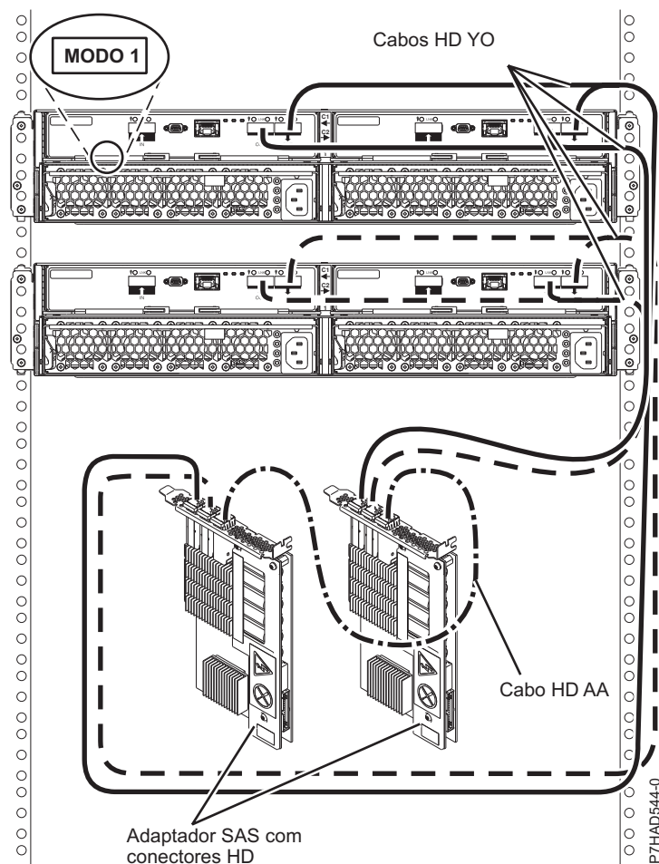
Figura 82. Ligação de modo 1 de dois suportes de 5887 ao utilizar conectores HD para dois adaptadores SAS PCIe2
