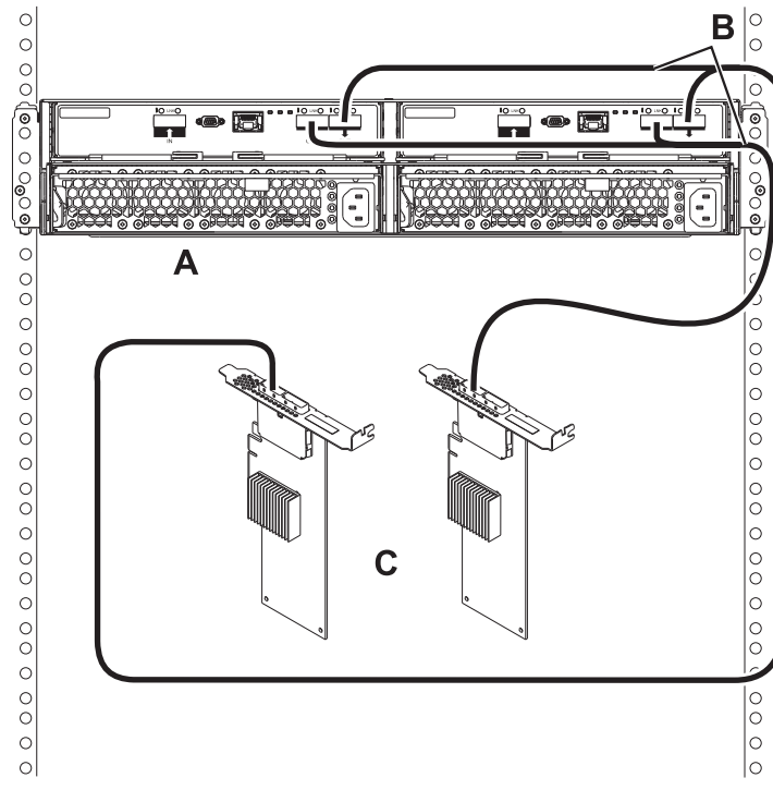
Figura 75. Ligação de modo 1 de um suporte de 5887 utilizando cabos YO para adaptadores SAS duplos
