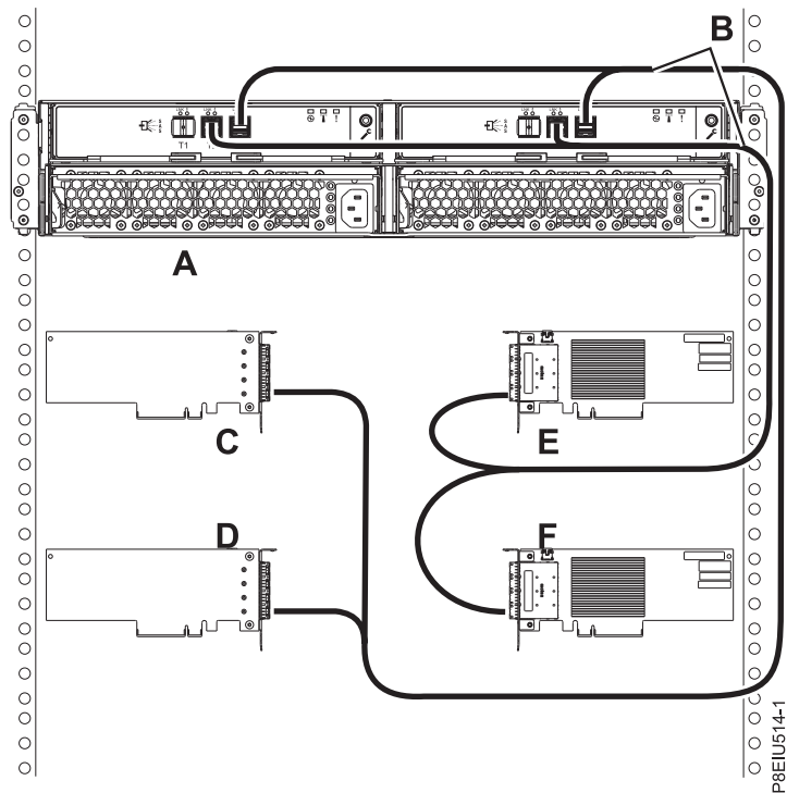
Figura 97. Ligação de modo 4 de um Suporte de armazenamento ESLL ou ESLS através da utilização de cabos X12 a quatro adaptadores SAS independentes
