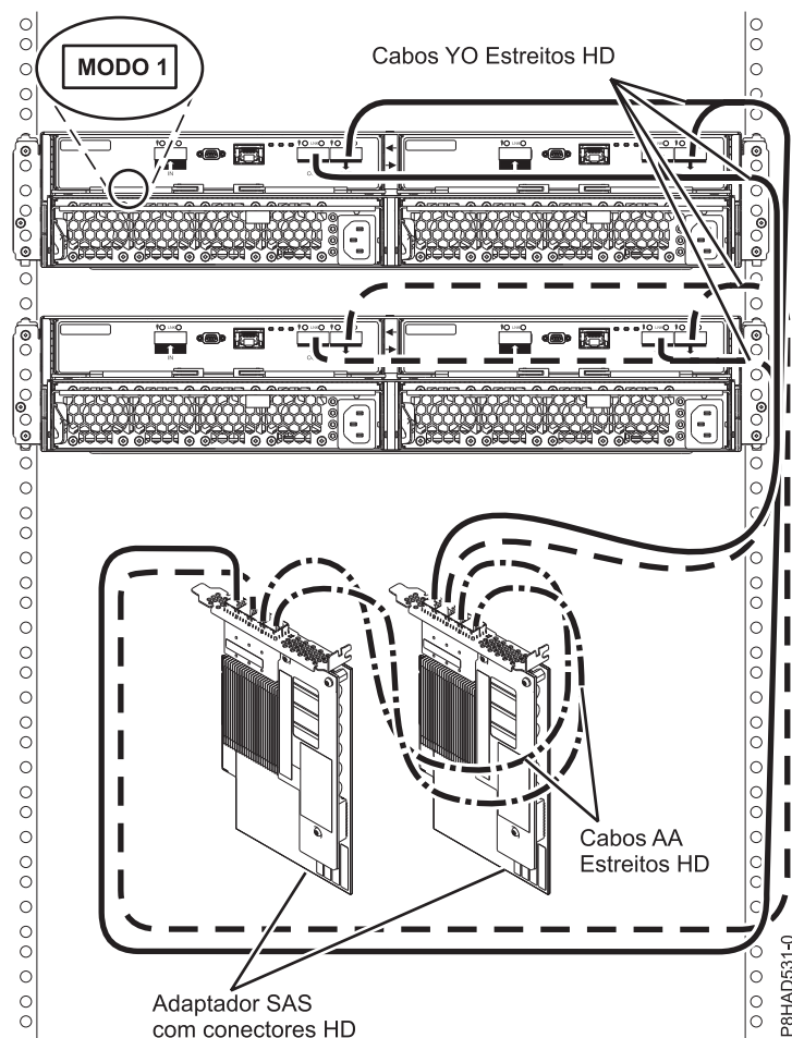
Figura 86. Ligação de modo 1 de dois suportes 5887 para dois adaptadores SAS PCIe3 com conectores estreitos HD.
