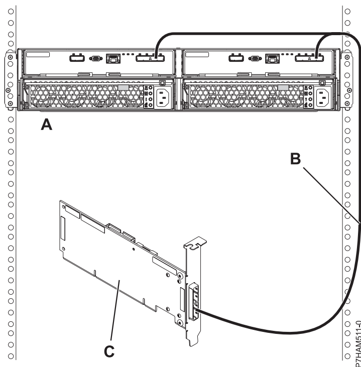
Figura 74. Ligação de modo 1 de um suporte de 5887 utilizando um cabo YO a um adaptador SAS único
