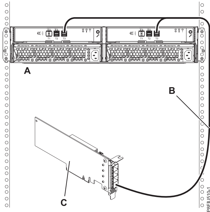
Figura 91. Ligação de modo 1 de um Suporte de armazenamento ESLL ou ESLS através da utilização de um cabo YO12 para um único adaptador SAS
