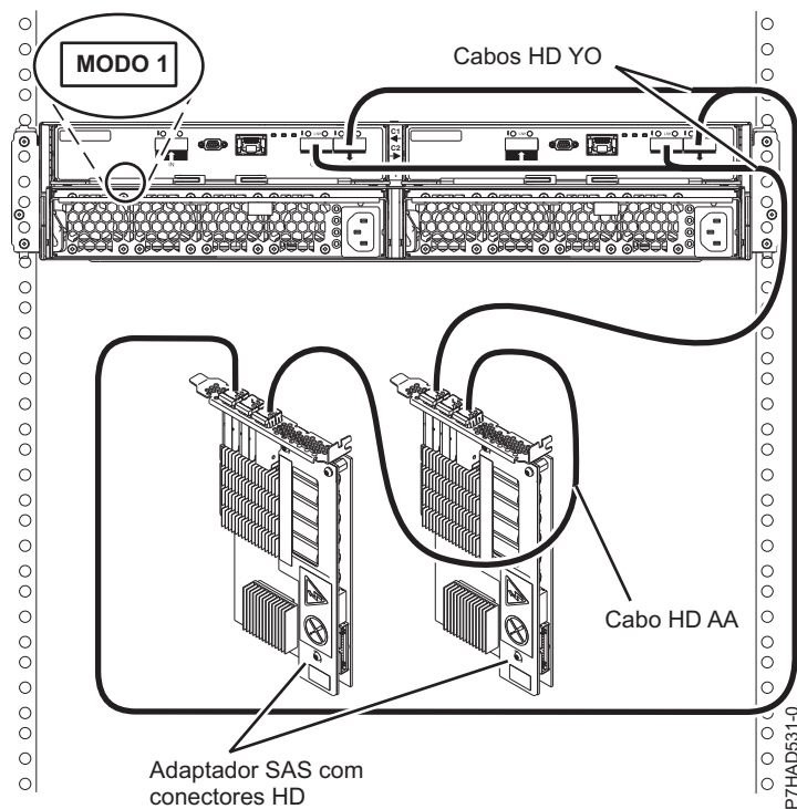
Figura 81. Ligação de modo 1 de um suporte de 5887 para dois adaptadores SAS PCIe2 com conectores HD
