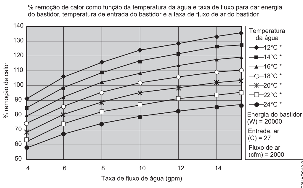
Figura 40. Desempenho típico do permutador de calor, carga de calor de 20 kW
