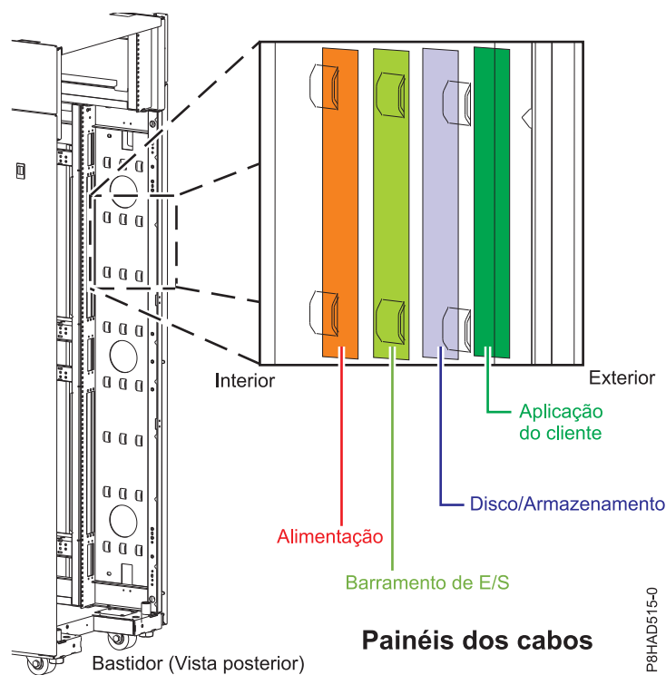
Figura 50. Lanças da ponte da gestão de cabos
