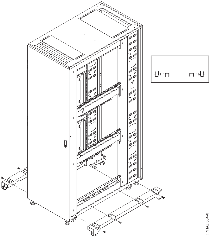
Figura 30. Localizações dos niveladores
