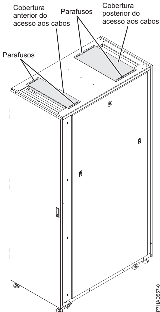
Figura 29. Tampas de acesso de cabos
