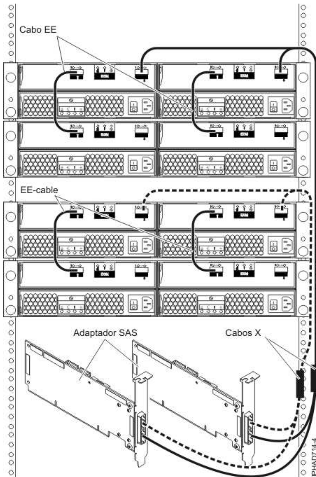
Figura 67. Dois adaptadores RAID SAS a quatro gavetas de expansão de disco numa configuração RAID de HA de múltiplos iniciadores
