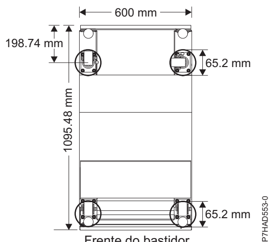
Figura 26. Localizações dos rodízios
