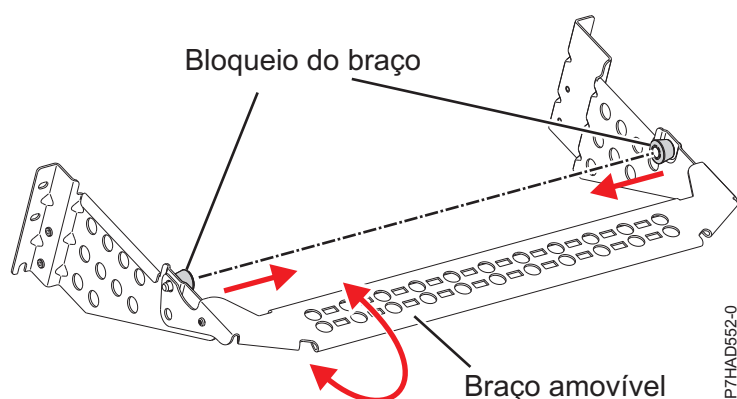
Figura 52. Suporte de gestão de cabos
