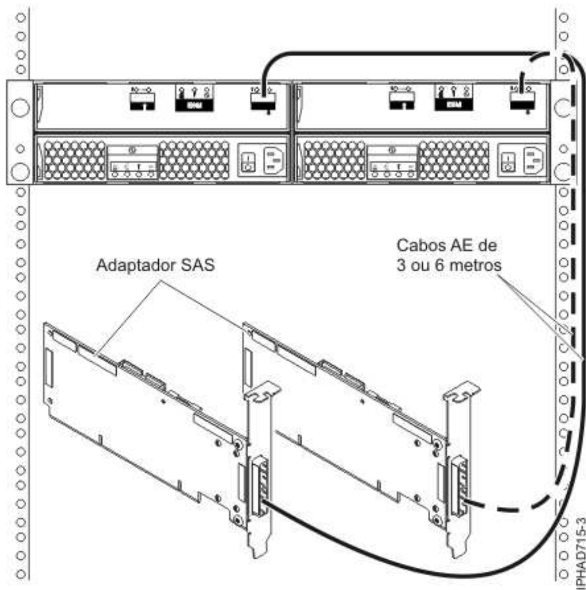
Figura 73. Dois adaptadores RAID SAS a uma gaveta de expansão de disco numa configuração JBOD de HA de múltiplos iniciadores
