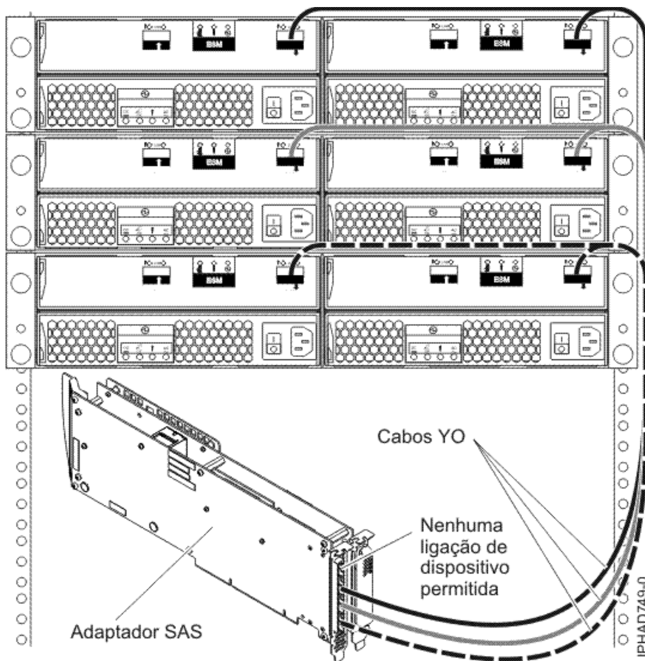
Figura 59. Adaptador SAS de três portas para gavetas de expansão de disco
