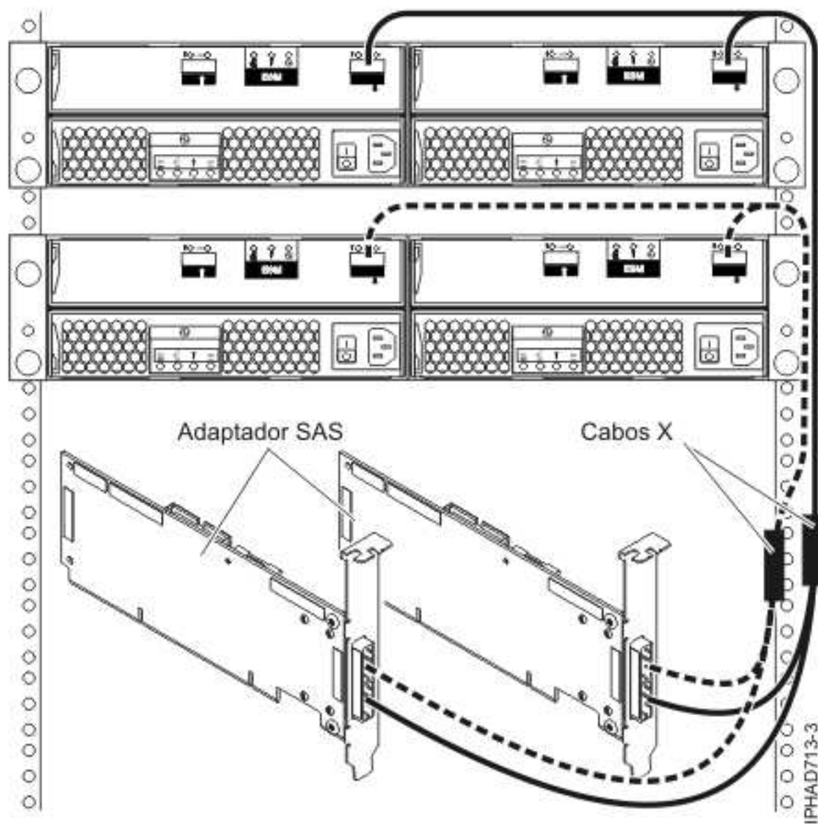
Figura 66. Dois adaptadores RAID SAS a duas gavetas de expansão de disco numa configuração RAID de HA de múltiplos iniciadores
