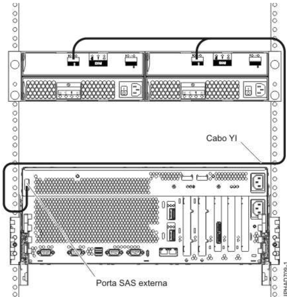
Figura 62. Porta de adaptador SAS externa ao sistema para uma gaveta de expansão de disco
