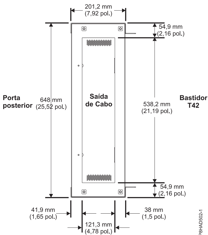
Figura 24. Extensor de bastidores posteriores FC ERG0 (vista de cima para baixo)
