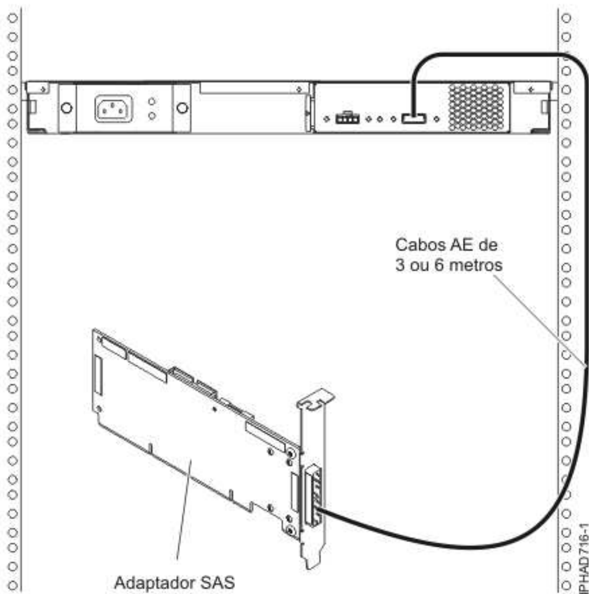
Figura 60. Adaptador SAS para gaveta de expansão de suportes
