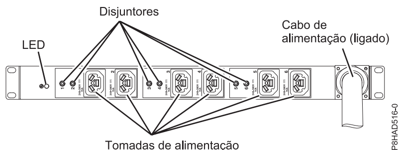
Figura 49. PDU de HVDC
