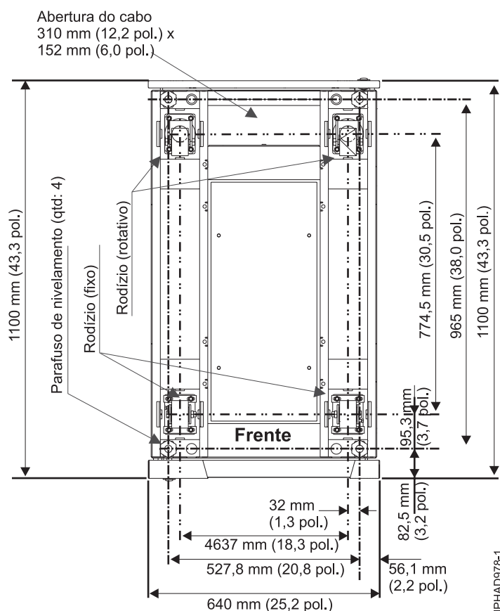
Figura 23. Localizações dos rodízios e parafusos de nivelamento
