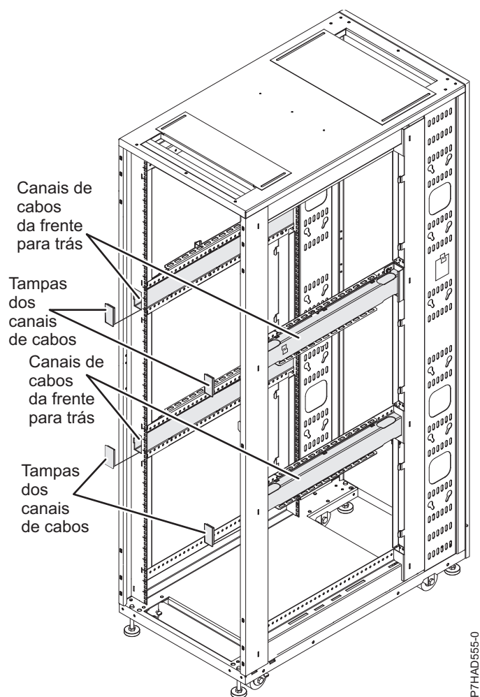
Figura 27. Cablagem no bastidor
