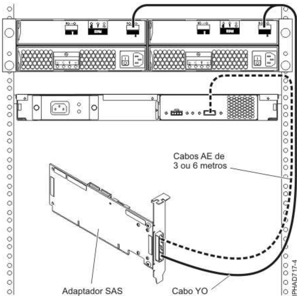
Figura 61. Adaptador SAS a uma gaveta de expansão de disco e a uma gaveta de expansão de suportes
