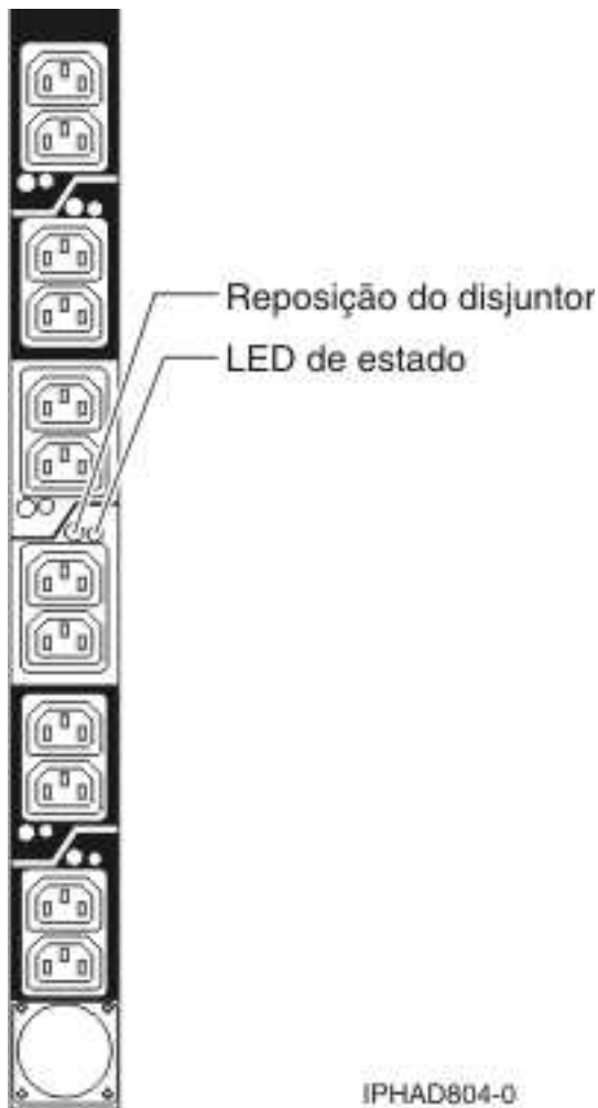
Figura 47. Gráfico de tomadas de PDU
