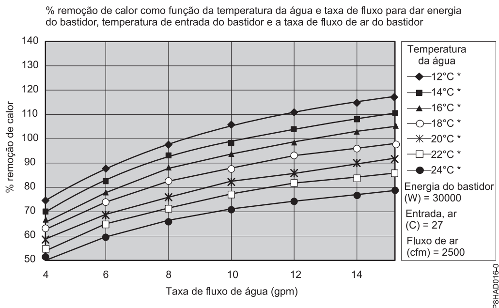
Figura 33. Desempenho típico do permutador de calor, carga de calor de 30 kW
