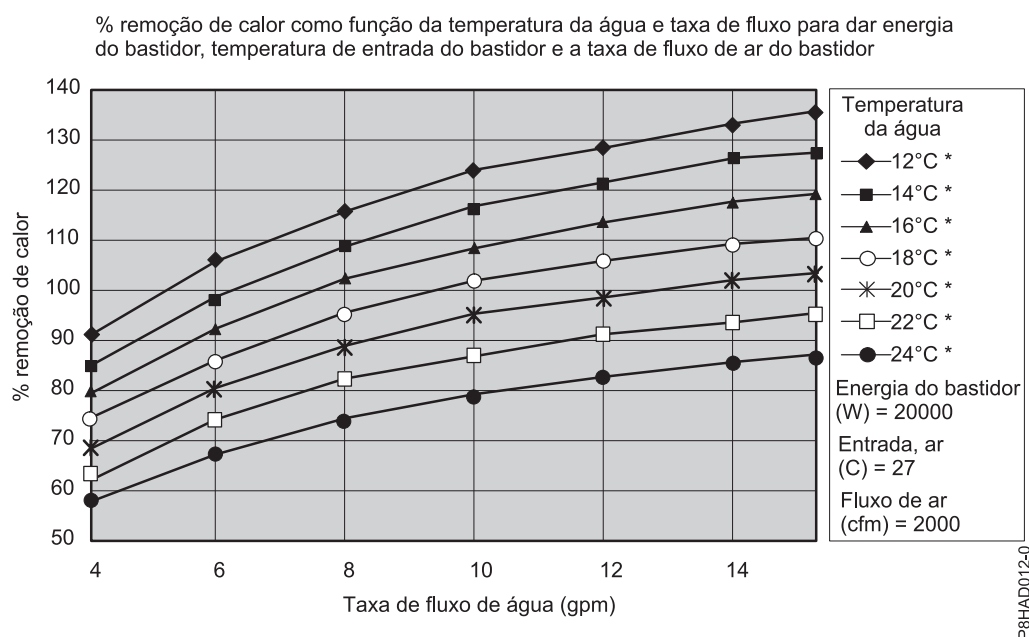
Figura 32. Desempenho típico do permutador de calor, carga de calor de 20 kW
