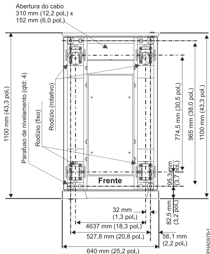
Figura 4. Localizações dos rodízios e parafusos de nivelamento
