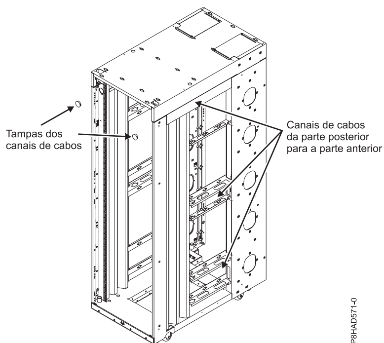
Figura 36. Cablagem no bastidor
