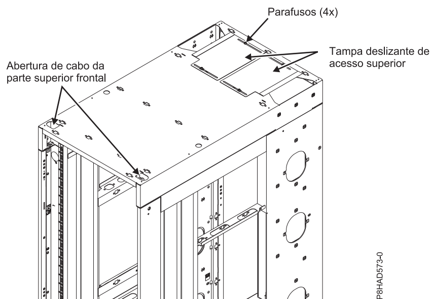
Figura 38. Cablagem na parte superior
