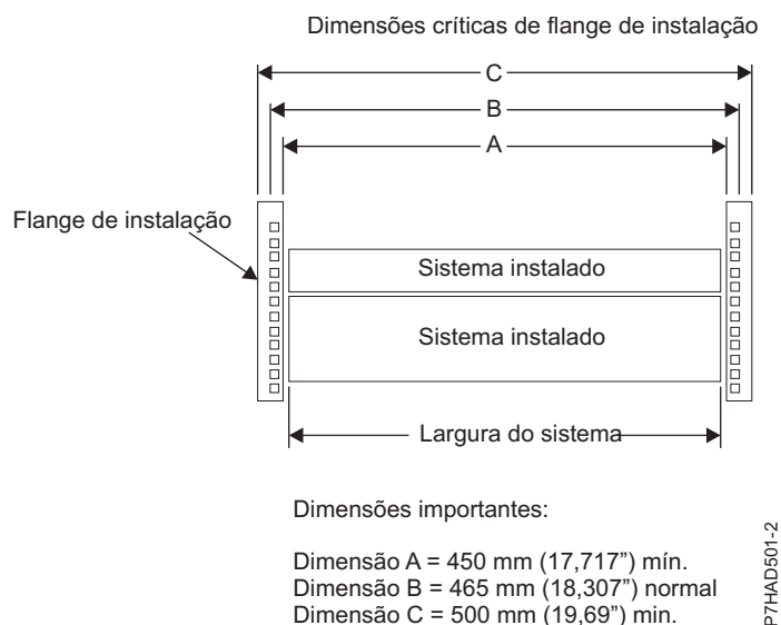
Figura 43. Dimensões críticas dos bordos de instalação
