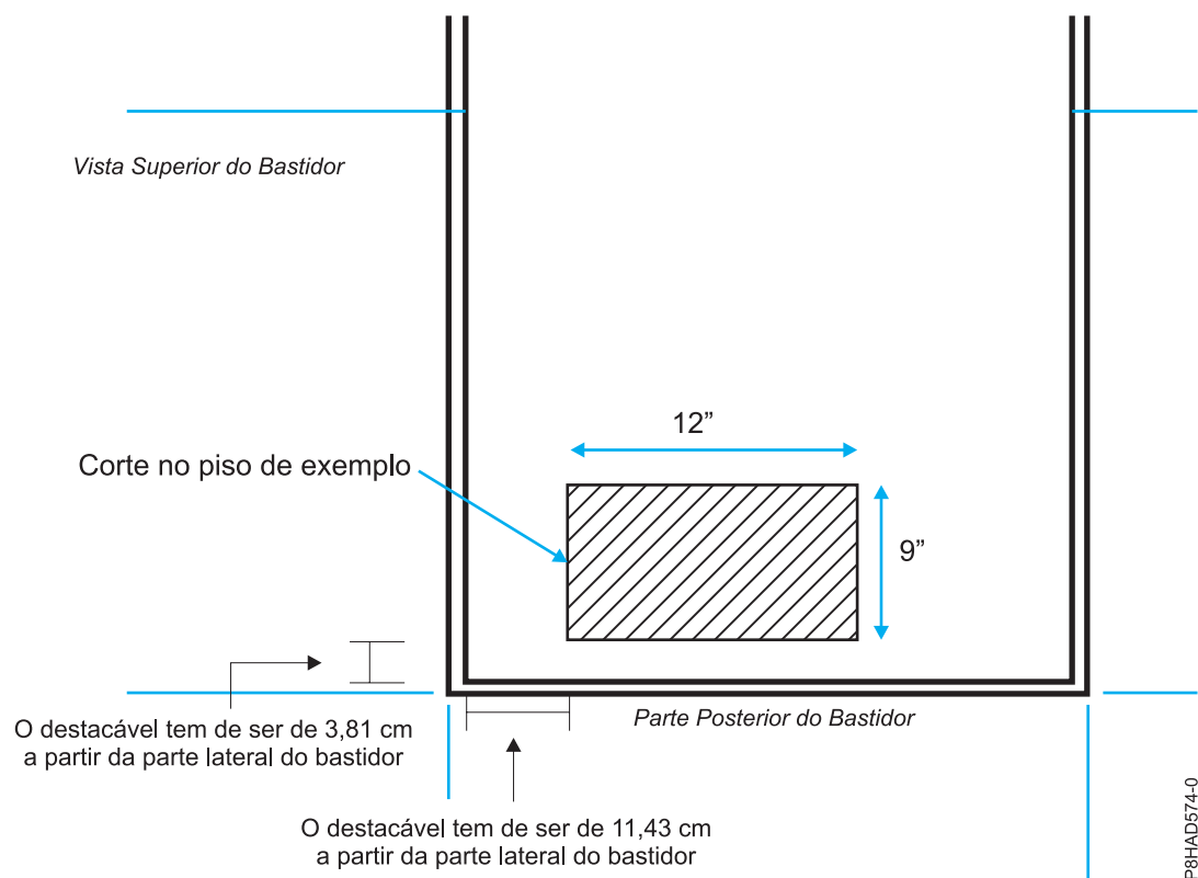
Figura 35. Corte no piso
