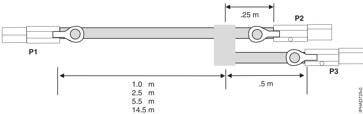
Figura 54. Comprimentos de cabo de montagem de cabo YO externo SAS
