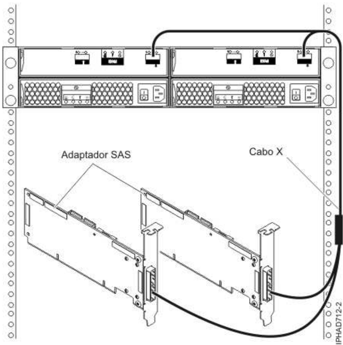
Figura 65. Dois adaptadores RAID SAS a uma gaveta de expansão de disco numa configuração RAID de HA de múltiplos iniciadores
