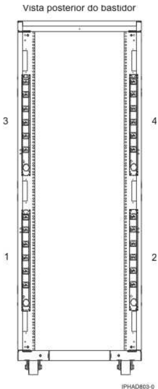
Figura 46. Localizações verticais das unidades de distribuição Power
