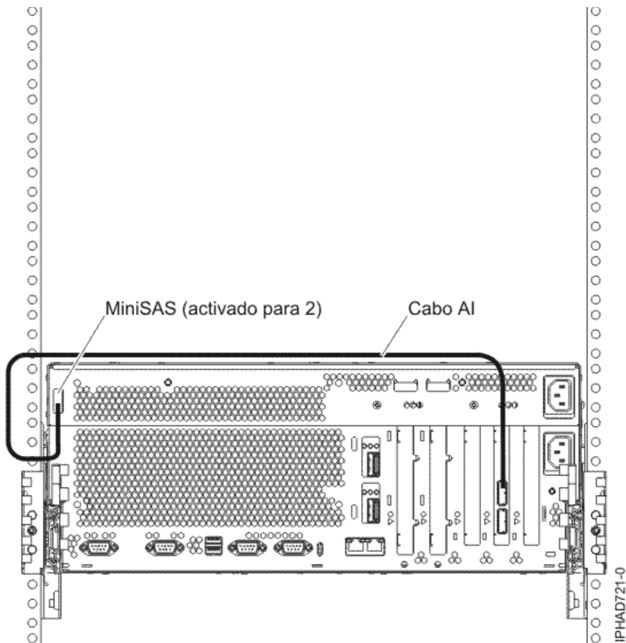
Figura 63. Adaptador SAS a ranhuras de disco SAS internas através de porta SAS externa do sistema
