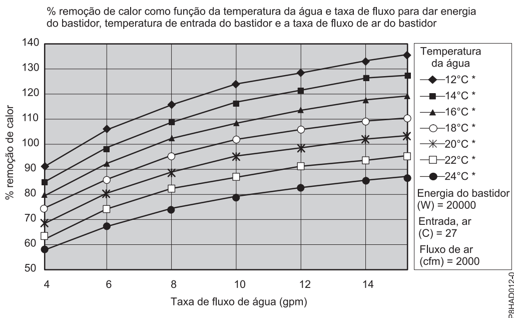
Figura 40. Desempenho típico do permutador de calor, carga de calor de 20 kW
