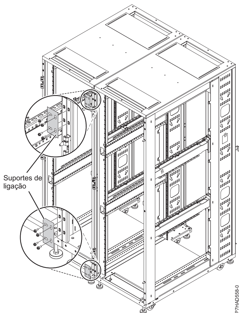
Figura 31. Suportes de ligação
