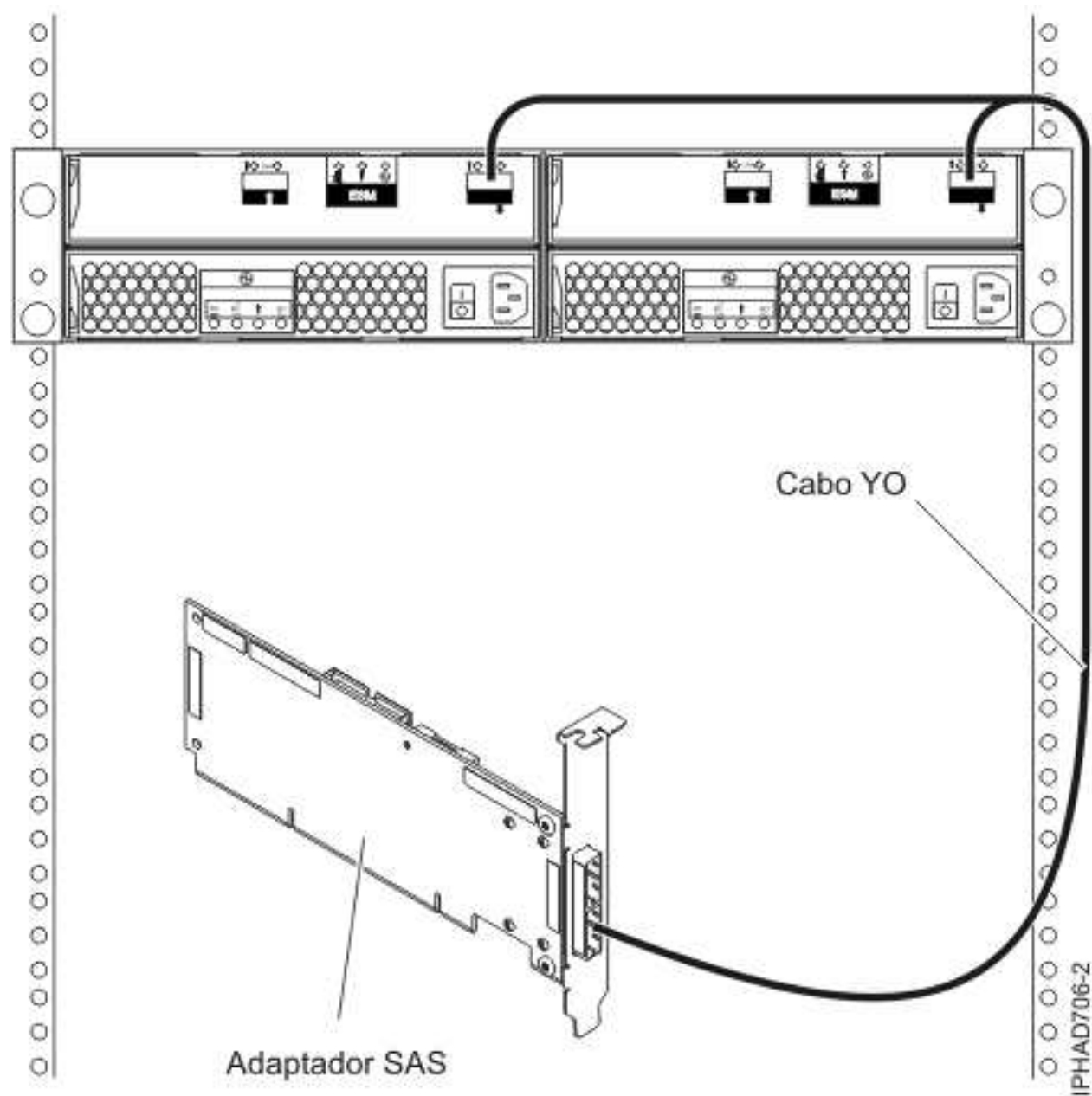
Figura 56. Adaptador SAS a uma gaveta de expansão de disco
