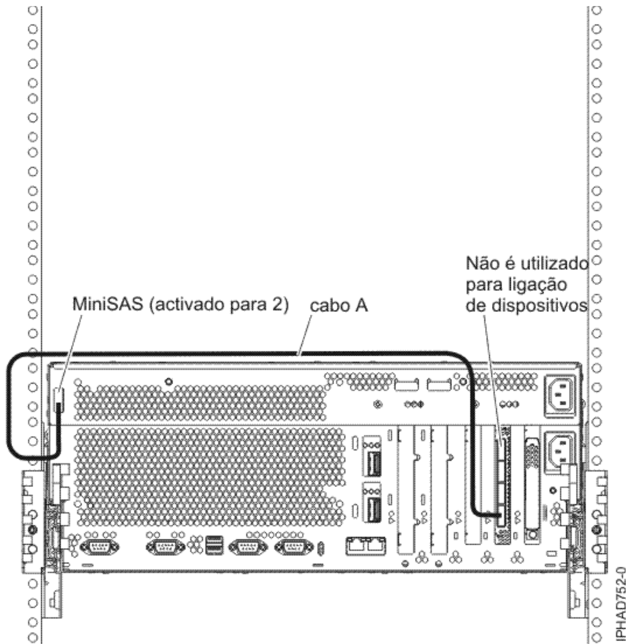
Figura 64. Adaptador FC5904 ou FC5908 ligado a gavetas de expansão de disco
