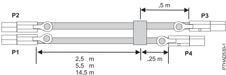
Figura 53. Comprimentos de cabos de montagem de cabo X externo SAS
