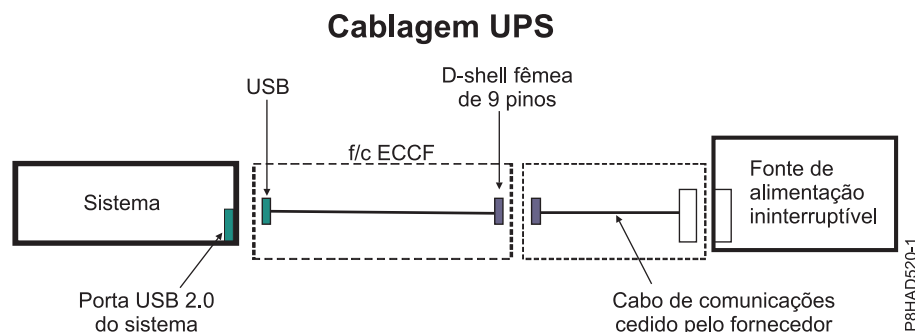
Figura 45. Encadeamento de UPS para os sistemas 5148-21L, 5148-22L, 8247-21L, 8247-21L, 8247-22L, 8247-42L, 8284-22A, 8286-41A e 8286-42A
