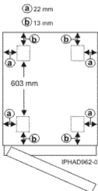
Figura 17. Localizações dos rodízios nos modelos 0554 e 7014-S11
