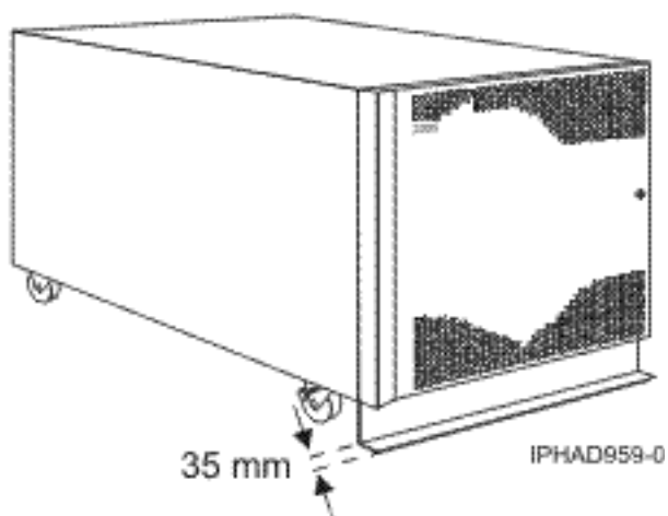
Figura 15. Modelo 0554 e 7014-S11 com barra estabilizadora
