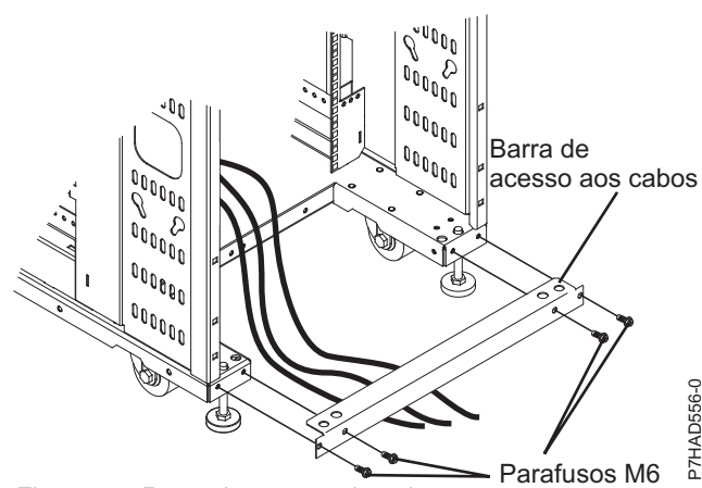
Figura 28. Barra de acesso de cabos
