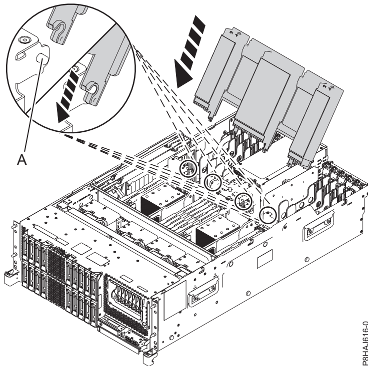
Figura 27. Substituir a conduta de ventilação
