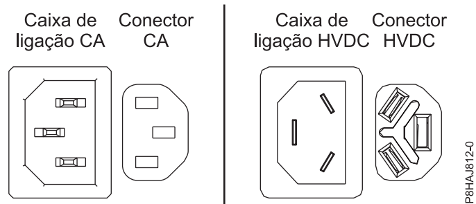
Figura 31. Conectores de CA e de HVDC
