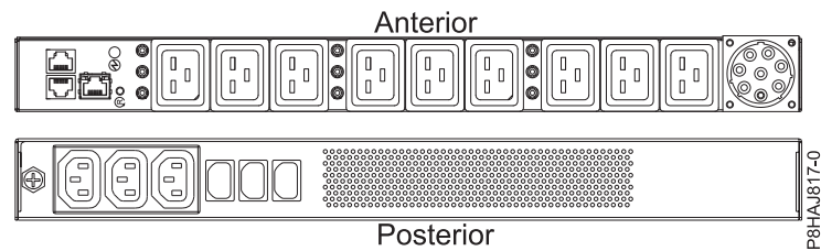
Figura 33. PDU para o sistema 8408-44E
