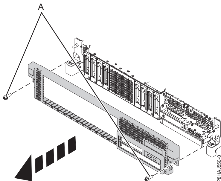
Figura 7. Remover a tampa anterior
