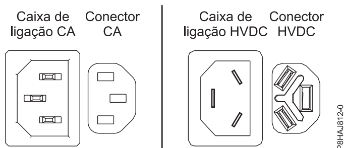
Figura 39. Conectores de CA e de HVDC
