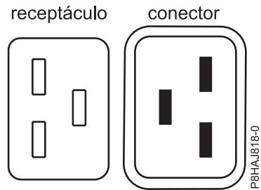
Figura 34. Conectores para o sistema 8408-44E
