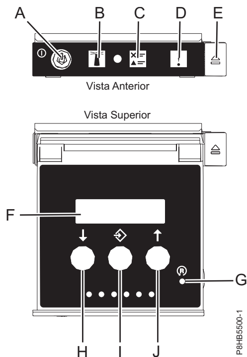
Figura 6. Painel de controlo
