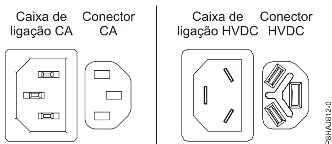
Figura 17. Conectores de AC e HVDC
