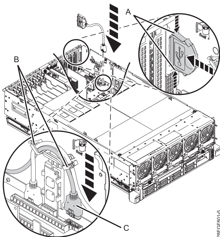
Figura 3. Substituir o cabo USB posterior
