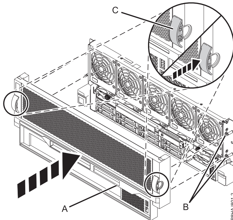
Figura 8. Instalar a tampa anterior
