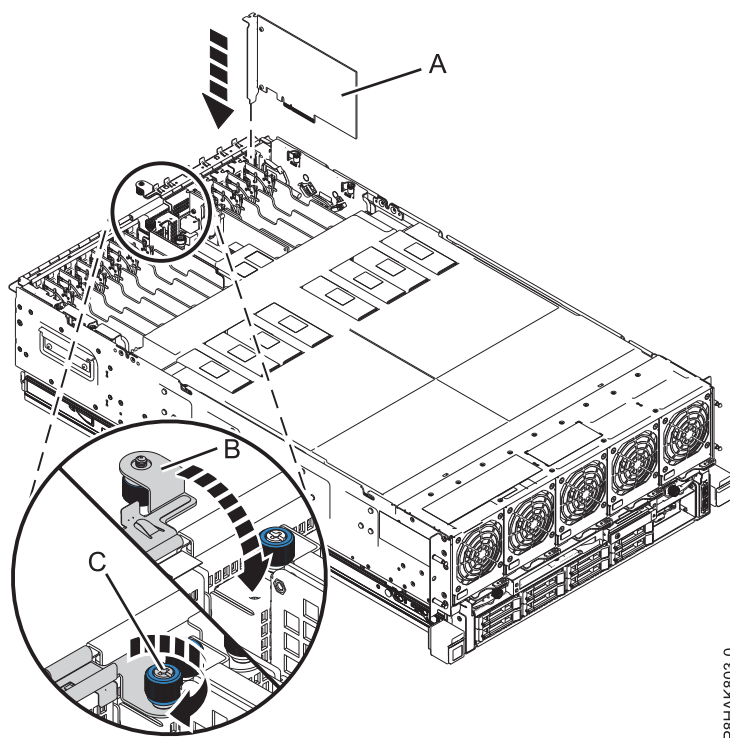
Figura 4. Substituir o adaptador PCIe na ranhura P1-C1
