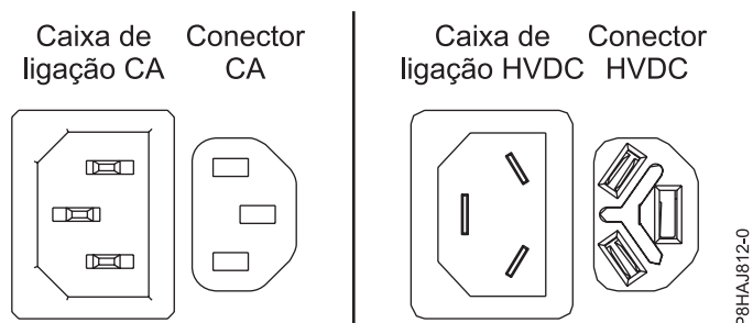
Figura 23. Conectores de AC e HVDC
