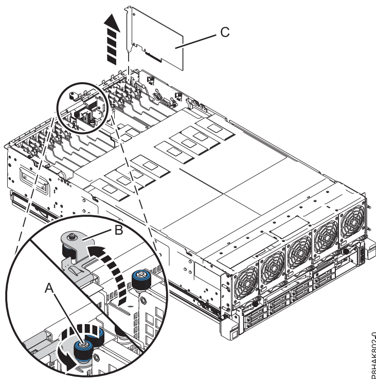
Figura 1. Remover um adaptador PCIe
