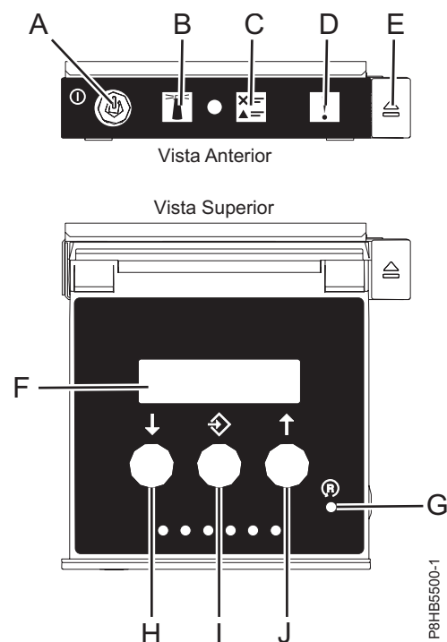
Figura 5. LEDs do painel de controlo
