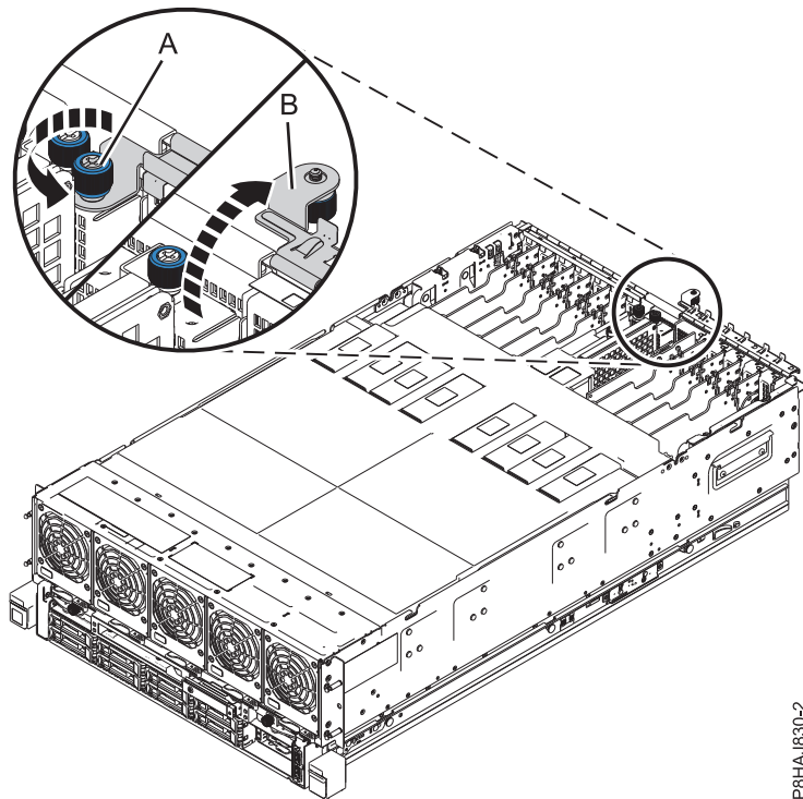
Figura 13. Abrir o trinco de E/S
