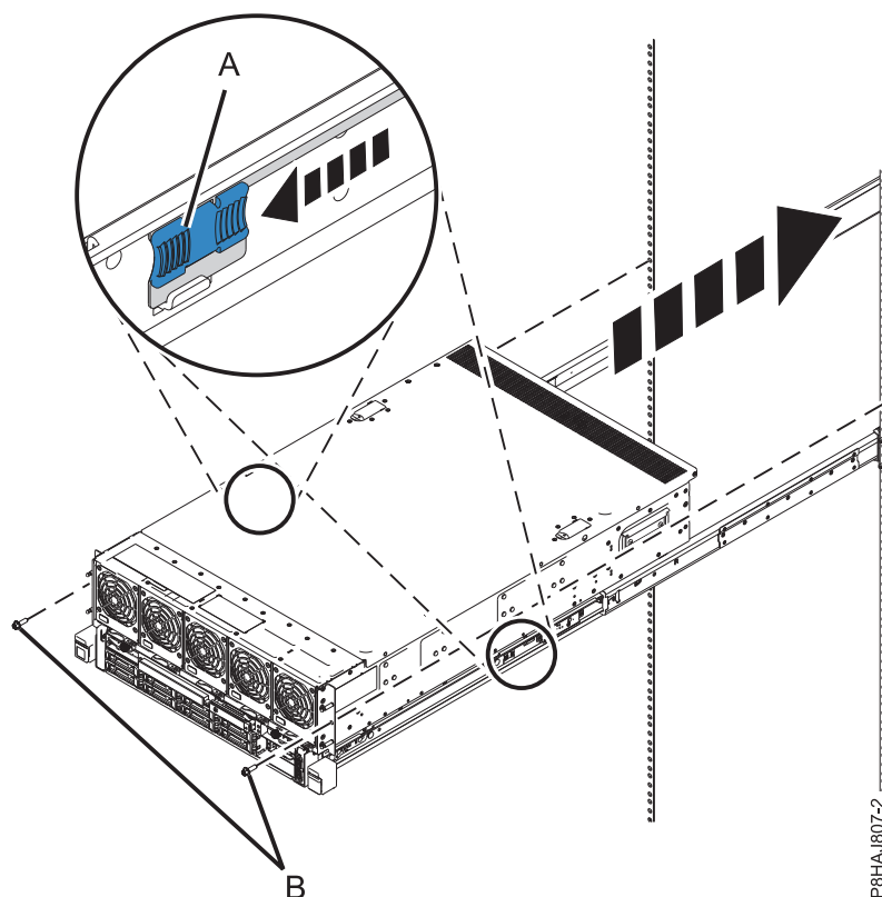
Figura 16. Colocar o sistema na posição de funcionamento
