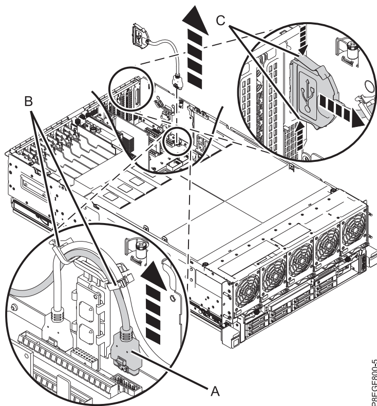
Figura 2. Remover o cabo USB posterior
