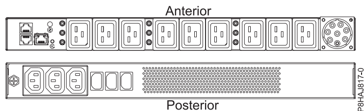
Figura 19. PDU para o sistema 8408-44E
