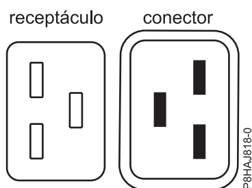
Figura 18. Conectores para o sistema 8408-44E
