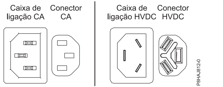
Figura 31. Conectores de AC e HVDC
