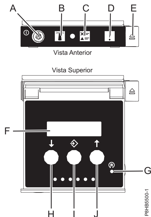
Figura 3. LEDs do painel de controlo
