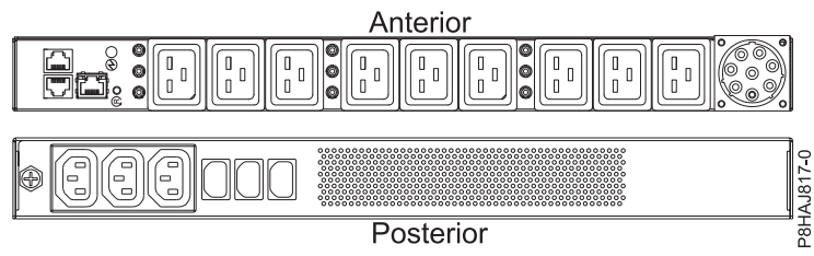
Figura 33. PDU para o sistema 8408-44E
