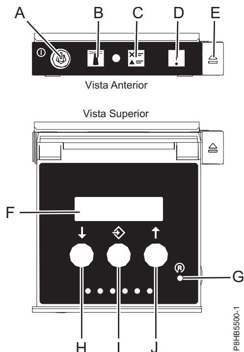
Figura 4. Painel de controlo
