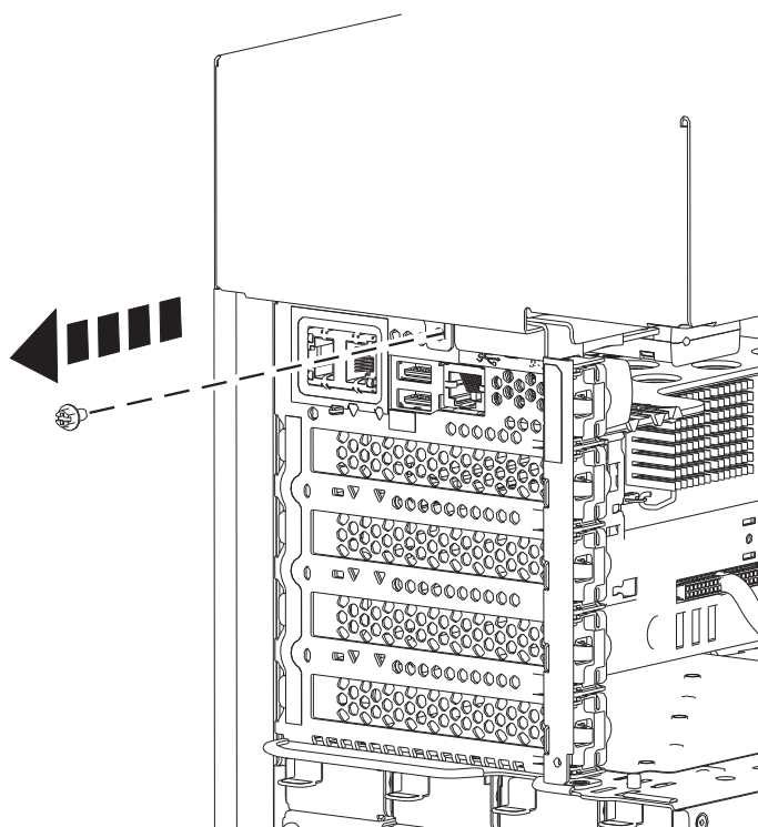
Figura 10. Remover o parafuso da tampa lateral 8286-41A
