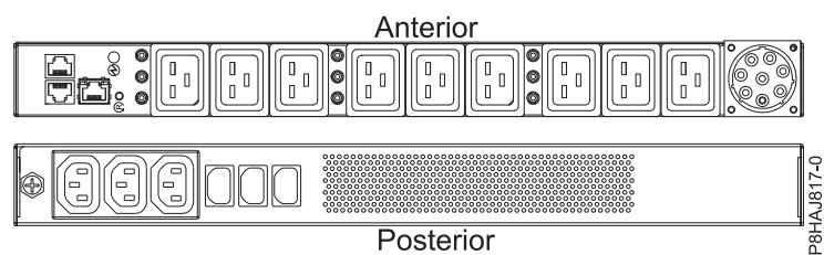
Figura 39. PDU para o sistema 8408-44E
