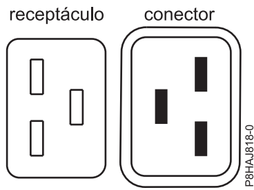
Figura 32. Conectores para o sistema 8408-44E
