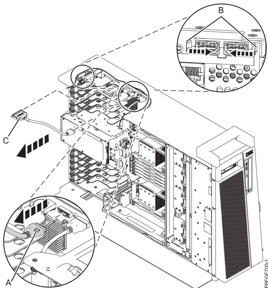
Figura 2. Remover o cabo USB posterior da versão autónoma do 8286-41A
