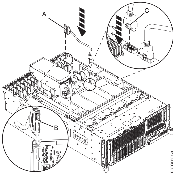
Figura 3. Substituir o cabo USB posterior
