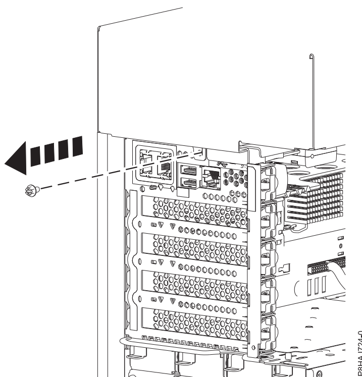
Figura 12. Remover o parafuso da tampa lateral 8286-41A
