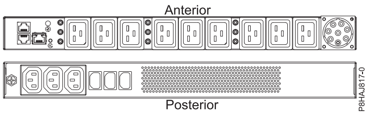
Figura 35. PDU para o sistema 8408-44E
