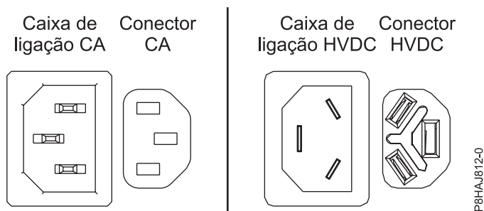
Figura 39. Conectores de AC e HVDC
