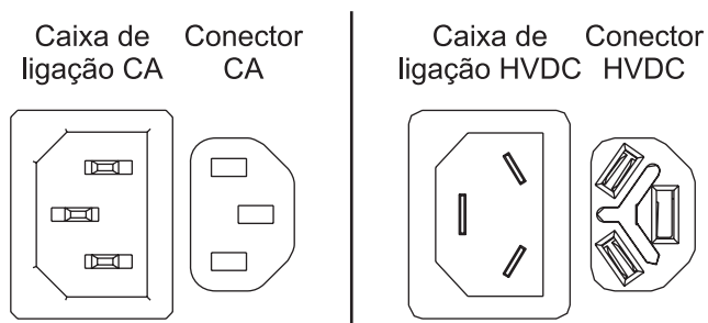
Figura 44. Conectores de CA e de HVDC
