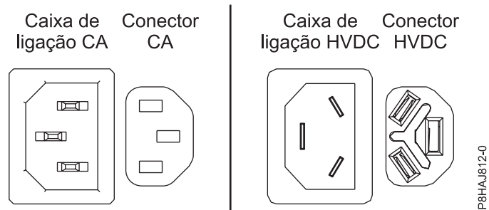
Figura 38. Conectores de CA e de HVDC
