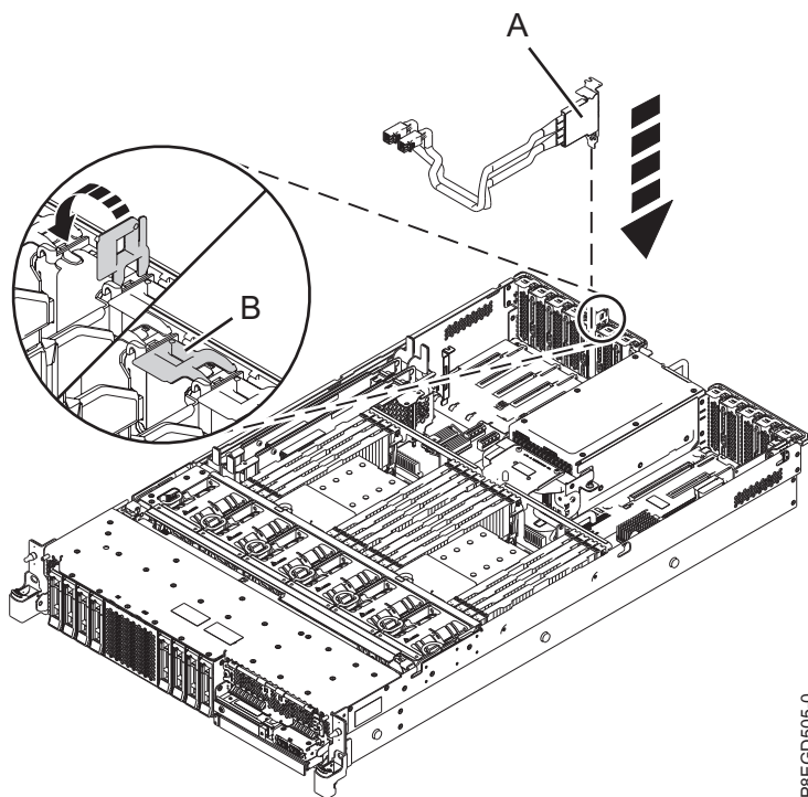
Figura 5. Instalar o cabo SAS posterior
