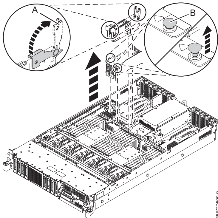
Figura 1. Remover a caixa e as placas dos módulos de alimentação de reserva
