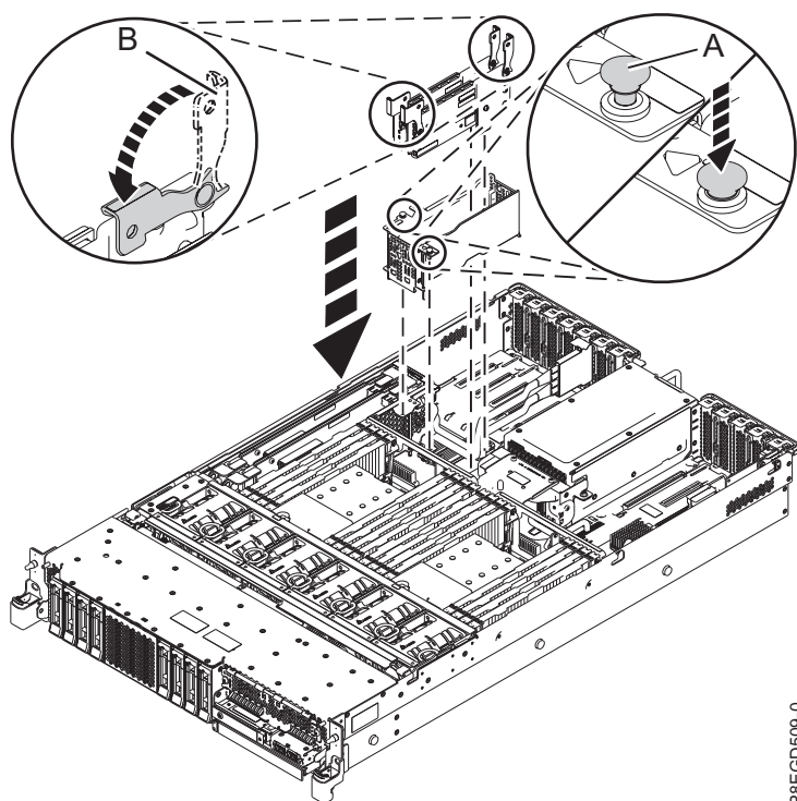
Figura 9. Substituir a estrutura do módulo de alimentação
