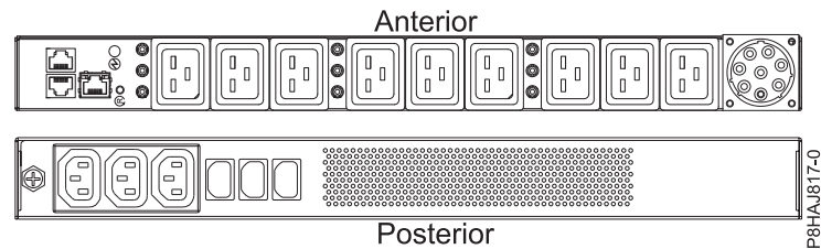
Figura 18. PDU para o sistema 8408-44E
