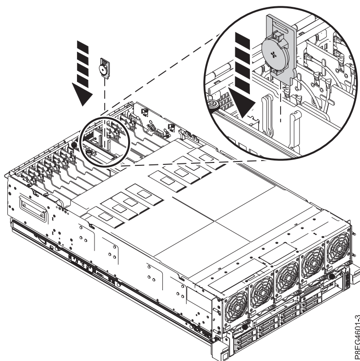
Figura 3. Inserir a placa da pilha do relógio na ranhura P1-C5-C1
