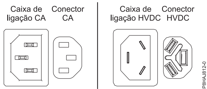
Figura 16. Conectores AC e HVDC
