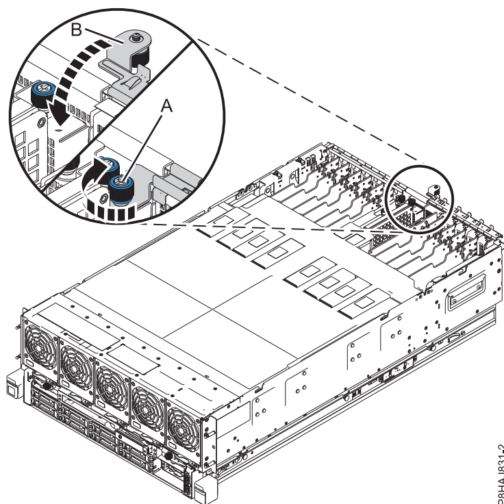
Figura 13. Fechar o trinco de E/S
