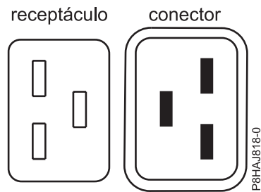
Figura 17. Conectores para o sistema 8408-44E
