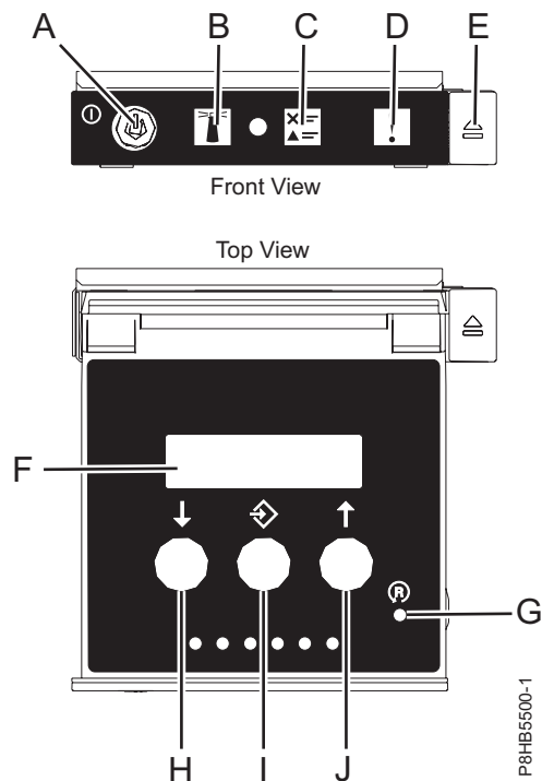
Figura 5. Painel de controlo
