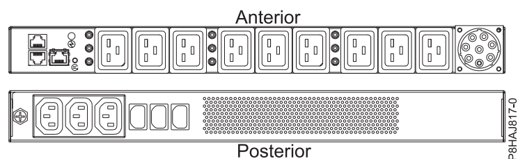
Figura 24. PDU para o sistema 8408-44E
