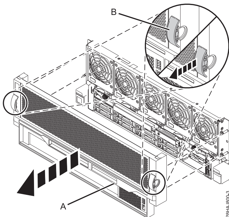
Figura 6. Remover a tampa anterior
