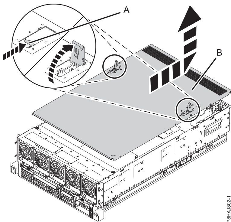
Figura 8. Remover a tampa de acesso para assistência
