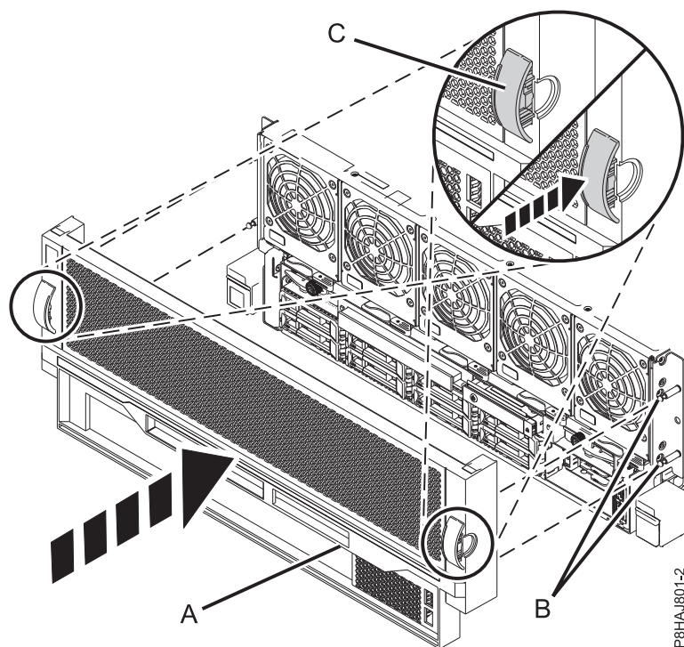
Figura 7. Instalar a tampa anterior
