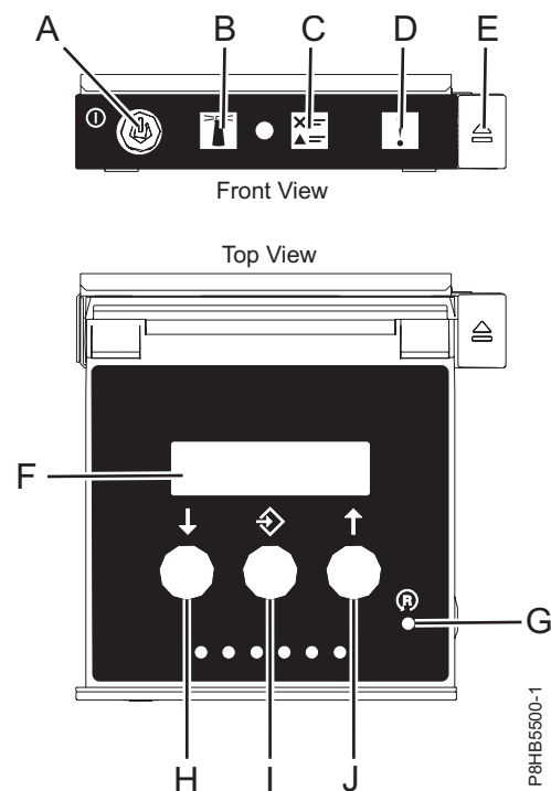
Figura 4. LEDs do painel de controlo
