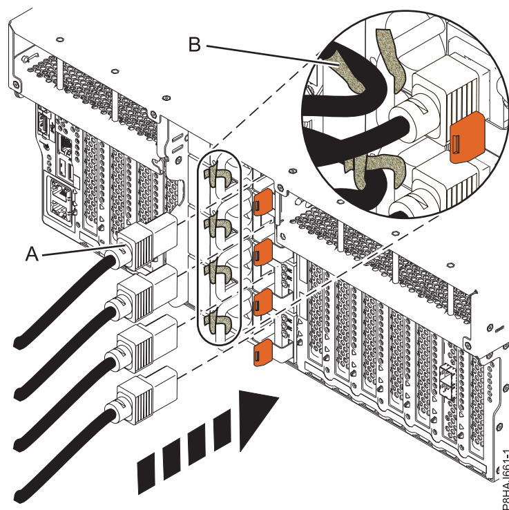
Figura 25. Ligar os cabos de alimentação a um sistema 8247-42L, 8286-41A ou 8286-42A
