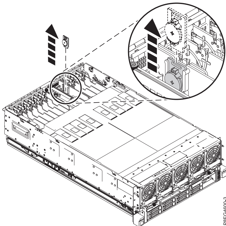
Figura 2. Remover a placa da pilha do relógio da ranhura P1-C5-C1
