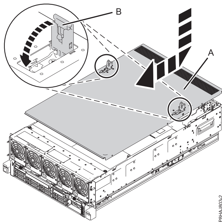
Figura 9. Instalar a tampa de acesso para assistência
