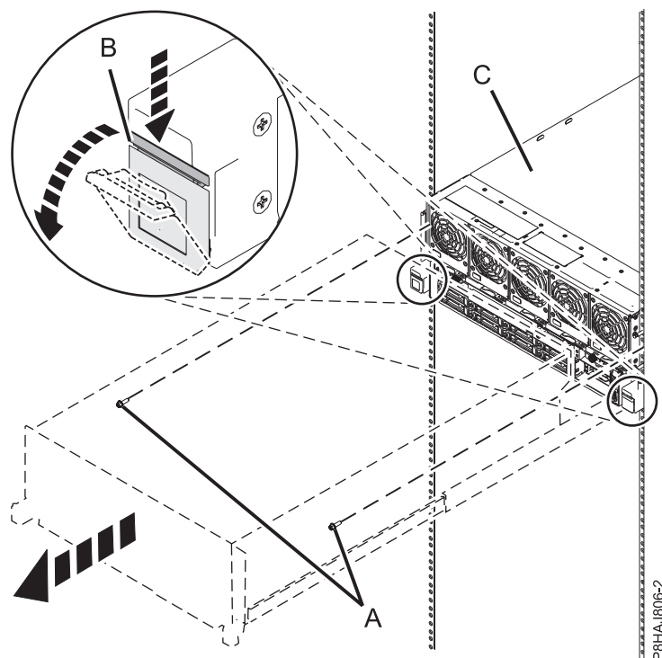
Figura 14. Colocar o sistema na posição de assistência
