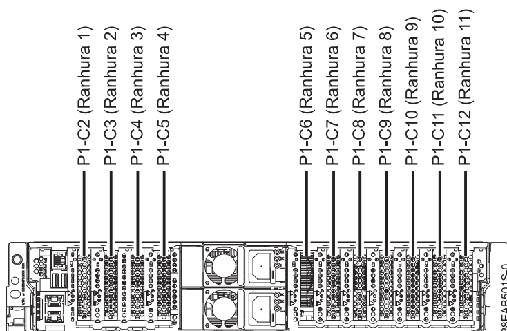
Figura 1. Vista posterior de um sistema 5148-21L, 5148-22L, 8247-21L,8247-22L,8284-21A ou 8284-22A com códigos de localização de ranhuras PCIe
