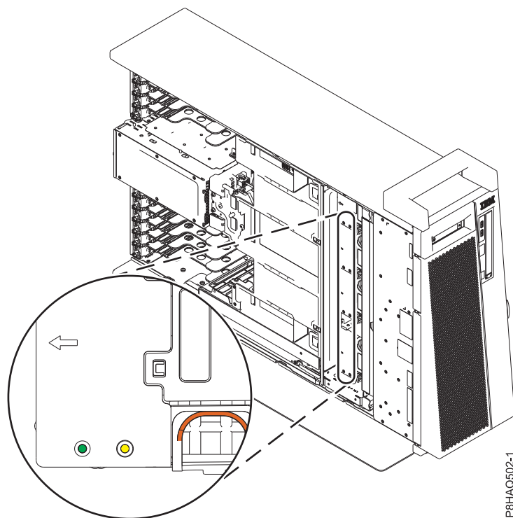
Figura 2. Os LEDs no compartimento do ventilador para AMDs em um sistema independente
