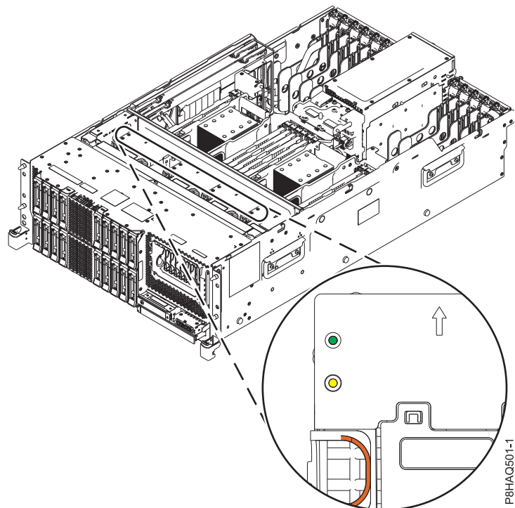
Figura 1. Os LEDs no compartimento do ventilador para AMDs em um sistema montado em rack
