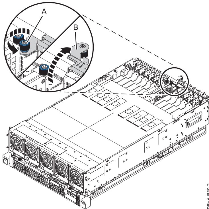
Figura 42. Abrindo a trava de E/S
