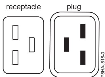
Figura 60. Conectores do sistema 8408-44E
