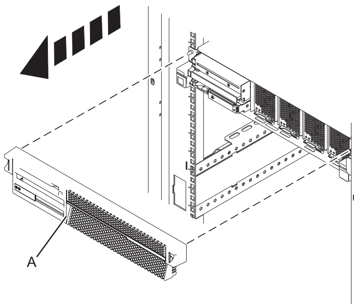
Figura 45. Removendo a tampa frontal da unidade de controle do sistema
