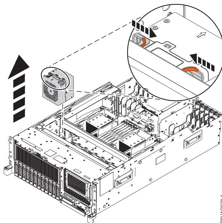
Figura 3. Removendo o ventilador de um sistema montado em rack
