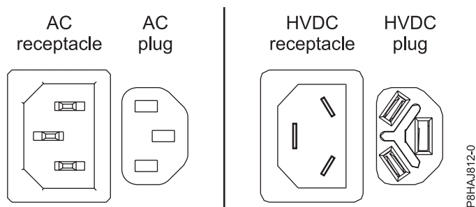
Figura 59. Conectores AC e HVDC
