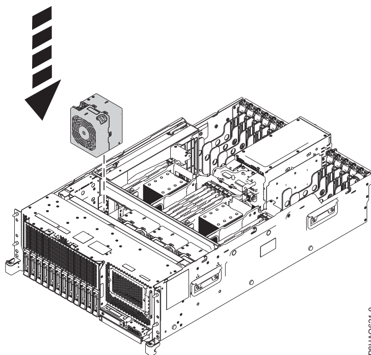
Figura 5. Substituindo o ventilador em um sistema montado em rack
