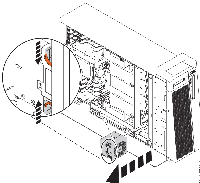
Figura 4. Removendo o ventilador de um sistema independente
