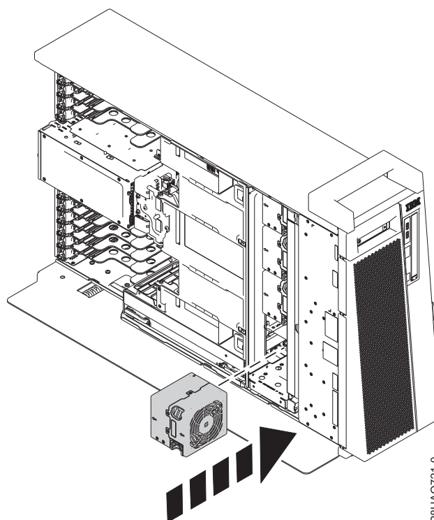
Figura 6. Substituindo o ventilador em um sistema independente
