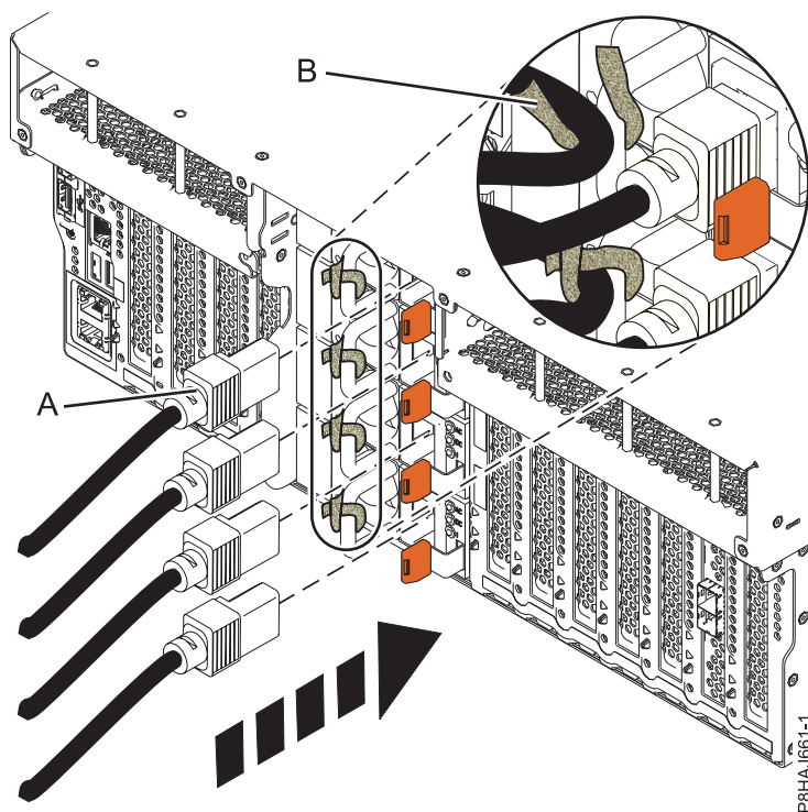
Figura 62. Conectando os cabos de energia a um sistema 8247-42L, 8286-41A ou 8286-42A
