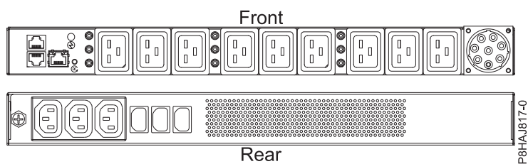
Figura 61. O PDU para o sistema 8408-44E
