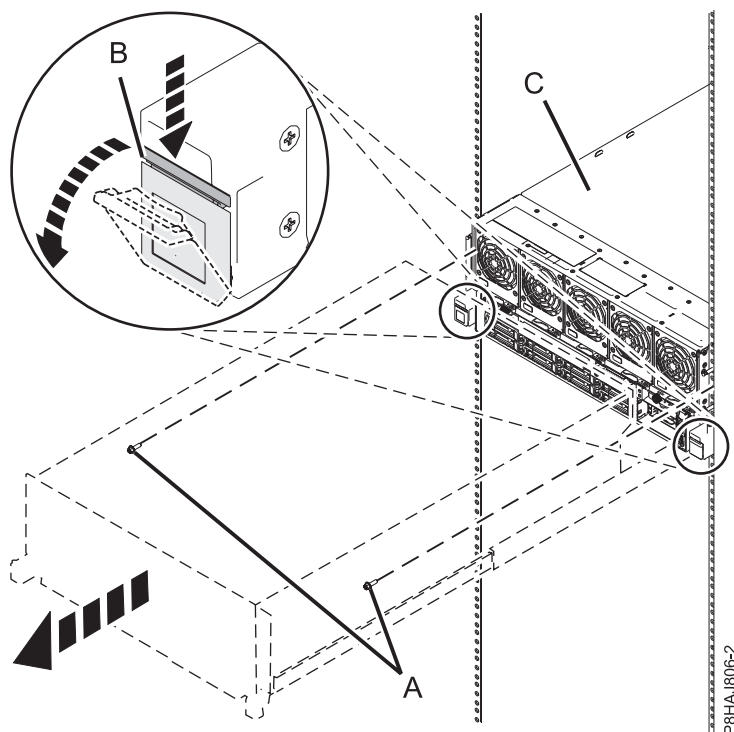
Figura 51. Colocando o sistema na posição de serviço
