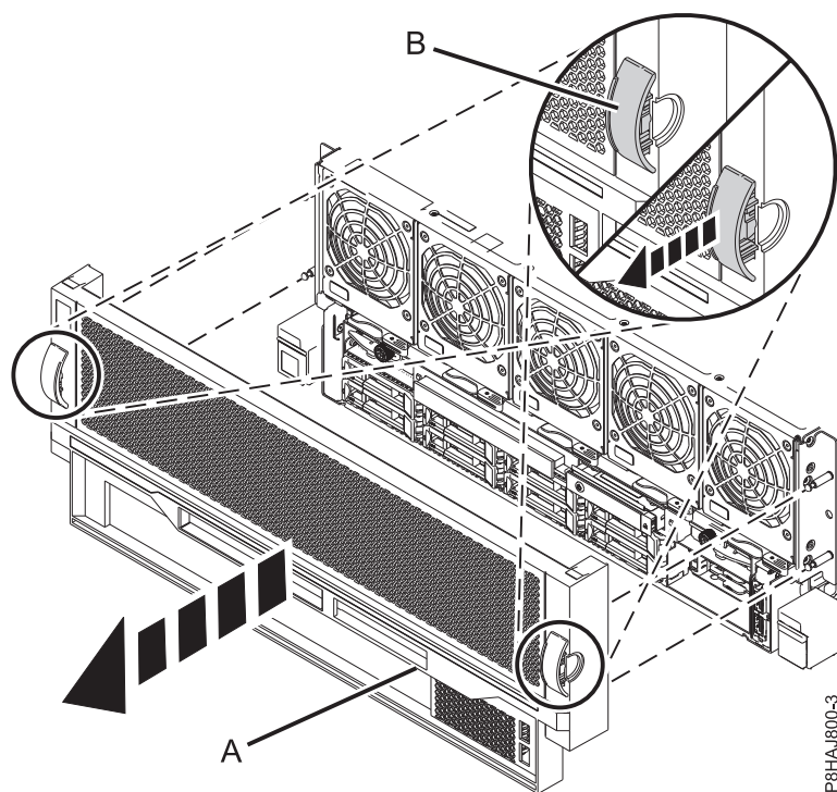
Figura 36. Removendo a Tampa Frontal
