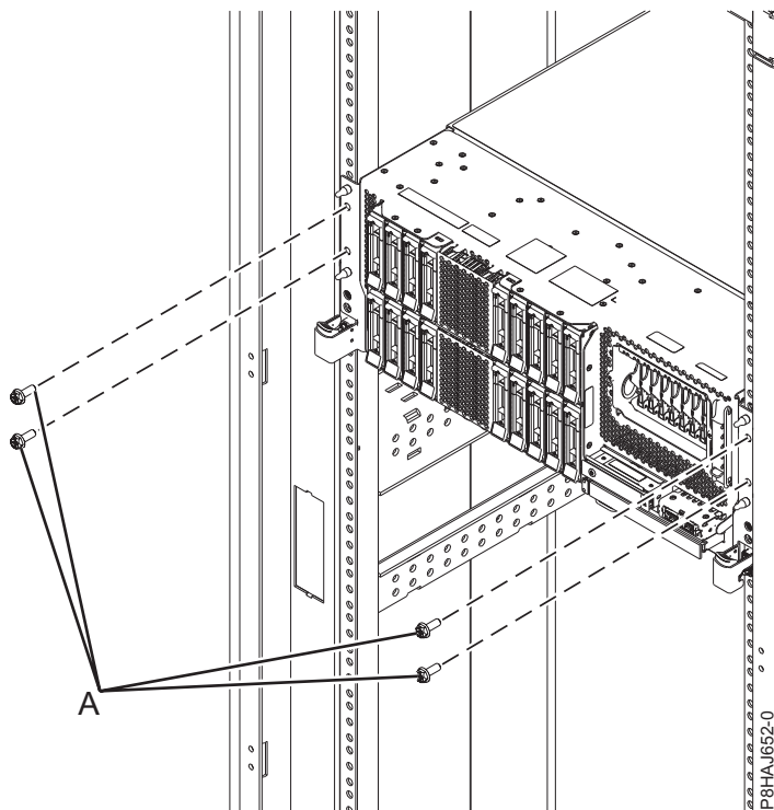
Figura 48. Removendo os parafusos frontais
