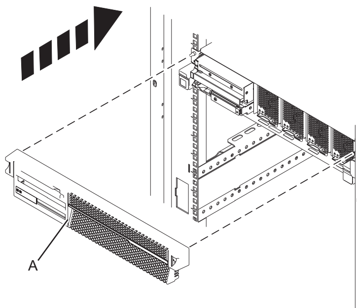
Figura 47. Instalando a tampa frontal da unidade de controle do sistema
