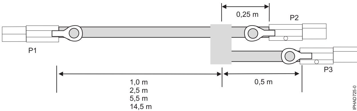
Figura 54. Comprimentos de cabo do conjunto de cabos YO externos SAS
