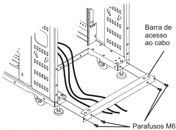
Figura 28. Barra de acesso do cabo
