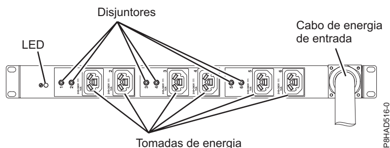
Figura 49. PDU HVDC
