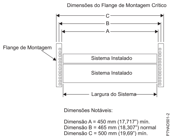
Figura 43. Dimensões de flange de montagem críticas
