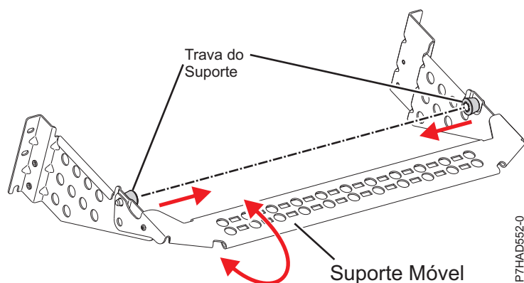
Figura 52. Suporte de gerenciamento de cabos
