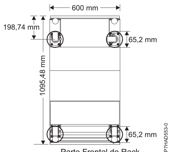
Parte Frontal do Rack Figura 26. Localizações do suporte inclinado de rodas
