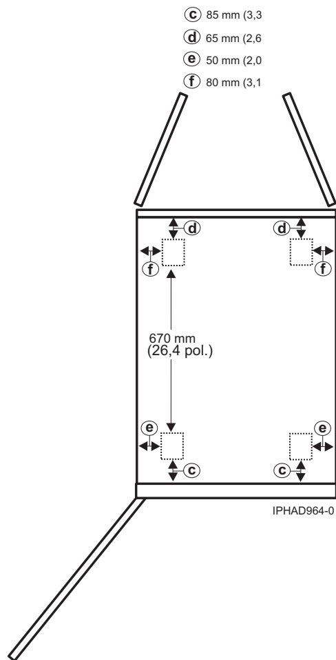
Figura 20. Localizações do suporte inclinado de rodas dos modelos 0555 e 7014-S25
