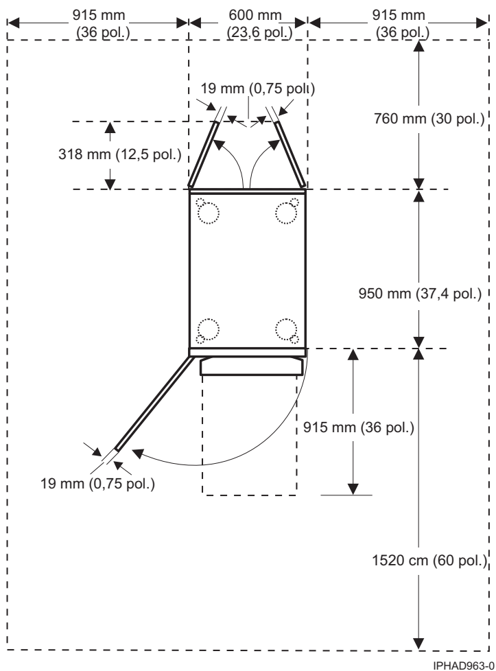
Figura 19. Visualização do plano dos modelos 0555 e 7014-S25
