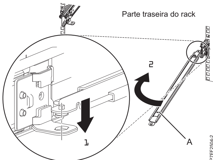
Figura 10. Conectando o Braço do Suporte
