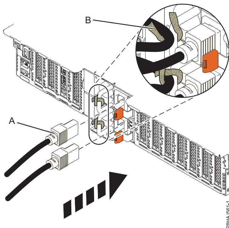
Figura 19. Conectando os cabos de energia à fonte de alimentação e conectando cabos às alças da fonte de alimentação
