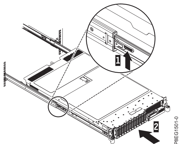
Figura 8. Instale o servidor no rack
