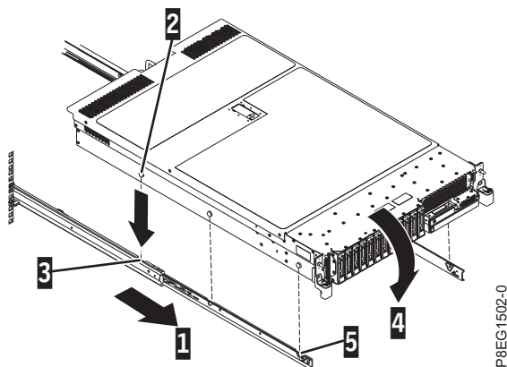
Figura 7. Ampliando os Trilhos Deslizantes e Alinhando as Cabeças dos Pregos do Servidor com os Slots no Trilho
