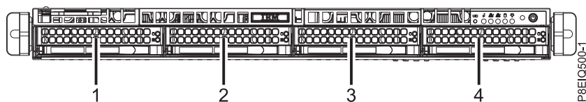
Figura 8. Locais da unidade NVMe
