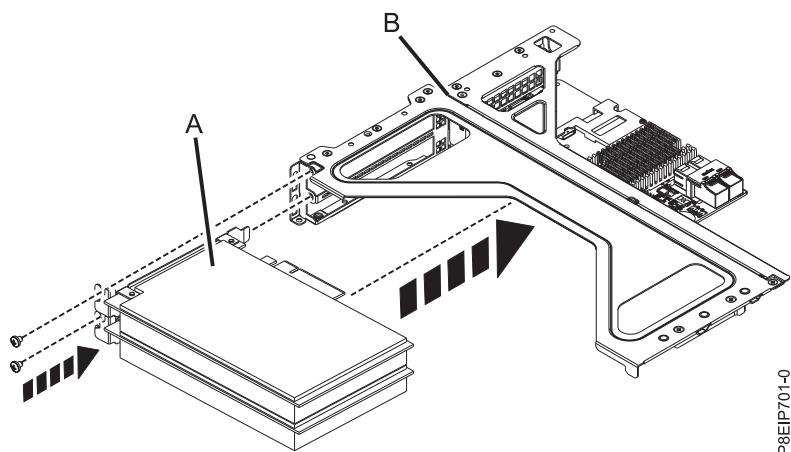
Figura 48. Inserindo um adaptador na posição 4 ou 5 do riser
