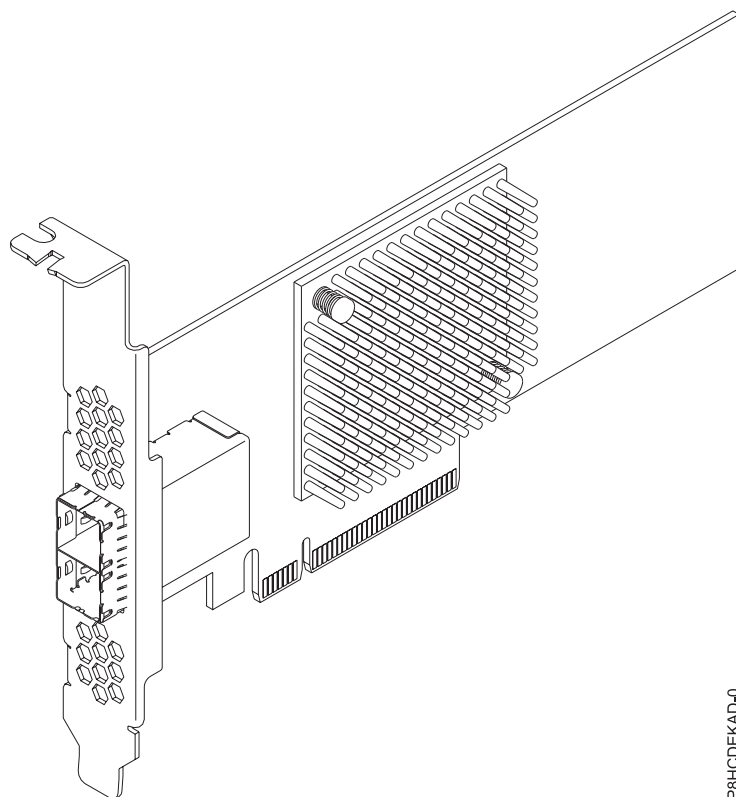
Figura 30. 8-Port SAS-3 3008 Chipset do Adaptador de Armazenamento
