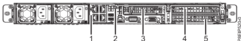
Figura 7. Posições do adaptador PCIe 8001-12C
