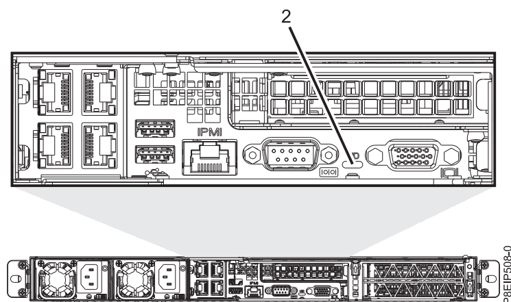
Figura 52. LEDs na parte traseira do sistema
