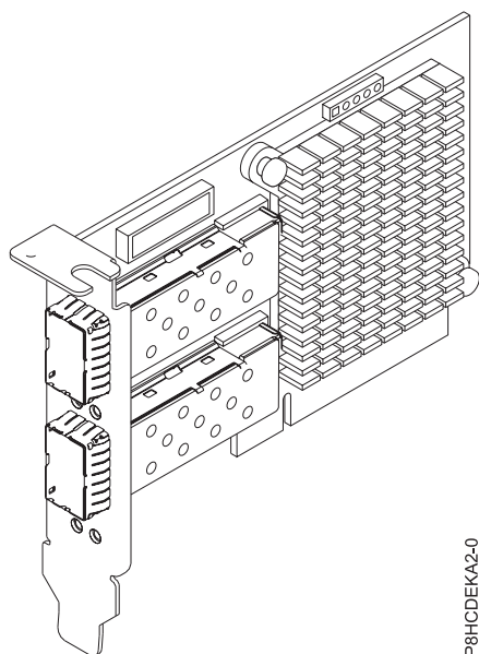
Figura 26. Adaptador PCIe3 Intel 82599ES, duas portas, SFP+ 10 GBe
