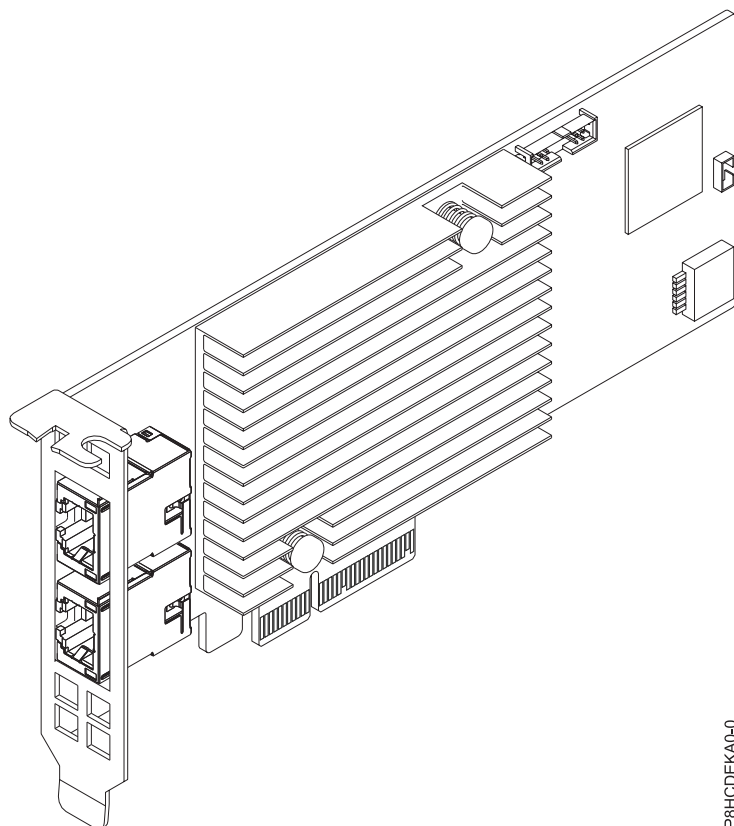
Figura 24. Adaptador 10GBase-T Low-profile Padrão de Porta Dual baseado no Intel X550-A
