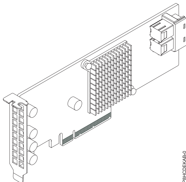
Figura 29. Adaptador RAID Interno SAS Low-profile 12 Gb/s de 8 Portas
