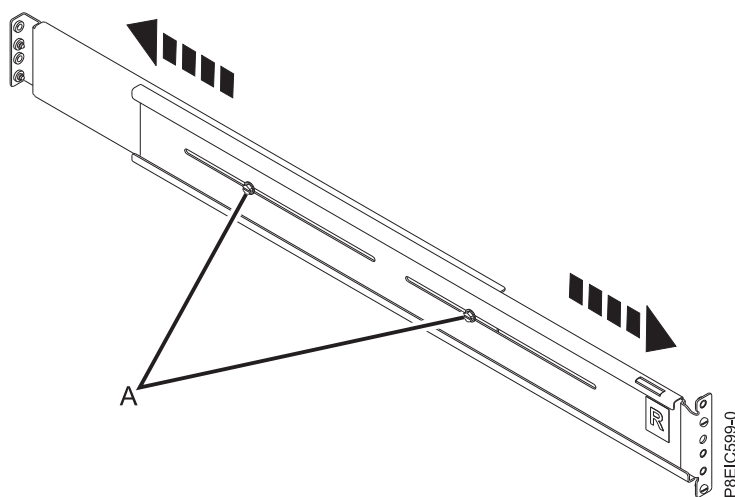
Figura 4. Apertando os dois parafusos no lado do trilho do rack
