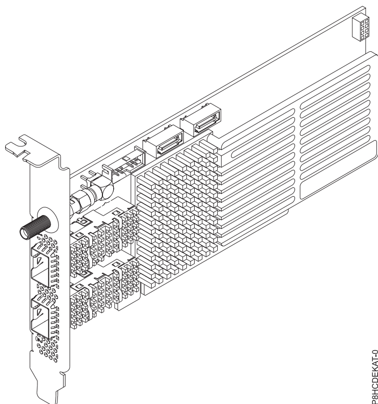
Figura 40. Adaptador Alpha-data CAPI: ADM-PCle KU3
