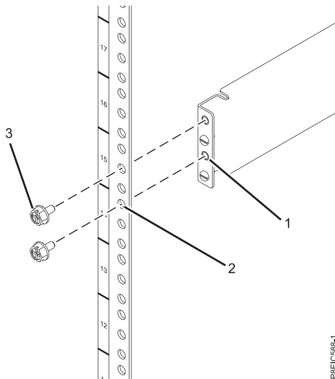
Figura 3. Instalando o trilho fixo na parte traseira do rack
