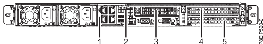
Figura 23. Vista posterior de um sistema 8001-12C com slots PCIe indicados
