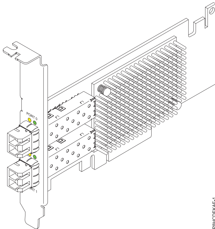
Figura 32. Adaptador de Fibre Channel padrão, perfil baixo, Emulex de 16 Gb/s
