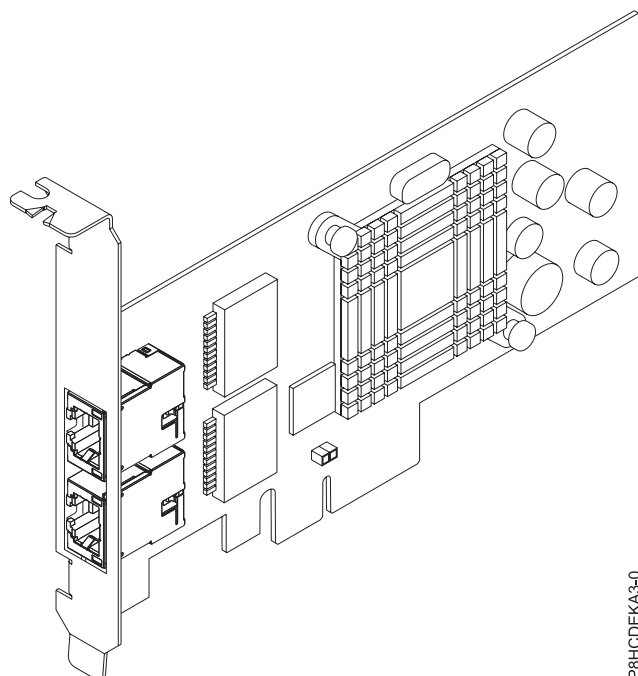
Figura 27. Controlador Gigabit Ethernet Padrão de Porta Dual baseado no Intel PCIe x4
