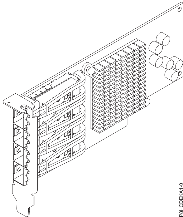
Figura 25. Controlador 10GbE Low-profile Padrão de 4 Portas com Conectores SFP+ baseados no Broadcom BCM57840
