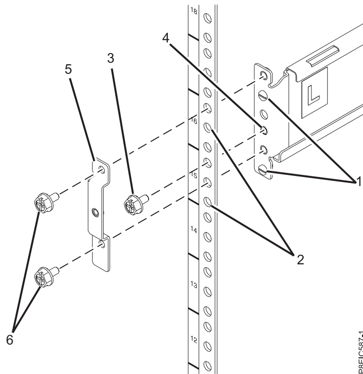
Figura 2. Instalando o trilho fixo na parte frontal do rack
