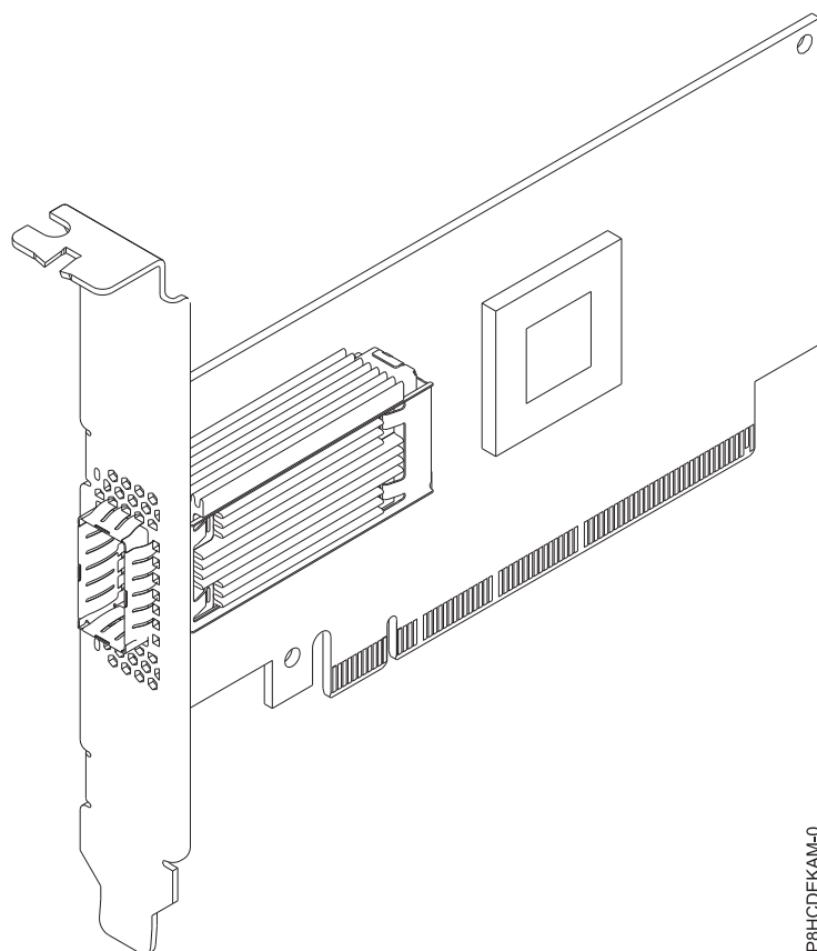
Figura 37. PCIe3 x16 ConnectX-4 EN 100 GbE, porta única, QSFP28 NIC
