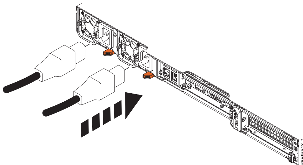
Figura 5. Conectando os cabos de energia às fontes de alimentação
