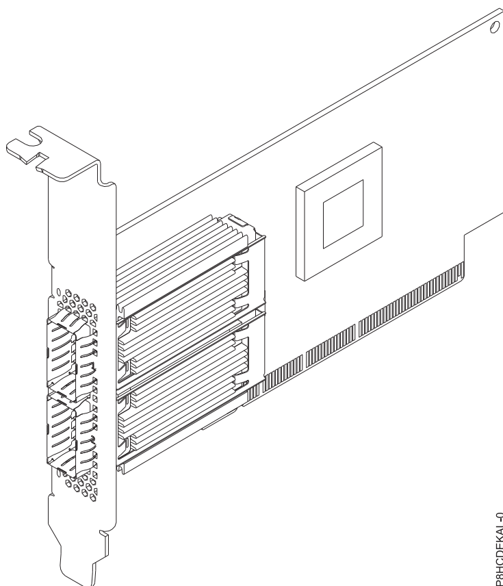
Figura 36. Adaptador Mellanox ConnectX-4 de Porta Dual que suporta 100 Gb/s com VPI
