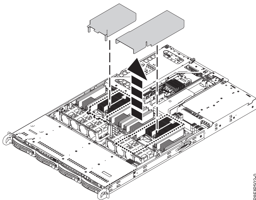
Figura 20. Removendo a placa defletora de ar do processador
