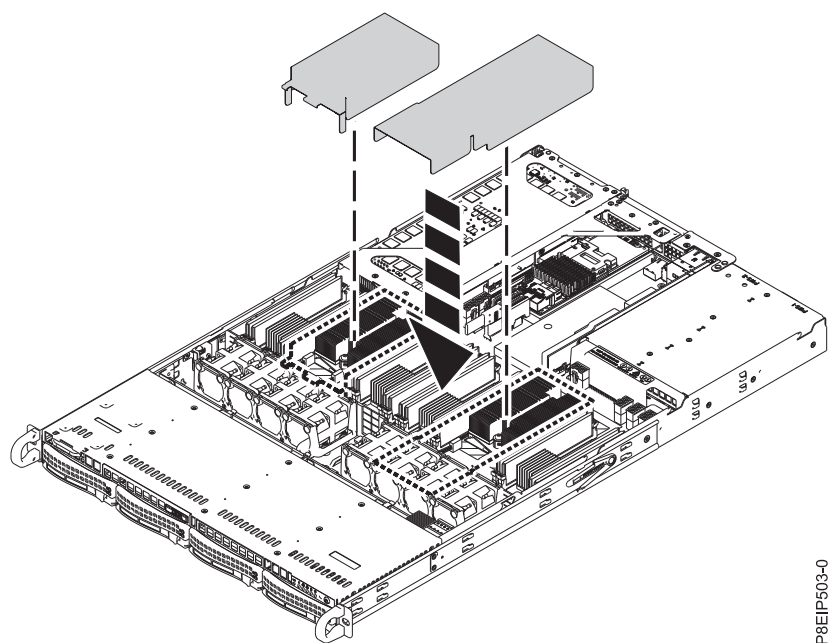
Figura 22. Instalando a placa defletora de ar do processador
