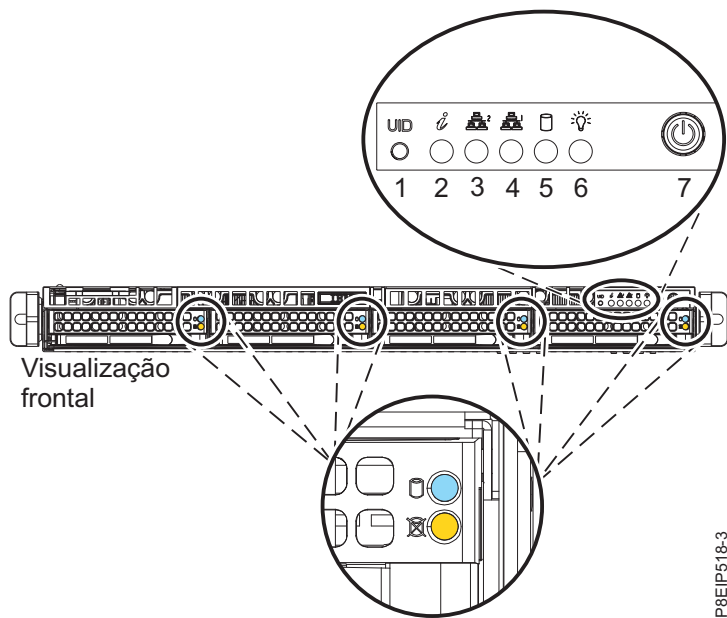
Figura 51. LEDs na parte frontal do sistema
