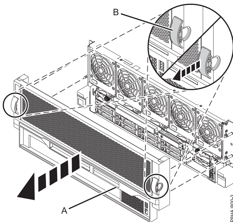
Figura 7. Removendo a cobertura frontal
