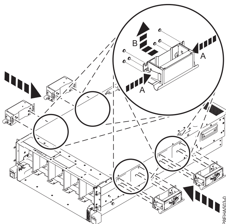
Figura 11. Instalando as alças de elevação
