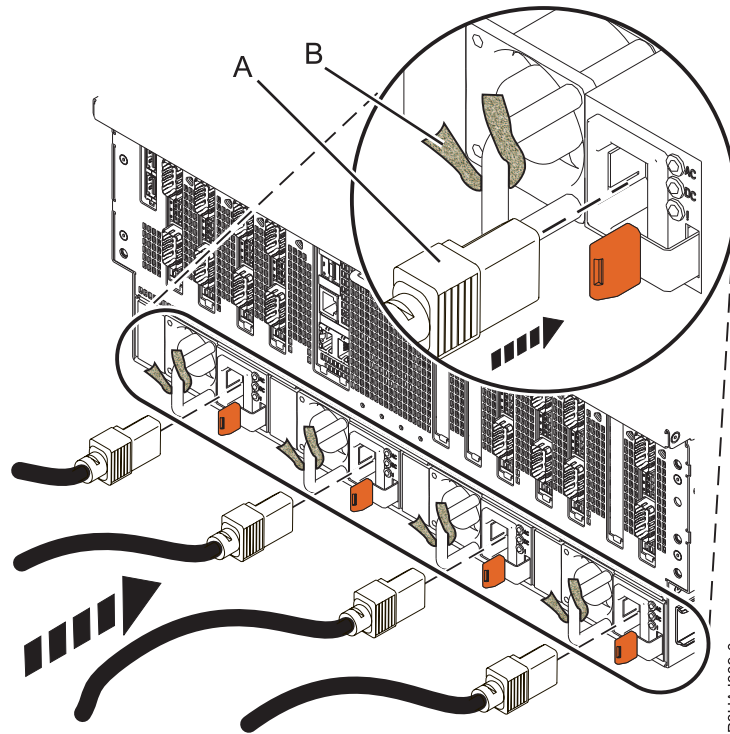
Figura 22. Conectando os cabos de energia e prendendo os cabos com prendedores.
