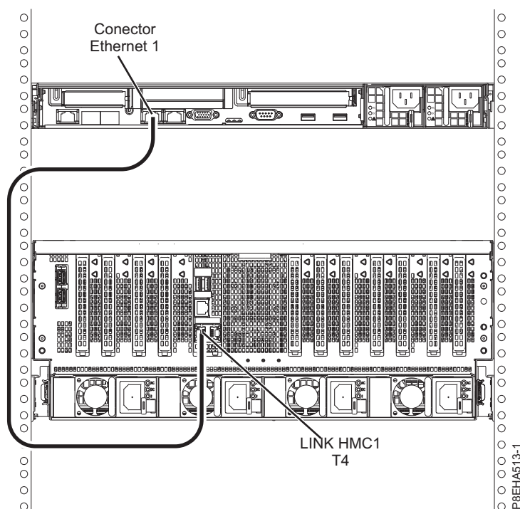
Figura 24. Conectando o HMC diretamente ao sistema gerenciado
