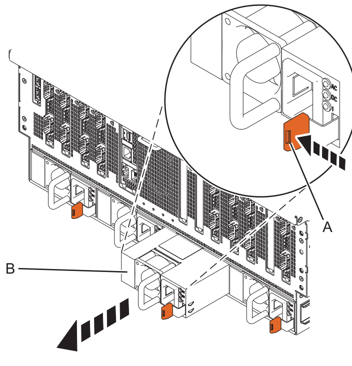
Figura 6. Removendo uma fonte de alimentação da traseira do chassi do sistema
