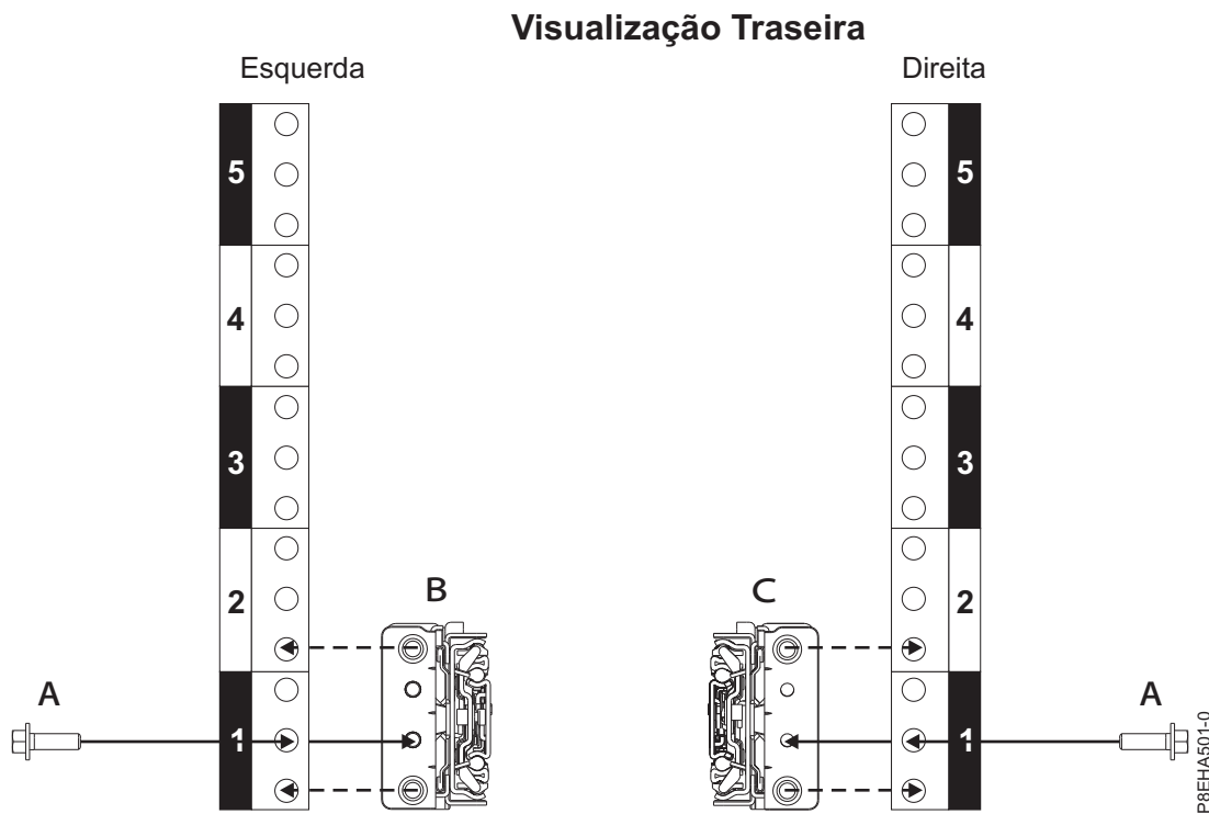
Figura 5. Conectando os trilhos deslizantes na parte traseira do rack
