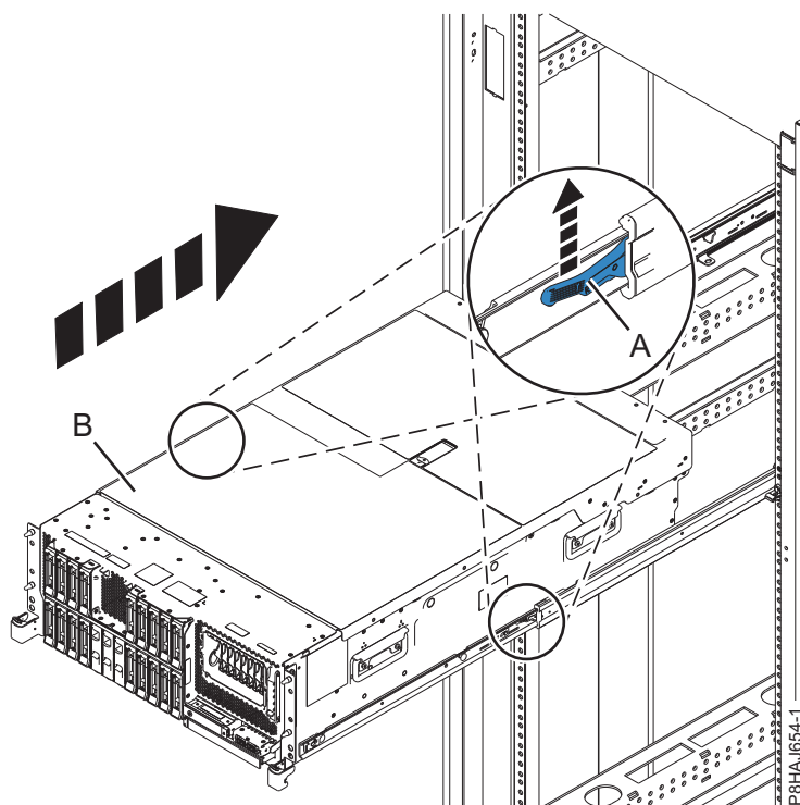
Figura 32. Colocando o Sistema na Posição de Operação
