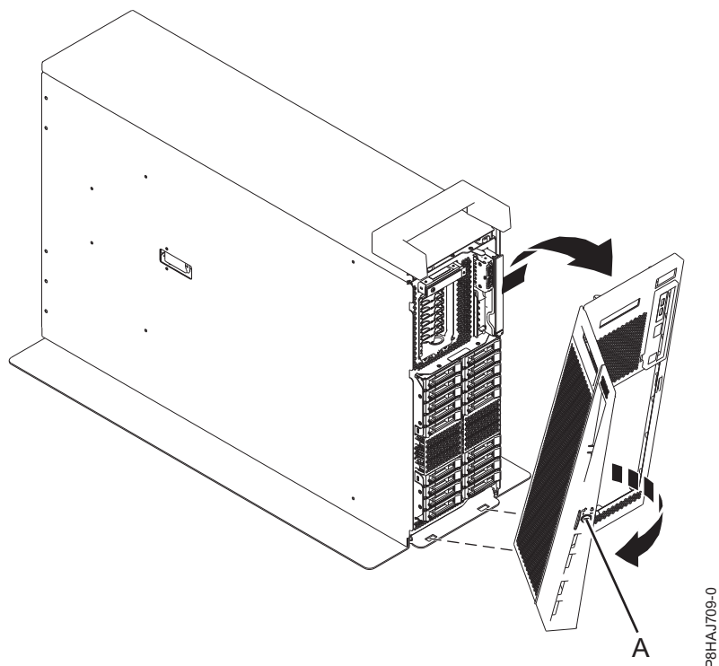
Figura 9. Removendo a Tampa Frontal
