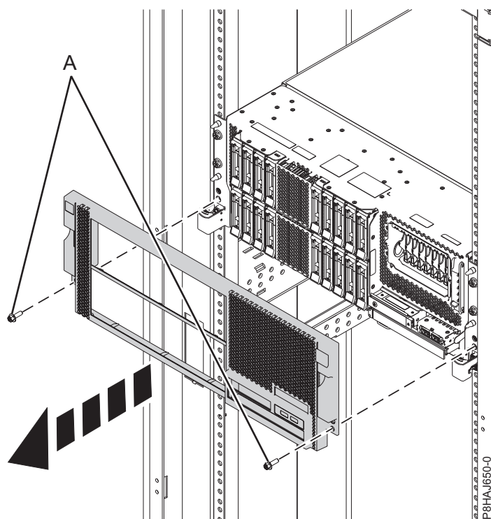
Figura 8. Removendo a Tampa Frontal
