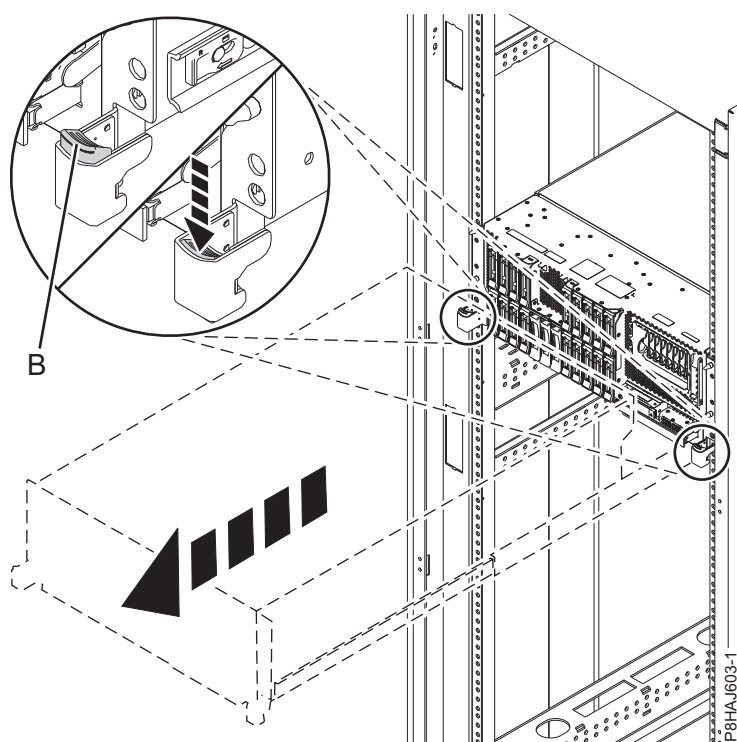
Figura 31. Liberando as Travas Laterais
