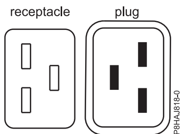
Figura 40. Conectores do sistema 8408-44E
