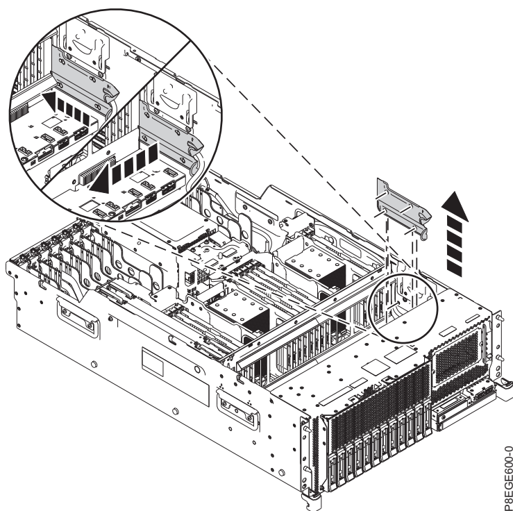
Figura 1. Removendo a tampa do cabo USB
