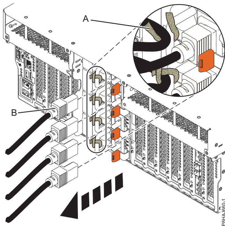
Figura 41. Removendo os cabos de energia de um sistema 8247-42L, 8286-41A ou 8286-42A
