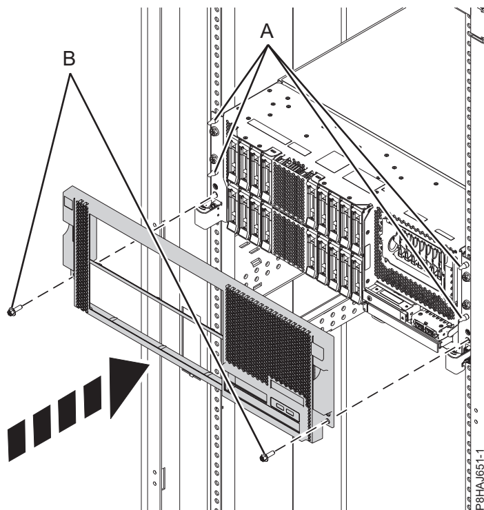
Figura 20. Instalando a Tampa Frontal
