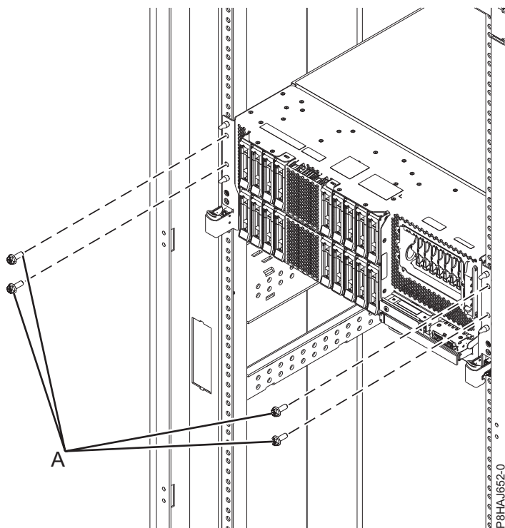
Figura 35. Removendo os parafusos frontais
