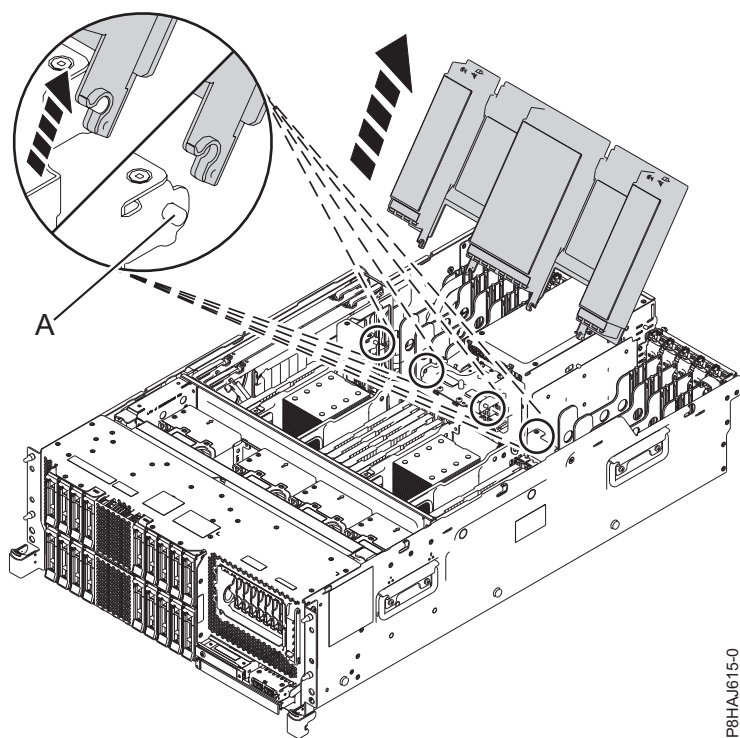
Figura 33. Removendo a placa defletora de ar
