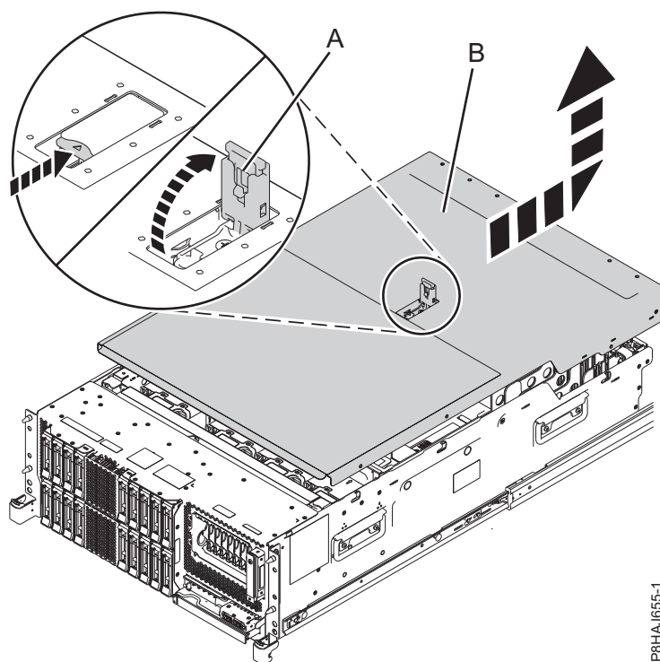
Figura 27. Removendo a Tampa de Acesso de Serviço
