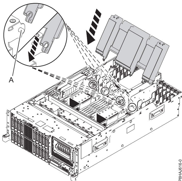
Figura 34. Substituindo a placa defletora de ar
