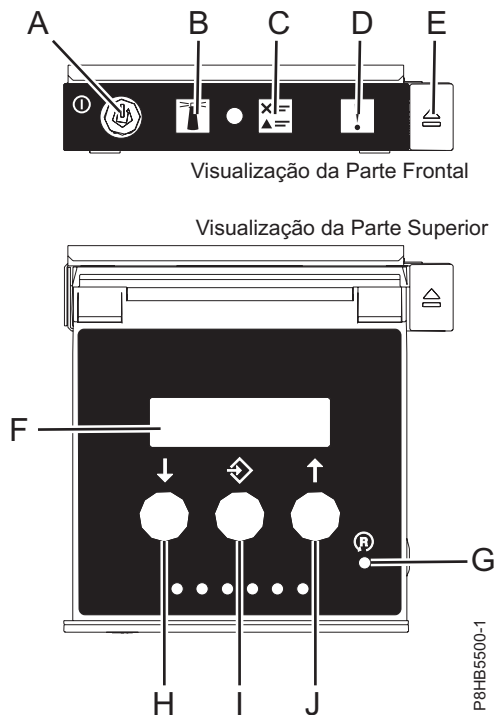
Figura 11. Painel de Controle
