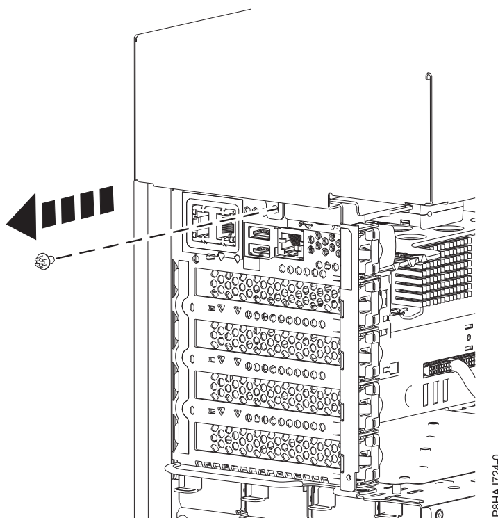
Figura 17. Removendo o parafuso da tampa lateral do 8286-41A
