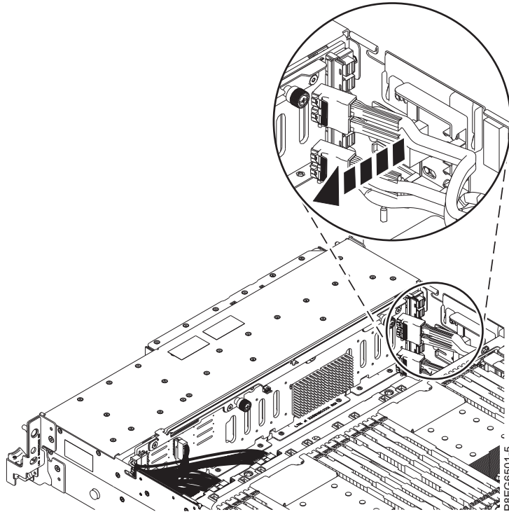
Figura 2. Desprendendo os cabos SAS frontais
