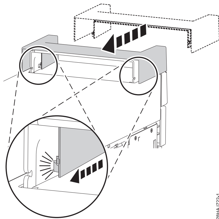
Figura 23. Protegendo a tampa da alça em um sistema 8286-41A independente
