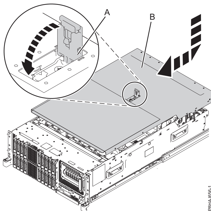
Figura 29. Instalando a Tampa de Acesso de Serviço
