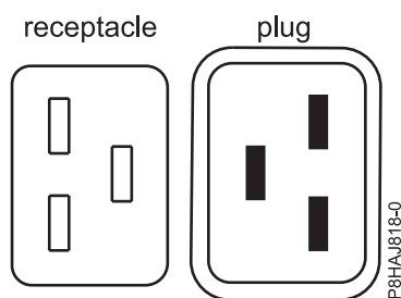
Figura 39. Conectores do sistema 8408-44E
