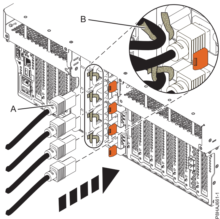
Figura 47. Conectando os cabos de energia a um sistema 8247-42L, 8286-41A ou 8286-42A
