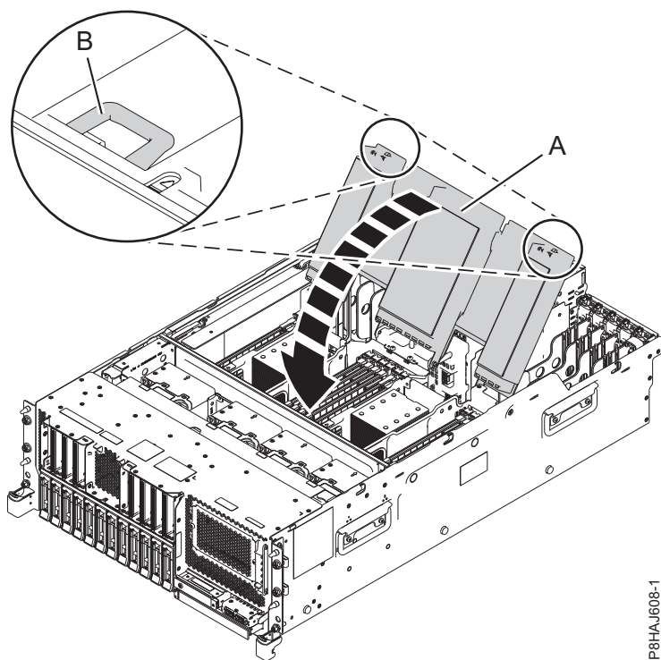
Figura 32. Fechando a placa defletora de ar
