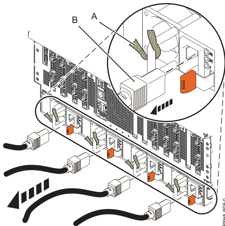
Figura 43. Removendo os cabos de energia de um sistema 8408-44E ou 8408-E8E
