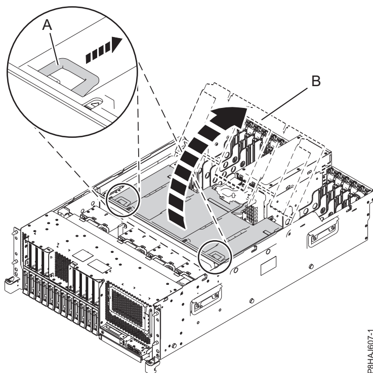
Figura 31. Abrindo a placa defletora de ar
