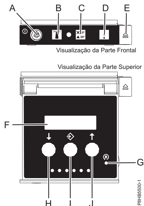
Figura 10. LEDs do Painel de Controle
