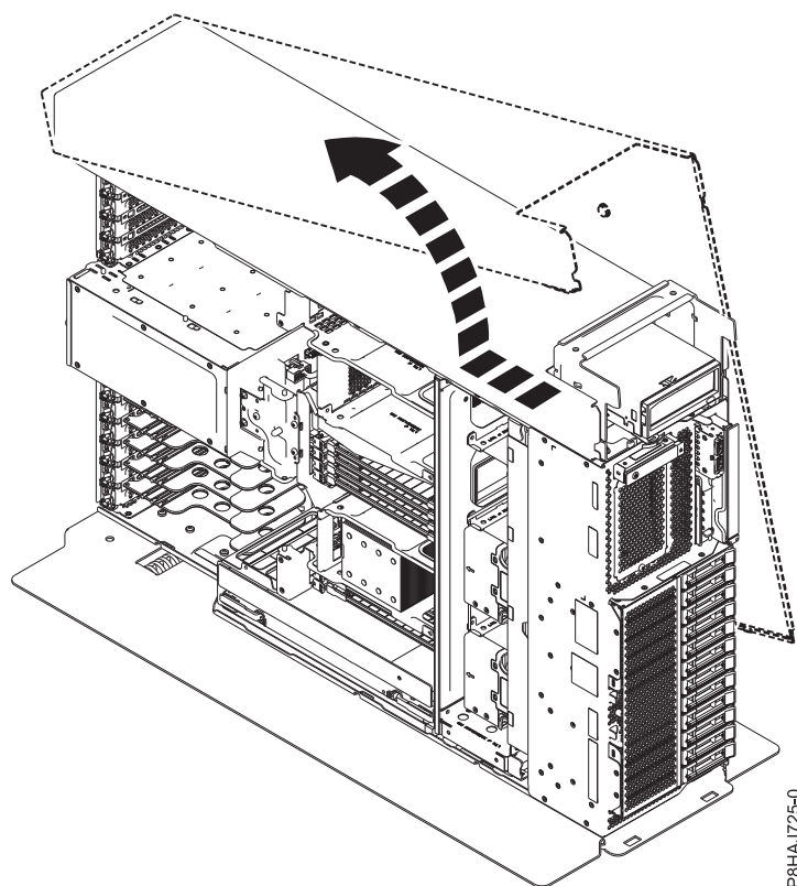
Figura 18. Removendo a tampa lateral do 8286-41A
