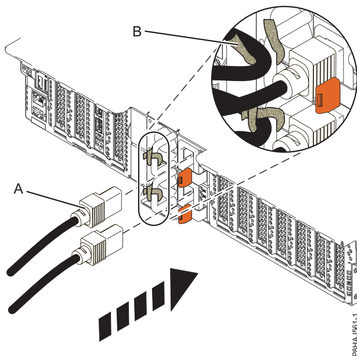
Figura 48. Conectando os cabos de energia a um sistema 5148-21L, 5148-22L, 8247-21L, 8247-22L, 8284-21A ou 8284-22A
