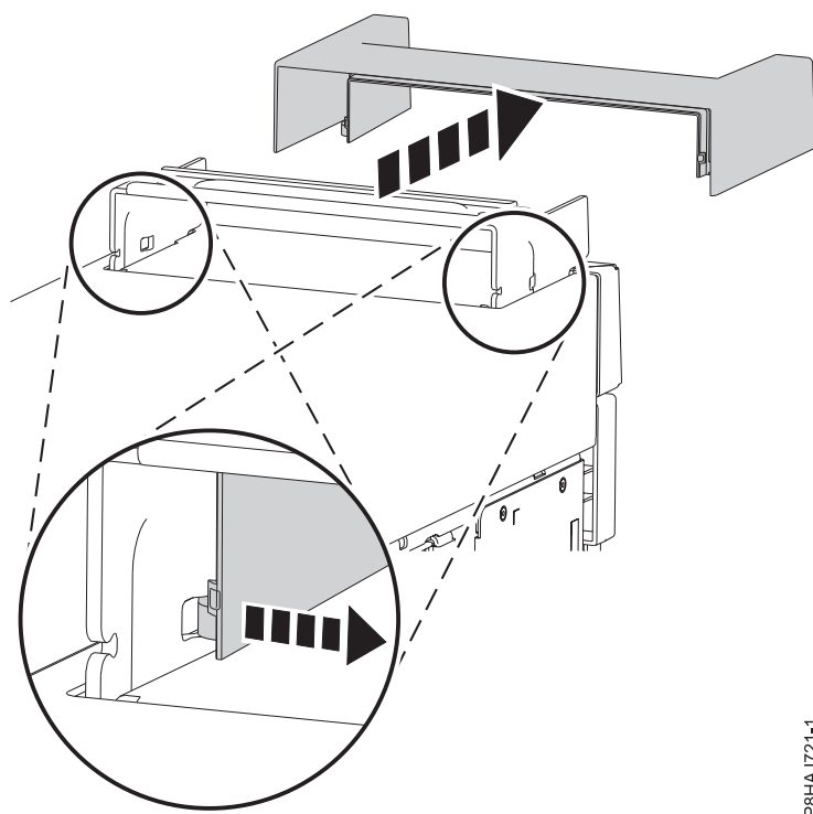
Figura 16. Removendo a tampa da alça de um sistema 8286-41A independente
