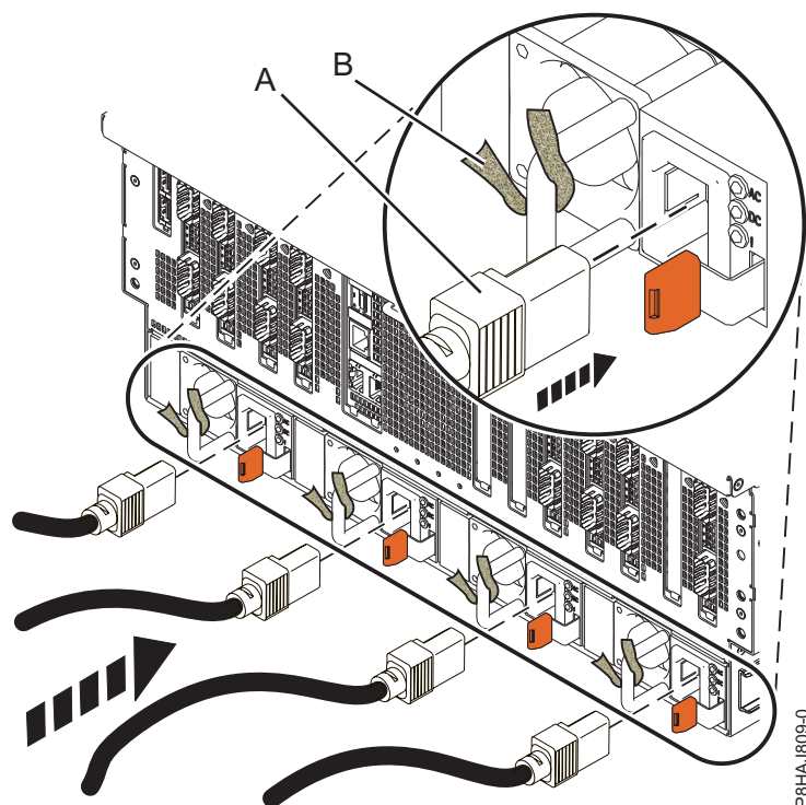
Figura 49. Conectando os cabos de energia a um sistema 8408-44E ou 8408-E8E
