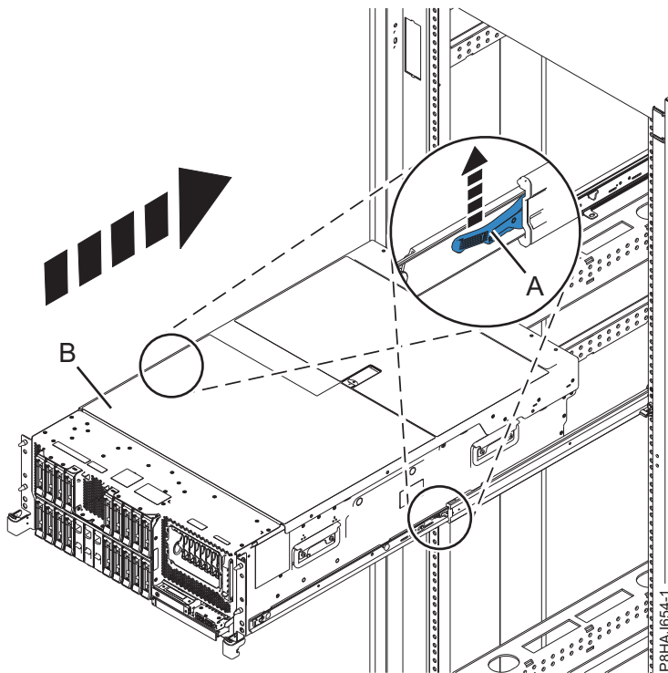
Figura 37. Colocando o Sistema na Posição de Operação
