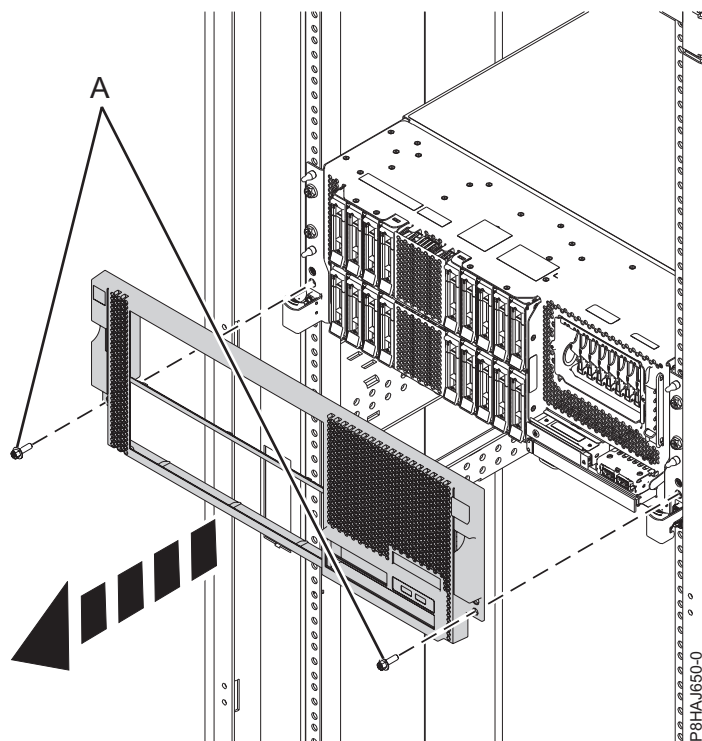
Figura 13. Removendo a Tampa Frontal
