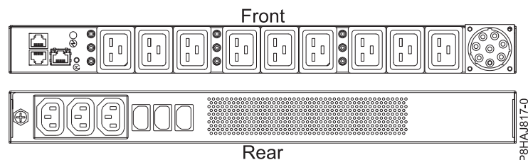
Figura 40. O PDU para o sistema 8408-44E
