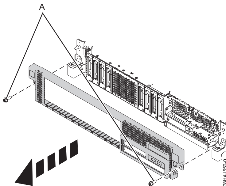
Figura 12. Removendo a Tampa Frontal
