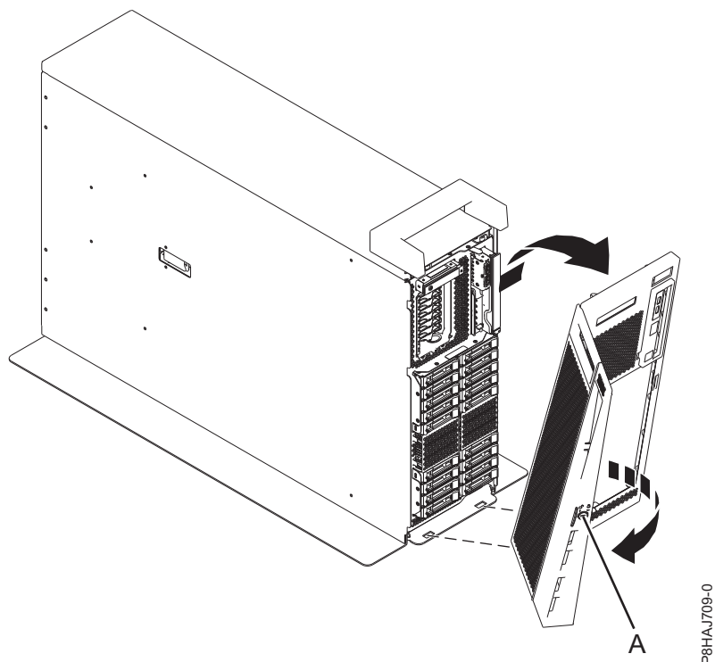
Figura 14. Removendo a Tampa Frontal
