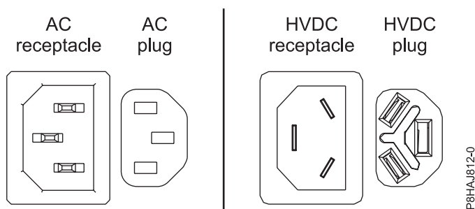
Figura 44. Conectores AC e HVDC
