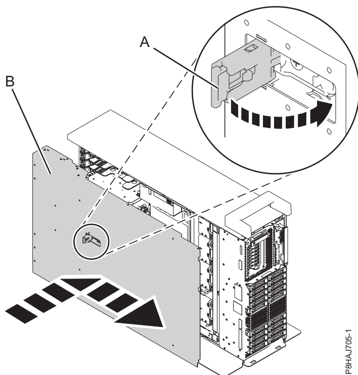
Figura 30. Instalando a Tampa de Acesso de Serviço
