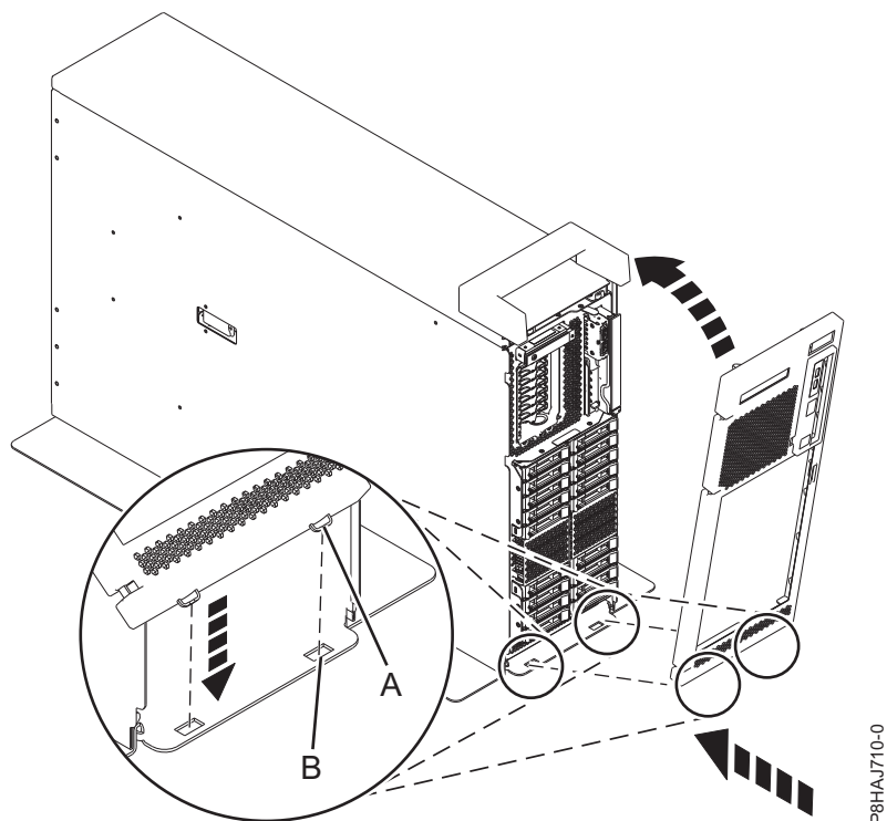
Figura 21. Instalando a Tampa Frontal
