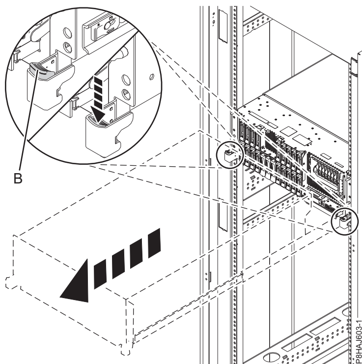
Figura 36. Liberando as Travas Laterais
