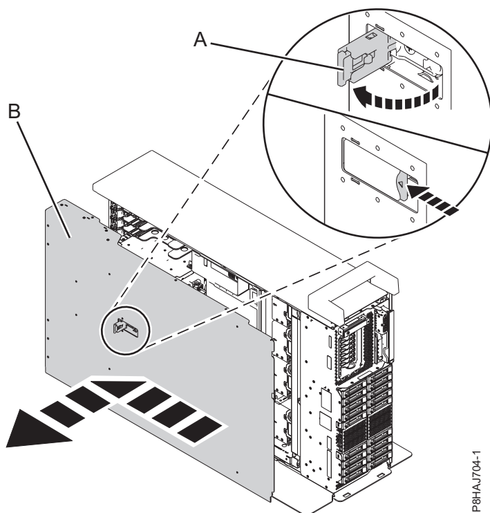
Figura 28. Removendo a Tampa de Acesso de Serviço
