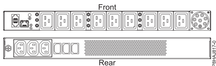
Figura 46. O PDU para o sistema 8408-44E
