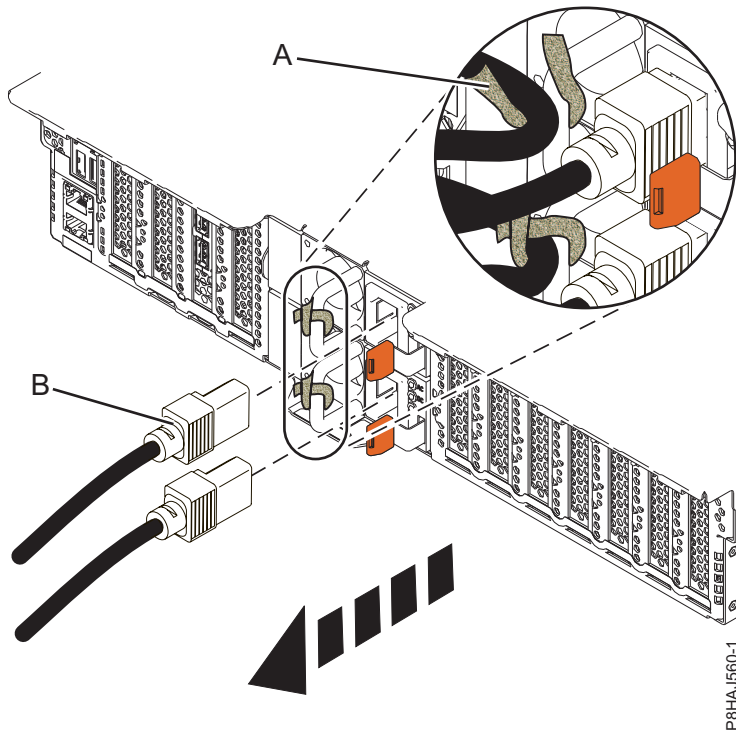
Figura 42. Removendo os cabos de energia de um sistema 5148-21L, 5148-22L, 8247-21L, 8247-22L, 8284-21A ou 8284-22A
