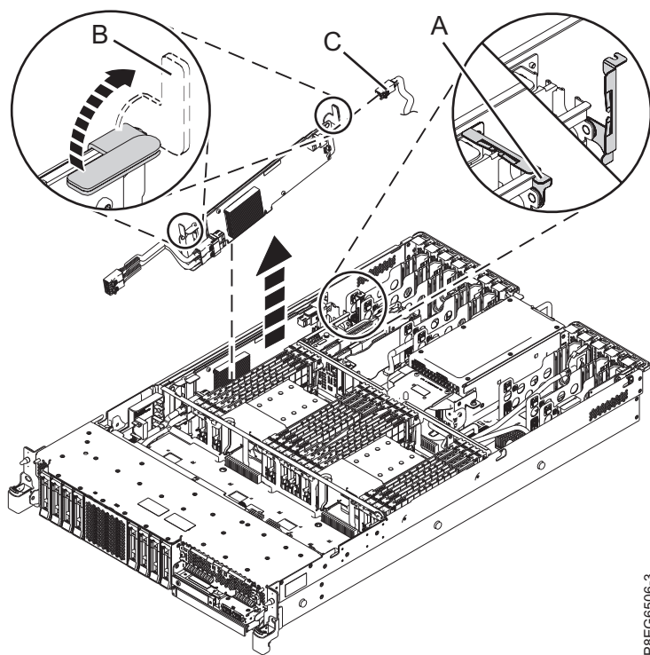
Figura 3. Removendo o adaptador SAS RAID
