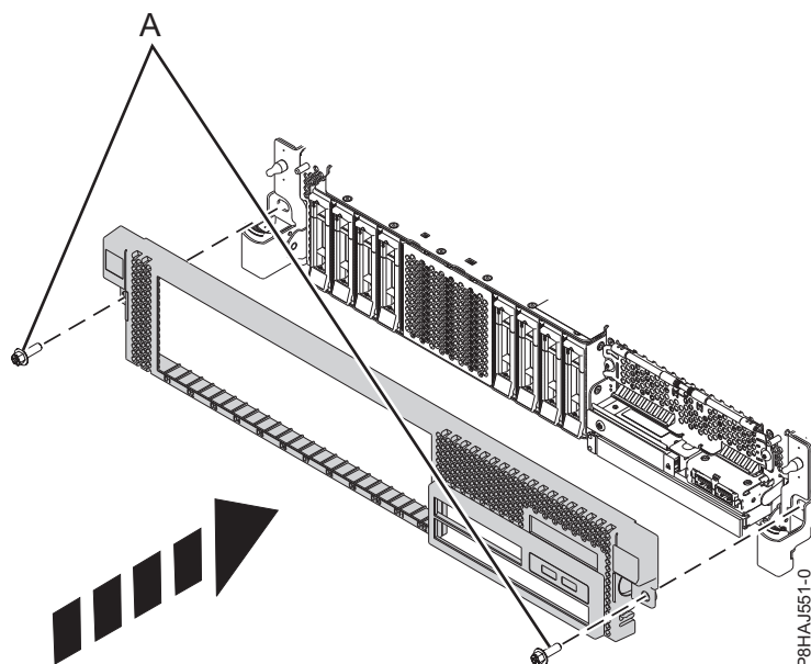
Figura 19. Instalando a Tampa Frontal
