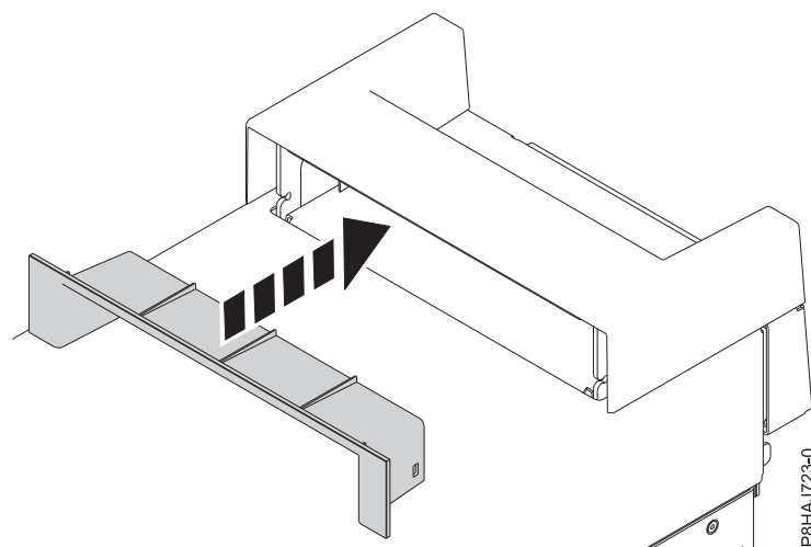
Figura 24. Inserindo a peça dentro da tampa da alça em um sistema 8286-41A independente
