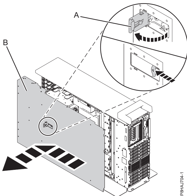
Figura 42. Removendo a Tampa de Acesso de Serviço
