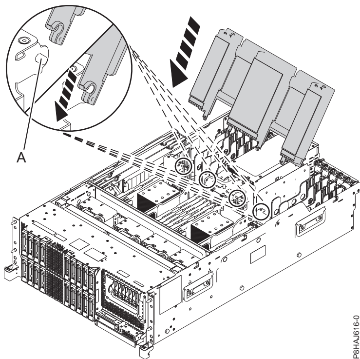
Figura 48. Substituindo a placa defletora de ar
