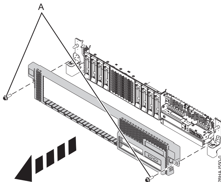
Figura 26. Removendo a Tampa Frontal
