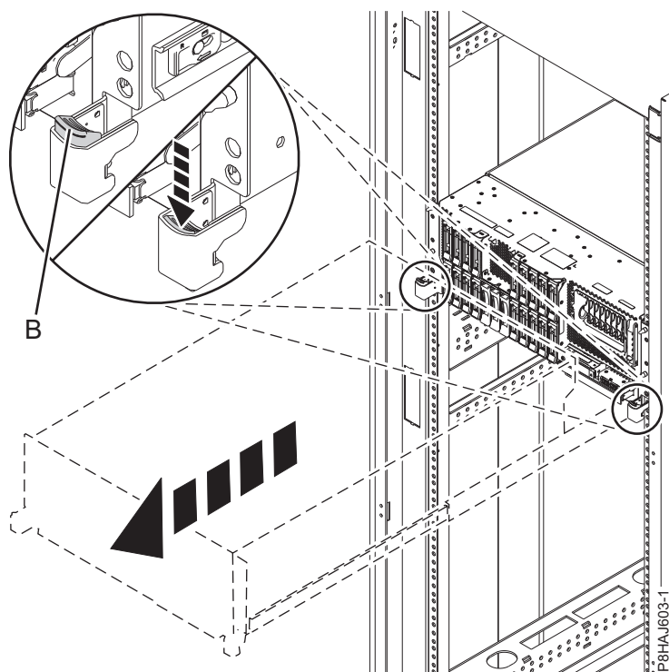
Figura 50. Liberando as Travas Laterais
