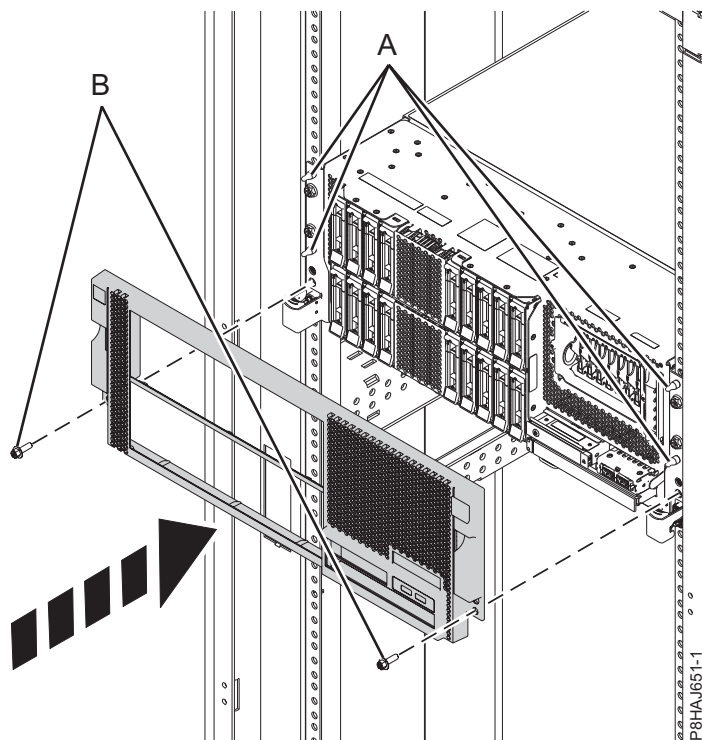
Figura 34. Instalando a Tampa Frontal
