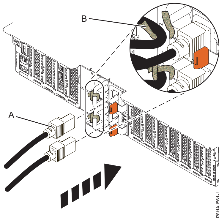
Figura 62. Conectando os cabos de energia a um sistema 5148-21L, 5148-22L, 8247-21L, 8247-22L, 8284-21A ou 8284-22A
