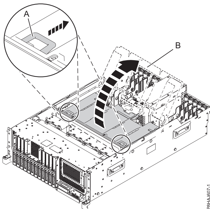
Figura 45. Abrindo a placa defletora de ar
