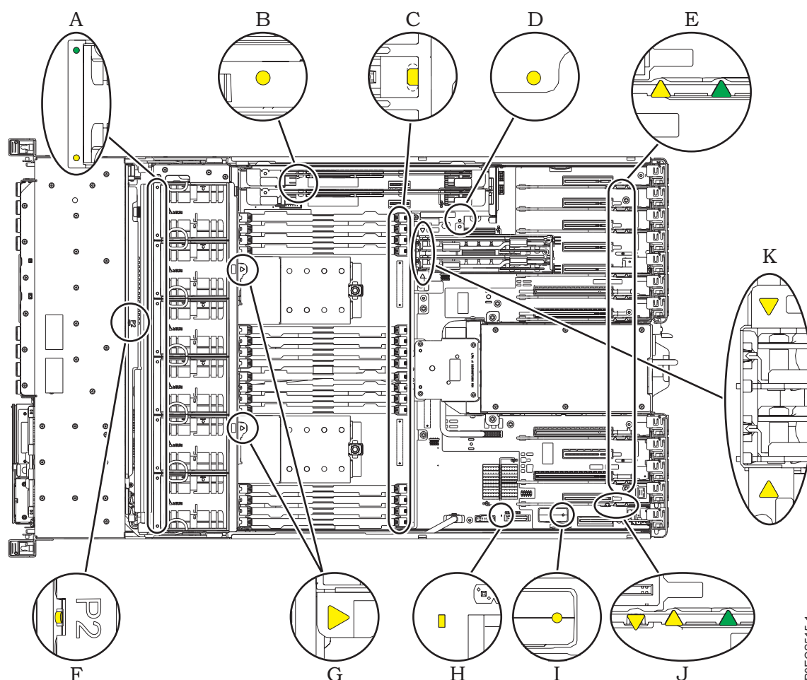
Figura 12. LEDs do indicador de serviço
