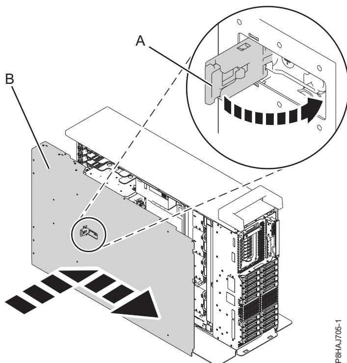
Figura 44. Instalando a Tampa de Acesso de Serviço
