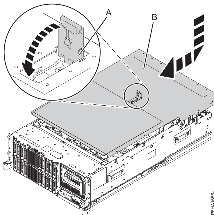
Figura 43. Instalando a Tampa de Acesso de Serviço
