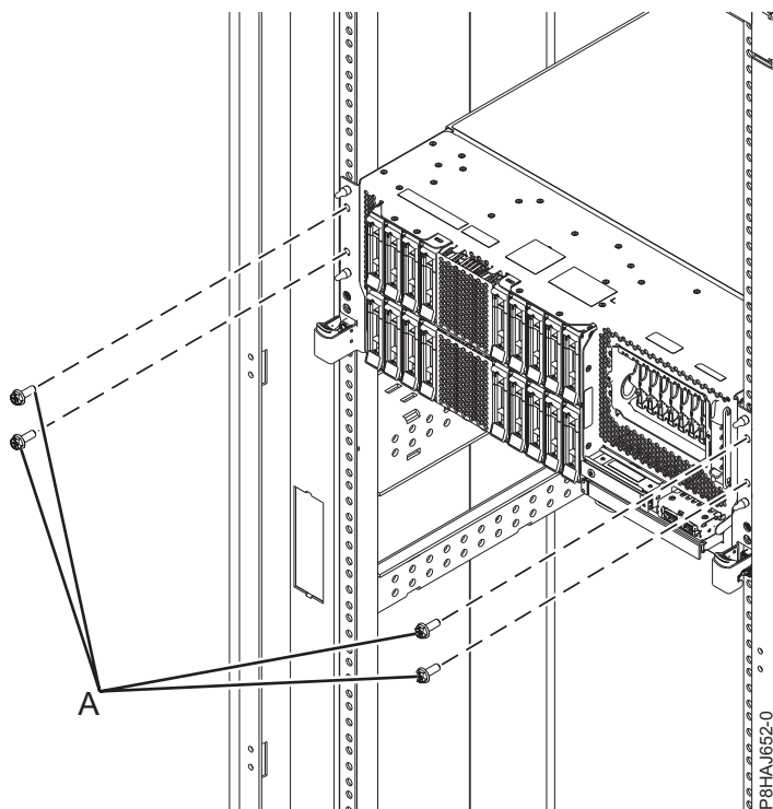
Figura 49. Removendo os parafusos frontais
