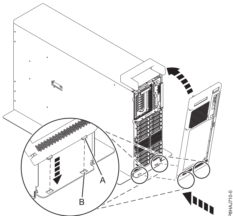
Figura 35. Instalando a Tampa Frontal
