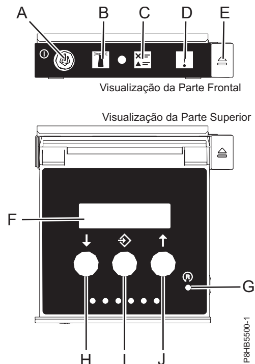
Figura 25. Painel de Controle
