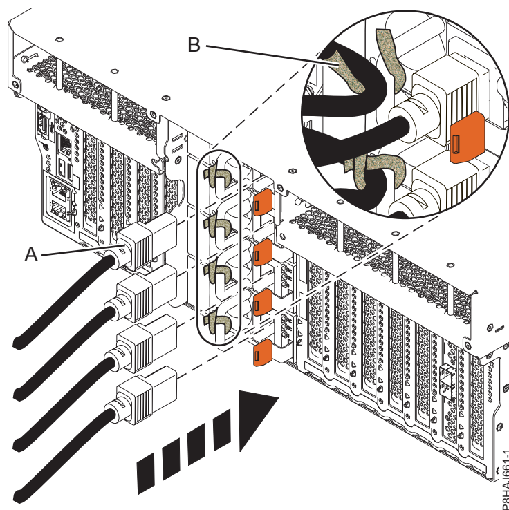
Figura 61. Conectando os cabos de energia a um sistema 8247-42L, 8286-41A ou 8286-42A
