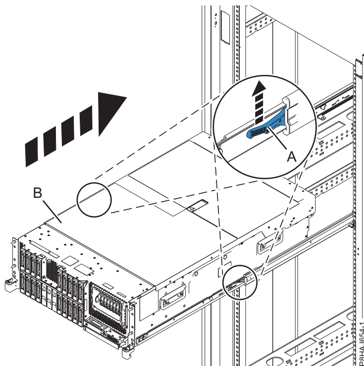
Figura 51. Colocando o Sistema na Posição de Operação
