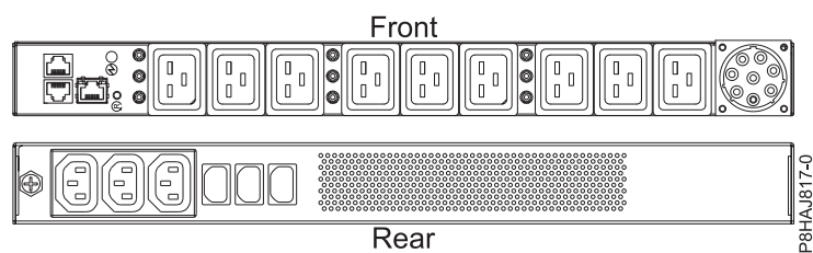
Figura 60. O PDU para o sistema 8408-44E
