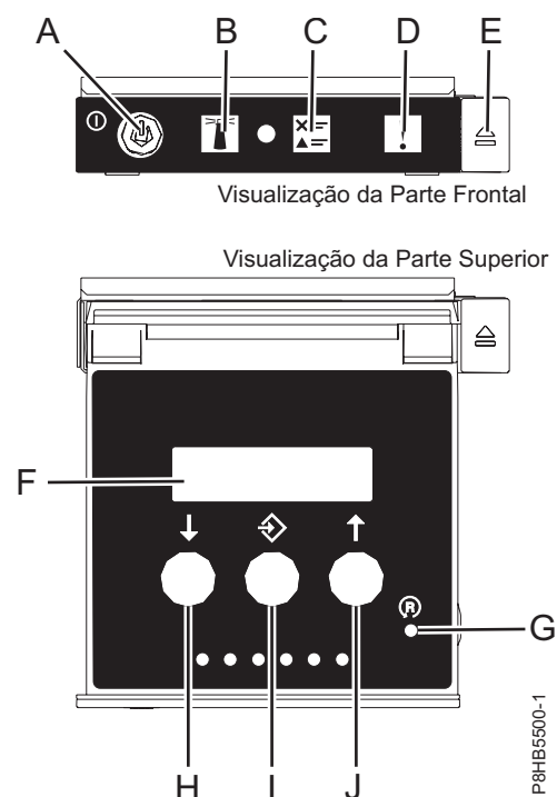
Figura 24. LEDs do Painel de Controle
