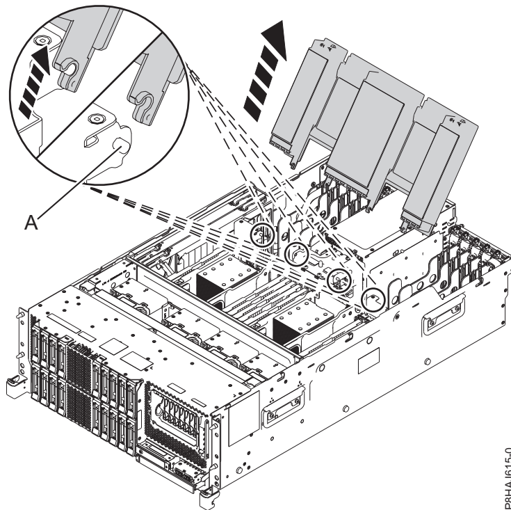
Figura 47. Removendo a placa defletora de ar
