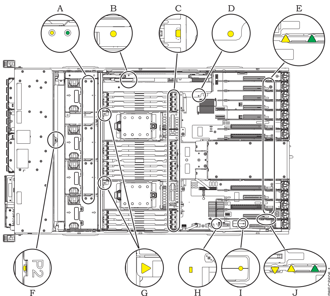
Figura 1. LEDs do indicador de serviço
