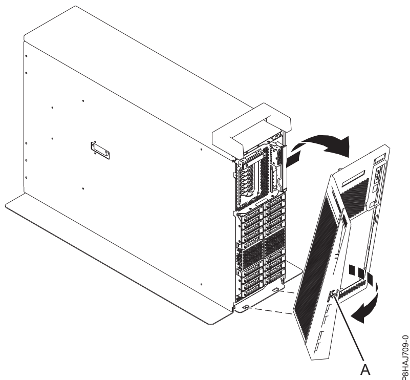
Figura 26. Removendo a Tampa Frontal
