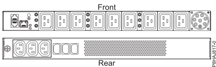
Figura 58. O PDU para o sistema 8408-44E
