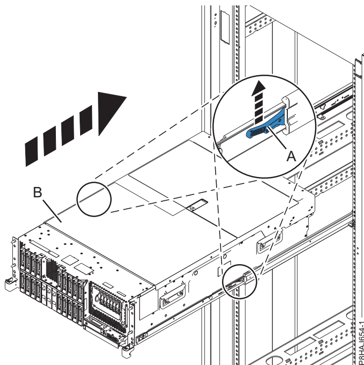
Figura 49. Colocando o Sistema na Posição de Operação
