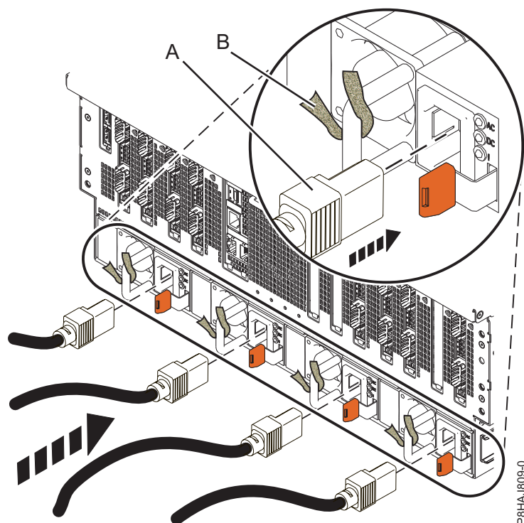
Figura 61. Conectando os cabos de energia a um sistema 8408-44E ou 8408-E8E
