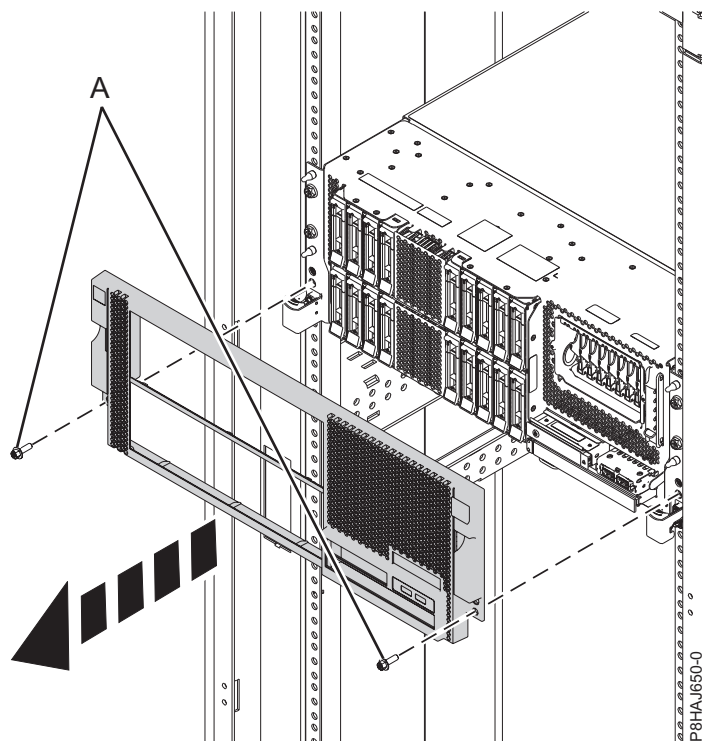
Figura 25. Removendo a Tampa Frontal
