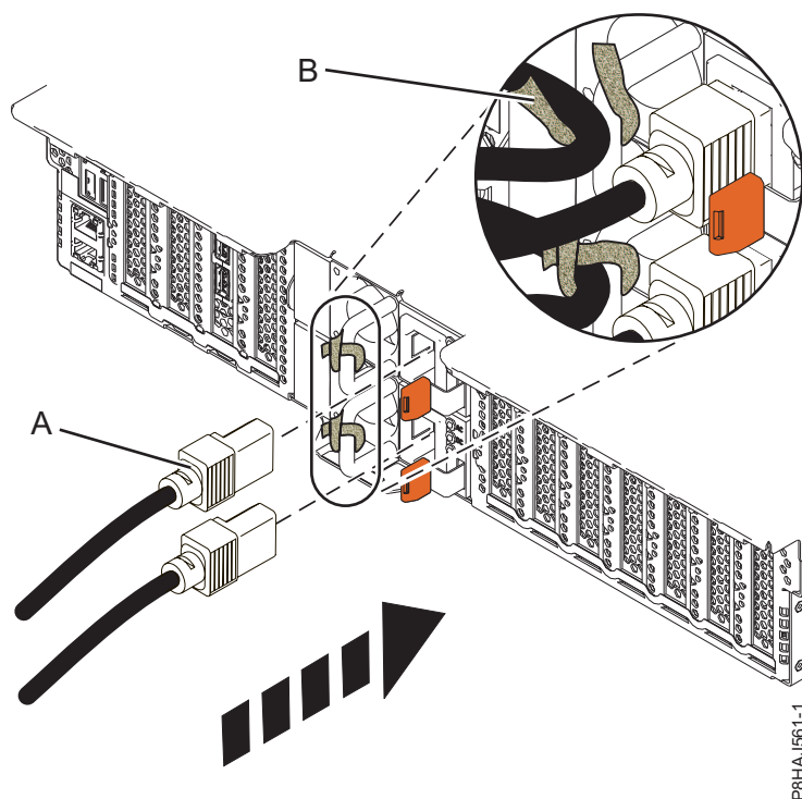
Figura 60. Conectando os cabos de energia a um sistema 5148-21L, 5148-22L, 8247-21L, 8247-22L, 8284-21A ou 8284-22A
