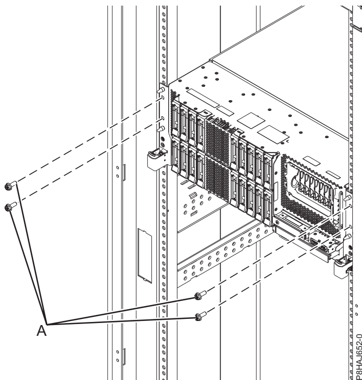
Figura 47. Removendo os parafusos frontais
