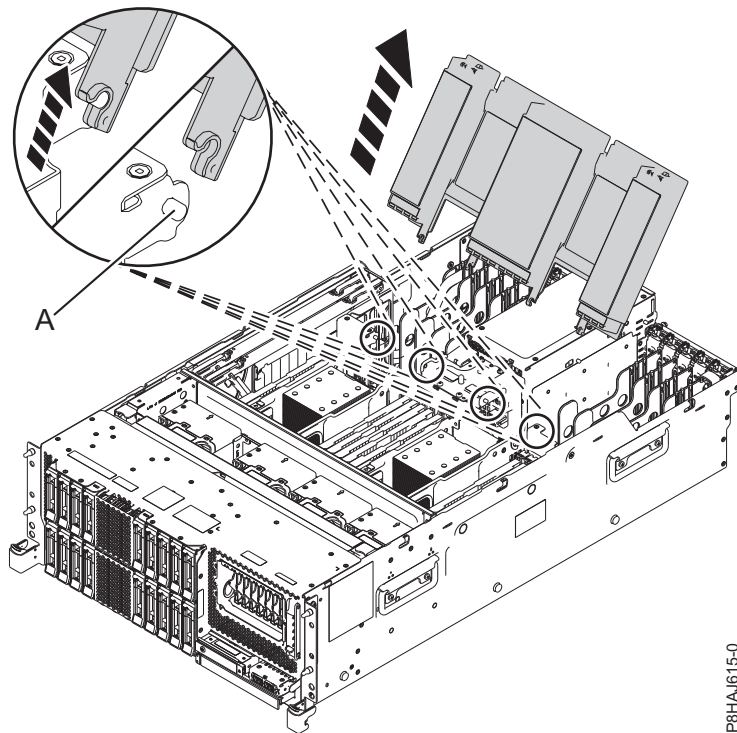
Figura 45. Removendo a placa defletora de ar
