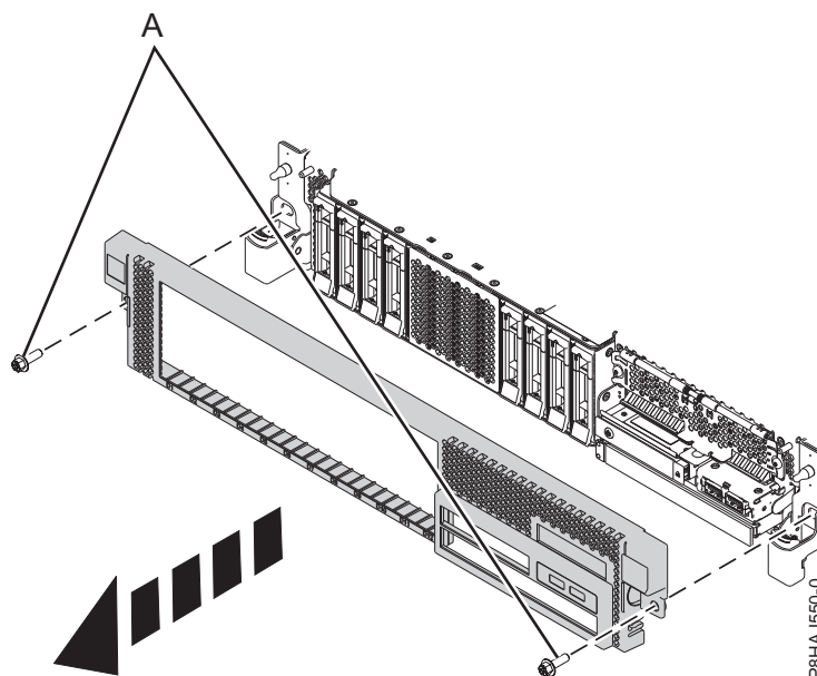
Figura 24. Removendo a Tampa Frontal
