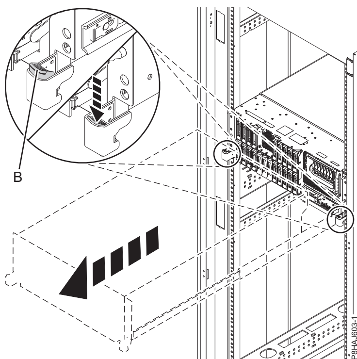
Figura 48. Liberando as Travas Laterais
