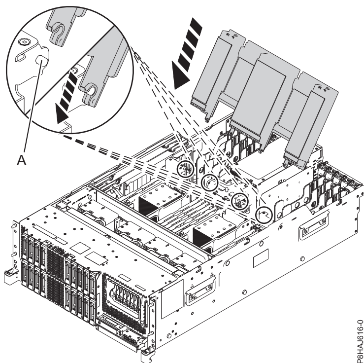
Figura 46. Substituindo a placa defletora de ar
