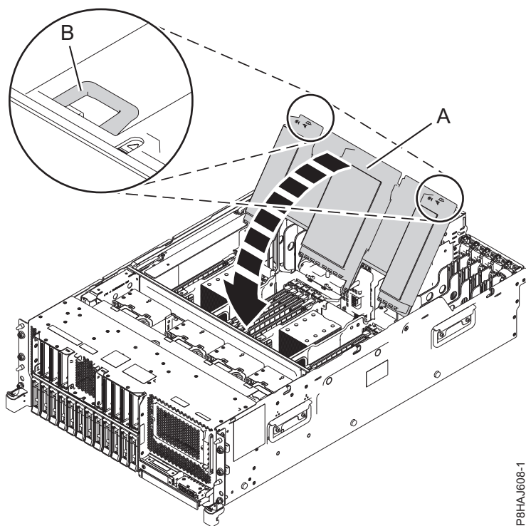
Figura 44. Fechando a placa defletora de ar
