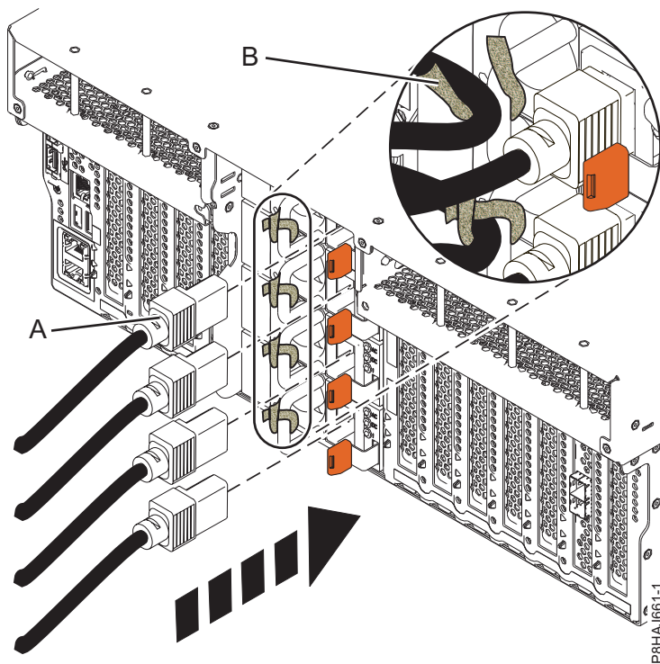
Figura 59. Conectando os cabos de energia a um sistema 8247-42L, 8286-41A ou 8286-42A
