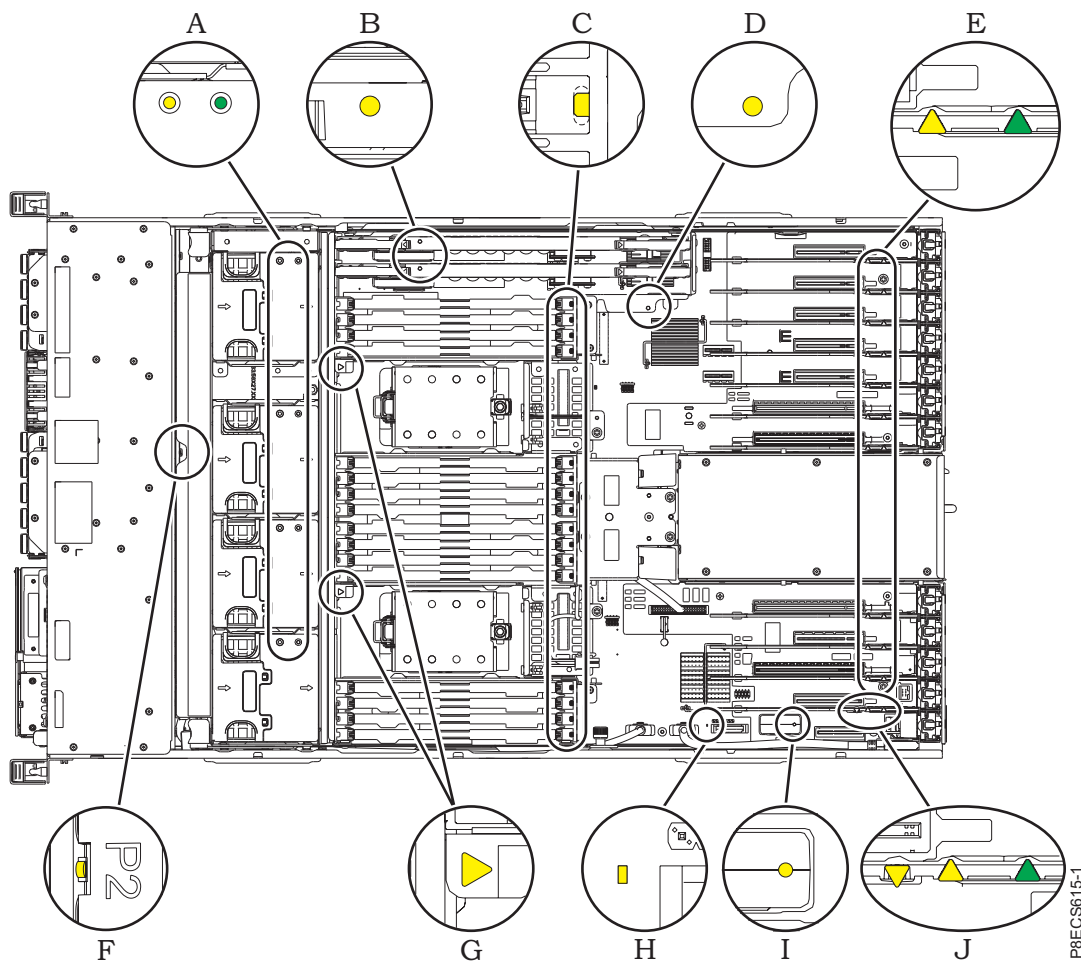
Figura 12. LEDs do indicador de serviço
