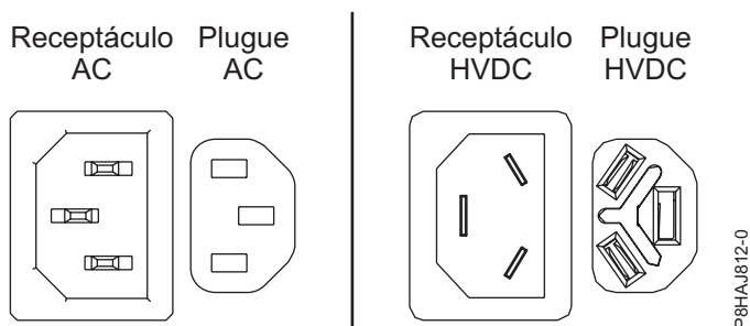
Figura 56. Conectores AC e HVDC
