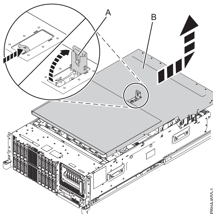
Figura 39. Removendo a Tampa de Acesso de Serviço
