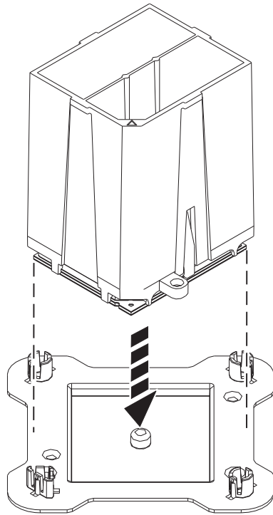
Figura 10. Colocando o Módulo de Processador do Sistema na Tampa Superior da Embalagem
