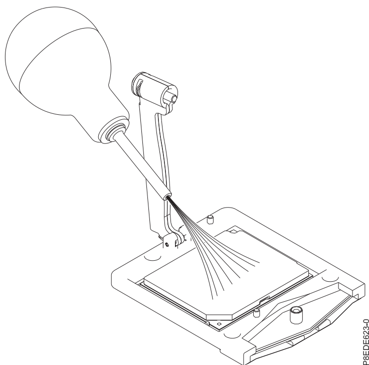
Figura 7. Limpando a Área do Módulo de Processador do sistema
