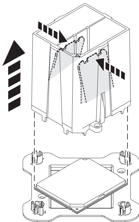
Figura 11. Liberando o módulo de processador do sistema da ferramenta
