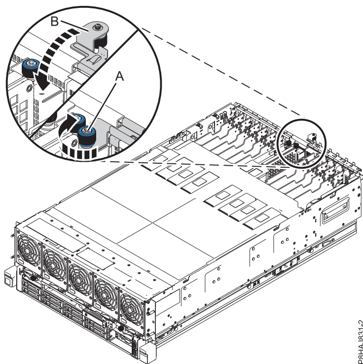
Figura 31. Fechando a trava de E/S
