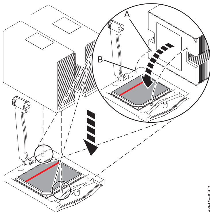
Figura 19. Instalando o dissipador de calor
