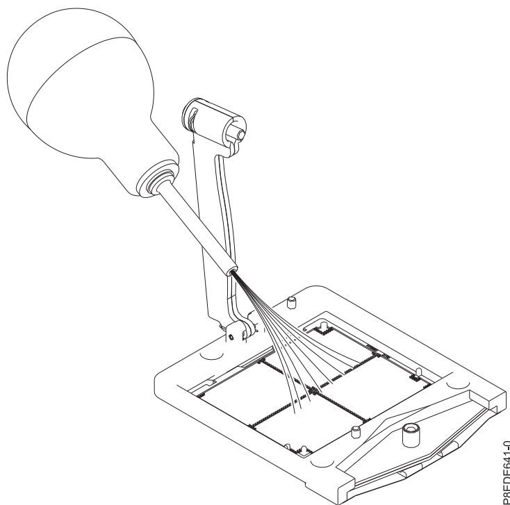
Figura 15. Removendo poeira e fragmentos do soquete do processador do sistema
