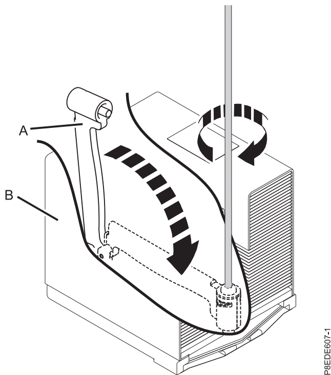
Figura 20. Apertando o Parafuso do Braço de Carregamento
