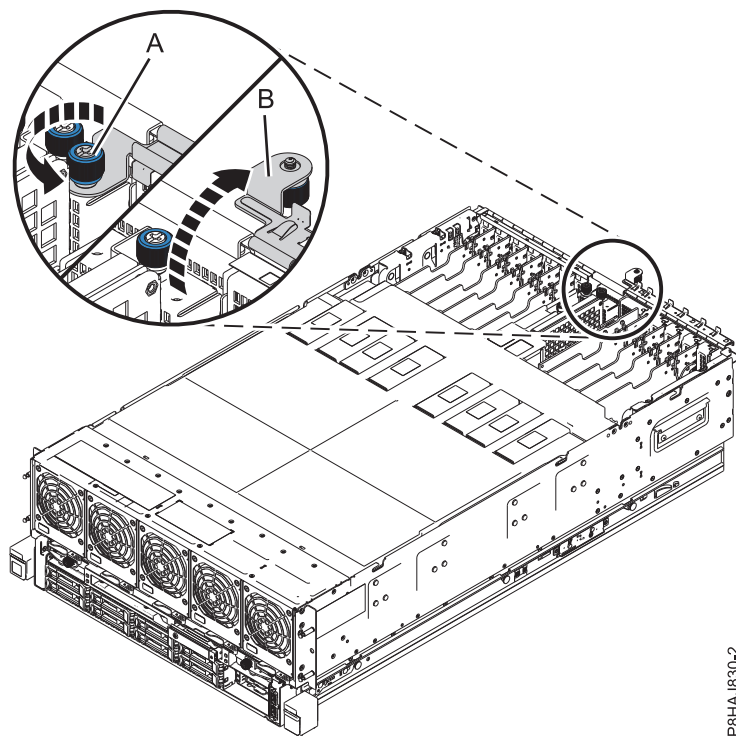
Figura 30. Abrindo a trava de E/S
