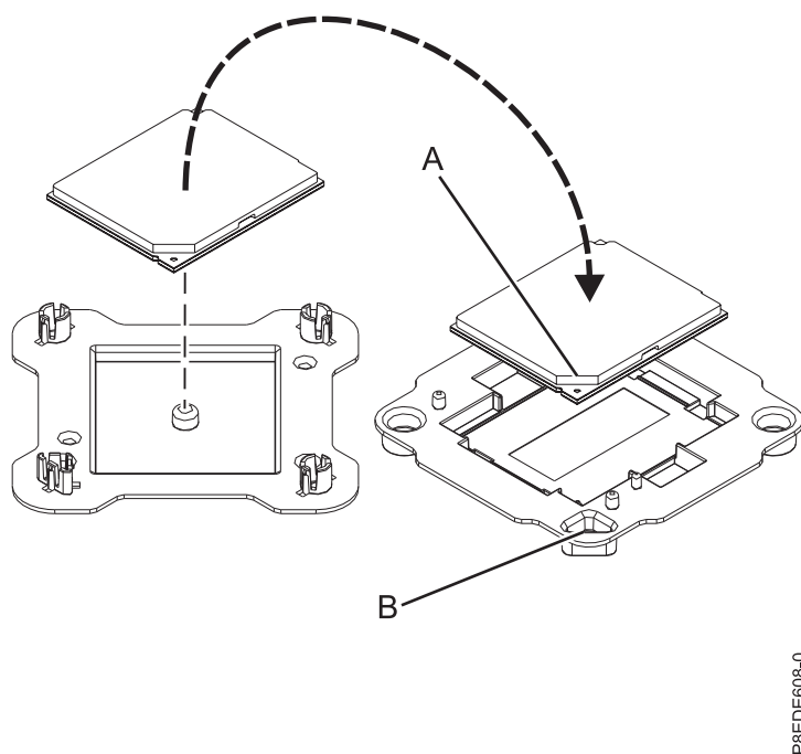
Figura 21. Colocando o Módulo do Processador do Sistema na Bandeja de remessa
