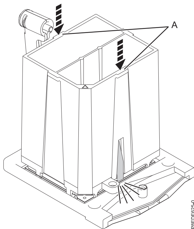
Figura 9. Bloqueando o Módulo de Processador do Sistema na Ferramenta de Remoção
