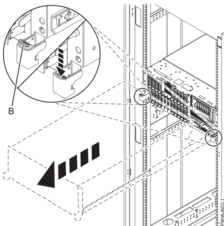
Figura 72. Liberando as Travas Laterais
