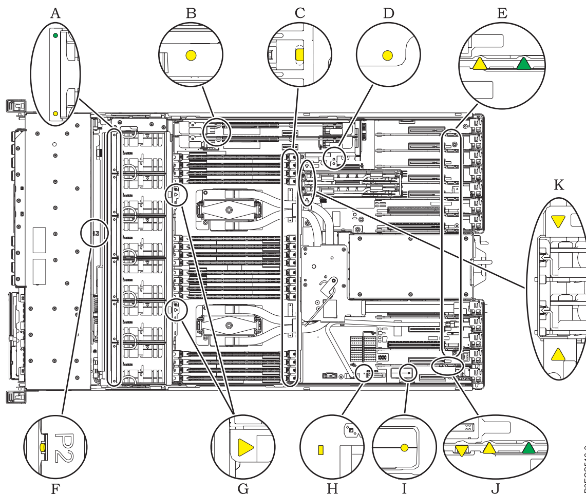
Figura 22. LEDs indicadores de serviço
