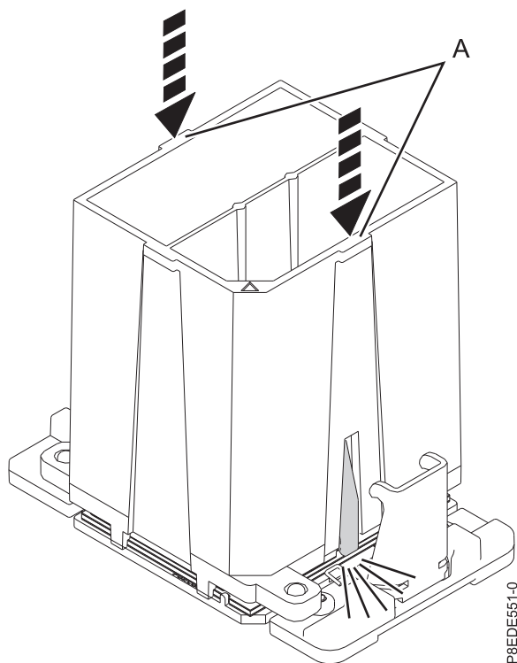
Figura 30. Bloqueando o módulo de processador do sistema na ferramenta
