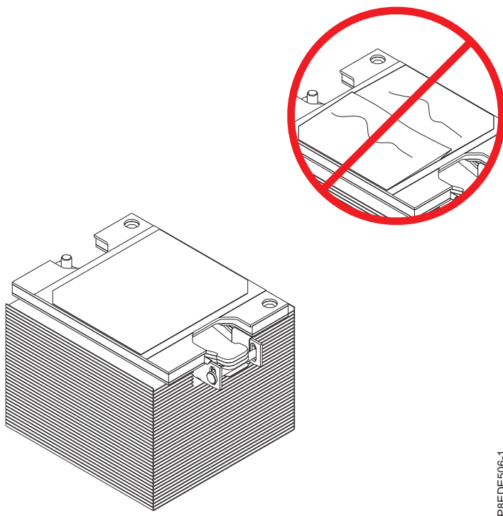
Figura 16. Inspeccionando o material da interface térmica
