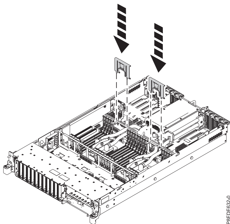
Figura 44. Abaixando as placas defletoras na posição
