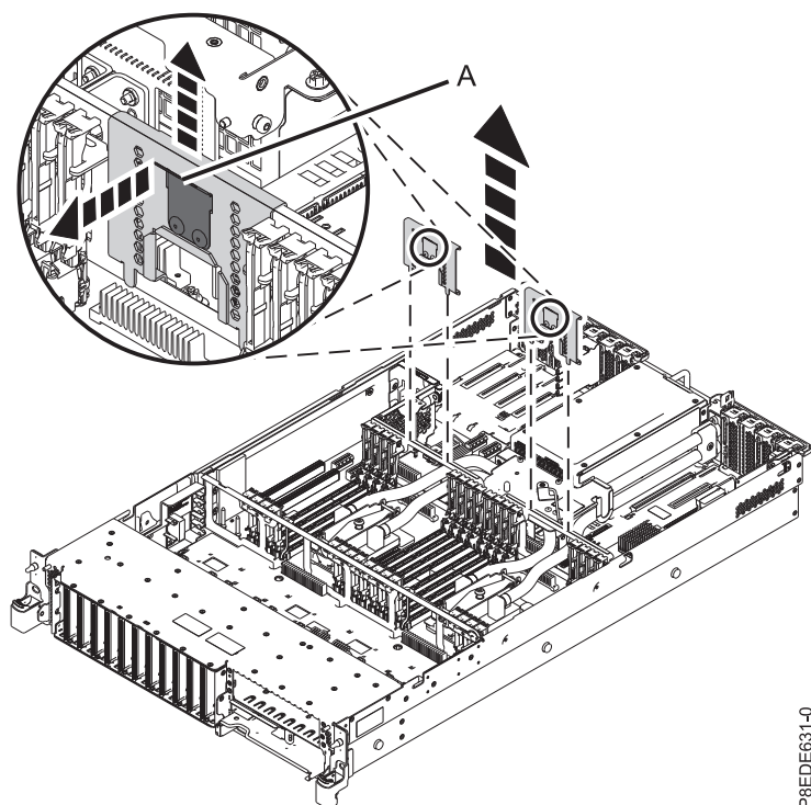
Figura 24. Removendo a placa defletora
