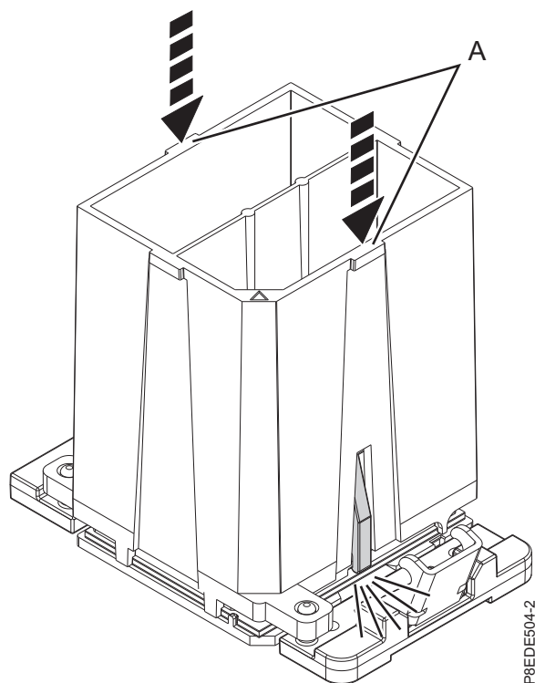
Figura 7. Bloqueando o módulo de processador do sistema na ferramenta
