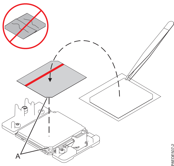
Figura 17. Instalando o TIM na tampa do processador
