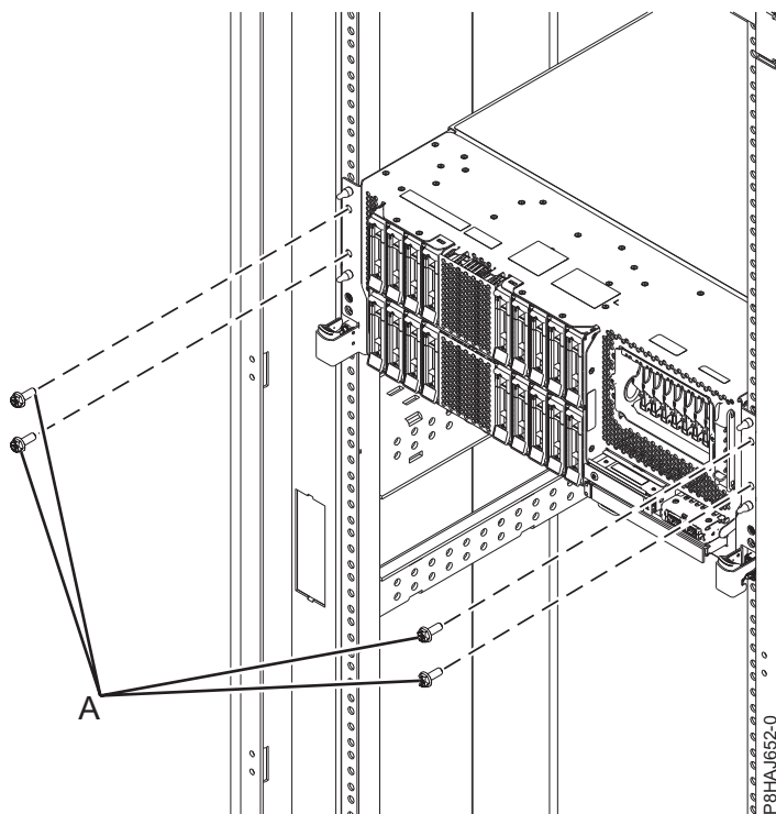
Figura 71. Removendo os parafusos frontais
