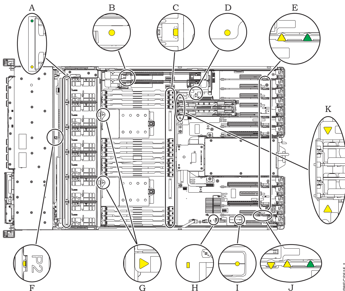
Figura 1. LEDs indicadores de serviço
