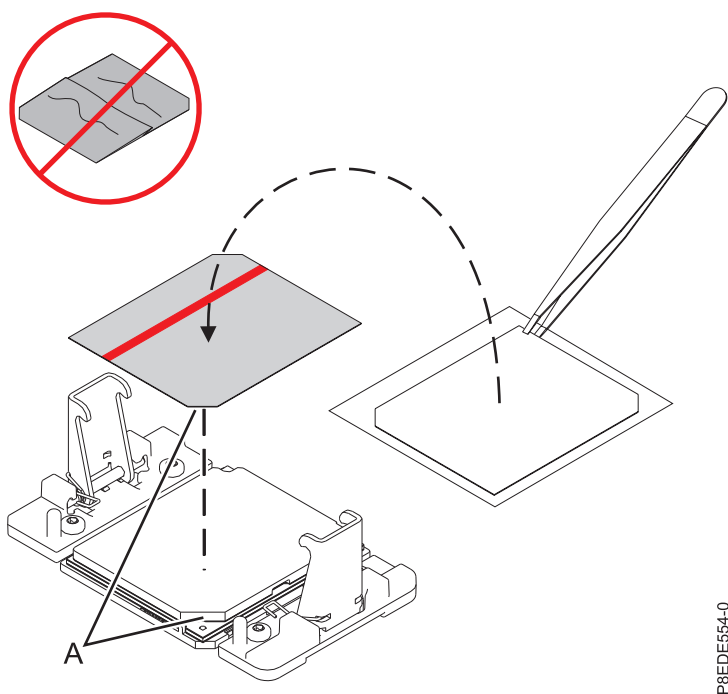
Figura 40. Substituindo o material da interface térmica (TIM)
