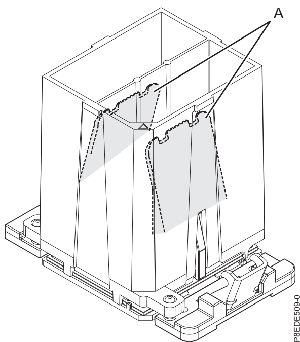
Figura 15. Removendo a ferramenta do módulo de processador do sistema
