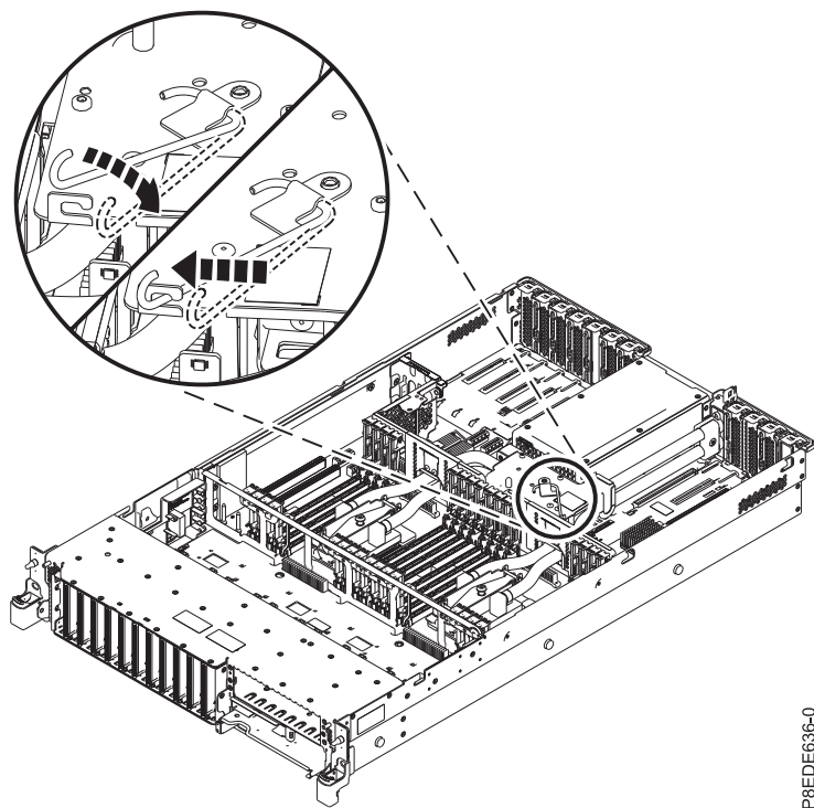
Figura 43. Retornando o gancho de serviço para a posição travada
