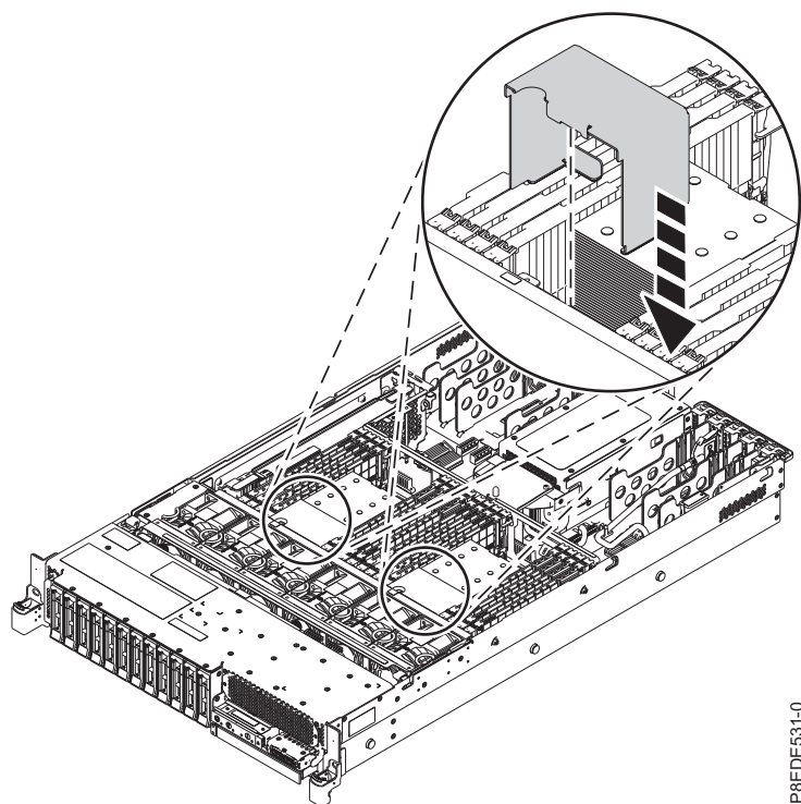
Figura 20. Substituindo a placa defletora de ar
