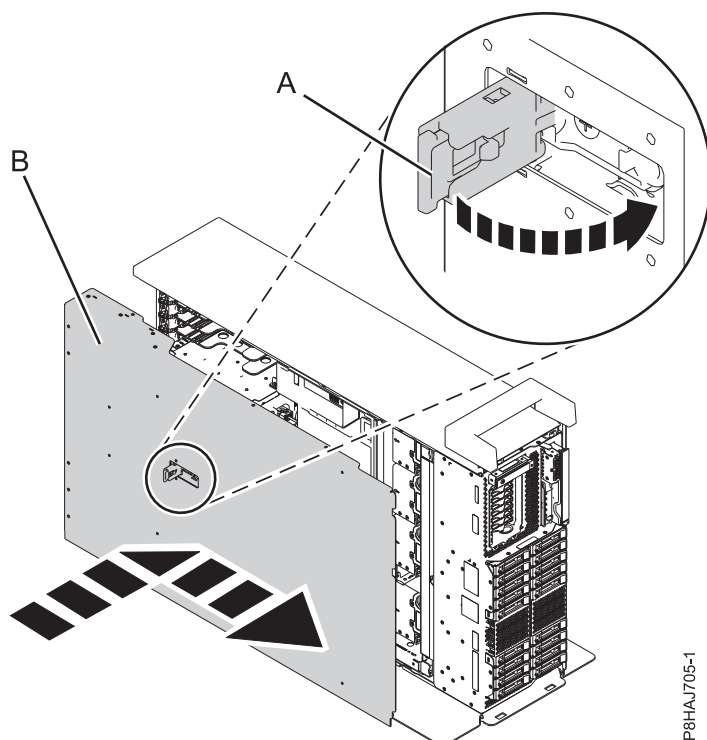
Figura 66. Instalando a Tampa de Acesso de Serviço
