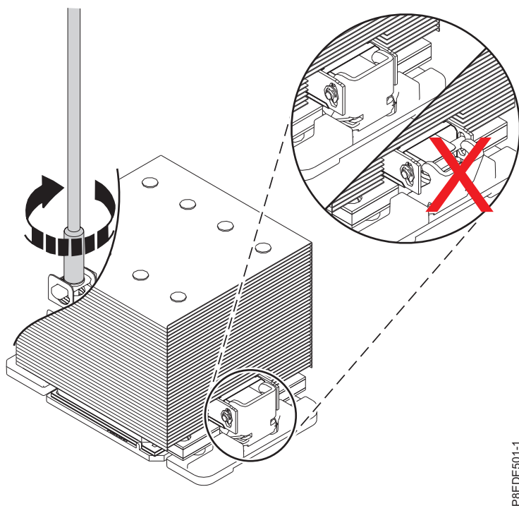
Figura 19. Fixando o dissipador de calor
