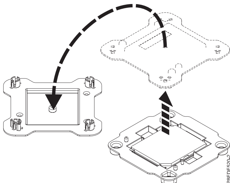
Figura 23. Abrindo a embalagem do módulo de processador do sistema
