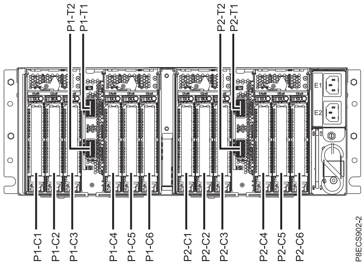
Figura 1. Vista posterior de um Gaveta de expansão PCIe3 EMX0 com códigos de local dos slots do PCIe
