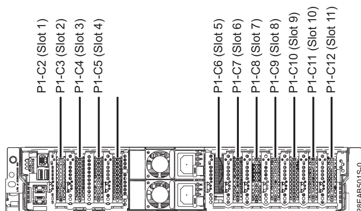
Figura 1. Vista posterior de um sistema 5148-21L, 5148-22L, 8247-21L, 8247-22L, 8284-21A ou 8284-22A com códigos de local dos slots PCIe
