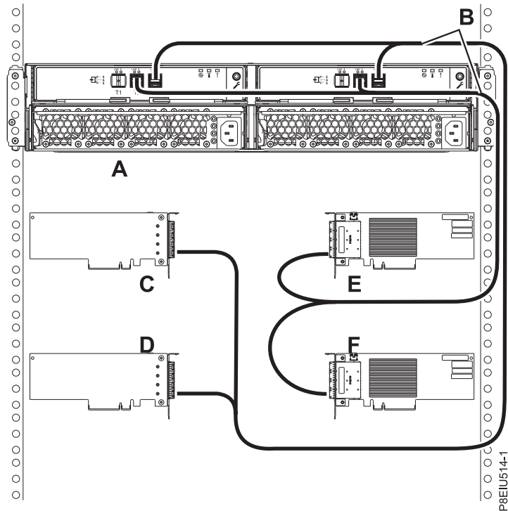
Rysunek 97. Połączenie trybu 4 jednej obudowy pamięci masowej ESLL lub ESLS z czterema niezależnymi adapterami SAS przy użyciu kabli X12
