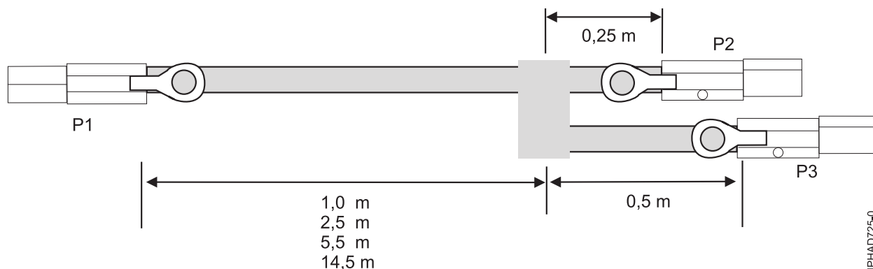
Rysunek 54. Długości kabli w zestawie zewnętrznych kabli YO do adapterów SAS
