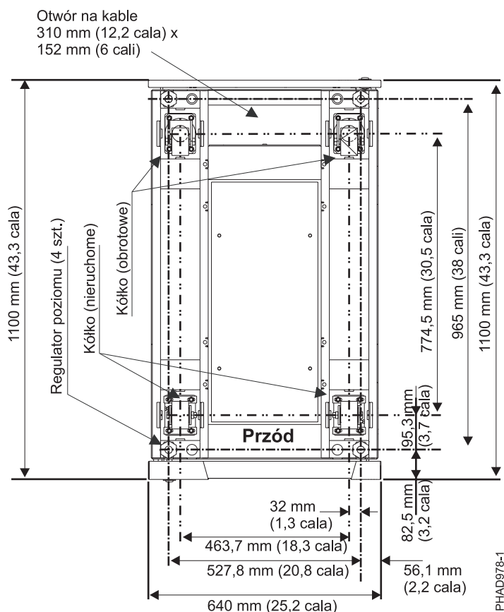
Rysunek 23. Miejsce kółek i regulatora poziomu
