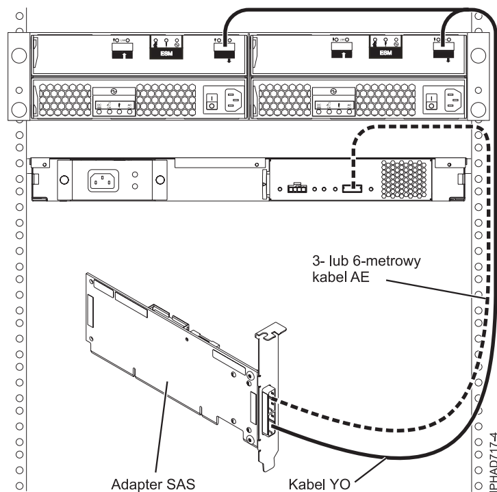
Rysunek 61. Podłączanie adaptera SAS do szuflady rozszerzeń dysków i szuflady rozszerzeń nośników
