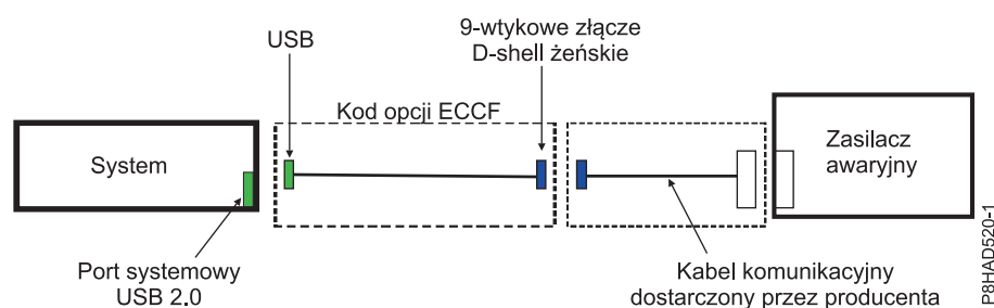
Rysunek 45. Okablowanie zasilacza UPS dla serwerów 5148-21L, 5148-22L, 8247-21L, 8247-21L, 8247-22L, 8247-42L, 8284-22A, 8286-41A i 8286-42A
