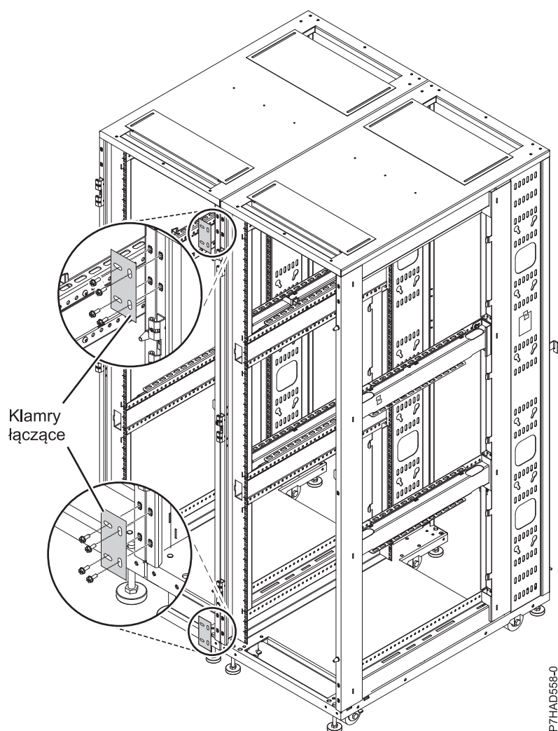
Rysunek 31. Klamry łączące
