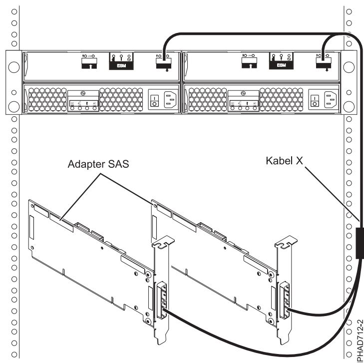
Rysunek 65. Podłączenie dwóch adapterów SAS RAID do szuflady rozszerzeń dysków w konfiguracji HA RAID z wieloma inicjatorami
