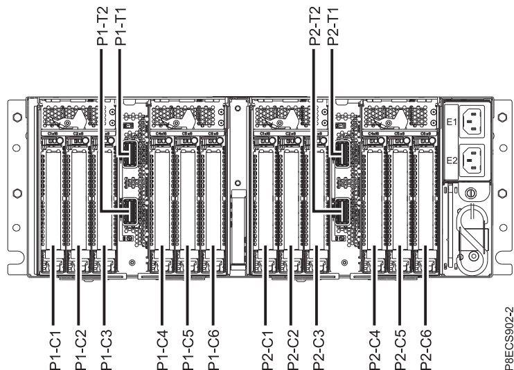
Rysunek 1. Widok z tyłu szuflady rozszerzeń EMX0 PCIe3 z kodami położenia gniazd PCIe
