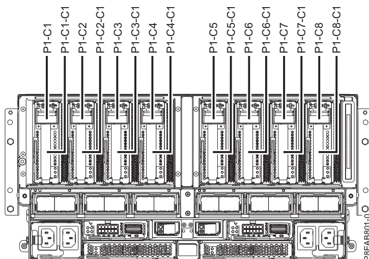
Rysunek 1. Widok z tyłu serwera 9080-MHE, 9080-MME, 9119-MHE lub 9119-MME z kodami położenia gniazd PCIe
